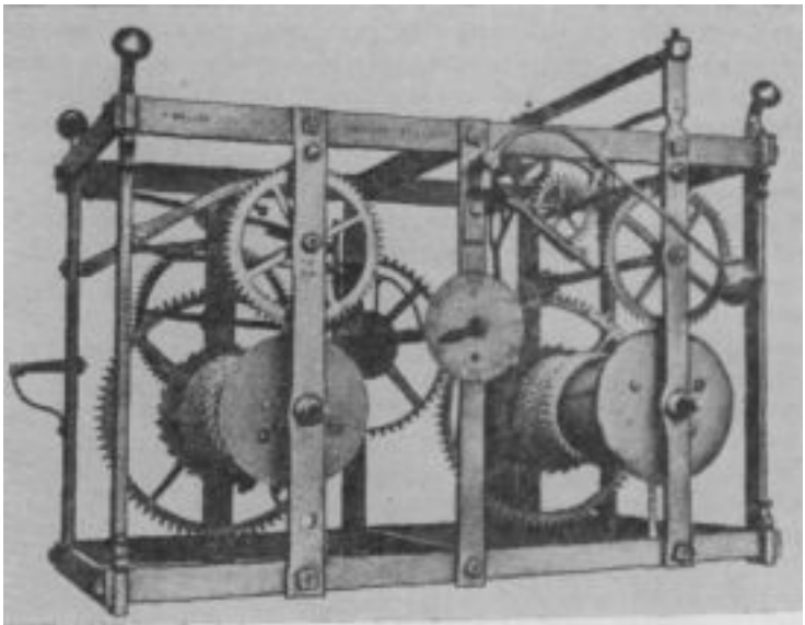
Рис. 137. Башенные часы Клемента 1671 г.
