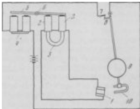
Рис. 235. Часы Гиппа, усовершенствованные Лемуаном
