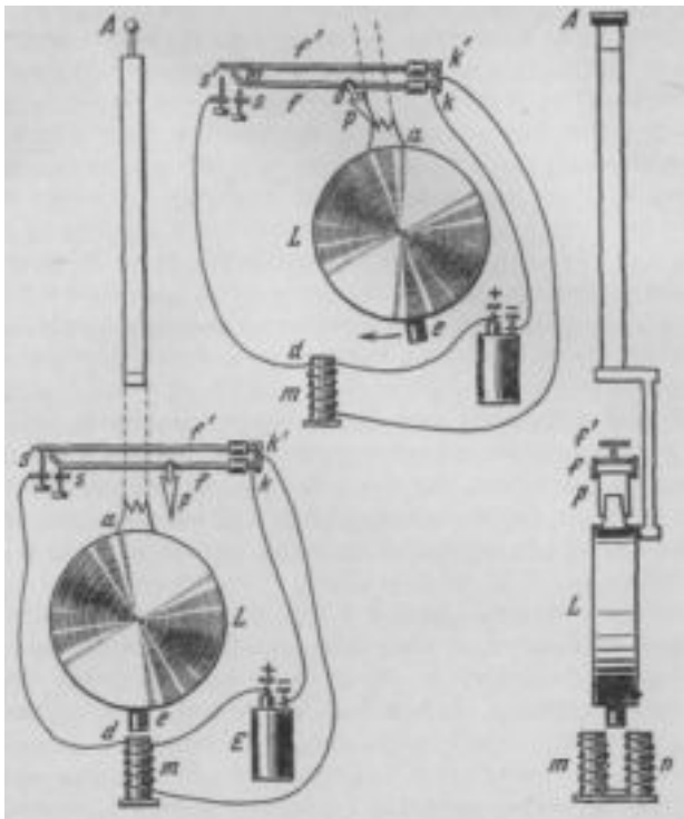
Рис. 234. Электрические маятниковые часы Гиппа
