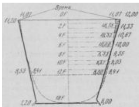
Рис. 10. Египетские водяные часы в виде конусообразной алебастровой чаши
