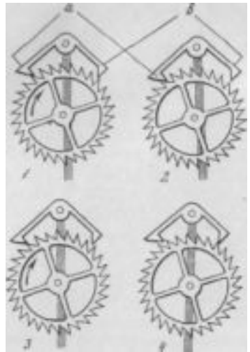
Рис. 135. Крючковый, или возвратный, ход Клемента
