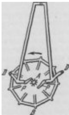
Рис. 146. Последовательность работы пружины в ходе Рифлера
