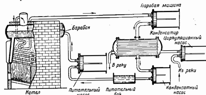
Фиг. 49. Схема паросиловой установки.
