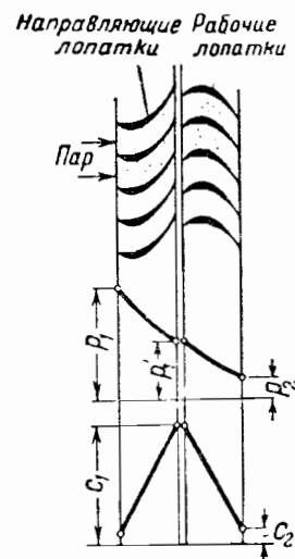
Фиг. 108. График изменения скорости и давления для реактивной турбины.
