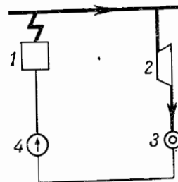
Фиг. 145. Схема паро-силовой установки, имеющей турбину с противодавлением.
