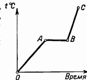
Фиг. 37. Ход изменения температуры по времени в процессе парообразования.
