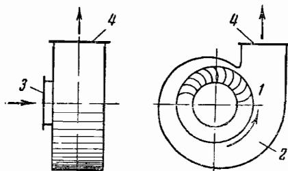
Фиг. 83. Схема центробежного вентилятора. 1—диск с лопатками; 2—кожух; 3—всасывающее отверстие; 4—нагнетательное отверстие.
