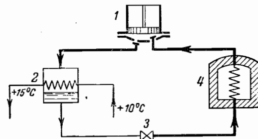
Фиг. 50. Схема холодильной установки.
