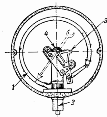
Фиг. 23. Манометр с трубкой Бурдона.
