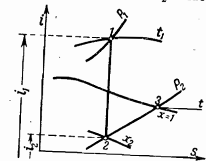
Фиг. 118. is -диаграмма адиабатного расширения пара в турбине.
