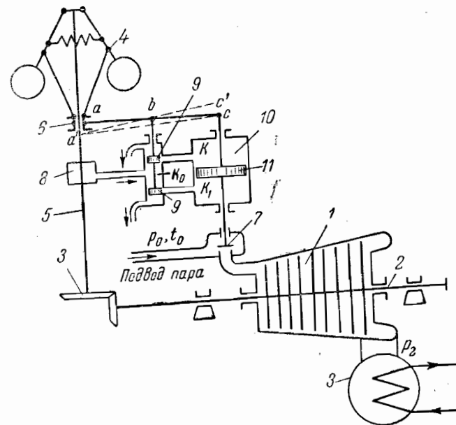
Фиг. 125. Схема непрямого регулирования паровой турбины. 1 — паровая турбина; 2 — вал ее; 3 — конденсатор; 4 — центробежный регулятор; 5 — вал регулятора; 6 — муфта регулятора; 7 — регулирующий клапан; 8 — масляный насос; 9 — золотники; 10 — исполнительный механизм регулятора; 11 — поршень исполнительного механизма.
