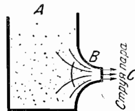
Фиг. 103. Истечение пара.
