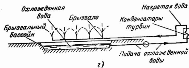
Фиг. 152. Схема водоснабжения для конденсаторов на электростанциях.
