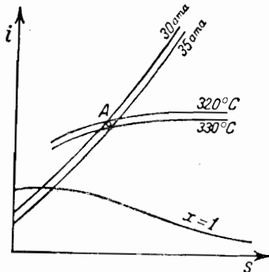
Фиг. 48. Нахождение состояния пара при отсутствии в i -с-диаграмме кривых заданных параметров.
