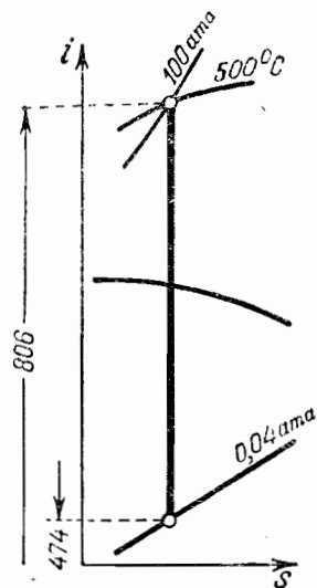
Фиг. 138. Адиабатный процесс в is -диаграмме.
