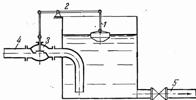
Фиг. 87. Схема регулирования питания водой резервуара. 1 — поплавок; 2 — рычаг; 3 — регулирующий клапан; 4 — питательная линия; 5 — задвижка.
