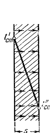
Фиг. 59. Тепловой поток через однослойную плоскую стенку.
