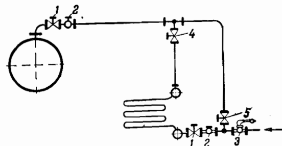
Фиг. 86. Схема питания котла.
