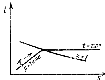
Фиг. 44. Определение температуры влажного пара в i -диаграмме.
