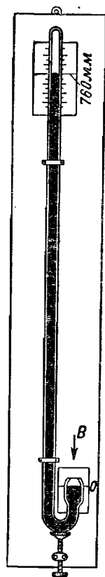
Фиг. 18. Ртутный барометр.
