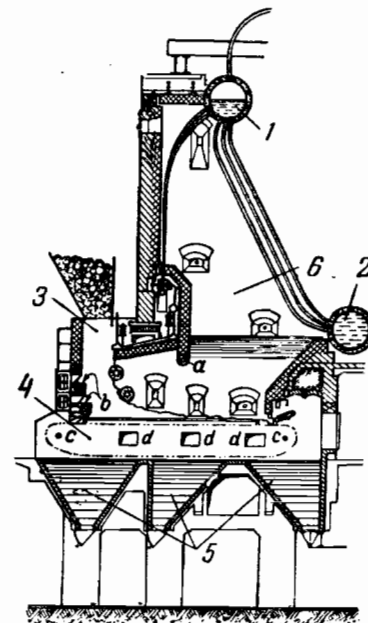
Фиг. 67. Топка проф. Т. Ф. Макарьева для фрезерного топлива. 1 и 2 — барабаны котла; 3 — шахта; 4 — цепная решетка; 5 — золовые бункеры; 6 — топочное пространство; a — балка; b — ступени; c — звездочки; d — короба для воздуха.
