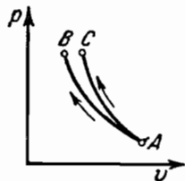
Фиг. 35. Относительное расположение изотермы и адиабаты (сжатие).
