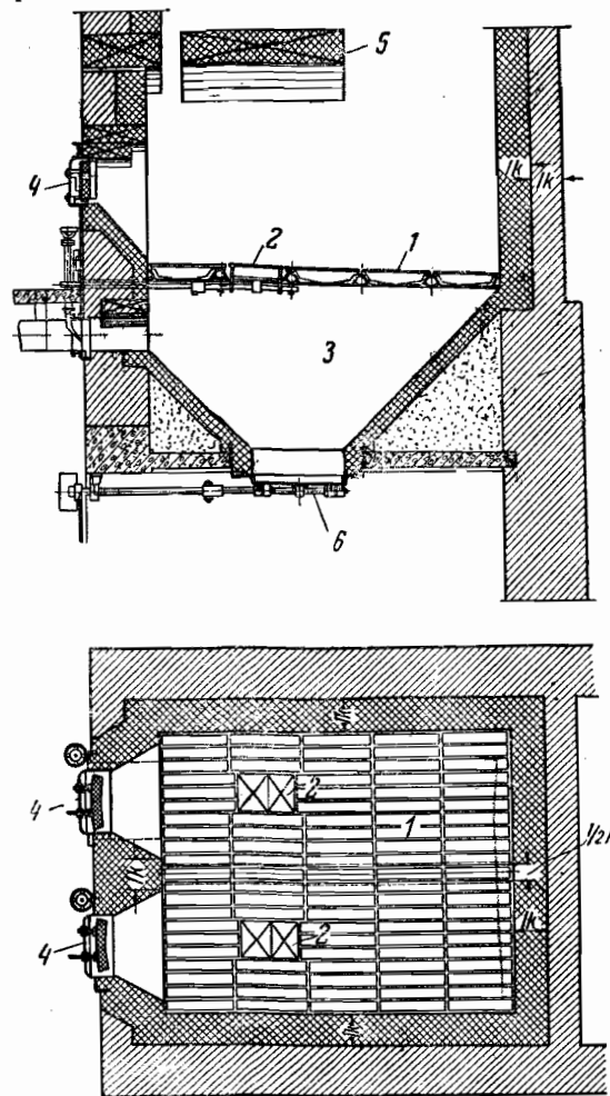
Фиг. 66. Ручная колосниковая решетка для бурого угля.
