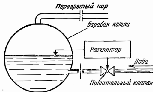
Фиг. 88. Схема одноимпульсного регулятора питания.
