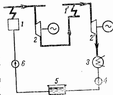
Фиг. 143. Схема паросиловой установки со вторичным перегревом пара.
