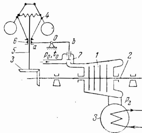
Фиг. 123. Схема прямого регулирования. 1 — паровая турбина; 2 — вал ее; 3 — конденсатор; 4 — центробежный регулятор; 5 — вал регулятора; 6 — муфта регулятора; 7 — регулирующий клапан.
