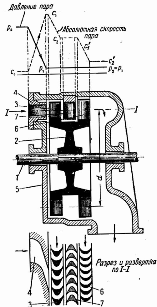
Фиг. 109. Разрез по активной турбине со ступенями скорости.
