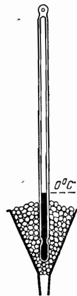
Фиг. 8. Определение нулевой точки на термометре ( 0^\circ \text{C} ).
