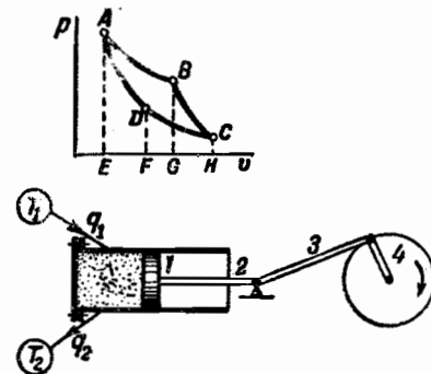
Фиг. 51. Цикл Карно
