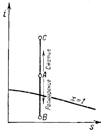
Фиг. 45. Адиабатный процесс в i -диаграмме.
