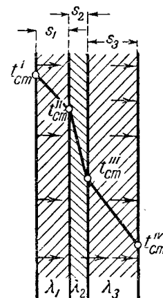
Фиг. 60. Тепловой поток через многослойную плоскую стенку.
