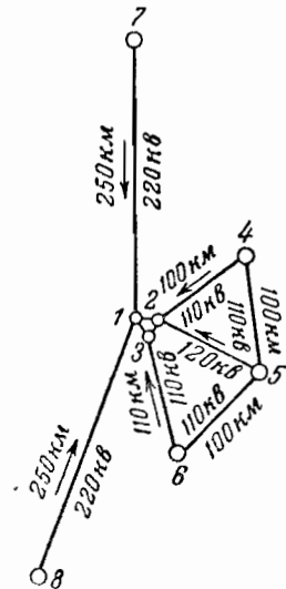
Фиг. 153. Схема расположения станций и сетей (первый тип).
