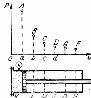
Фиг. 26. Изображение последовательных изменений состояния газа в цилиндре.
