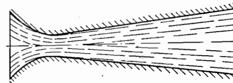
Фиг. 104. Расширяющееся сопло.
