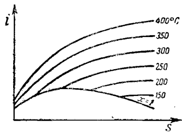
Фиг. 42. Изотермы в i -диаграмме.
