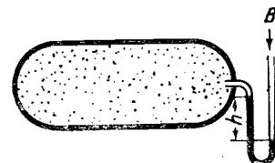
Фиг. 20. Измерение разрежения газа в сосуде.
