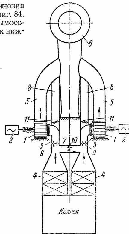
Фиг. 85. Схема дымососной установки котельного агрегата (с двумя дымососами).
