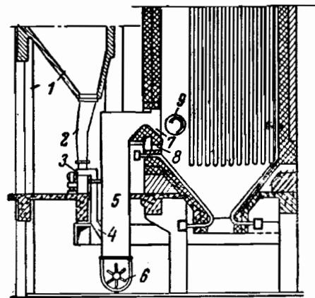
Фиг. 70. Шахтно-мельничная топка.
