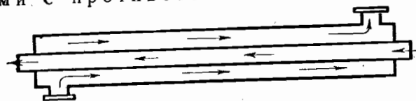
Фиг. 56. Теплообменный аппарат с противотоком.
