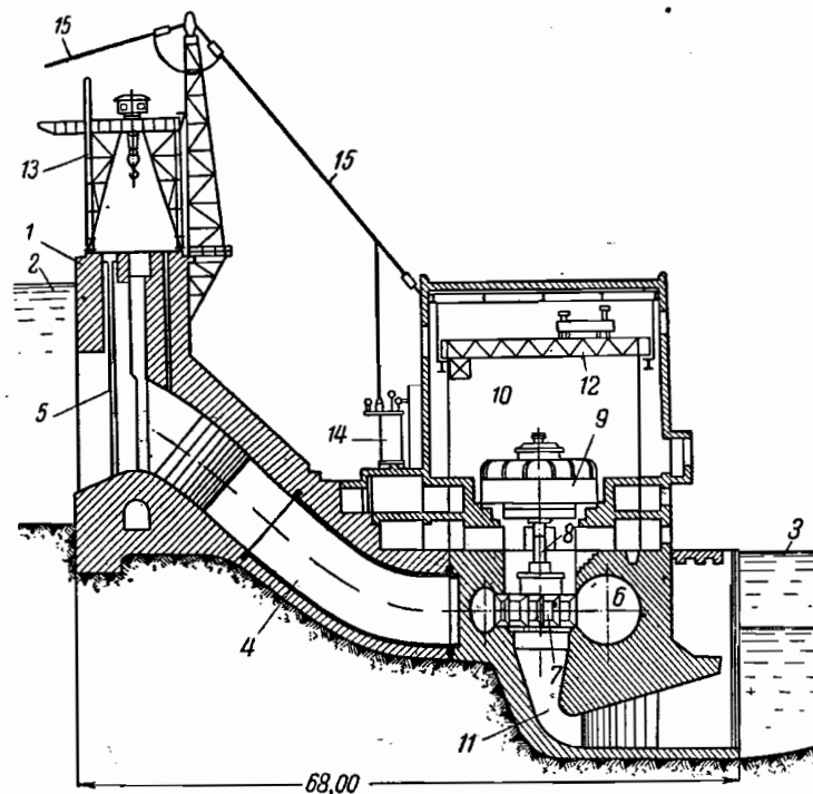
Фиг. 1. Схематический чертеж гидравлической электрической станции. 1 — плотина; 2 — верхний уровень воды в реке; 3 — нижний уровень воды; 4 — напорный трубопровод; 5 — водозапорные щиты; 6 — спиральная камера; 7 — рабочее колесо турбины; 8 — вал турбины; 9 — генератор электрического тока; 10 — машинный зал; 11 — отсасывающая труба; 12 — подъемный кран для разбора агрегата; 13 — подъемный кран для водозапорных щитов; 14 — повышающий трансформатор; 15 — линия высокого напряжения.
