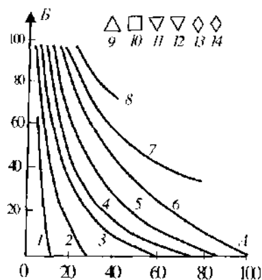
Рис. 18.10. Номограмма для определения удельной поверхности S_{уд} сополимеров стирола с ДВБ, синтезированных в среде n -гептана (А - содержание ДВБ в смеси мономеров в %; Б - количество добавляемого n -гептана в % по отношению к смеси полимеров) ( S_{уд} - в м²/г):
