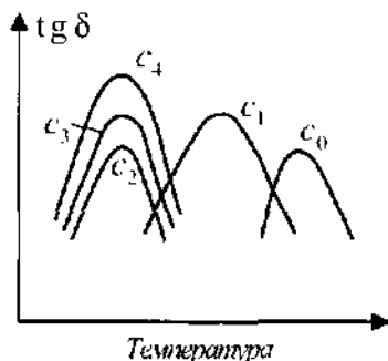
Рис. 16.11. Изменение \operatorname{tg} \delta при межструктурной пластификации ( C_4 > C_3 > C_2 > C_1 > C_0 ).
