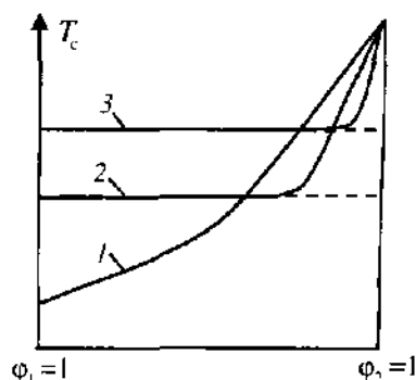
Рис. 16.7. Изменение T_c при внутриструктурной (1) и межструктурной (2,3) пластификации.
