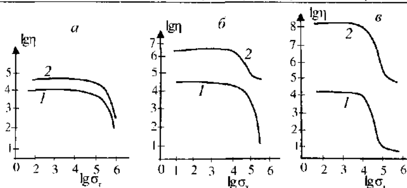
Рис. 13.16. Кривые течения концентрированных растворов полиизобутилена ( а ), полистирола ( б ) и ацетата целлюлозы ( в ) в хорошем (1) и плохом (2) растворителях.
