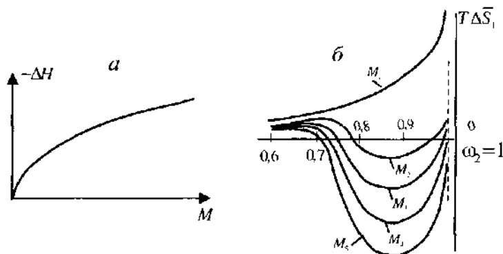
Рис. 11.16. Влияние молекулярной массы полимера на теплоту (а) и энтропию (б) смешения ( M_1 < M_2 < M_3 < M_4 < M_5 ).
