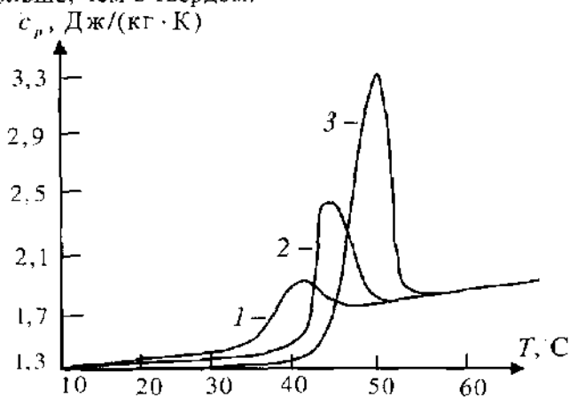
Рис.6.4. Зависимость удельной теплоемкости поливинилацетата от температуры при различных скоростях нагревания: 1 – 0.1 °C/мин; 2 – 0.4 °C/мин; 3 – 1.5 °C/мин.
