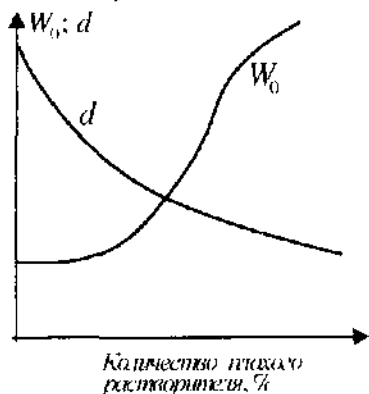
Рис. 18.11. Влияние количества добавленного в реакционную смесь плохого растворителя на суммарный объем пор и плотность сополимера.
