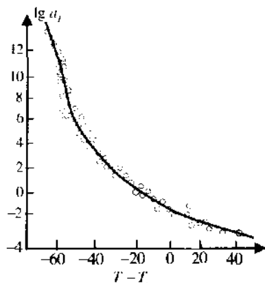
Рис. 5.10. Зависимость \lg a_T от T - T_s для полимеров.
