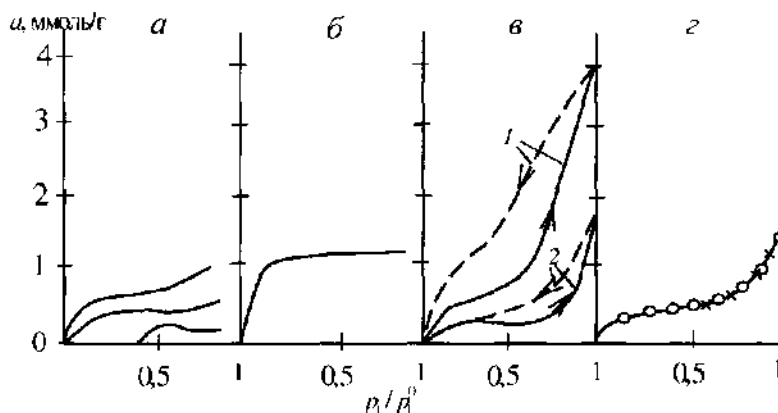
Рис. 18.3. Изотермы сорбции паров "инертных" жидкостей на полимерах: а — непористые (1 — ПВС; 2 — ПВХ; 3 — ПС); б — микропористые; в — сорбенты с переходными порами (1 — сополимер стирола с дивинилбензолом, синтезированный в среде растворителя; 2 — полиакрилат (сплошные кривые — сорбция, пунктирные — десорбция); г — макропористые (О — пленка стирофлекс; х — макропористая пленка ПС).
