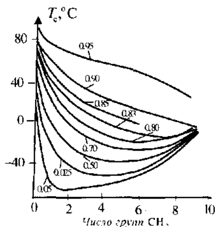
Рис. 16.13. Зависимость T_c полистирола от длины алкильного радикала в молекуле фталата (числа у кривых — кажущаяся массовая доля ПС).
