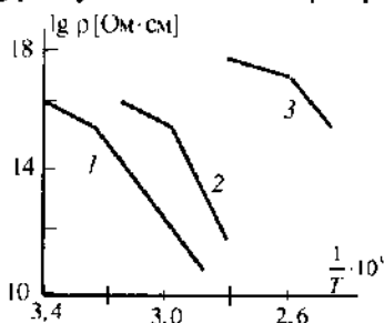
Рис. 9.1. Зависимость удельного электрического сопротивления \rho от температуры для некоторых полимеров:
