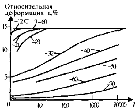
Рис. 5.4. Временная зависимость высокоэластической деформации вулканизатов каучука при различных температурах.
