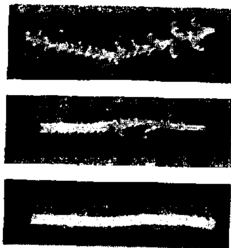
Рис. 8.6. Вид струи стереорегулярного каучука, вытекающего из капиллярной насадки при высоких напряжениях сдвига.
