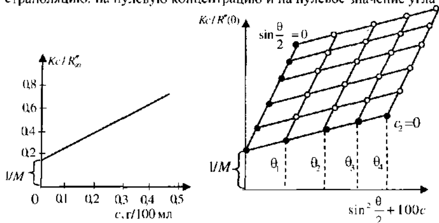
Рис. 14.4. Зависимость Kc_2/R''_{90} от концентрации раствора.
