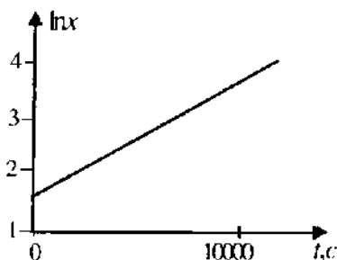
Рис. 14.10. График зависимости \ln x = f(t) .
