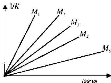
Рис. 14.8. Зависимость 1/K от времени для различных фракций полимера ( M_1 < M_2 < M_3 < M_4 < M_5 ).
