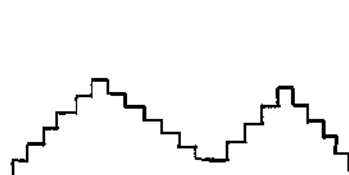
Рис. 2.9. Конформация цепи типа "коленчатый вал".
