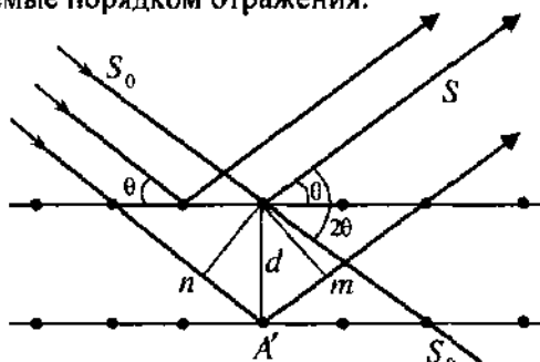
Рис. 3.1. Схема отражения лучей от одномерной структуры с периодом d ( S_0 – падающие лучи, S – дифрагированные; разность хода между лучами, отраженными от двух плоскостей, равная nA'M + mA'A = 2d \sin \theta ; угол между падающим и дифрагированным лучом равен 2\theta ).
