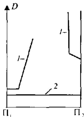
Рис. 17.1. Изменение оптической плотности D пленок смесей полимеров при добавлении к одному полимеру другого ( P_1 и P_2 ): 1 – несовместимые полимеры; 2 – совместимые полимеры.
