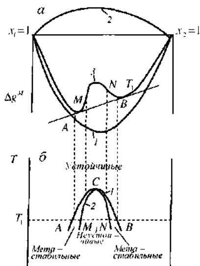
Рис. 11.7. Концентрационная зависимость средней свободной энергии смешения (а) и фазовое равновесие (б) ( ACB – бинодаль; MN – спинодаль).
