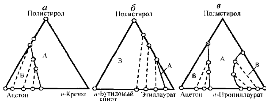
Рис. 10.8. Диаграмма состояния растворов полистирола:
