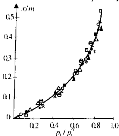
Рис. 18.5. Изотермы сорбции n -гексана высокоэластическими полимерами: ○ - ПК; × - СКБ; Δ - СКИ; □ - высокомолекулярная фракция СКИ; ▲ - СКБМ; ■ - высокомолекулярная фракция СКБМ; ● - СК - 1; ● - СК - 2; * - СК - 3.
