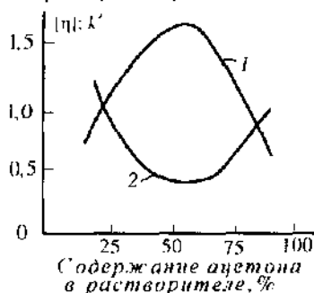
Рис. 13.4. Зависимость характеристической вязкости (1) и вискозиметрической константы k' (2) фракции полистирола от состава бинарной смеси растворителей (ацетон – метилциклогексан).
