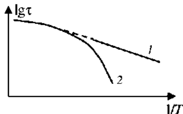
Рис. 9.6. Зависимость логарифма времени релаксации от обратной температуры:
