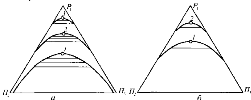
Рис. 17.12. Симметричные бинадали систем растворитель 1 – полимер 2 – полимер 3:
