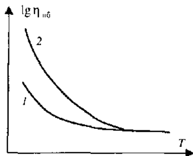
Рис. 13.11. Зависимость \eta_{\text{об}} от температуры для растворов полимеров в хороших (1) и плохих (2) растворителях.
