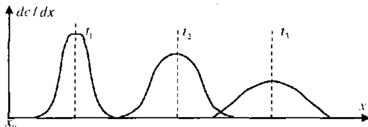
Рис. 14.9. Изменение градиента концентрации в процессе центрифугирования.
