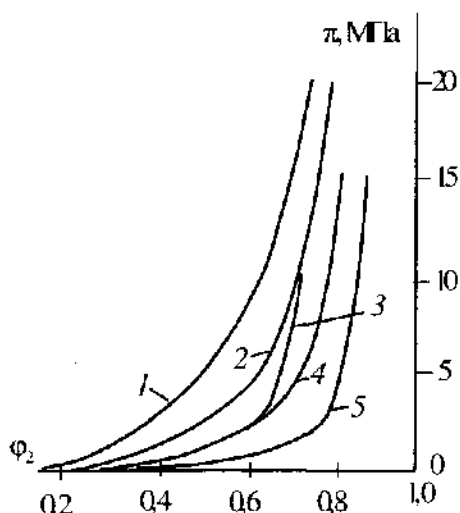
Рис. 11.18. Зависимость давления набухания при 25°C от объемной доли полимера в набухшем вулканизате натурального каучука: 1—декалин; 2— n -гексан; 3—гептан; 4—декан; 5—гексадекан.
