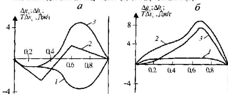
Рис. 17.10. Зависимость свободной энергии (1), энтальпии (2) и энтропии (3) смешения для систем ПВХ–ПММА (а) и ПММА–ПБМА (б).
