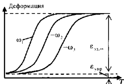
Рис. 5.8. Зависимость деформации полимеров от температуры при разных частотах воздействия ( \omega_1 < \omega_2 < \omega_3 ).
