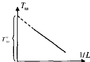
Рис. 4.7. Зависимость наблюдаемой температуры плавления T_{пл} от размера складки монокрystalла полимера.
