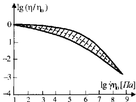
Рис. 8.10. Универсальная температурно-инвариантная вязкостная характеристика полидисперсных полимеров (пунктирная линия — усредненная зависимость).
