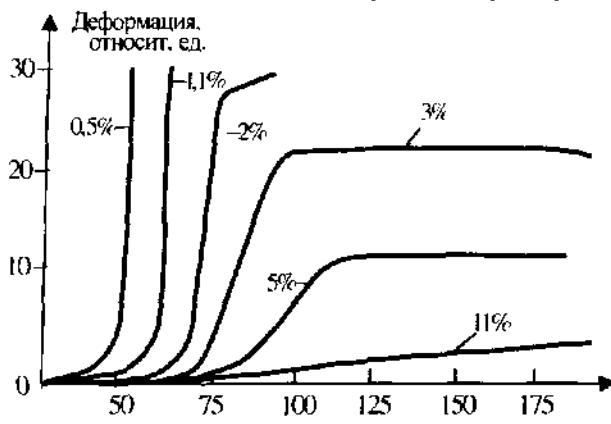
Рис. 6.14. Влияние содержания уротропина (цифры у кривых) на отверждение фенолоформальдегидных олигомеров.
