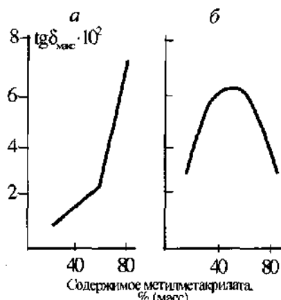
Рис. 9.10. Зависимость \text{tg } \delta_{\text{макс}} от соотношения метилметакрилата и стирола в сополимере:
