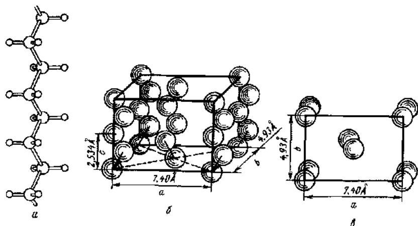
Рис. 3.5. Конформация цепи ( a ) и расположение цепей в кристаллографической ячейке полиэтилена ( б ); в — проекция решетки на плоскость ( ab ).
