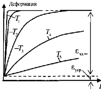
Рис. 5.5. Временная зависимость деформации полимеров при различных температурах ( T_1 > T_2 > T_3 > T_4 > T_5 ).
