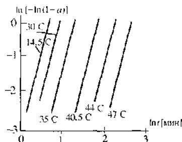
Рис. 4.4. Графики в координатах уравнения Авраами для процесса кристаллизации фракционированного полиэтилена-адилината при разных температурах.
