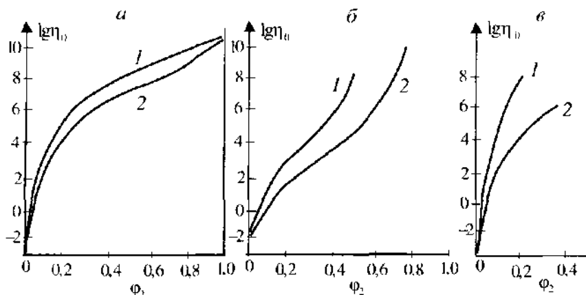
Рис. 13.10. Зависимость \lg \eta_0 от объемной доли полимера для растворов ПИБ ( a ), ПС ( б ) и АЦ ( в ) в плохих (1) и хороших (2) растворителях.
