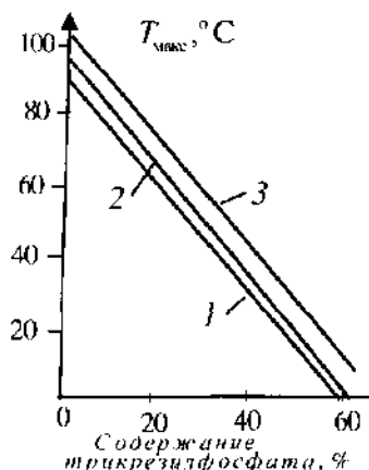
Рис. 16.12. Зависимость температуры, соответствующей максимуму дипольно-сегментальных потерь T_{\max} смесей поливинилхлорида, от концентрации трикрезилфосфата: 1—15 Гц; 2—260 Гц; 3—1000 Гц.
