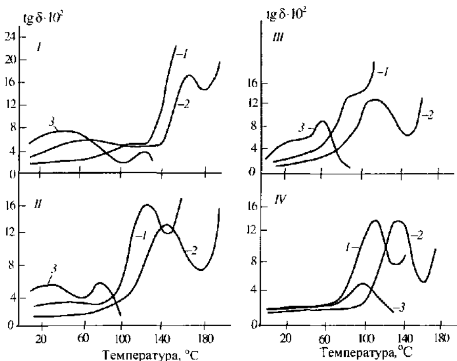
Рис. 9.8. Температурная зависимость \operatorname{tg} \delta для полимерных алкил- \alpha -хлоракрилатов (I – метил- \alpha -хлоракрилат; II – этил-; III – пропил-; IV – изобутил- \alpha -хлоракрилат); 1 – при 20 Гц; 2 – при 400 Гц; 3 – та же зависимость для полиалкил-метакрилата при 20 Гц.
