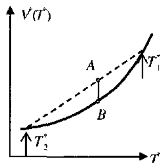
Рис. 12.8. Зависимость приведенного объема от приведенной температуры для жидких полимеромологов.
