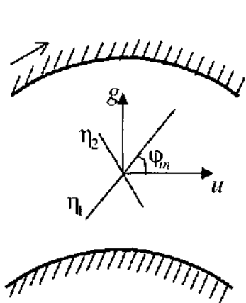
Рис. 14.13. Векторы скорости поступательного движения частиц и градиента скорости при динамооптических измерениях.
