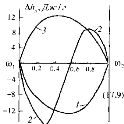
Рис. 17.8. Зависимость энтальпии смешения полимеров друг с другом от состава полимерной композиции:
