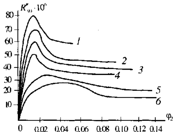
Рис. 15.5. Зависимость избыточного светорассеяния от объемной доли полимера – фракций ПС различной молекулярной массы в бензоле:
