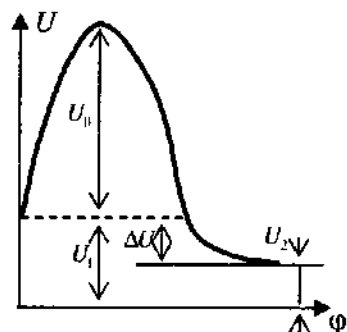
Рис. 2.15. Энергия активации вращения.
