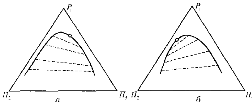
Рис. 17.13. Несимметричные бинодали систем растворитель 1 — полимер 2 — полимер 3: а: растворитель лучше смешивается с полимером P_2 ( \chi_{1,2} < \chi_{1,3} ); б: растворитель лучше смешивается с полимером P_3 ( \chi_{1,3} < \chi_{1,2} ).
