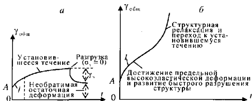
Рис.8.3. Развитие деформации во времени при низком (а) и высоком (б) постоянных напряжениях сдвига: ОА – условно-мгновенная деформация; I – развитие высокоэластической деформации и слабое разрушение структуры.
