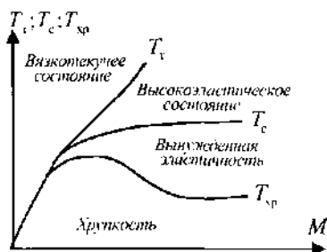
Рис. 7.10. Зависимость температур текучести, стеклования и хрупкости от молекулярной массы полимера.
