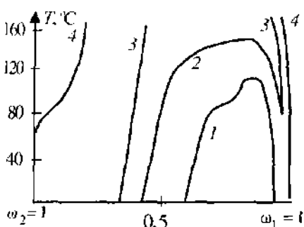
Рис. 17.14. Диаграмма состояния системы полиизобутилен – полидиметилсилоксан при разных соотношениях молекулярных масс смешиваемых полимеров:
