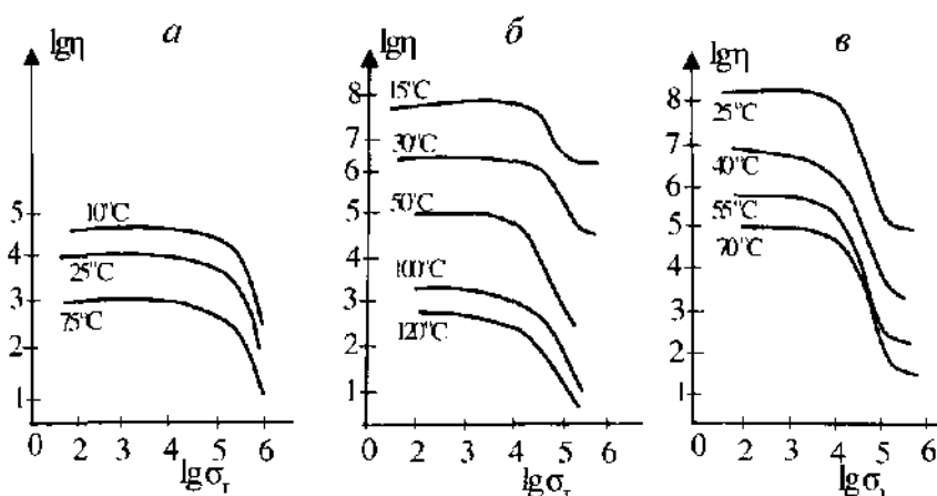
Рис. 13.17. Кривые течения растворов полиизобутилена ( а ), полистирола в плохом растворителе – декалине ( б ) и ацетата целлюлозы ( в ) при разных температурах.
