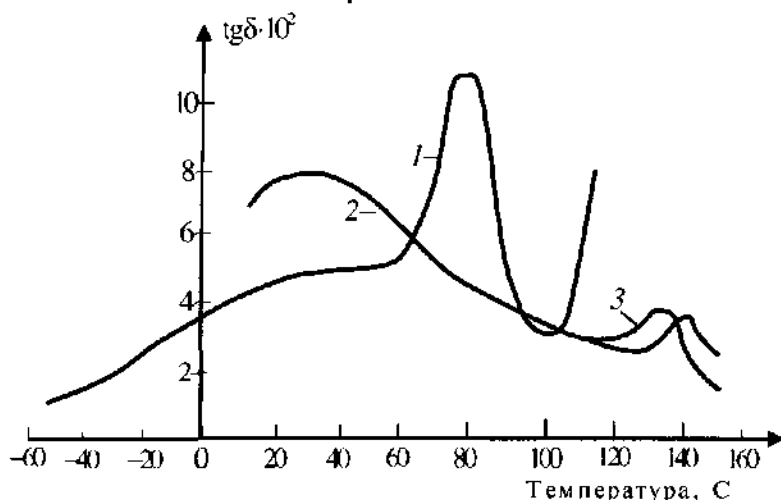
Рис. 9.11. Температурная зависимость стереорегулярных образцов полиметилметакрилата при 20 Гц:
