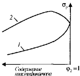
Рис. 16.8. Зависимость разрушающего напряжения при растяжении от содержания пластификатора при внутриструктурной (1) и межструктурной (2) пластификации.
