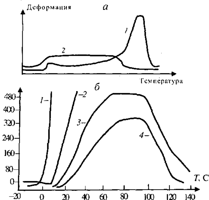
Рис. 6.13. Термомеханические кривые структурирующихся полимеров а – общий вид кривых; б – кривые для фенолоформальдегидных резольных смол, снятые в процессе поликонденсации.
