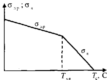
Рис. 7.7. График для определения температуры хрупкости.
