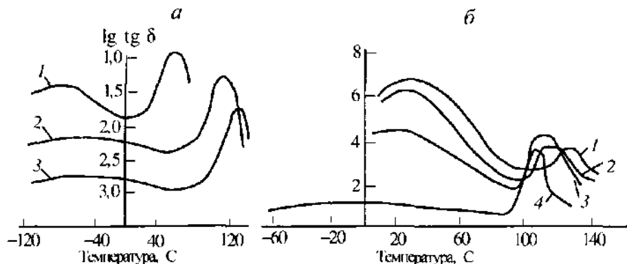
Рис. 9.9. Температурная зависимость \lg \delta сополимеров метилакрилата и метилметакрилата со стиролом:
