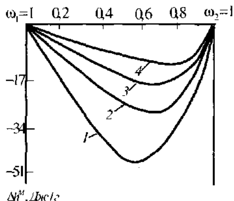
Рис. 11.8. Концентрационная зависимость средней энтальпии смешения: 1 – нитрат целлюлозы – ацетон; 2 – полиметилметакрилат – дихлорэтан; 3 – трифенил целлюлозы – хлороформ; 4 – полистирол – бензол.
