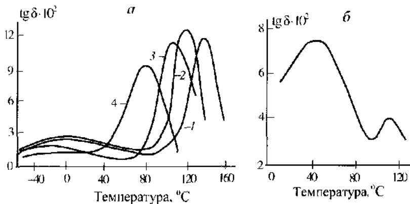
Рис. 9.7. Зависимость \lg \delta от температуры для некоторых ацеталей поливинилового спирта (а) и полиметилметакрилата (б): 1—этилаль; 2—пропилаль; 3—бутилаль; 4—октилаль.
