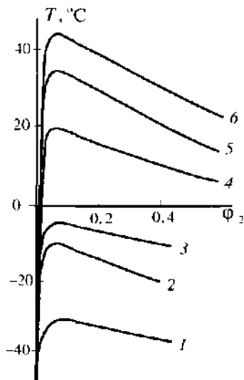
Рис. 16.6. Диаграммы состояния систем полистирол — фталаты: 1 — диметилфталат; 2 — дибутилфталат; 3 — диэкилфталат; 4 — диоктилфталат; 5 — динонилфталат; 6 — дидецилфталат.
