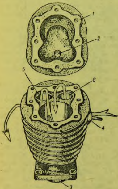
Рис. 24. Цилиндр двигателя ТИЗ-АМ-600
