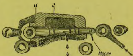
Рис. 52. Привод верхних клапанов Л-8
