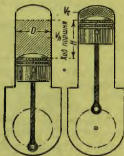
Рис. 21. Рабочий объем ( V_h ); общий объем ( V ); объем камеры сжатия ( V_c )
