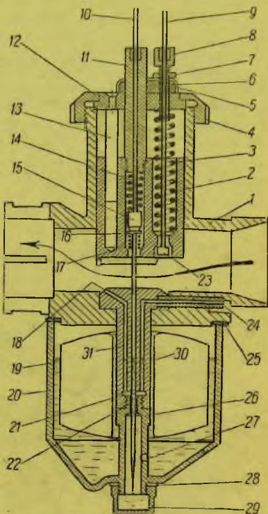
Рис. 80. Карбюратор ЛКЗ-22
