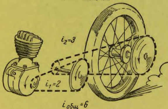
Рис. 162. Силовая передача
