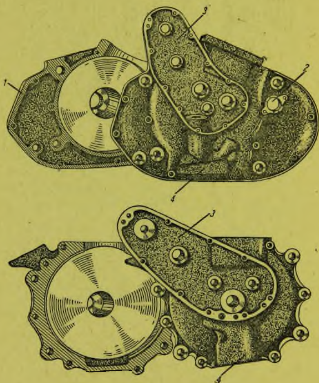
Рис. 45. Картер ТИЗ-АМ-600 и Л-8
