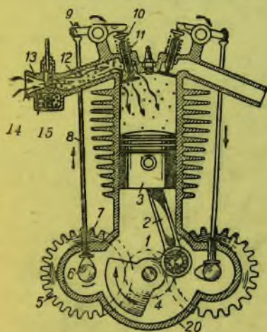
Рис. 5. Такт впуска
