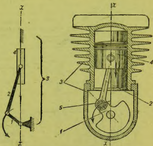
Рис. 3. Схема шатунно-кривошипного механизма: 1 — кривошип; 2 — шатун; 3 — рама (цилиндр и картер); 4 — ползун (поршень); 5 — палец кривошипа
