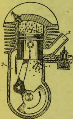
Рис. 9. Поршень идет вверх. В цилиндре сжимается ранее засосанная рабочая смесь. В картере создано разрежение; в приоткрывающееся выпускное окно (1) начинает поступать из карбюратора рабочая смесь
