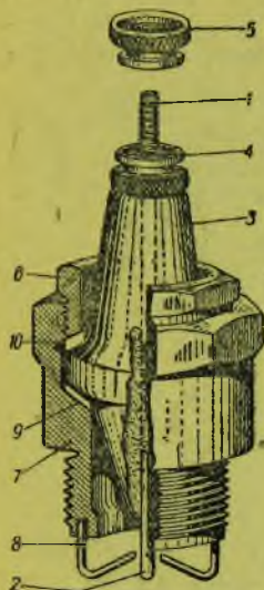
Рис. 138. Запальная свеча
