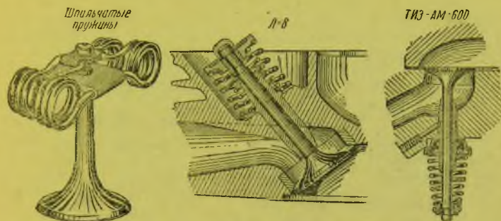
Рис. 49. Пружины клапанов
