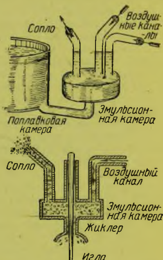
Рис. 82. Схема образования эмульсии в эмульсионной камере карбюратора
