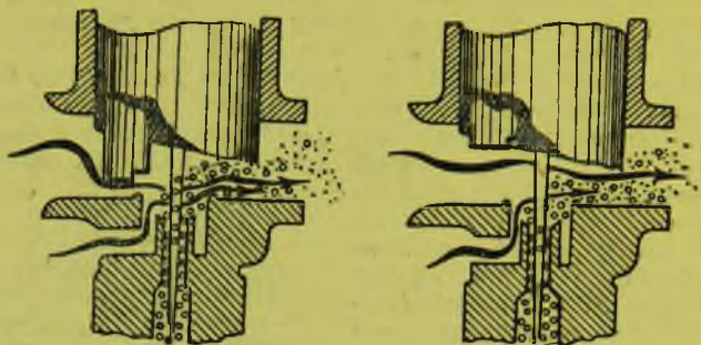
Рис. 97. Регулировка качества смеси корректором
