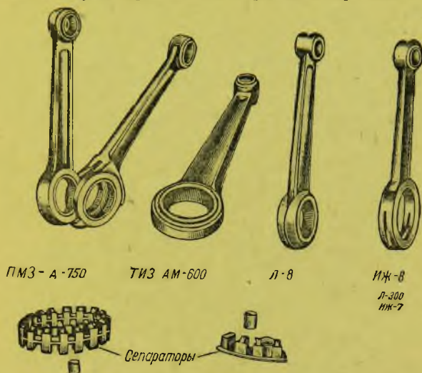
Рис. 33. Шатуны
