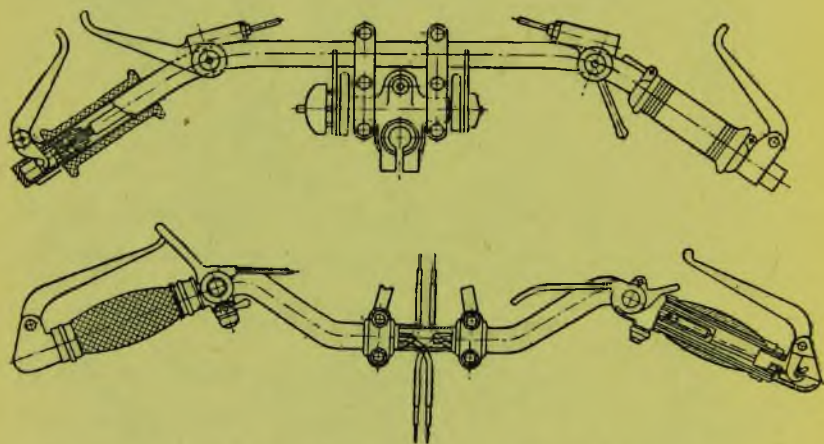
Рис. 188. Рули Л-300 (вверху), ТИЗ-АМ-600 (внизу)
