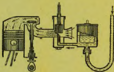
Рис. 76. Схема действия простейшего карбюратора
