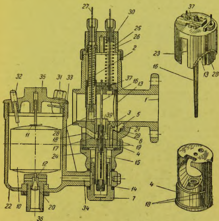
Рис. 88. Карбюратор МК-17
