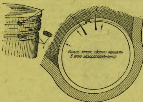
Рис. 28. Стопоры поршневых колец
