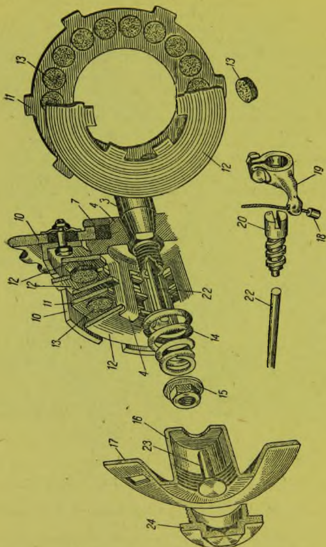
Рис. 168. Детали муфты сцепления Л-300, ИЖ-7, ИЖ-8
