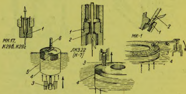
Рис. 103. Жиклеры, поплавки и запорные иглы
