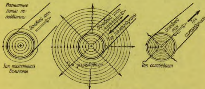
Рис. 112. Самоиндукция
