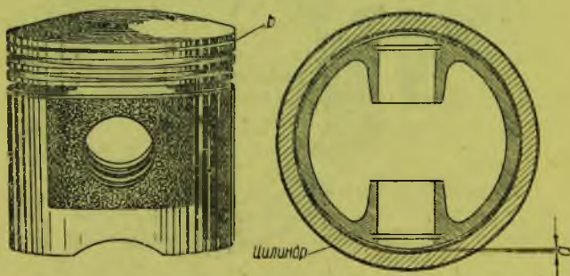
Рис. 29а. Поршень двигателя М-72 а — зазор между юбкой поршня и цилиндром в холодном состоянии
