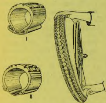
Рис. 193. Типы покрышек: кособортная (клинчерная) (I), прямобортная (II)
