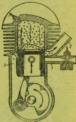
Рис. 16. Поршень продолжает двигаться вверх. В цилиндре выпускное окно (2) закрывается, так выпуск заканчивается. При дальнейшем ходе поршня вверх снова начнется сжатие. В картере создается разрежение, которое будет увеличиваться до тех пор, пока поршень не откроет впускное окно (7) для следующего наполнения картера рабочей смесью
