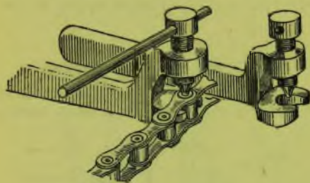
Рис. 179. Экстрактор цепи
