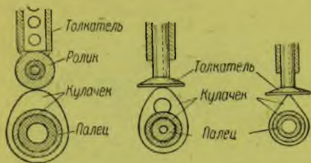
Рис. 53. Кулачки
