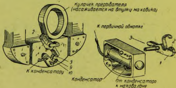
Рис. 137. Прерыватель Л-300
