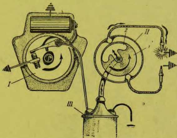
Рис. 137-А. Прерыватель-распределитель мотоцикла «М-72»:
