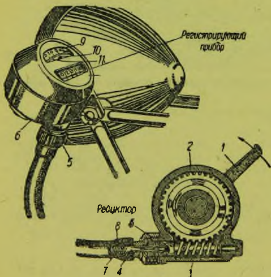
Рис. 208. Спидометр и счетчик пройденного пути
