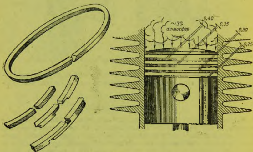
Рис. 31. Поршневые кольца
