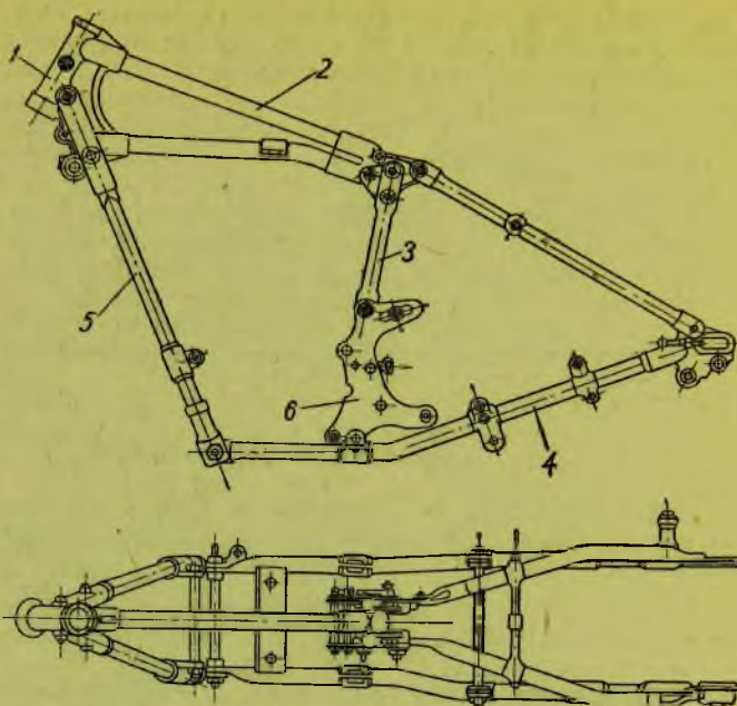
Рис. 182, Рама мотоцикла ТИЗ-АМ-600
