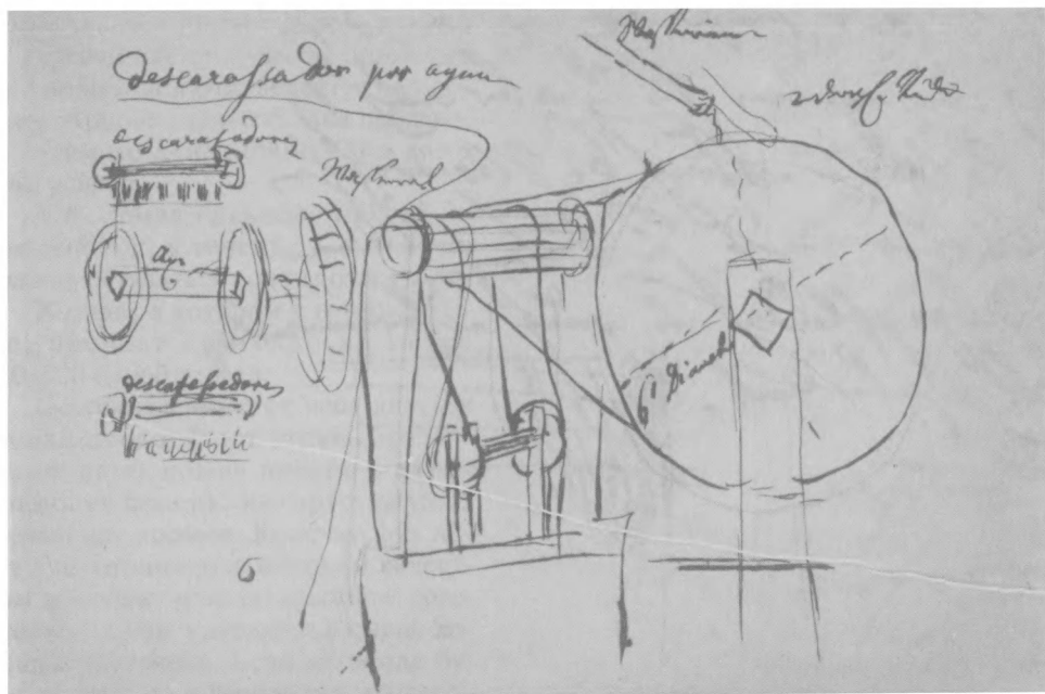
Машина "дескаросадор". Зарисовка в тексте Г.И. Лангсдорфа
