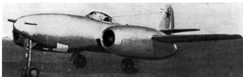
Самолет Су-11 с первым отечественным турбореактивным двигателем конструкции А. М. Люльки.
