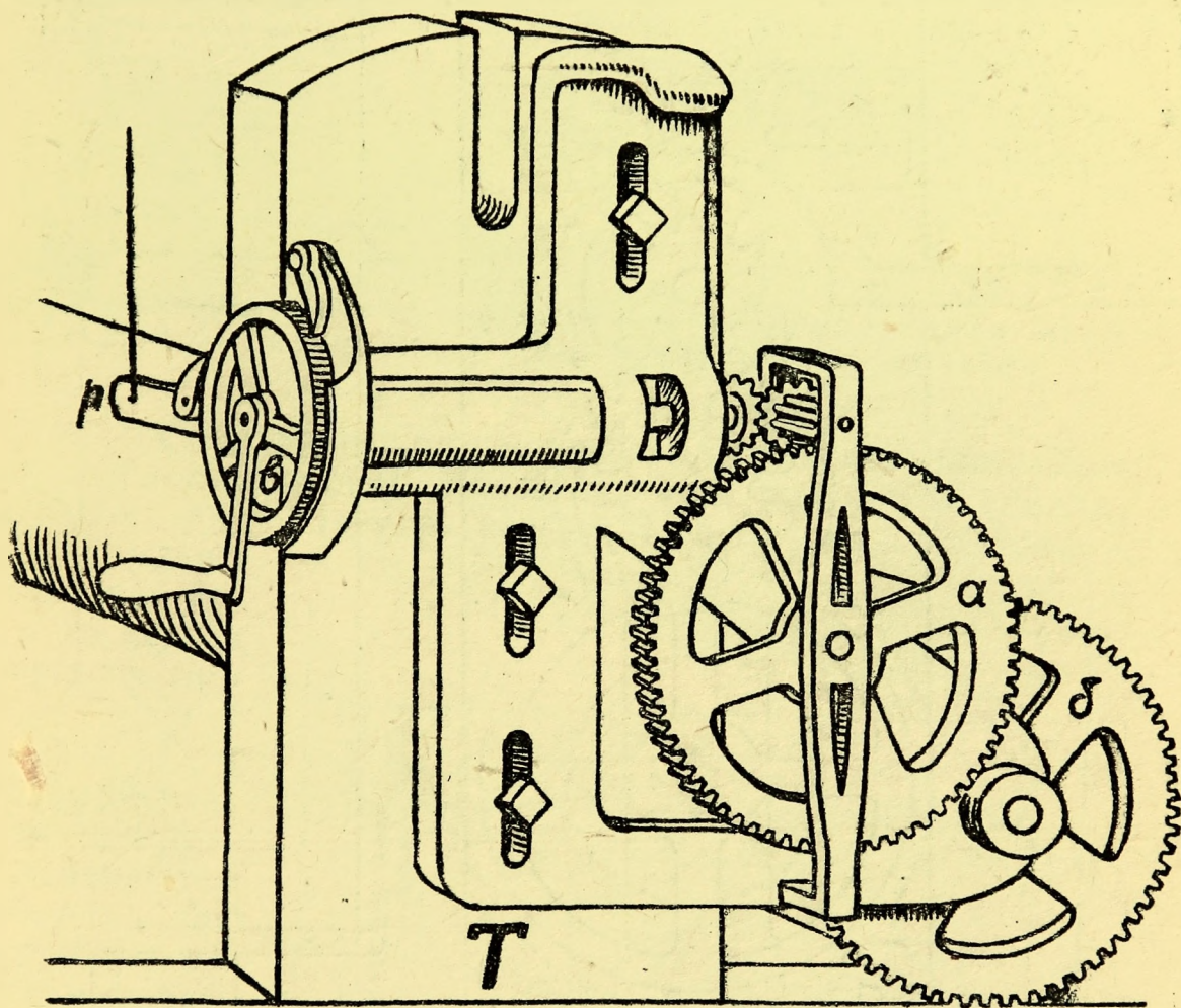
Рис. 135. Регулятор.
