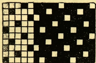
Рис. 28. Атласное переплетение основное и уточное.
