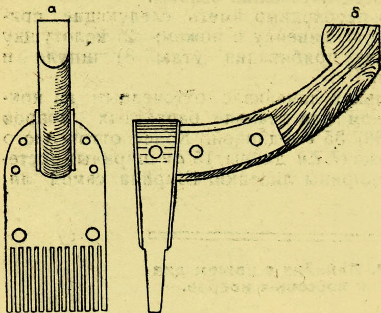
Рис. 199. Ковровая колотушка - лятка, вид спереди и со боку.
