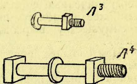
Рис. 163. Болт L^3 для укрепления линейки и других железных частей, L^4 —болт для соединения плечей батана со станком.
