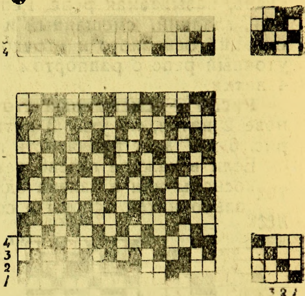
Рис. 10. Саржевое ломаное переплетение 2/2 .
