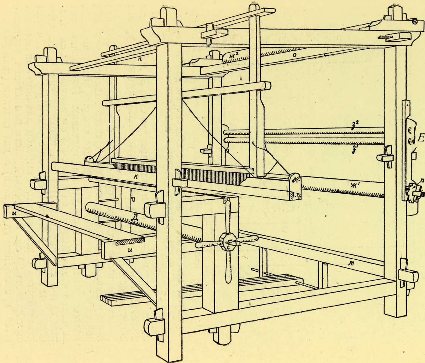
Рис. 148. Общий вид ткацкого станка с двумя навоями для основ—верхним и нижним (каретка снята) для махровых полотенец и др. тканей.
