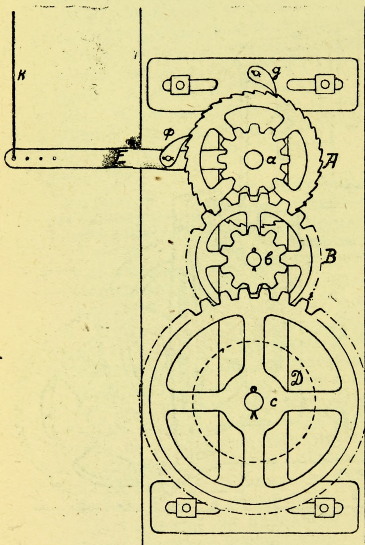
Рис. 136. Регулятор.
