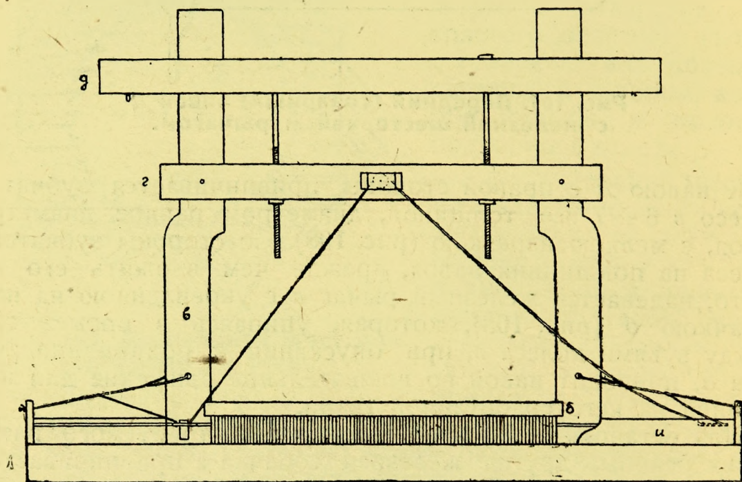
Рис. 109. Батан-самолет—вид спереди.
