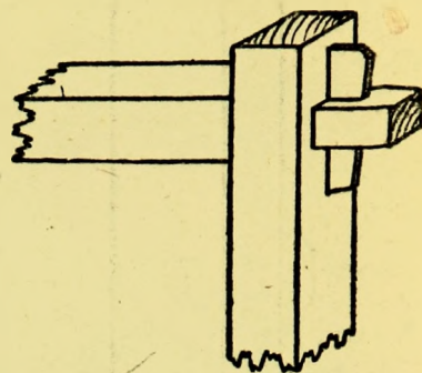
Рис. 100. Способ соединения поперечных частей станка с боковинами — заклинивание.
