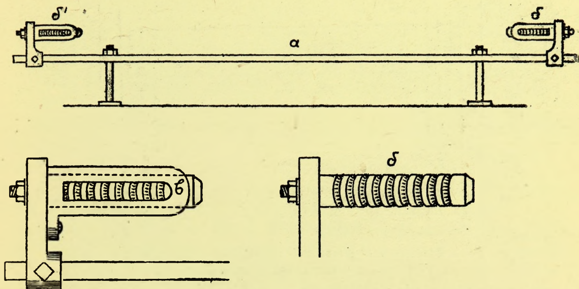
Рис. 138. Самошпарутки: а —общий вид б —кольцевидная часть с иглами без щитка, в —часть, прикрытая щитком.
