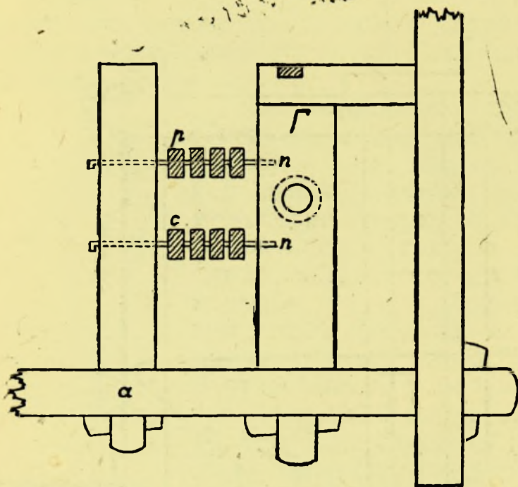
Рис. 152. Помещение рычагов в левой раме станка.
