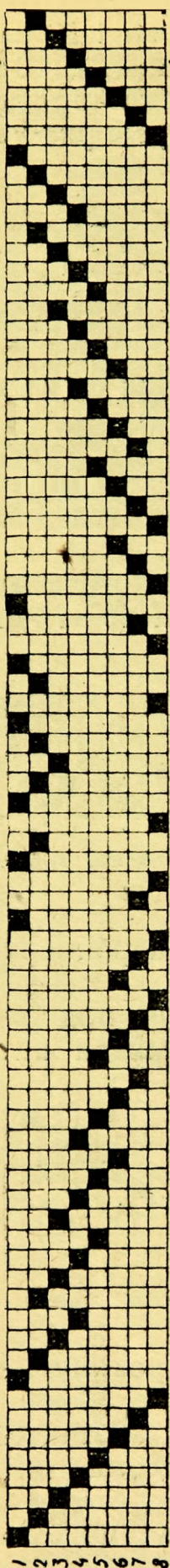
Рис. 38. Пробор в ремизки ступенчатый.
