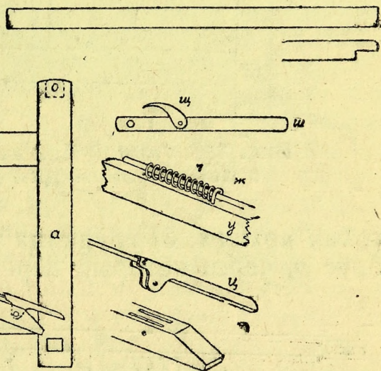
Рис. 157. Детали прибора М : пружина ч , обвивающая железный прут ф ; дужка ж для ее упора в бруске у ; рычаг ц и подним гнезда для укрепления его в бруске у .
