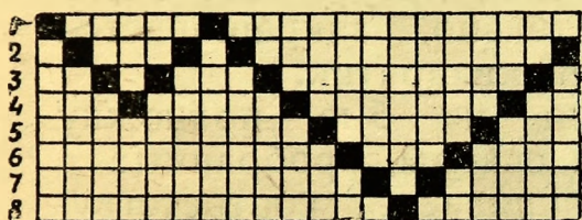
Рис. 35. Пробор в ремизки зигзагами.
