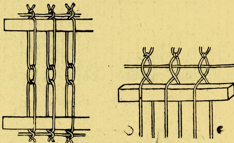
Рис. 86 и 86а. Ремиз раздвижной.
