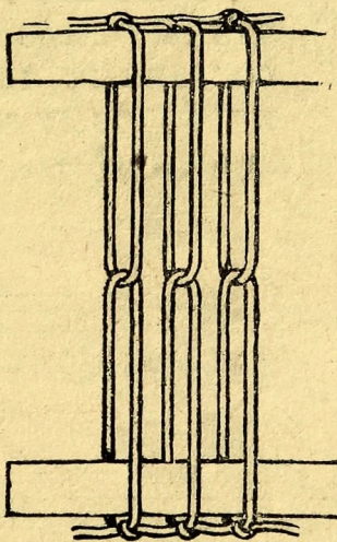
Рис. 85. Ремиз [глухой.]
