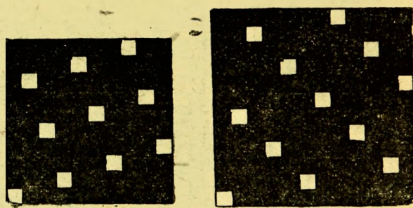
Рис. 26 и 27. Атласное переплетение 10 и 12-ремизное уточное.
