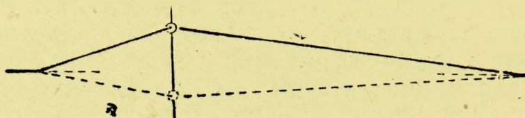
Рис. 128. Верхний зев.
