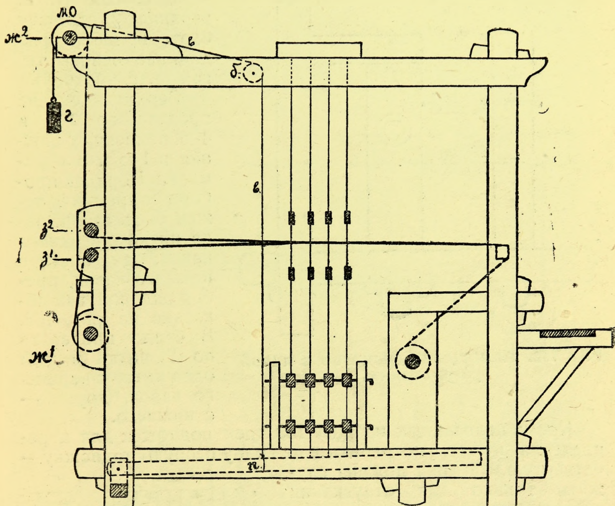
Рис. 151. Левая рама станка с помещением верхнего навоя Ж^2 , грузом г , блочком б , направлением нижней и верхней основ и соединением шнура в с подножкой п .
