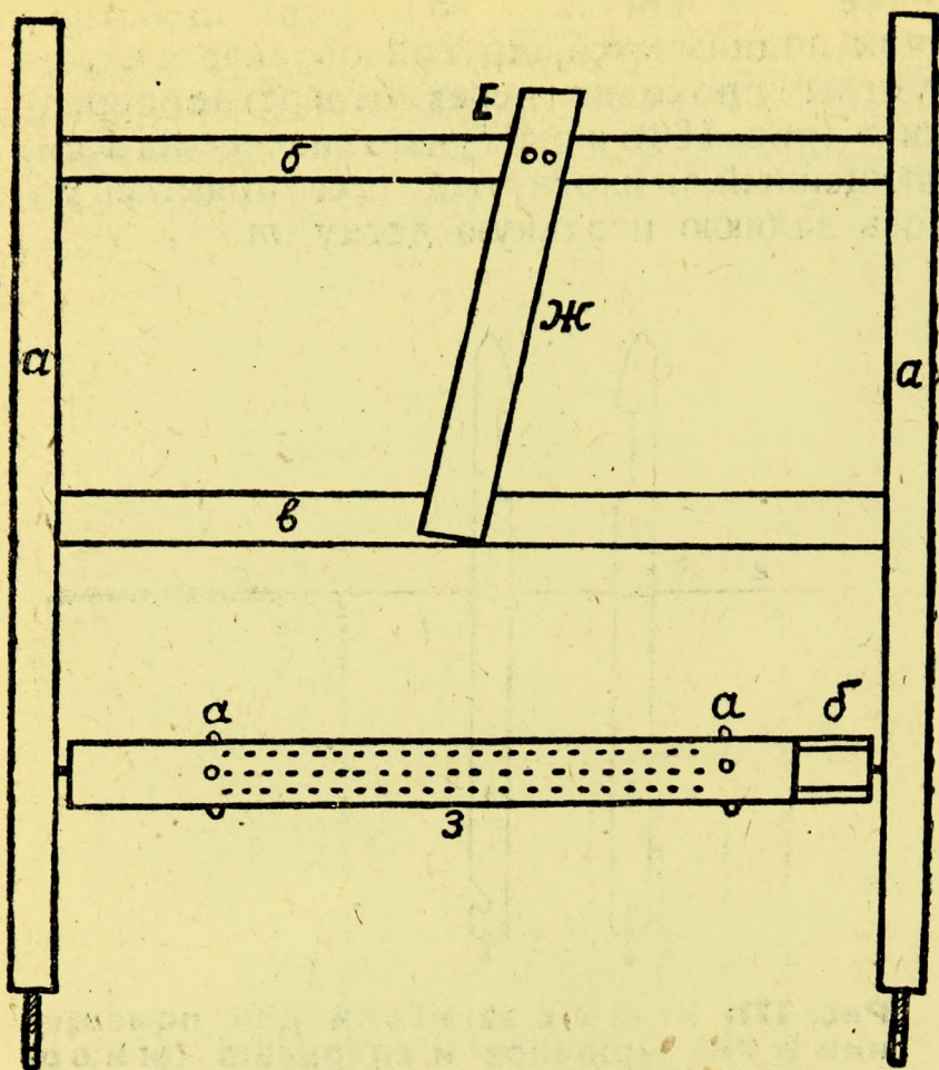
Рис. 173. Батанчик Е —вид спереди.
