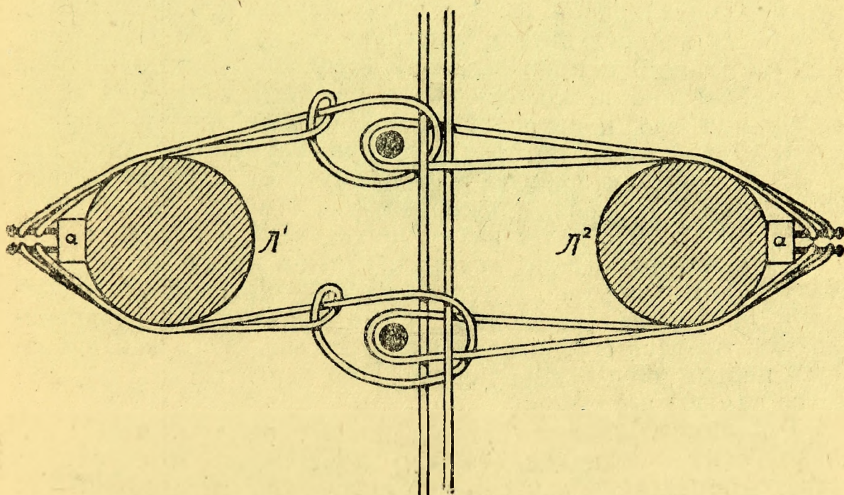
Рис. 193. Ремизные валики L^1 и L^2 с ремизами—вид сбоку.
