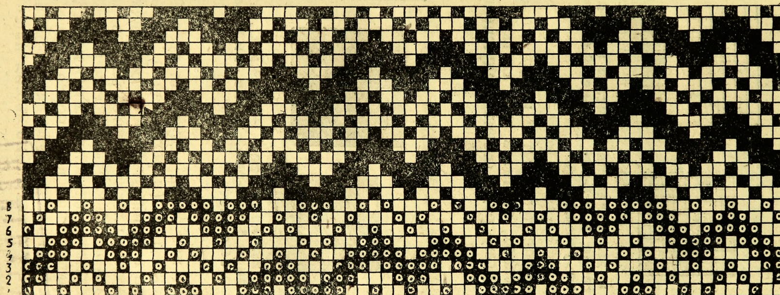
Рис. 19. Саржевое зигзагообразное переплетение \frac{3}{2}-\frac{1}{2} .
