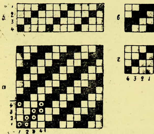
Рис. 131. Патрон для заправки ткани с подвязью в.
