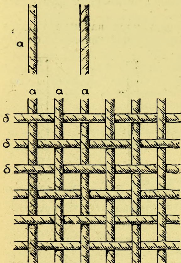
Рис. 44. Ткань из пряжи правой крутки по основе а—а—а и левой крутки б—б—б по утку.
