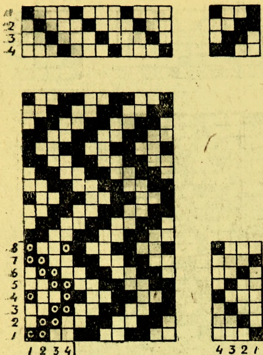
Рис. 17. Саржевое зигзагообразное переплетение 2/2 .
