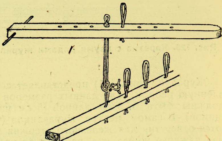
Рис. 122а. Способ соединения рычага с подножкой.
