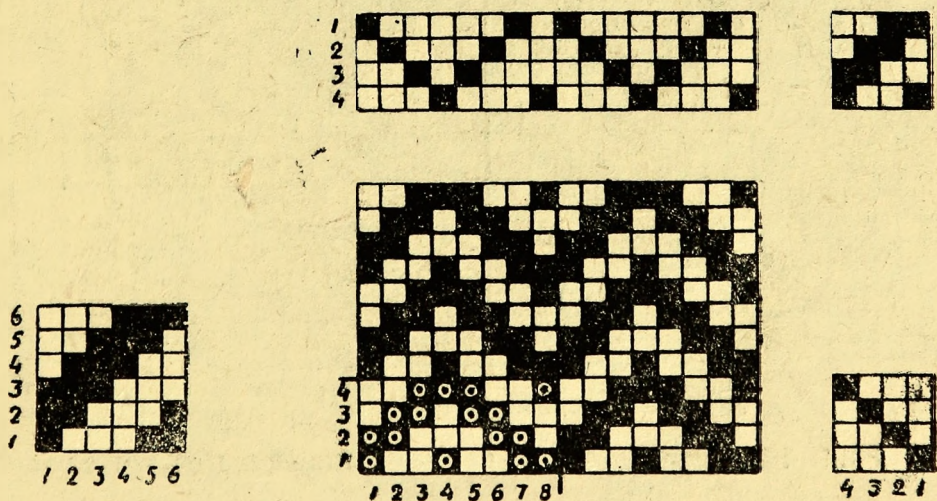
Рис. 16. Саржевое зигзагообразное переплетение \frac{2}{2} .
