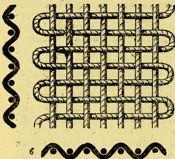
Рис. 1. Полотняная ткань: а—вид сверху, б—разрез по основе, в—разрез по утку.
