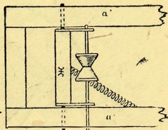
Рис. 50б. Вид сверху.
