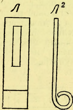
Рис. 162. Железная линейка L с загибом—вид спереди, L^2 —вид сбоку.
