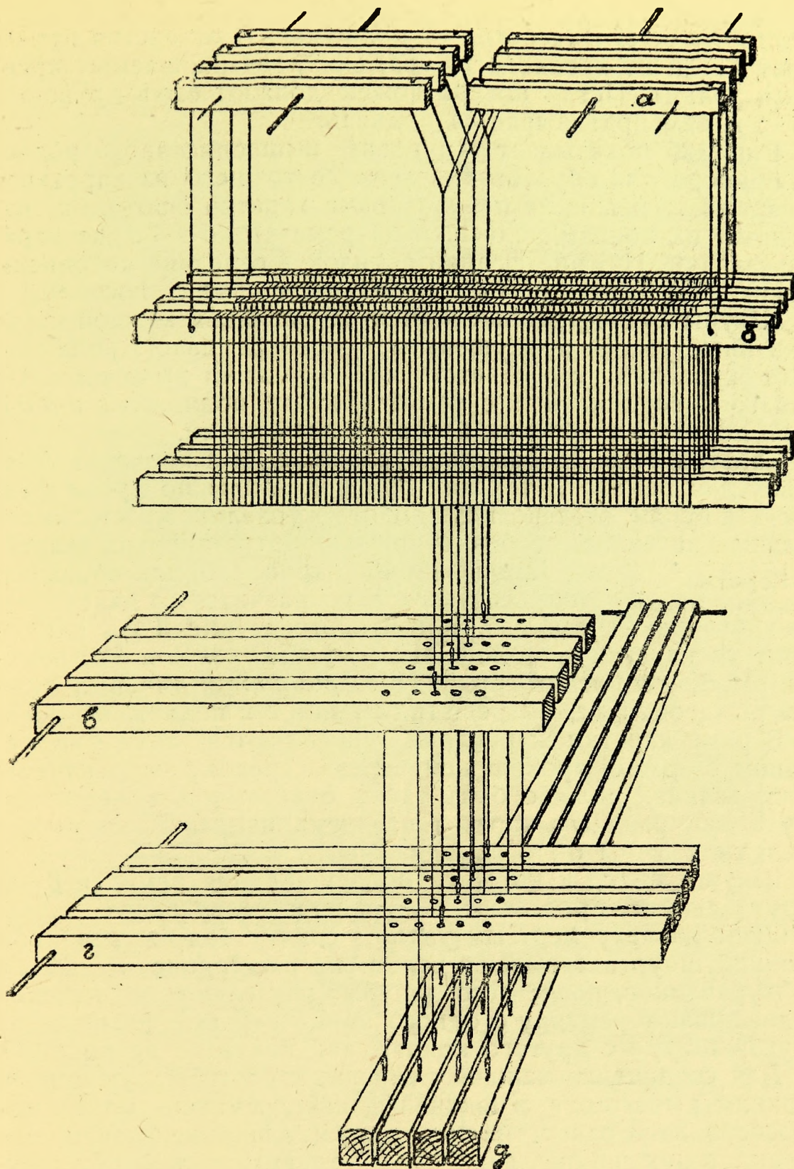
Рис. 125. Соединение каретки с ремизками, рычагами и под- кожками — оснуровка.
