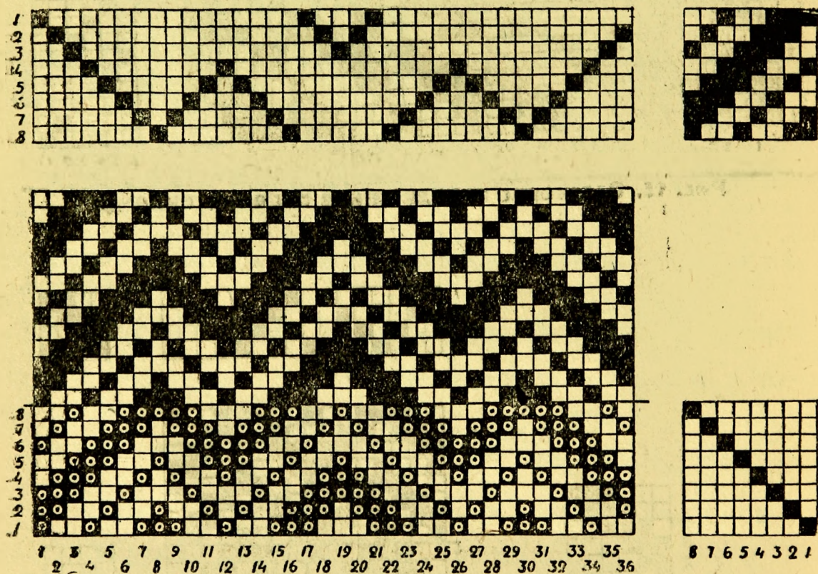
Рис. 18. Саржевое зигзагообразное переплетение \frac{3}{2}-\frac{1}{2} .
