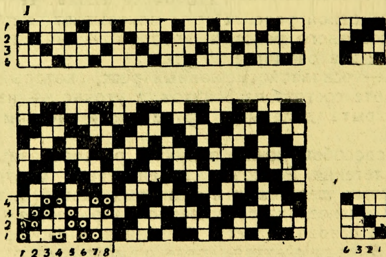
Рис. 11. Саржевое ломаное переплетение 2/2 .
