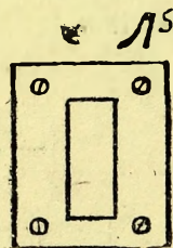
Рис. 164. L^5 —железная рамка для предохранения от разработки дерева болтами.
