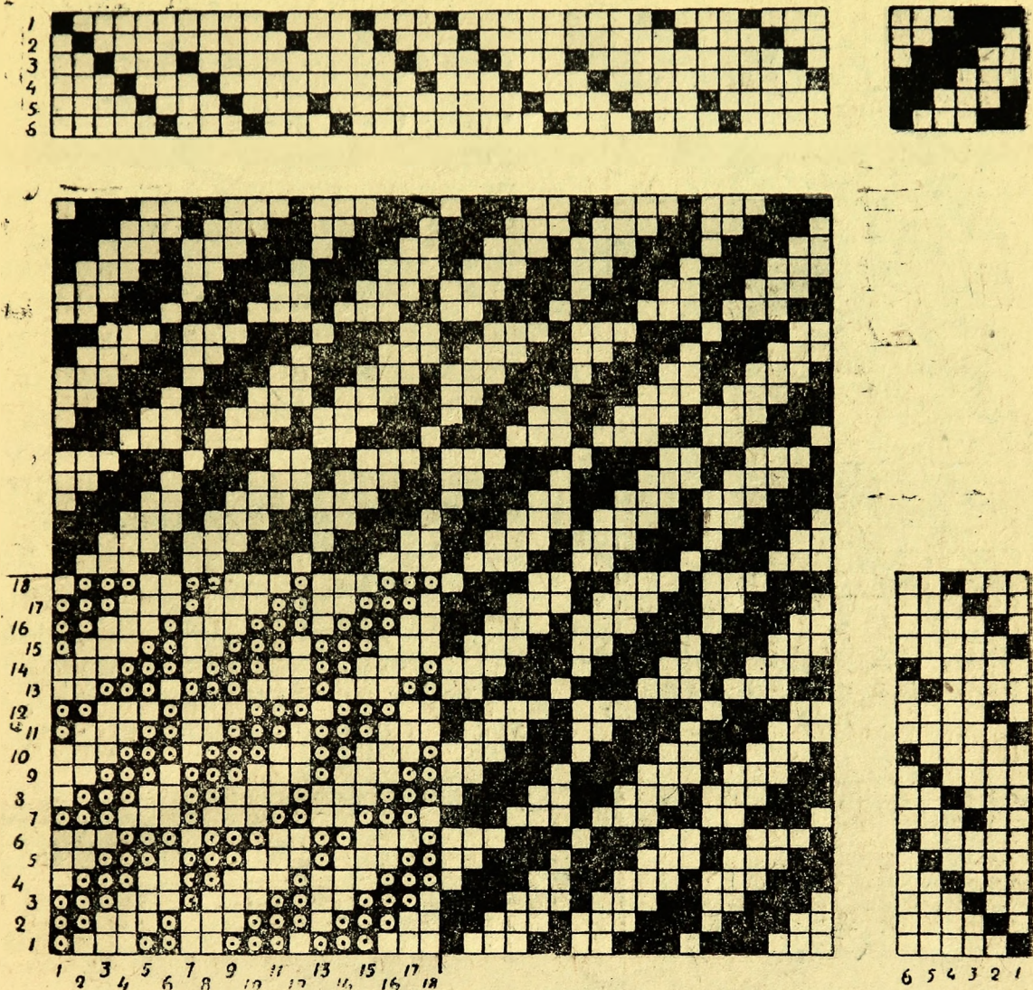
Рис. 15. Саржевое передвижное переплетение \frac{9}{8} .
