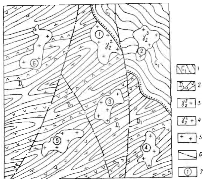
Рис. 1. Схематический геологический план участка 1 — углисто-кремнистые сланцы нижнего карбона; 2 — эффузивно-осадочные породы нижнего девона; 3 — гранитные интрузии среднего палеозоя; 4 — гранитные интрузии позднего палеозоя; 5 — палеозойские гранитные интрузии; 6 — тектонические нарушения; 7 — порядковый номер интрузии
