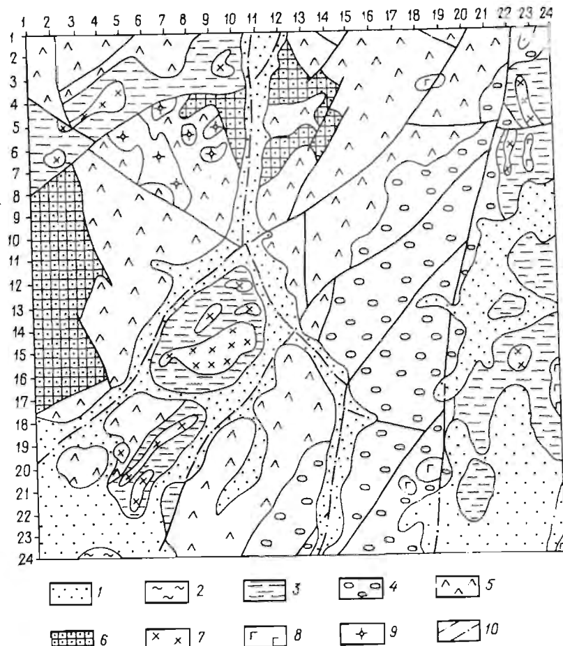
Рис. 9. Схематическая геологическая карта:
