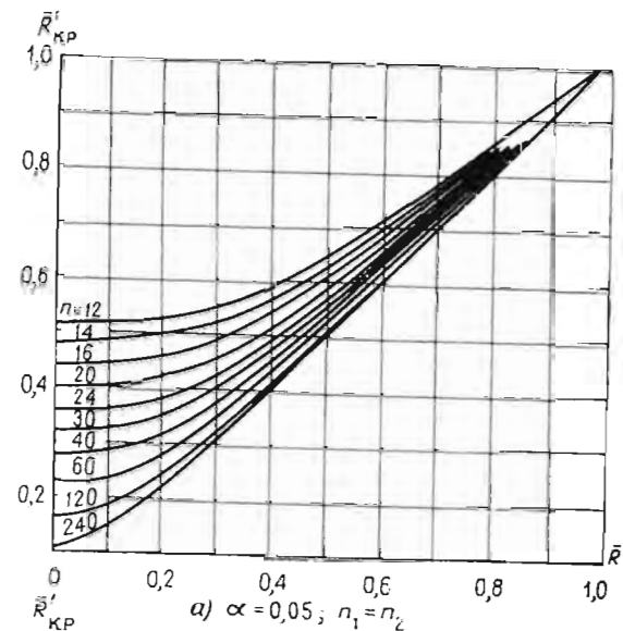
Номограмма для определения критических значений критерия Ватсона – Вильямса
