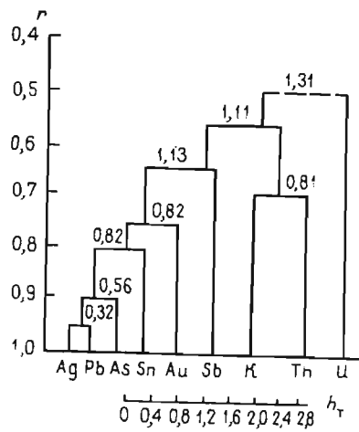
Рис. 4. Дендрограф взаимосвязей химических элементов на эталонном объекте
