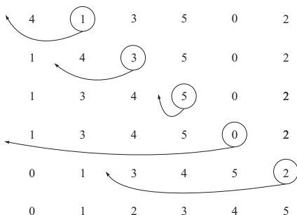
Рис. П.3. Работа процедуры сортировки
