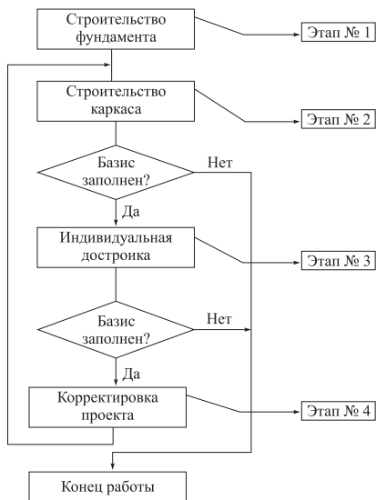
Рис. 5.29. Структурная схема генетического алгоритма
