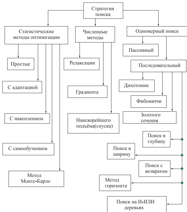
Рис. 2.1. Классификация стратегий поиска
