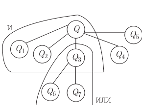
Рис. 2.6. Пример схемы поиска на основе И-ИЛИ деревьев
