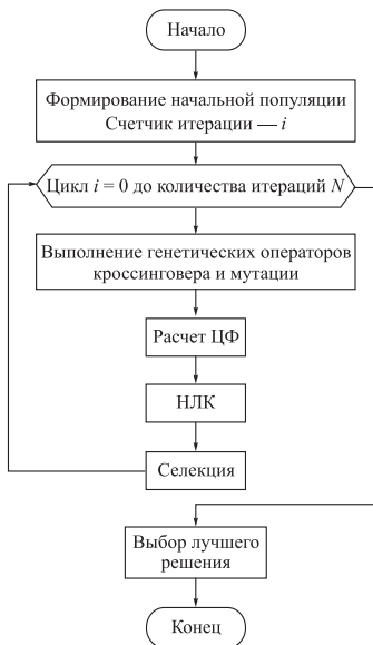
Рис. 5.49. Структурная схема нечеткого генетического алгоритма
