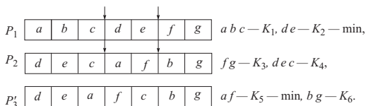
Рис. 5.9. Схема модифицированного оператора кроссинговера
