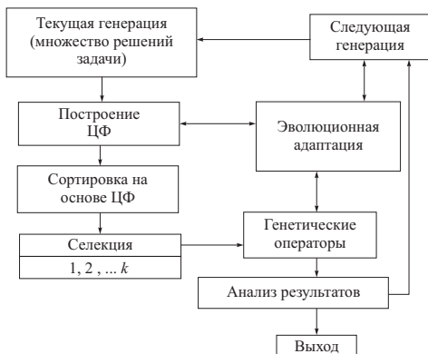
Рис. 4.4. Базовая структура генетического алгоритма
