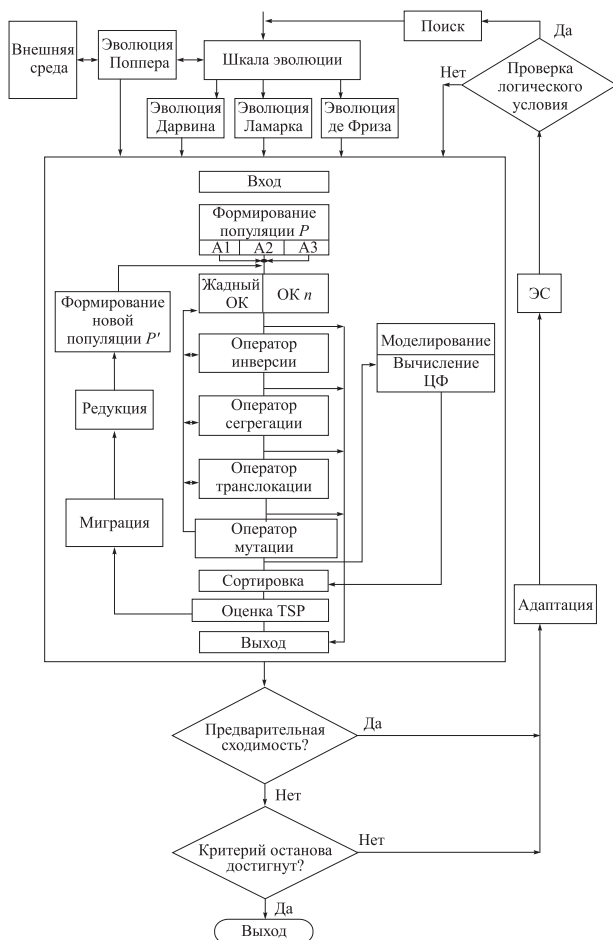
Рис. 5.13. Структурная схема алгоритма решения задачи коммивояжера
