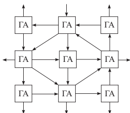
Рис. 4.7, в. Последовательная схема поиска на основе треугольников
