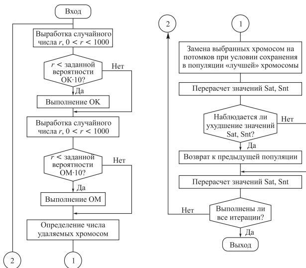
Рис. 5.47. Структурная схема алгоритма
