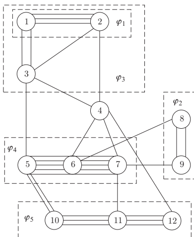
Рис. 5.8. Граф G
