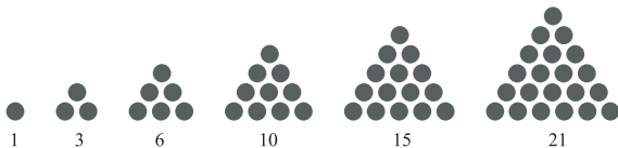
Рис. 4.23. Последовательность треугольных чисел
