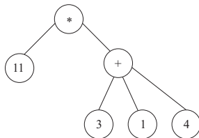
Рис. 4.17. Дерево LISP-выражения (*11(+314))
