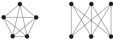
Рис. 5.19. Графы K_5 и K_{3,3}
