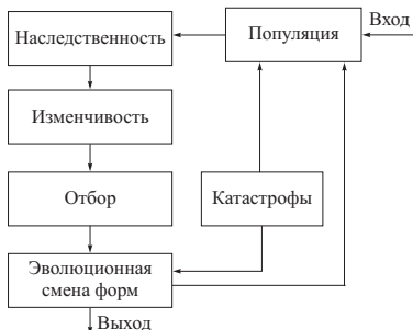
Рис. 1.8. Условная упрощенная схема модели эволюции де Фриза
