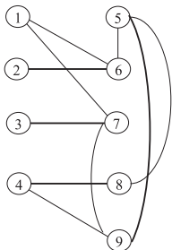
Рис. 5.43. Граф G
