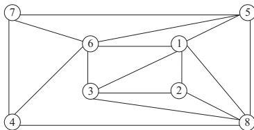
Рис. 5.32. Плоская укладка графа G
