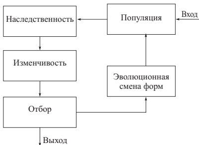
Рис. 1.3. Условная упрощенная схема модели эволюции Дарвина
