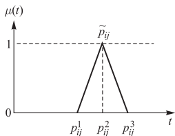
Рис. 5.45. Нечеткое время выполнения операции
