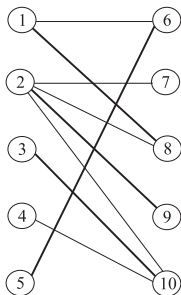
Рис. 5.42. Двудольный граф G
