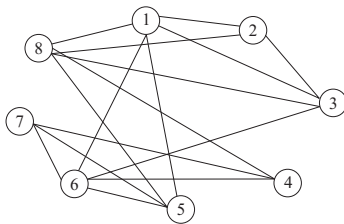
Рис. 5.27. Граф G , заданный случайным образом
