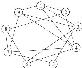
Рис. 5.33. Граф G' , заданный случайным образом
