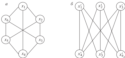
Рис. 5.35. а — граф G , б — граф G'
