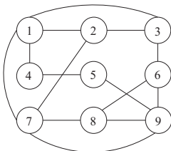
Рис. 5.14. Граф G
