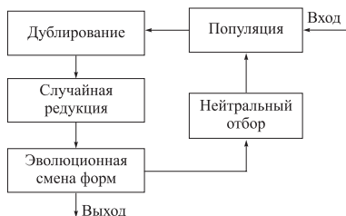
Рис. 1.10. Условная упрощенная схема модели нейтральной эволюции
