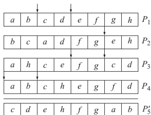
Рис. 5.11. Пример оператора сегрегации
