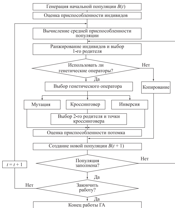
Рис. 5.25. Модифицированная схема работы генетического алгоритма
