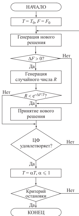
Рис. 2.10. Схема алгоритма моделирования отжига
