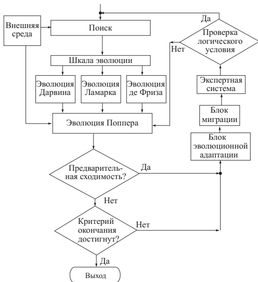
Рис. 4.19. Модификация базовой структуры
