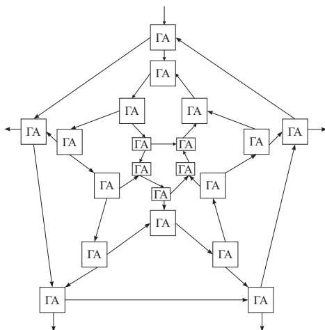
Рис. 4.6, д. Схема поиска на основе додекаэдра
