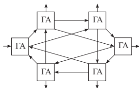
Рис. 4.6, в. Схема поиска на основе октаэдра
