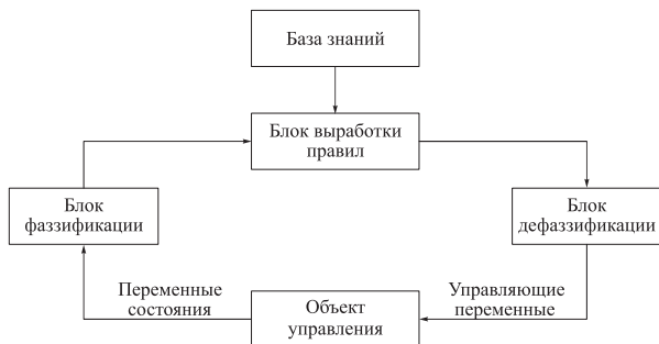
Рис. 5.44. Обобщенная структура нечеткого логического контроллера
