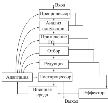
Рис. 4.14. Пример реализации архитектуры соподчинения в эволюционном поиске
