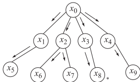
Рис. 2.3. Схема метода поиска в ширину
