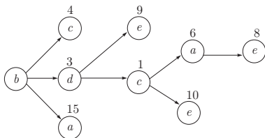
Рис. 3.1. Пример реализации «жадного» оператора кроссинговера
