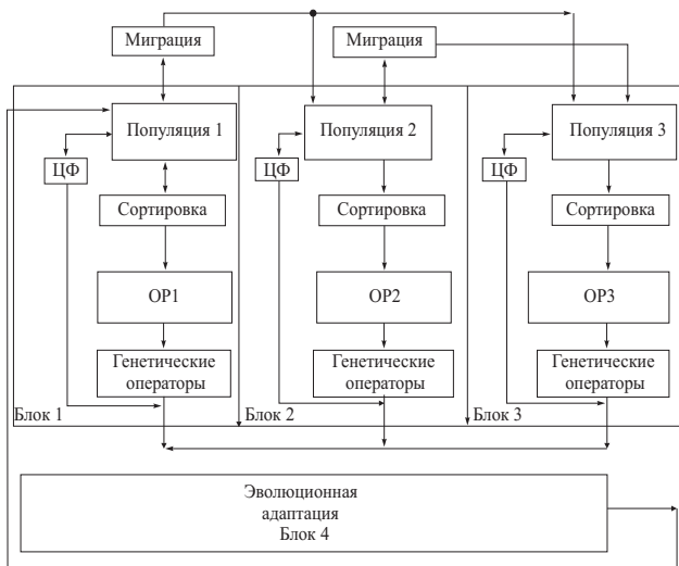
Рис. 4.5. Схема эволюционного поиска на основе миграции
