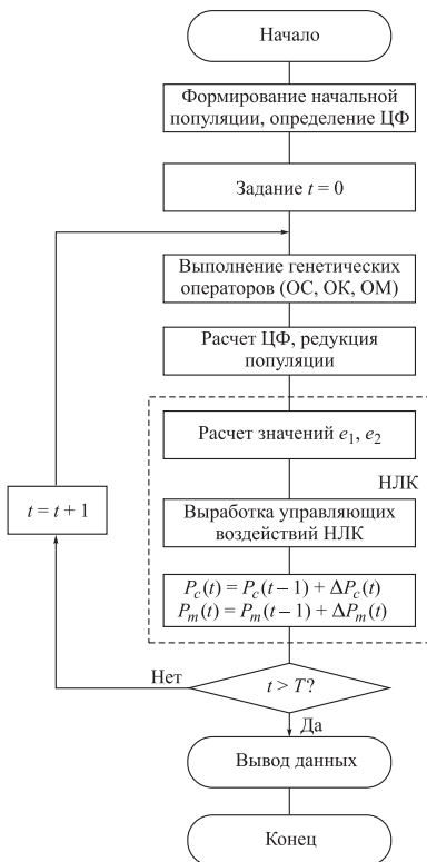
Рис. 5.50. Структурная схема НГА
