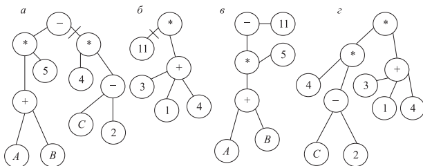
Рис. 4.21. Реализация оператора кроссинговера
