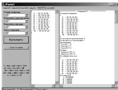
Рис. П.9. Пример работы простого генетического алгоритма по поиску максимума функции
