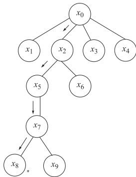
Рис. 2.2. Схема метода поиска в глубину
