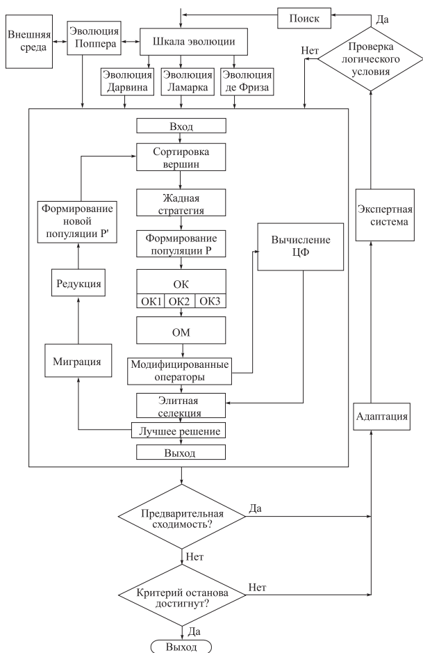
Рис. 5.16. Структура гибридного генетического алгоритма
