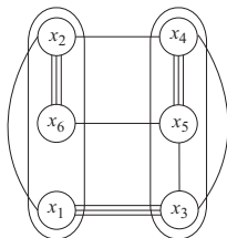
Рис. 5.4. Разбиение G на две части
