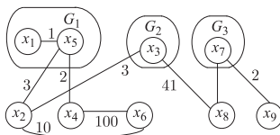
Рис. 2.4. Частичное разбиение графа G на три части
