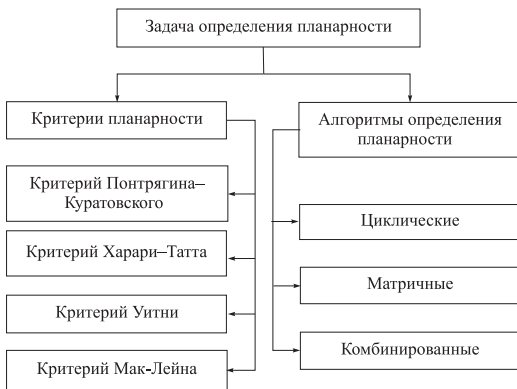
Рис. 5.21. Классификация методов определения планарности
