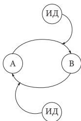
Рис. 1.5. Пример простейшего гиперцикла Эйгена
