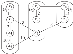
Рис. 2.5. Окончательное разбиение графа G
