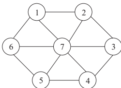
Рис. 5.15. Колесо W_7
