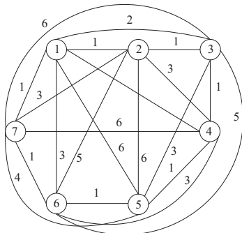
Рис. 5.12. Граф G = (X, U)
