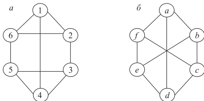
Рис. 5.37. a — граф G , б — граф G'
