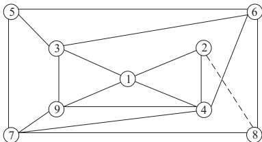
Рис. 5.34. Максимальная планарная укладка графа G'
