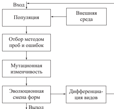
Рис. 1.9. Условная упрощенная схема модели эволюции Поппера
