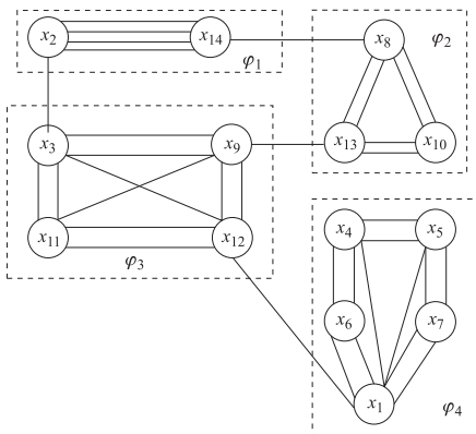
Рис. 5.7. Граф G
