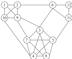
Рис. 5.18. Граф G для определения клик
