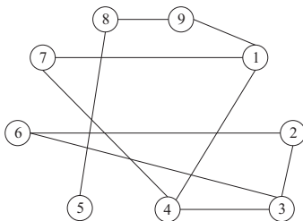
Рис. 5.17. Граф G для определения независимых подмножеств
