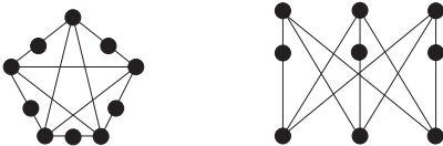
Рис. 5.20. Графы, гомеоморфные графам K_5 и K_{3,3}
