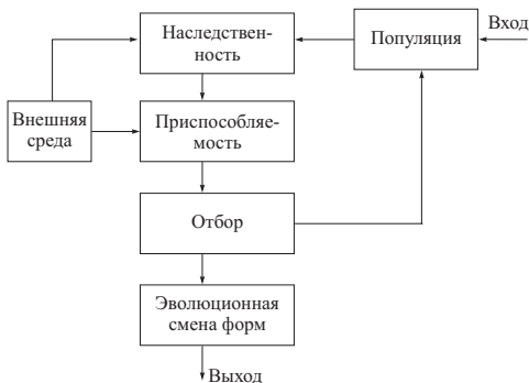
Рис. 1.7. Условная упрощенная схема модели эволюции Ламарка
