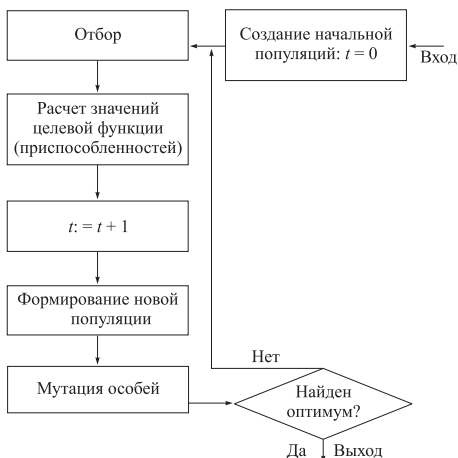
Рис. 1.6. Условная схема эволюции в модели квазивидов
