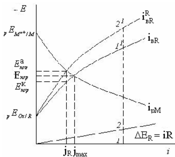
Диаграмма при наличии омического фактора
