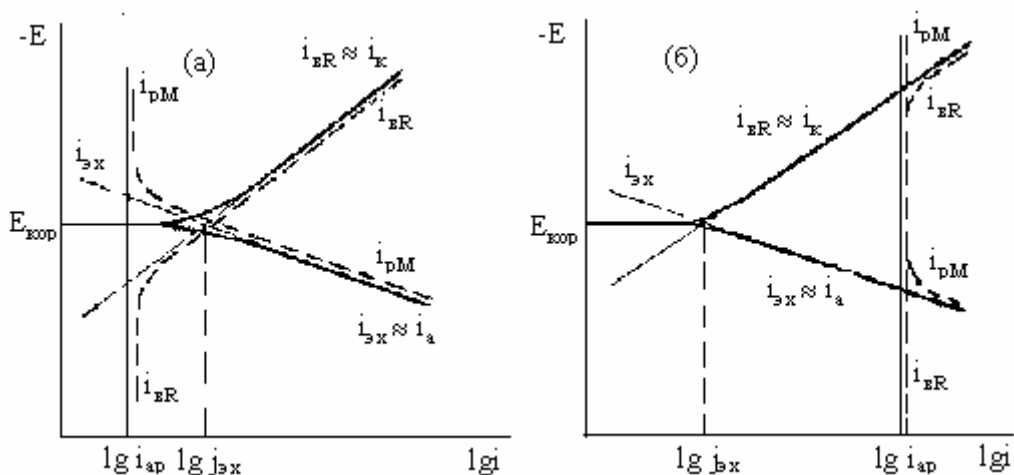
Диаграммы при химико-электрохимическом растворении металлов
