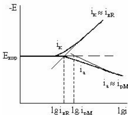
Диаграмма при гетерогенно-электрохимическом механизме коррозии
