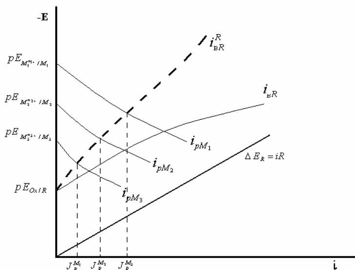
Диаграмма для трех металлов при наличии омического фактора
