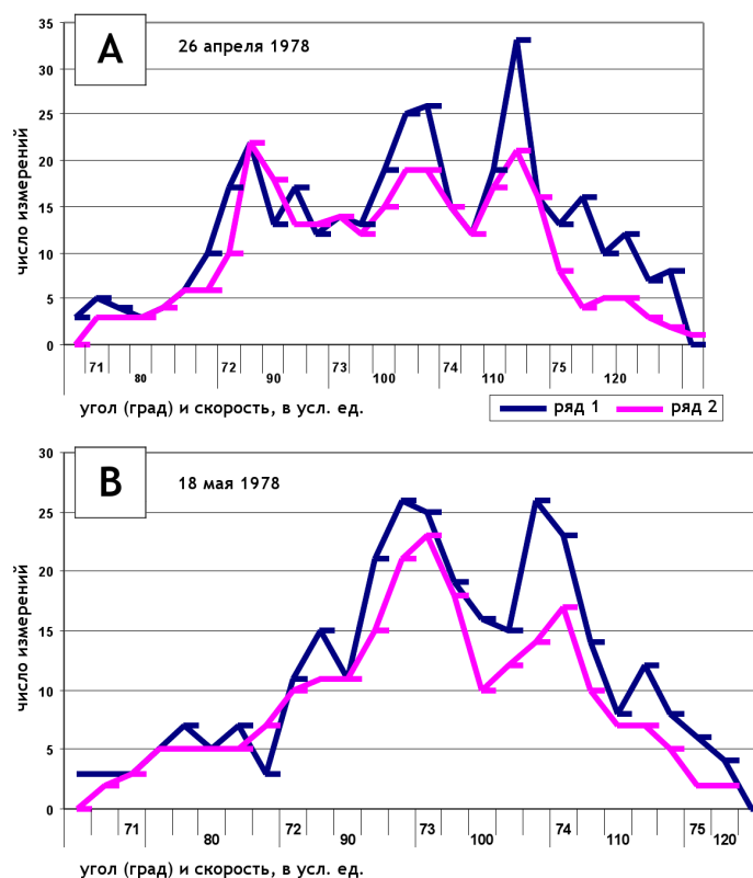
Рис. 20: Гистограммы, построенные по синхронным измерениям углов поворота лимба при настройке поляриметра (1) (В. Е. Жвирблис, Москва) и скорости крестинкиназной реакции (2) в Пущино оказались сходными, как в опыте 26 апреля, так и в опыте 18 мая 1978 г. [92].
