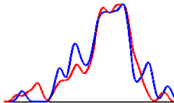
Рис. 18-3-20: Полнолуния 24 июля в момент максимума и 23 августа 2002 года за 2 минуты до момента максимума.
