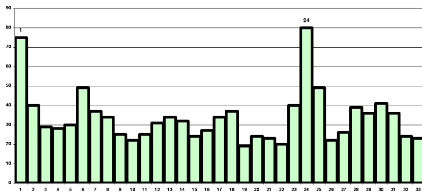
Рис. 5-2: Эффект “ближней зоны” и околосуточный период повторного появления 1-часовых гистограмм сходной формы при измерениях альфа-активности ^{239}\text{Pu} 1–2 марта 2003 г. на ст. Новозазаревская в Антарктиде. Оси как на рис. 5-1.
