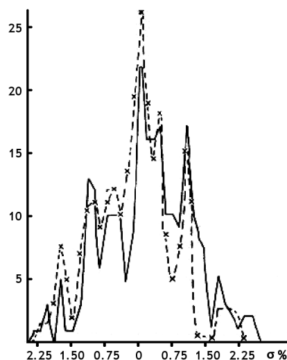
Рис. 32: Форма гистограмм не зависит от природы измеряемого процесса. Измерения бета-активности ^{14}\text{C} (В. И. Брусов) и скорости реакции АК + ДХФИФ (С. Э. Шноль, Т. Я. Брицина и Н. П. Иванова). Опыт 4 июля 1984 г. Ось абсцисс для обоих процессов — в долях среднеквадратичного отклонения ( \sigma ), рис. 19 из [32].
