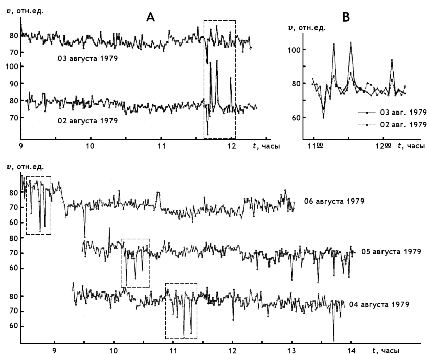
Рис. 21: Резкие изменения скорости реакции аскорбиновой кислоты с дихлорфенолинофенолом под действием внешних “сигналов” неизвестной природы. Опыты на ББС МГУ 2–13 августа 1979 г. Оси абсцисс — время. Ординаты — скорость реакции в относительных единицах. Справа наверху — сопоставление сигналов 2 августа и 3 августа 1979 г. [92].
