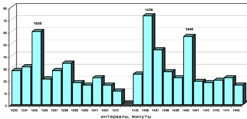
Рис. 16-12: В день летнего солнцестояния 22 июня 2004 года видны три экстремума — с периодами равными (слева направо) длительности светлого времени (но не 1037, а 1035 минут!), звездным суткам (1436) и солнечным суткам (1440).
