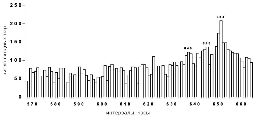
Рис. 9-3: То же распределение, что и на рис. 9-2 с угрублением разряда по оси абсцисс до 60 минут. Указаны величины периодов в часах.
