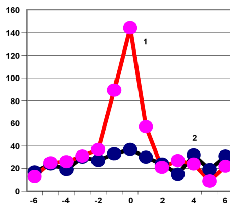
Рис. 21-3: 1-й опыт с “эффектом палиндрома”. Последовательность одноминутных “дневных” гистограмм с высокой вероятностью сходна с обратной (инверсной) последовательностью “ночных” гистограмм, в опыте с измерением альфа-активности ^{239}\text{Pu} счетчиком без коллиматора 23.04.2004 г. (кривая 1). Без инверсии, т.е. при сравнении прямых дневных и ночных рядов, (кривая 2) синхронного сходства нет. Абсцисса — интервалы = разность номеров (минутных) гистограмм. Ордината — число сходных пар, соответствующее данному интервалу.
