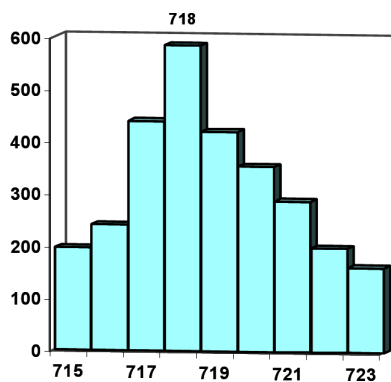
Рис. 16-3: В дни равноденствий 2000–2003 г.г. сходные гистограммы с высокой вероятностью наблюдались с периодом равным 718 минутам — половине звездных, а не солнечных суток.
