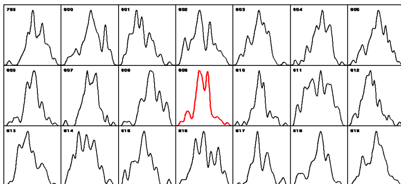
Рис. 19-13: 1- минутные гистограммы построены по результатам измерений альфа-активности ^{239}\text{Pu} плоским детектором во время солнечного затмения 3 октября 2005 г. в Пушино ( 54,8^\circ с.ш., 37,6^\circ в.д.). Гистограмма № 809 — в центре 2-й строки — на 1 минуту позже момента максимума затмения.
