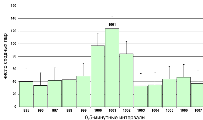
Рис. 22-6: Синхронность по местному времени. Зависимость вероятности появления гистограмм сходной формы при сравнении результатов измерений 8 апреля 2005 г. с генераторами № 28 (Роджер Нельсон, Принстон, Нью Джерси, США, 40^\circ 35' с.ш. и 74^\circ 65' з.д.) и № 100 (Робин Тэйлор и Симон Гривз, Сува, острова Фиджи, -17,75^\circ ю.ш. и -177,45^\circ в.д.) от величины разделяющего их интервала времени. Расчетная разность местного времени равна 1006 минутам.
