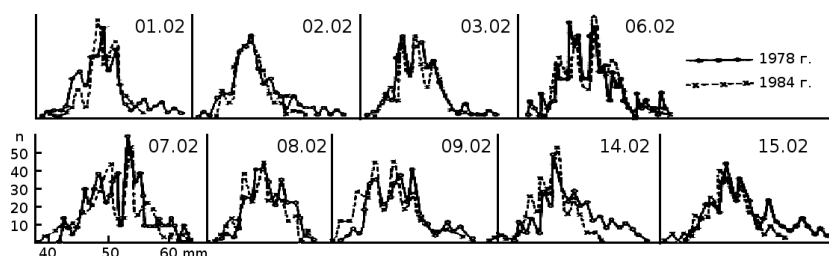
Рис. 10-1: Серии сходных гистограмм в одни и те же даты и часы ровно через 6 лет — в 1978 году измерения ферментативной активности креатинкиназы, в 1984 году измерения скорости реакции АК+ДХФИФ. По 250 измерений в каждой гистограмме.
