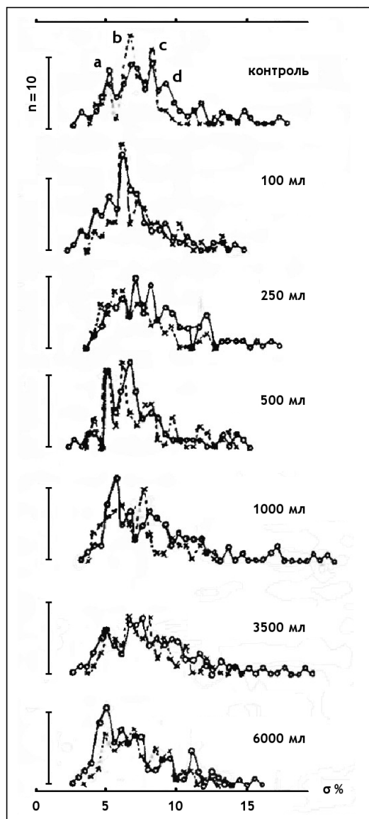
Рис. 16: Зависимость формы гистограмм средневладратичных амплитуд флуктуации титра SH-групп (—○—○—) и АТФазной активности (—×—×—) растворов актомиозина от объема шарообразных колб с водой, окружающей пробирки с белком. Опыты 30 мая 1967 г. — 27 июня 1968 г. Ось абсцисс — величины \sigma\% . Ось ординат — число опытов, соответствующее данной величине \sigma\% [32, 33].
