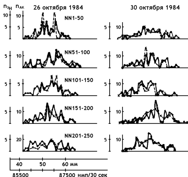
Рис. 36: Опыты 26 и 30 октября 1984 г. Синхронные по местному времени измерения бета-активности {}^3\text{H} в Ленинграде ( 59^\circ 57' с.ш. и 30^\circ 12' в.д., А. Ю. Сунгуров) и скорости реакции \text{AK} + \text{ДХФИФ} в Пущино (С. Э. Шноль, Н. П. Иванова и Т. Я. Брицина), рис. 25 из [32, 33].
