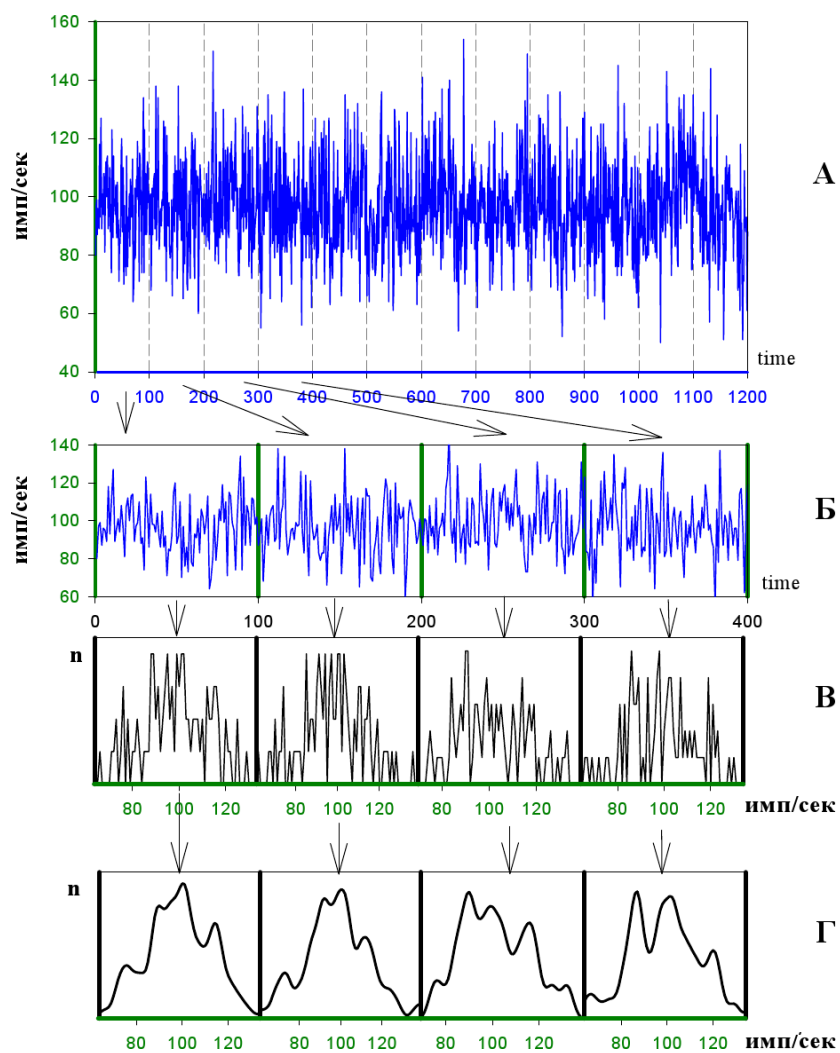
Рис. 2-4: А — изображен “растянутый” фрагмент временного ряда результатов измерения альфа-активности препарата ^{239}\text{Pu} . Б — временной ряд поделен на неперекрывающиеся отрезки по 100 последовательных чисел в каждом. В — для каждого отрезка построена гистограмма (оси абсцисс — величина активности имп/сек; по оси ординат число измерений, соответствующее данной величине активности). Г — закономерности проявляются в результате сглаживания “скользящим суммированием” или с “окном”, равным, например, 4.
