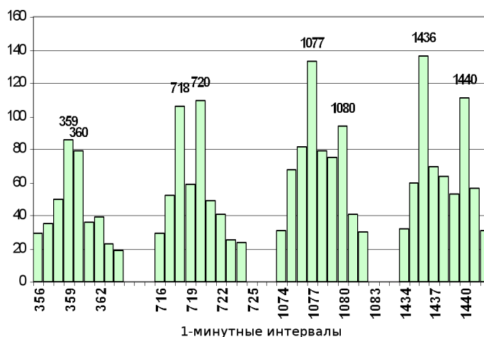
Рис. 13-3: Сравнение одномоментных гистограмм. При 4-х оборотах в сутки против часовой стрелки коллиматора, вырезающего узкий пучок альфа-частиц, вылетающих при радиоактивном распаде ^{239}\text{Pu} , сходные гистограммы реализуются с периодами соответствующими долям звездных и солнечных суток. Один оборот совершается за 360 минут. При этом вероятность реализации сходных 1-минутных гистограмм возрастает с периодом, равным 359 и 360 минутам. При совершении двух оборотов вероятность появления сходных гистограмм возрастает, соответственно, через 359 \times 2 = 718 минут и 360 \times 2 = 720 минут. При совершении трех оборотов эти величины равны 359 \times 3 = 1077 минутам и 360 \times 3 = 1080 минутам и при четырех оборотах равны 359 \times 4 = 1436 и 1440 минутам, соответственно. Измерения 27.05.2004–09.06.2004 г. Ордината — число сходных пар гистограмм; абсцисса — число 1-минутных интервалов.
