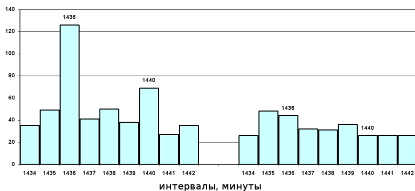
Рис. 13-6: 1-минутные гистограммы. Один оборот коллиматора по часовой стрелке компенсирует вращение Земли и приводит к исчезновению суточных (звездного и солнечного) периодов. (Левый график — контроль: неподвижный западный коллиматор; правый график — вращаемый коллиматор.) Опыт 8–10 июня 2004 г.
