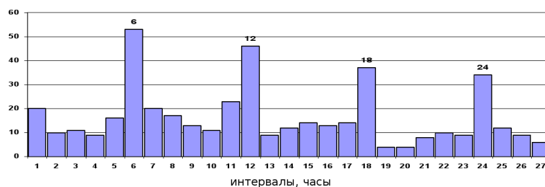
Рис. 13-1: Сравнение 60-минутных гистограмм. При 4-х оборотах в сутки против часовой стрелки коллиматора, вырезающего узкий пучок альфа-частиц, вылетающих при радиоактивном распаде ^{239}\text{Pu} , вероятность реализации сходных одночасовых гистограмм возрастает с периодом, равным 6 часам. Измерения 27.05.2004–09.06.2004 г. Ордината — число сходных пар гистограмм; абсциса — интервалы (часы).
