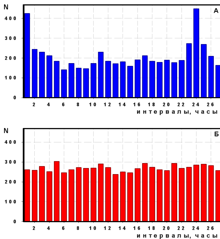
Рис. 11-2: Распределение интервалов между сходными гистограммами зависит от направления, в котором вылетают альфа-частицы при измерениях альфа-распада ^{239}\text{Pu} . Измерения январь-июнь 2002 г. А: измерения плоским детектором потока альфа частиц от плоского образца, ориентированного на Запад. Б: Измерения потока альфа частиц, проходящих до детектора через узкий коллиматор, направленный на Полярную звезду. По оси ординат — число пар гистограмм, соответствующее данному интервалу. В “контроле”, как обычно, наблюдается четкий “эффект ближней зоны” и околосуточный период.
