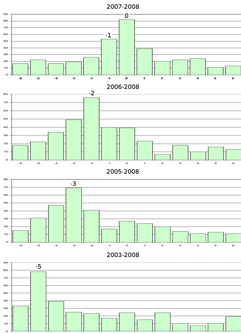
Рис. 10-12: Ежегодный одноминутный сдвиг Галактического годичного периода при сравнении с Календарным, при измерениях альфа-активности ^{239}\text{Pu} на ст. Новолазаревская С. Н. Шаповаловым в 2003–2008 г.г. Одноминутные интервалы.
