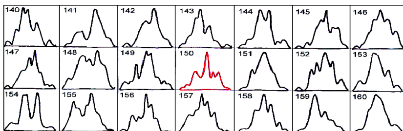
Рис. 17-2-2: Измерения 29.08.2000 г. в Пушино. Новолуние в 11 ч 21 мин, и соответствует гистограмме № 150, имеющей характерную форму.
