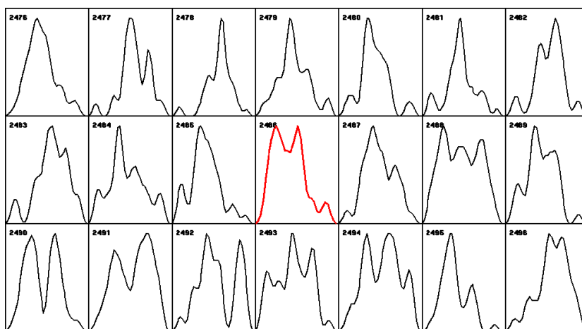
Рис. 19-6: 0,5 минутные гистограммы построены по результатам измерений шумов в генераторе GCP № 28, Princeton, NJ, USA ( 40,35^\circ с.ш., 74,66^\circ з.д.), во время солнечного затмения 8 апреля 2005 г. Гистограмма № 2486 — в центре 2-й строки — с точностью в 0,5 минуты соответствует моменту максимума затмения.
