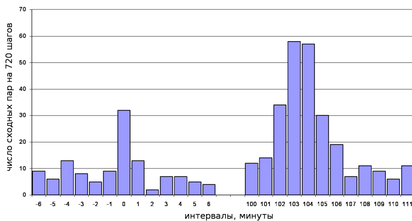
Рис. 7-10: При построении 1-минутных гистограмм по результатам измерений альфа-активности ^{239}\text{Pu} счетчиками без коллиматоров в Пущино и в Новолазаревской наблюдается синхронность по местному времени и практически отсутствует абсолютная синхронность Измерения 24 января 2008 г.
