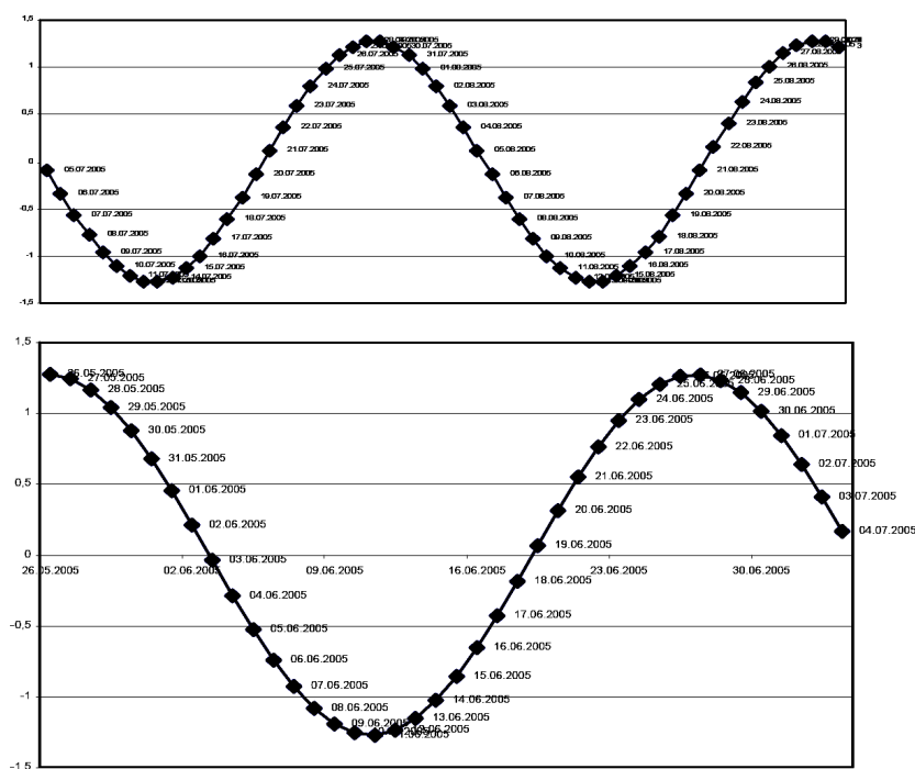
Рис. 20-7: Феномен эвекции — периодическое изменение степени искажения кеплеровской орбиты Луны в июле-августе 2005 года. Максимумы эвекции: 26 мая; 26 июня, 27 июля; 28–29 августа; 29–30 сентября; 1 ноября; 2 декабря. Минимумы: 10 июня, 11–12 июля, 12–13 августа; 13–14 сентября; 15–16 октября; 16 ноября.
