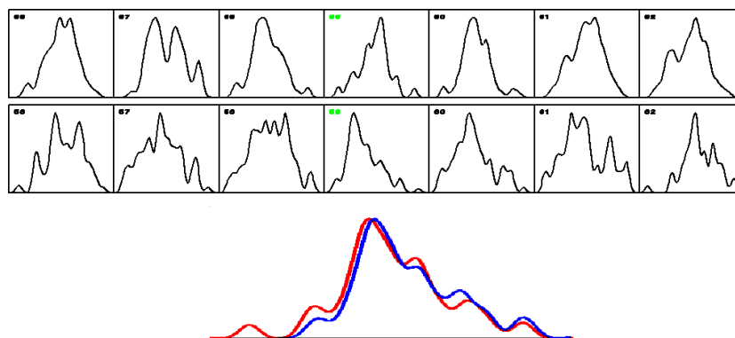
Рис. 19-17: Характерная “переходная” форма 1-минутных гистограмм наблюдается за 1 минуту до времени максимума затмения и 4 декабря 2002 г. и 24 ноября 2003 г. Измерения альфа-активности ^{239}\text{Pu} в Пущино счетчиком с коллиматорами, направленными на Полярную звезду.
