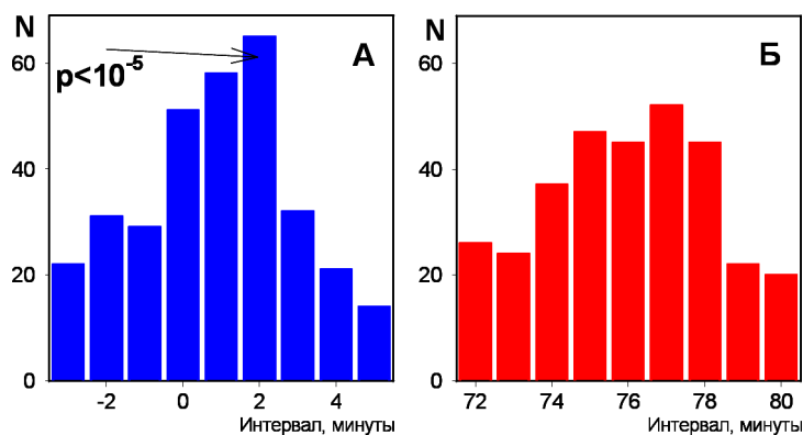
Рис. 7-4: “А” и “Б”: синхронность реализации сходных гистограмм по абсолютному “А” и местному — “Б” — времени при измерениях альфа-активности ^{239}\text{Pu} 2 июня 2001 г. в Пушино и на корабле в Антарктической экспедиции ( 38^{\circ}18' - 35^{\circ}53' ю.ш.; 18^{\circ}27' - 18^{\circ}01' в.д.) Расстояние около 10700 км. Расчетная разность местного времени 76–77 минут. Абсциссы — интервалы времени между сходными одномоментными гистограммами. Нуль соответствует одинаковому абсолютному времени в Пушино и на корабле. Ординаты — числа сходных пар гистограмм, соответствующие данной величине интервала. Оценка P_i по гипергеометрическому распределению.
