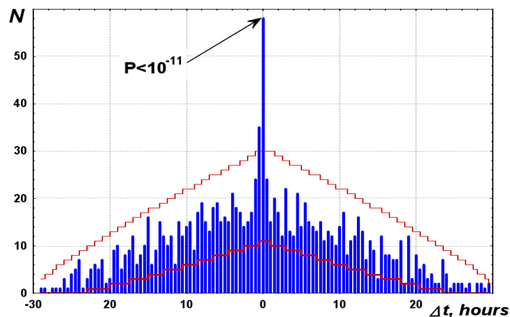
Рис. 3-8: Синхронность изменения формы 1-часовых гистограмм, построенных по измерениям интенсивности потока нейтронов из земной коры в НИИЯФ МГУ (Б. М. Кузевский), в Москве, и альфа-активности ^{239}\text{Pu} в ИТЭБ РАН, в Пущино (К. И. Зенченко и В. А. Коломбет) 27–31 декабря 1997 г. Сравнение гистограмм в рандомизированных рядах провела Т. А. Зенченко [43]. Оценка P_i по гипергеометрическому распределению.
