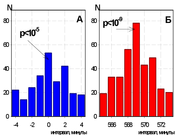
Рис. 7-1: “А” и “Б”: синхронность реализации сходных гистограмм по абсолютному “А” и местному — “Б” — времени при измерениях альфа-активности ^{239}\text{Pu} 31 августа 2000 г. в Пуццо (К. И. Зенченко) и в Арктике ( 82^\circ с.ш.; 179^\circ з.д.) (С. Н. Шаповалов). Расчетная разность местного времени 572 минуты. Абсциссы — интервалы времени между сходными одномоментными гистограммами. Нуль соответствует одинаковому абсолютному времени в Пуццо и в Арктике. Ординаты — числа сходных пар гистограмм, соответствующие данной величине интервала. Оценка P_i по гипергеометрическому распределению.
