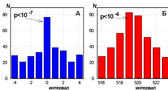
Рис. 7-2: “А” и “Б”: синхронность реализации сходных гистограмм по абсолютному “А” и местному — “Б” — времени при измерениях альфа-активности ^{239}\text{Pu} 11 сентября 2000 г. в Пуццо (К. И. Зенченко) и в Арктике ( 82^\circ с.ш.; 167^\circ 53' в.д.) (С. Н. Шаповалов). Расчетная разность местного времени 521 минута. Абсциссы — интервалы времени между сходными одномоментными гистограммами. Нуль соответствует одинаковому абсолютному времени в Пуццо и в Арктике. Ординаты — числа сходных пар гистограмм, соответствующие данной величине интервала [3] Оценка P_i по гипергеометрическому распределению.
