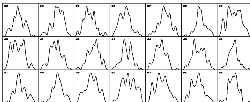
Рис. 19-2: Фрагмент компьютерного журнала — последовательность гистограмм, построенных каждая по 60-ти одnoseкундных измерений альфа-активности образца ^{239}\text{Pu} , неподвижно укрепленном на полупроводниковом детекторе. Указаны номера гистограмм в ряду. Номера соответствуют числу минут от 00 ч московского зимнего времени 09.04.2005. Форма одноминутной гистограммы № 43 (в центре 2-й строки), построенной по результатам измерений во время максимума затмения, отличается от формы других гистограмм. Оси абсцисс каждой гистограммы — результаты измерений. Оси ординат — числа измерений, соответствующие данной величине результата. Гистограммы сглажены 11-кратным скользящим суммированием.
