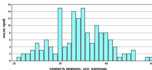
Рис. 4: Гистограмма — распределение результатов измерений в опыте 30 мая 1978 г. По оси ординат — число проб с данной активностью.
