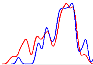
Рис. 18-3-6: Полнолуния 29 января в момент максимума и 23 августа 2002 года за 2 минуты до максимума.
