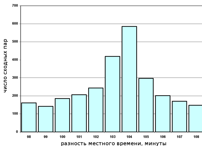
Рис. 7-9: Эффект синхронного по местному времени появления сходных гистограмм в Пуцино и на станции Новолазаревская в Антарктиде. Средние данные из 7-ми опытов рис. 26 [53].
