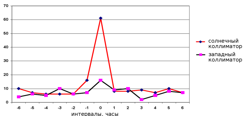
Рис. 7-14: При построении 60-минутных гистограмм по результатам измерений альфа-активности ^{239}\text{Pu} в Пуццино счетчиком с коллиматором, направленным на Солнце, и в Новолазаревской счетчиком без коллиматора (также как при построении 1-минутных гистограмм) наблюдается четкая абсолютная синхронность с Антарктикой. При измерениях в Пуццино счетчиком с коллиматором, направленным на Запад совсем нет абсолютной синхронности.
