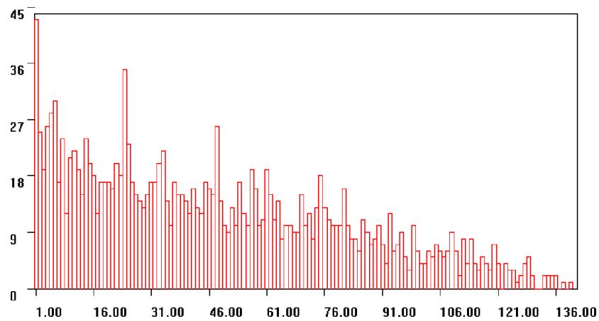
Рис. 5-3: Результаты сравнения одночасовых гистограмм, построенных по результатам измерений альфа-активности ^{239}\text{Pu} с 7 по 15 июля 2000 г. в Пуцзино. Всего в ряду было 143 часовых гистограммы. Сравнение с полным перемешиванием (рандомизацией) выполнила Т. А. Зенченко. Выбрано 1592 схожих пары. По абсциссе — интервалы (часы). Прекрасно видны ближняя зона, пики на 24 и 48 часах.
