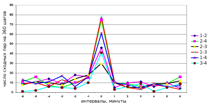
Рис. 7-15: В 1-минутных гистограммах (результаты измерений альфа-активности ^{239}\text{Pu} 15 октября 2005 г. в Пуццино счетчиком с коллиматором, направленным на Полярную звезду, и в Новолазаревской счетчиком без коллиматора) наблюдается: 1) “сильная” абсолютная синхронность изменения гистограмм при измерениях в Пуццино (№ 1): при измерениях без коллиматора и в Пуццино с Западным коллиматором (№ 3); 2) “сильная” абсолютная синхронность в Пуццино с коллиматором, направленным на Солнце (№ 2) и в Новолазаревской (без коллиматора) (№ 4); 3) “средняя” абсолютная синхронность при измерениях в Пуццино (№ 1) и в Новолазаревской (№ 4) без коллиматоров; 4) “слабая” абсолютная синхронность при измерениях в Пуццино с Западным коллиматором (№ 3) и в Новолазаревской без коллиматора (№ 4); 5) “слабая” абсолютная синхронность в Пуццино без коллиматора (№ 1) и счетчика с Солнечным коллиматором (№ 2). 6) № 2–3: отсутствует абсолютная синхронность при измерениях в Пуццино с “солнечным” (№ 2) и “Западным” (№ 3) коллиматорами, находящимися рядом в Пуццино.
