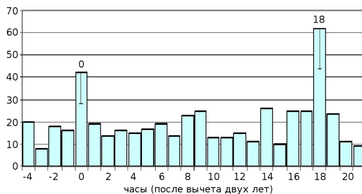
Рис. 10-8: С точностью до 1 часа сходные гистограммы реализуются ровно через три года и через 3 года 18 часов. Измерения альфа-активности ^{239}\text{Pu} — август-октябрь 2000–2003 г. По оси абсцисс — часы — интервалы времени появления сходных гистограмм после вычитания числа часов за 3 года. По оси ординат — число пар сходных гистограмм, соответствующих данной величине интервала.
