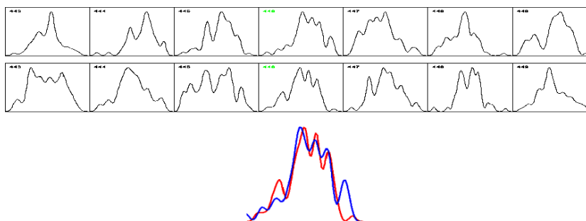
Рис. 15-2Б: Сходные гистограммы (№ 446, № 446) наблюдались на 1 минуту позже календарного времени Восхода Солнца 28 октября 2000 и 2004г.г. Измерения альфа-активности ^{239}\text{Pu} в 2000 г. — плоским полупроводниковым детектором; в 2004 г. — измерения с неподвижным коллиматором, направленным на Запад.
