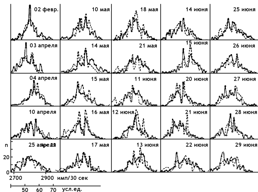
Рис. 31: Форма гистограмм, построенных по результатам 250 синхронных измерений альфа-активности в Москве (МИФИ, Н. Б. Хохлов, М. П. Шарапов) и скорости реакции АК + ДХФИФ в Пуцино (С. Э. Шноль, Т. Я. Брицина и Н. П. Иванова) сходна в разные дни 1984 г.
