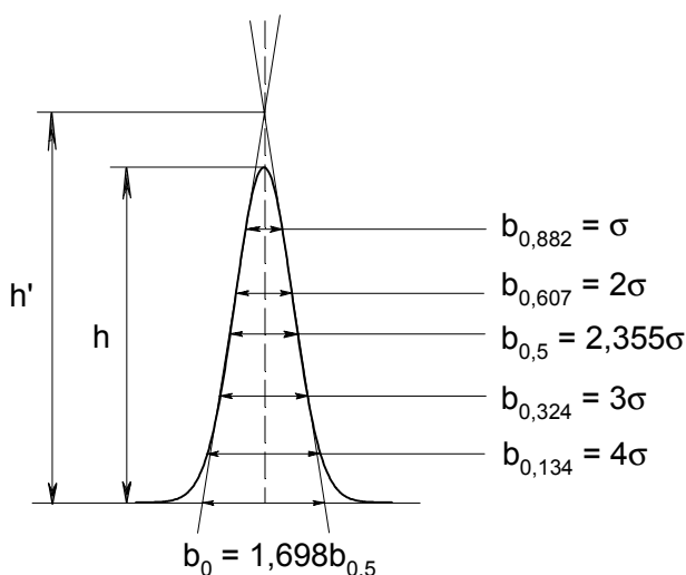
Рисунок 27 – Свойства гауссовского пика:
