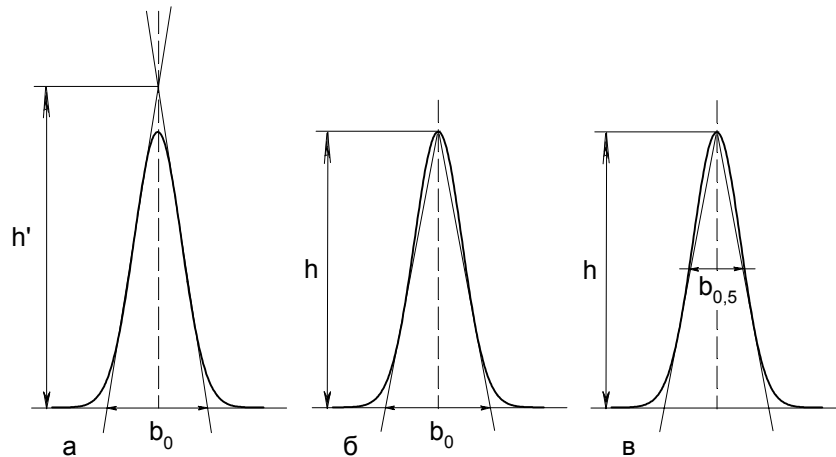
Рисунок 30 – Методы триангуляции:
