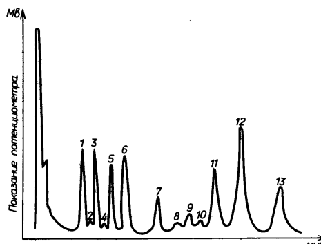
Рисунок 35 – Хроматограмма модельной смеси ТМС производных моносахаридов:
