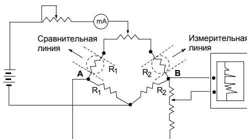
Рисунок 18 – Схема включения двухплечевого катарометра в измерительный мост
