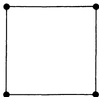
Рисунок 7.21. Кандидаты в подграфы
