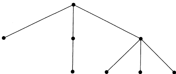
Рисунок 7.16. Схема генеалогического дерева Бернулли
