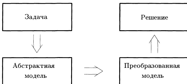
Рисунок 1.1. Схема моделирования
