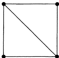
Рисунок 7.21. Кандидаты в подграфы
