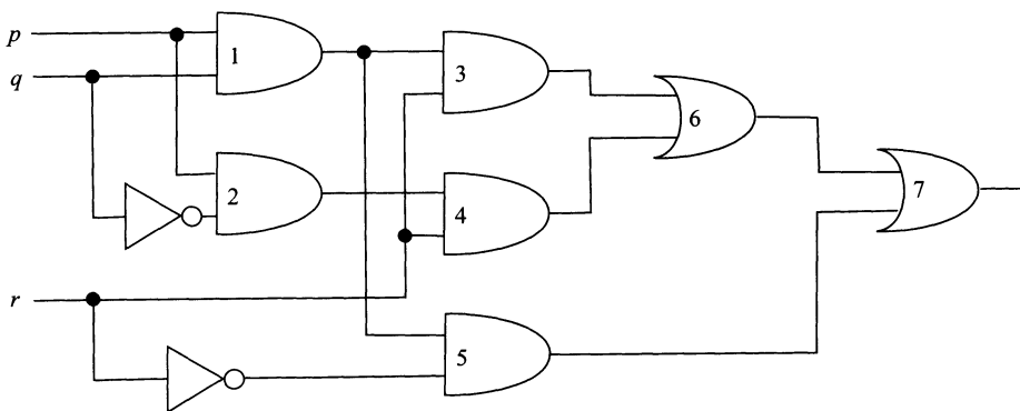
Рисунок 9.9. Функциональная схема
