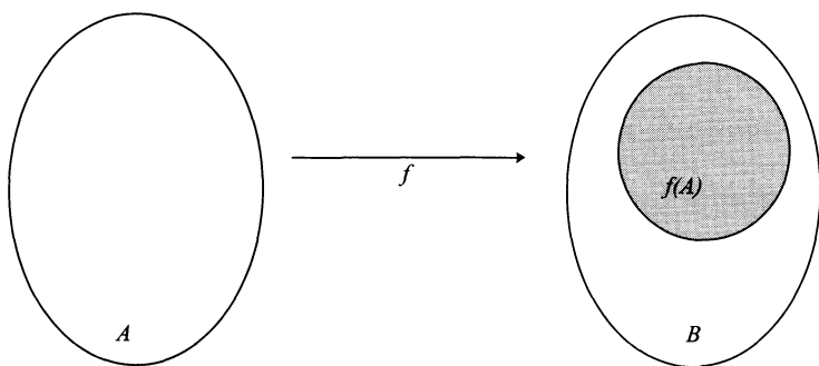
Рисунок 5.4. Диаграмма Венна функции f : A \longrightarrow B
