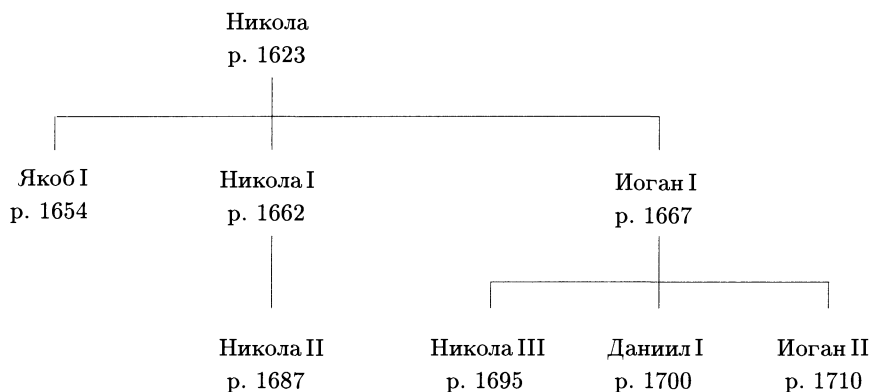
Рисунок 7.15. Династия Бернулли
