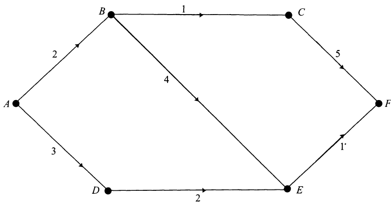
Рисунок 8.5. Нагруженный граф
