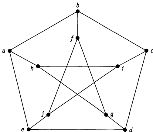
Рисунок 7.23. Граф Петерсена
