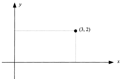
Рисунок 3.9. Декартова плоскость
