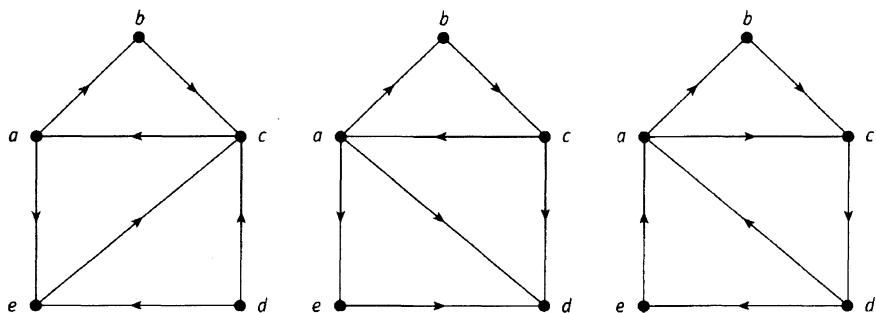
Рисунок 8.6. Связные орграфы
