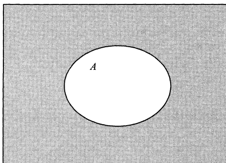
Рисунок 3.5. Диаграмма Венна дополнения \overline{A}
