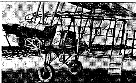
Конструктивные детали аэроплана S-29A. Установка бензиновых и ма- сляных баков сза- ди моторов.
