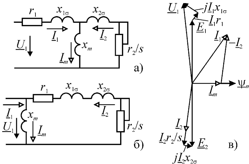
Рис. 1.7. Схема замещения и векторная диаграмма АД
