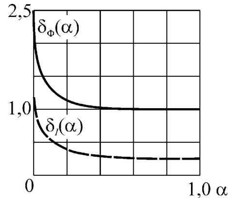
Рис. 2.7. Изменение магнитного потока и тока намагничивания АД при стабилизации располагаемого момента.
