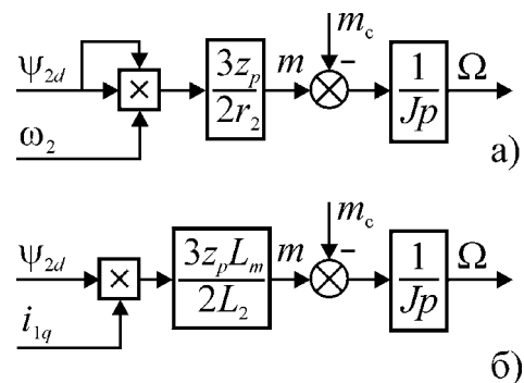
Рис. 2.21. Эквивалентные структурные схемы АД при трансекторном управлении различными входными сигналами.
