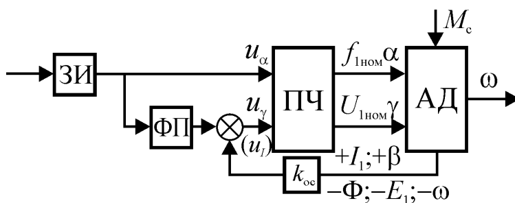
Рис. 2.8. Функциональная схема замкнутой системы частотного управления
