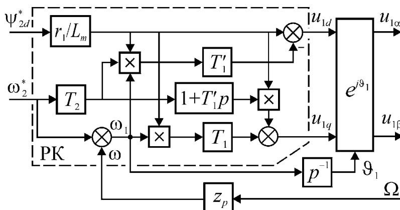
Рис. 2.22. Структурная схема устройства управления напряжением
