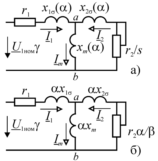
Рис. 2.1. Схема замещения АД при частотном управлении
