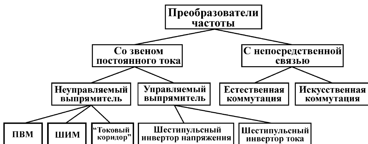
Рис. 2.32. Основные типы преобразователей
