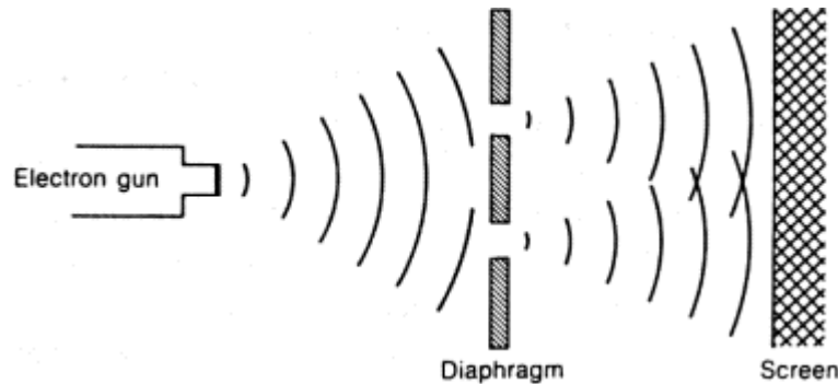
Рис. 13.1. Дифракция электронов
