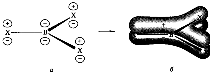
Рис. 4.7. Схема образования p\pi - p\pi -связей в тригалогенидах бора:
