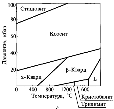
Рис. 5.20. Взаимные переходы между различными модификациями \text{SiO}_2 ( a ); строение \alpha -кварца ( б ); строение \alpha -кристаллита (показаны кремний-кислородные тетраэдры) ( в ); фазовая диаграмма \text{SiO}_2 ( г )
