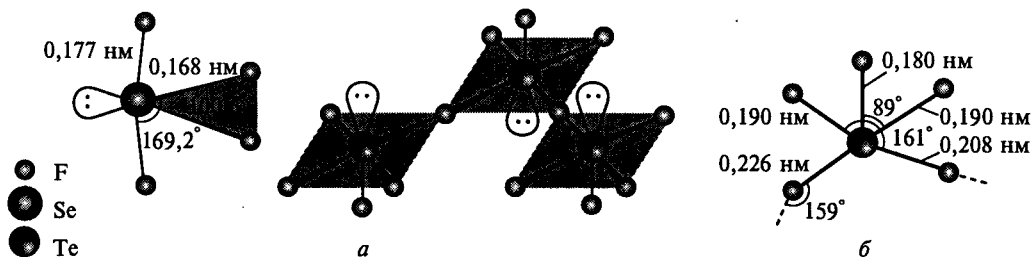
Рис. 7.25. Строение молекул:
