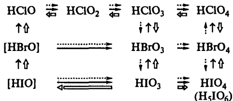
Рис. 8.16. Увеличение силы кислот ( \rightarrow ), термодинамической стабильности ( \cdots\rightarrow ) и окислительной способности ( \Rightarrow ) оксокислот галогенов
