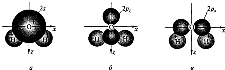
Рис. 1.8. Перекрытие орбиталей 2s (а), 2p_z (б), 2p_x (в) атома кислорода с орбиталями 1s двух атомов водорода молекулы воды
