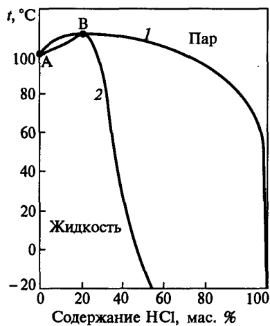
Рис. 8.10. Фазовое равновесие жидкость — пар в системе НF—Н 2 О (а) и НCl—Н 2 О (б) при P = 1 атм
