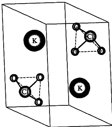
Рис. 8.14. Строение бертолетовой соли \text{KClO}_3
