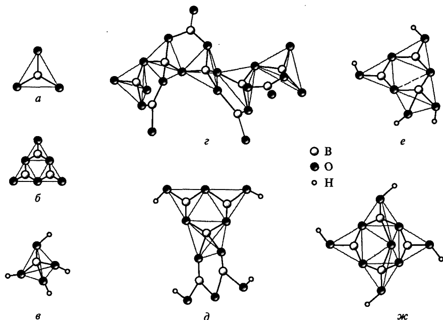
Рис. 4.10. Строение борат-анионов:
