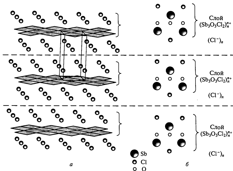
Рис. 6.28. Строение молекулы хлорида антимоила \text{SbOCl} :
