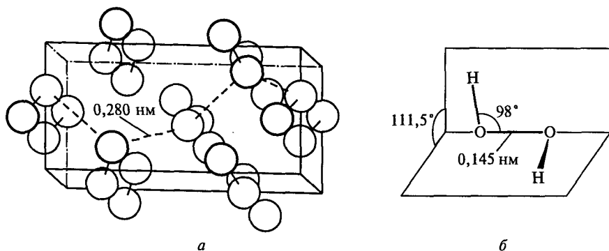
Рис. 1.18. Строение кристалла (а) пероксида водорода (атомы Н не показаны) и отдельной молекулы \text{H}_2\text{O}_2 (б) в кристалле
