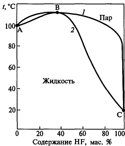
Рис. 8.10. Фазовое равновесие жидкость — пар в системе НF—Н 2 О (а) и НCl—Н 2 О (б) при P = 1 атм
