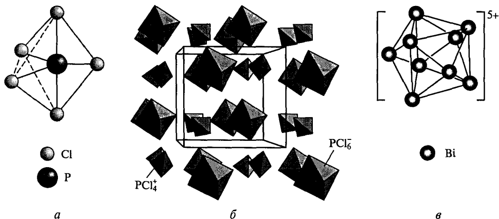
Рис. 6.32. Строение молекулы \text{PCl}_5 в газовой фазе (а); кристалла \text{PCl}_5 (б); иона [\text{Bi}_9]^{5+} (в)
