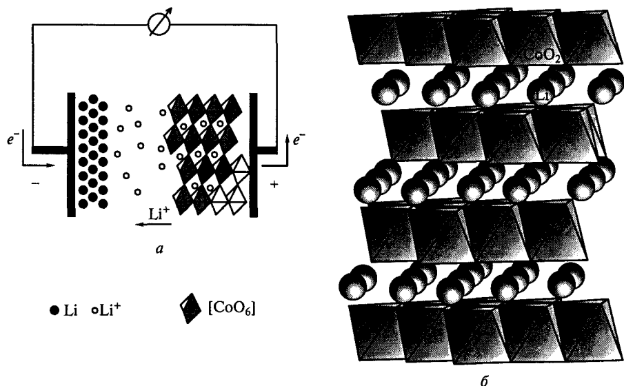
Рис. 2.2. Схема работы литиевого элемента при разрядке (а); строение кристалла кобальтита лития (б) (ионы лития расположены между слоями, образованными октаэдрами \text{CoO}_6 )
