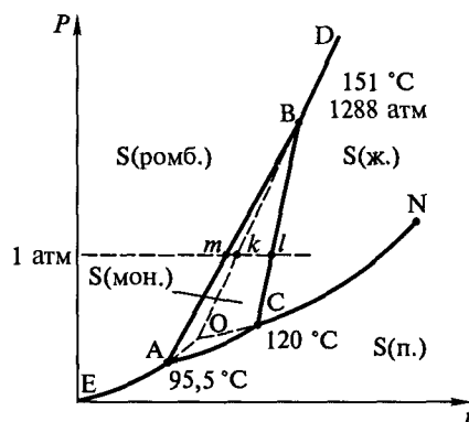
Рис. 7.3. Фазовая диаграмма серы (N — критическая точка)
