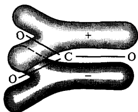
Рис. 5.19. Строение карбонат-иона
