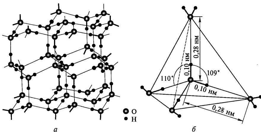
Рис. 1.9. Строение ( a ) и система межмолекулярных связей ( б ) в гексагональной I_h структуре льда
