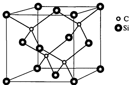
Рис. 5.13. Строение карборунда
