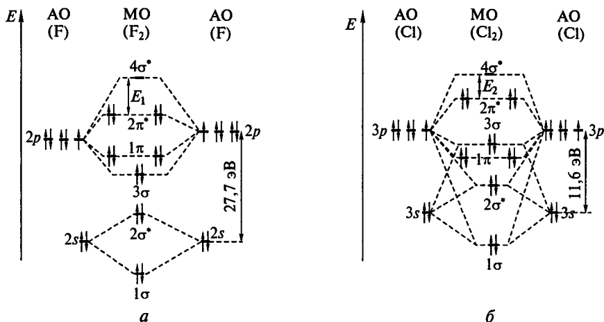
Рис. 8.3. Схема молекулярных орбиталей молекул F_2 (а) и Cl_2 (б)
