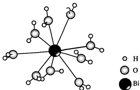
Рис. 6.1. Строение акваиона [\text{Bi}(\text{H}_2\text{O})_9]^{3+}
