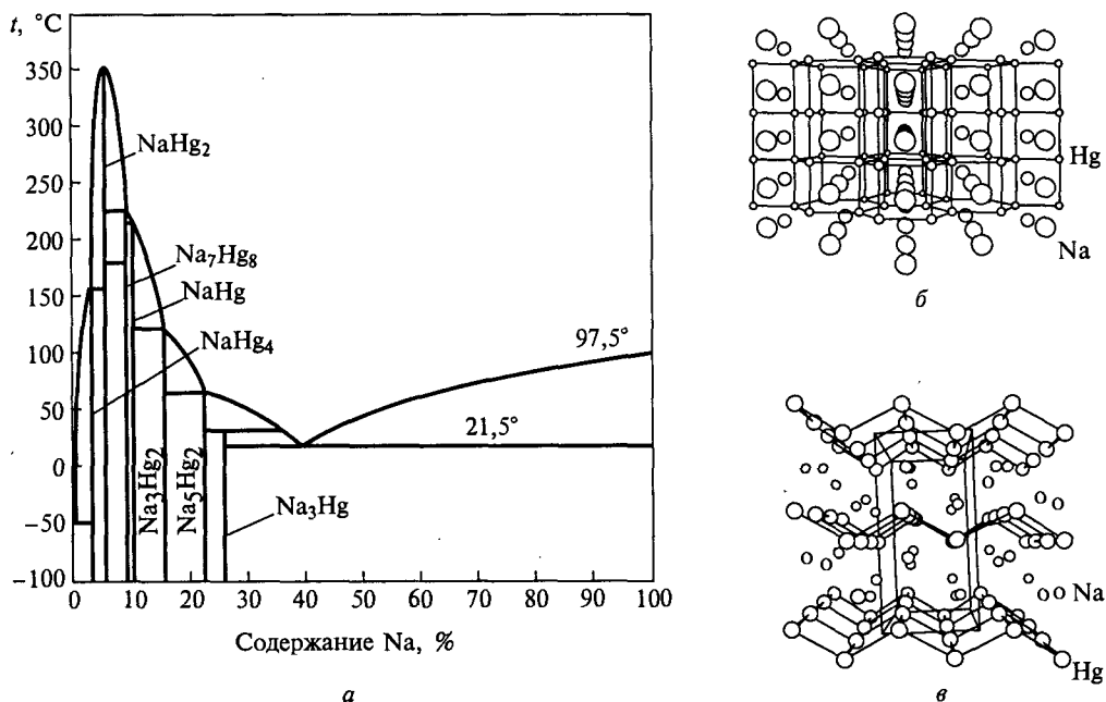
Рис. 2.5. Диаграмма состояния системы Na—Hg (а); схема упаковки атомов натрия и ртути в структуре NaHg_2 (б) и NaHg (в)
