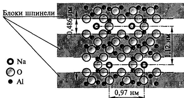
Рис. 4.18. Строение β-глинозема
