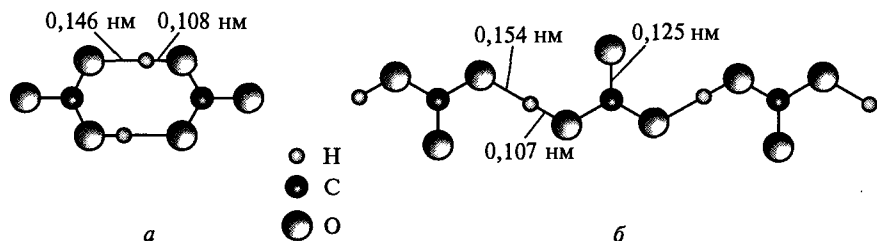
Рис. 2.10. Структуры гидрокарбонатов:
