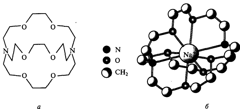
Рис. 2.11. Строение криптанда-222 (а) и катиона в структуре алкалида [\text{Na}(\text{криптанд-222})]^+\text{Na}^- (б)**
