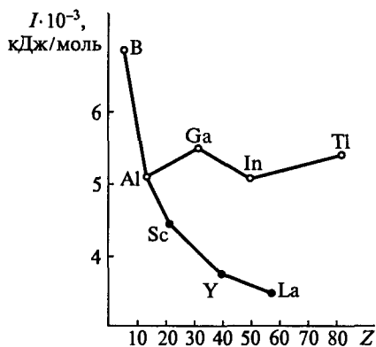
Рис. 4.1. Изменение суммы первых трех энергий ионизации элементов 3-й (Sc, Y, La) и 13-й (B, Al, Ga, In, Tl) групп Периодической системы
