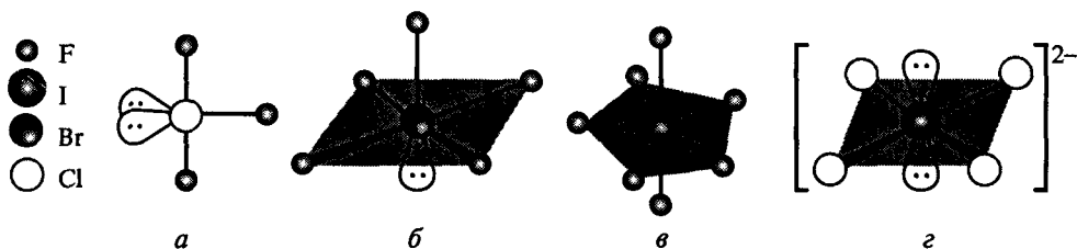
Рис. 8.17. Строение молекул ClF_3 (а), BrF_5 (б), IF_7 (в) и иона ICl_4^{2-} (г)
