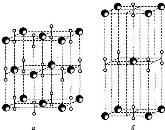
Рис. 3.2. Кристаллическая структура карбида кальция \text{CaC}_2 (a) и пероксида бария \text{BaO}_2 (б)
