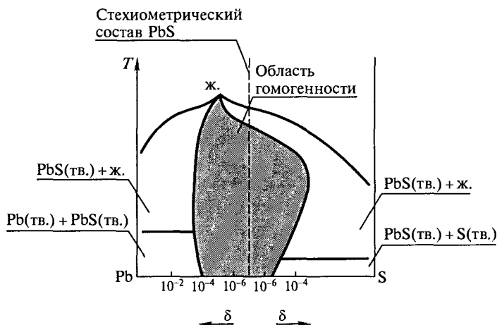
Рис. 1.25. Схема T — x -диаграммы системы с соединением, имеющим область гомогенности
