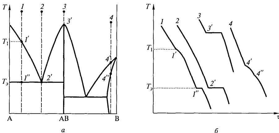
Рис. 1.27. Схема T — x -диаграммы системы А—В (а) и кривые охлаждения (б)
