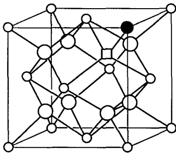
Рис. 4.29. Структура ZrO_2 , легированного CaO .
