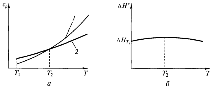
Рис 1.7. Пример зависимости от температуры теплоемкости исходных веществ и продуктов реакции (а), и изменения энтальпии реакции \Delta_r H_T^\circ (б):
