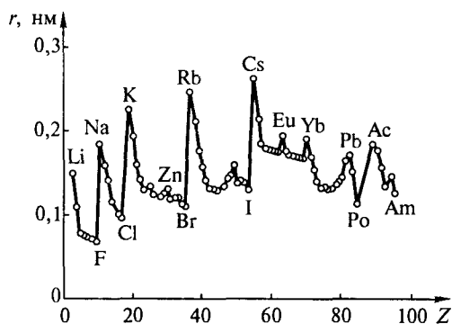
Рис. 3.18. Зависимость радиуса атома ( r ) от порядкового номера элемента ( Z )
