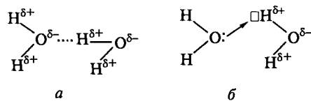
Рис. 4.32. Схема образования водородной связи
