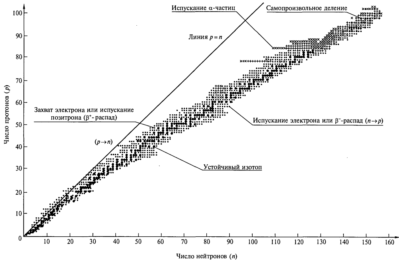
Рис. 3.14. Область существования устойчивых изотопов в зависимости от имеющегося у них числа протонов и нейтронов
