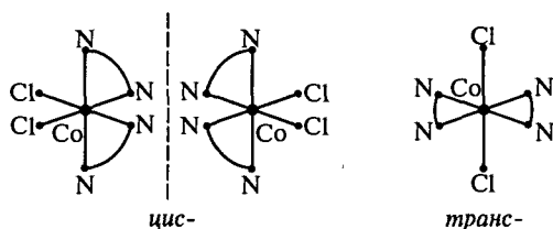
Рис. 4.37. Изомеры [\text{Co}(\text{en})_2\text{Cl}_2]^+
