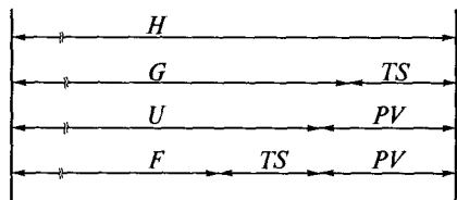
Рис. 1.11. Соотношение между функциями U , H , G и F
