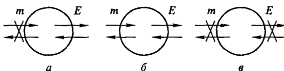
Рис. 1.2. Примеры закрытой (а), открытой (б) и изолированной (в) систем
