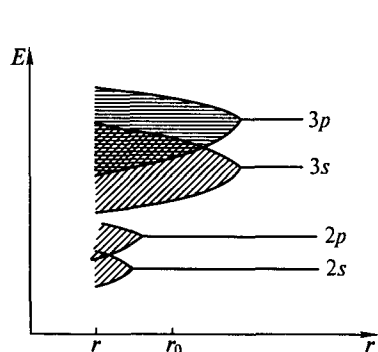
Рис. 4.19. Зависимость степени перекрыwania энергетических зон от расстояния
