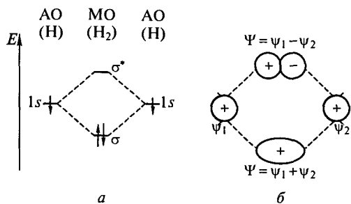
Рис. 4.8. Энергетическая диаграмма МО молекулы водорода (а) и схема образования \sigma -орбиталей (б)
