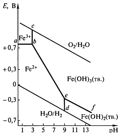
Рис. 1.39. Диаграмма Пурбэ ( E — pH ) для железа в водной среде
