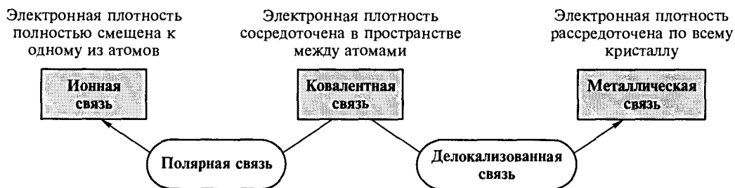
Рис. 4.2. Типы химической связи
