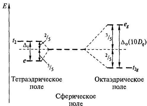
Рис. 4.40. Схема распределения орбиталей по энергиям в октаэдрическом и тетраэдрическом поле лигандов
