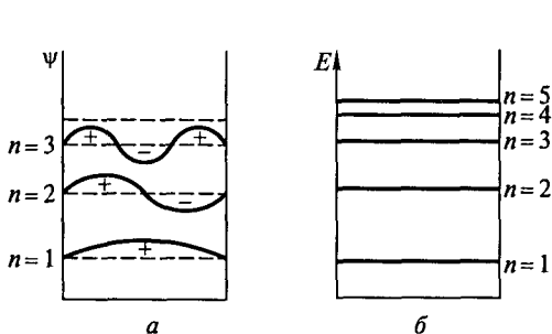
Рис. 3.2. Решение волнового уравнения для случая «электрон в потенциальном ящике»:
