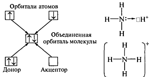
Рис. 4.3. Два механизма образования ковалентной связи
