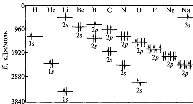
Рис. 3.8. Изменение энергии 1s-, 2s- и 2p-орбиталей у атомов 2-го периода Периодической системы
