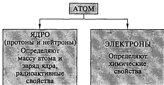
Рис. 3.1. Строение атома
