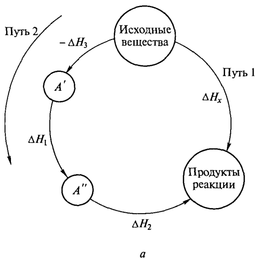
Рис. 1.3. Схема (а) и энтальпийная диаграмма (б), иллюстрирующие изменение энтальпии при взаимодействии газообразного аммиака с раствором хлороводородной кислоты
