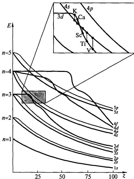
Рис. 3.7. Зависимость энергии орбиталей от заряда ядра ( n — главное квантовое число)
