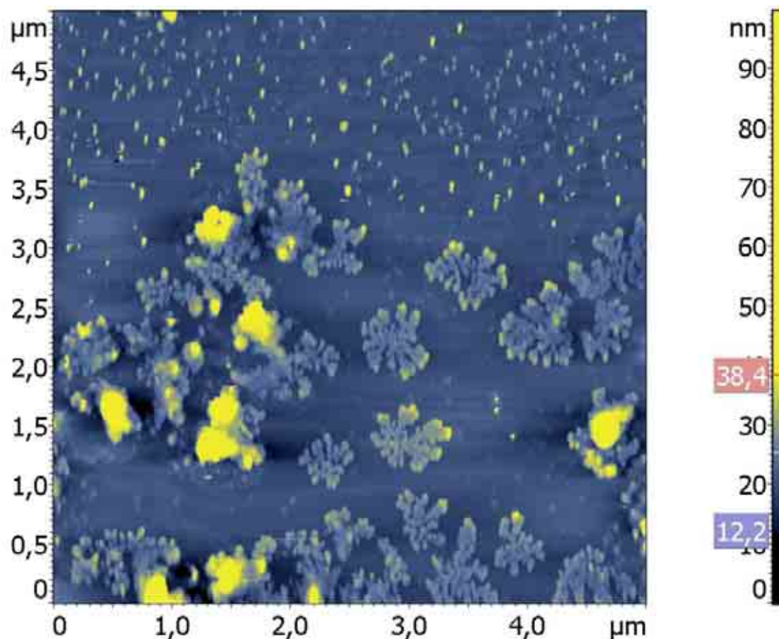
Буферный раствор иммуноглобулина, нанесенный на свежий скол слюды. На слюде образовались дендритные структуры из элементов буферного раствора. (Грищенко Ю.В., Институт кристаллографии им. Шубникова РАН, Россия)
