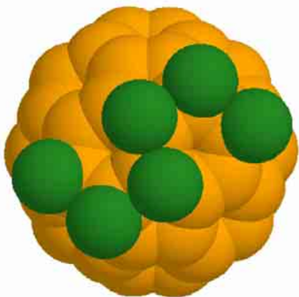
Структура галоген-замещенного фуллера (одна из моделей, предложенная магистрантами и аспирантами ФНМ МГУ в рамках выполнения работ по исследованию структуры, термодинамических свойств и биологической активности фуллеренов)
