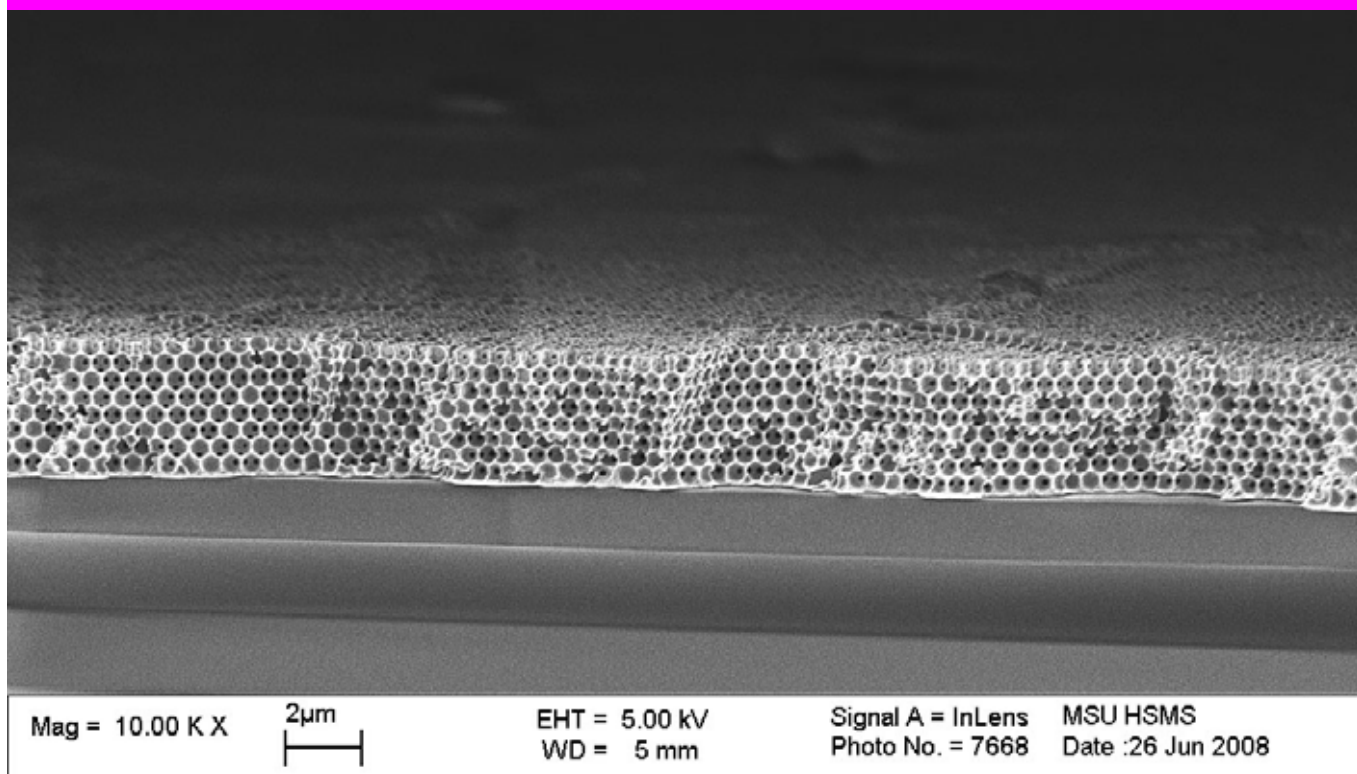
Поперечное сечение металлического фотонного кристалла на поверхности электропроводящего стекла (ITO).
