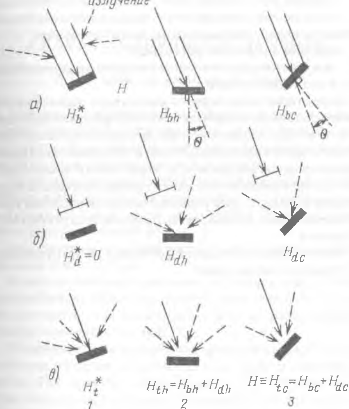
Рисунок 4.3. Способы измерения различных составляющих солнечного излучения:
