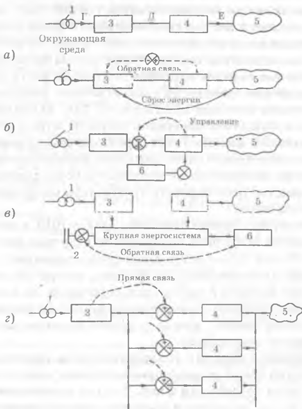
Рисунок 1.3. Схемы согласования ВИЭ с потребителями
