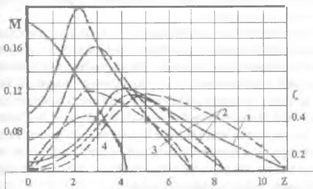
Рисунок 9.12. Характеристики ветроколес различной быстроходности:
