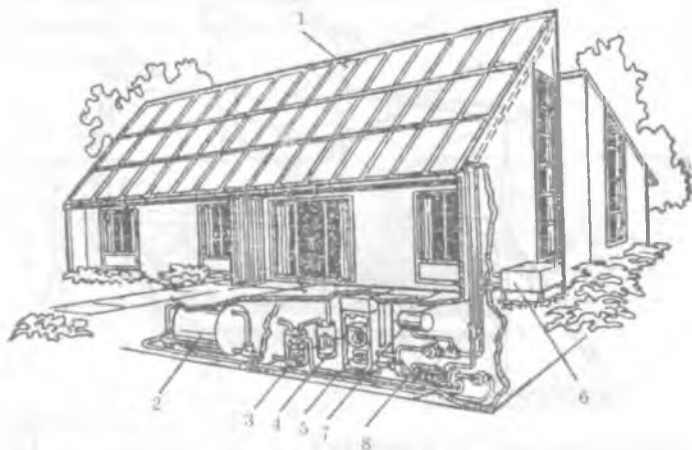
Рисунок 6.4. Дом с активной гелиосистемой теплоснабжения:
