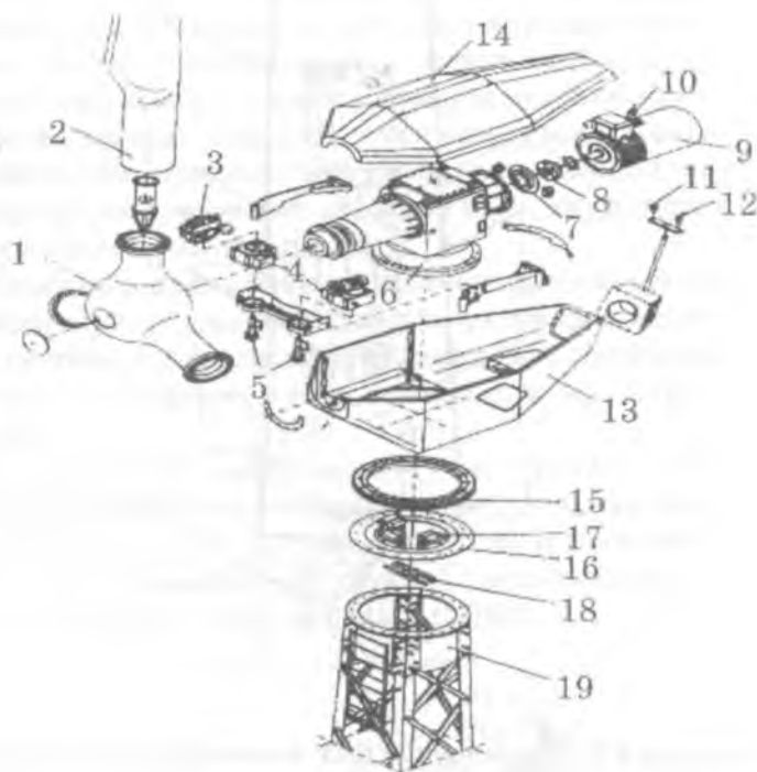
Рисунок 9.8. Компоновка основного энергетического оборудования в гондоле ВЭУ типа «ГЮРЗА»:
