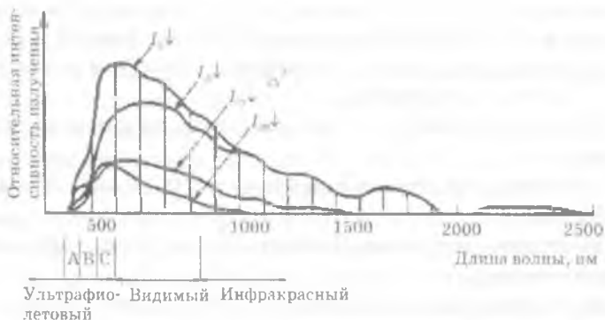
Рисунок 5.2. Спектральный состав суммарной радиации при безоблачном небе
