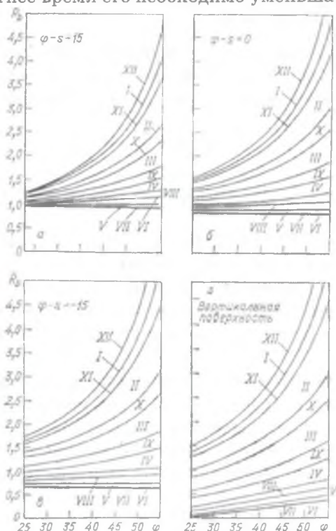
Рисунок 7.12. Величина R_b для ориентированных на юг поверхностей (римскими цифрами указаны месяцы)
