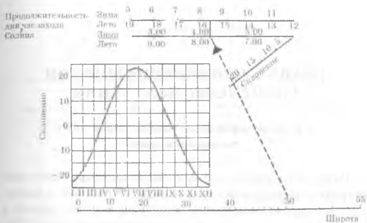
Рисунок 5.11. Определение склонения Солнца, продолжительности светового дня T_c и время захода (восхода)
