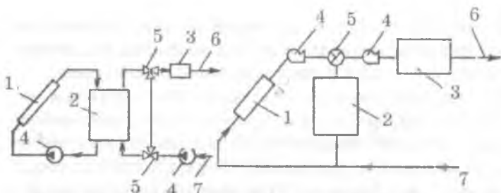
Рисунок 6.5. Принципиальные схемы водяной (а) и воздушной (б) активных систем солнечного отопления:
