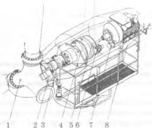
Рисунок 9.6. Конструкция ВЭУ типа «NORD TANK»: 1 – ступица ветроколеса; 2 – гидропривод для тормоза ветроколеса; 3 – главный вал в сборе (вал тормоза и кожух вала); 4 – зубчатая передача; 5 – дисковый тормоз; 6 – вал трансмиссии; 7 – гидропривод для расцепления тормоза; 8 – генератор
