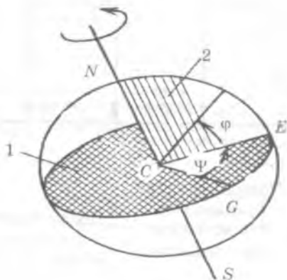
Рисунок 5.7. Схема обращения Земли вокруг своей оси
