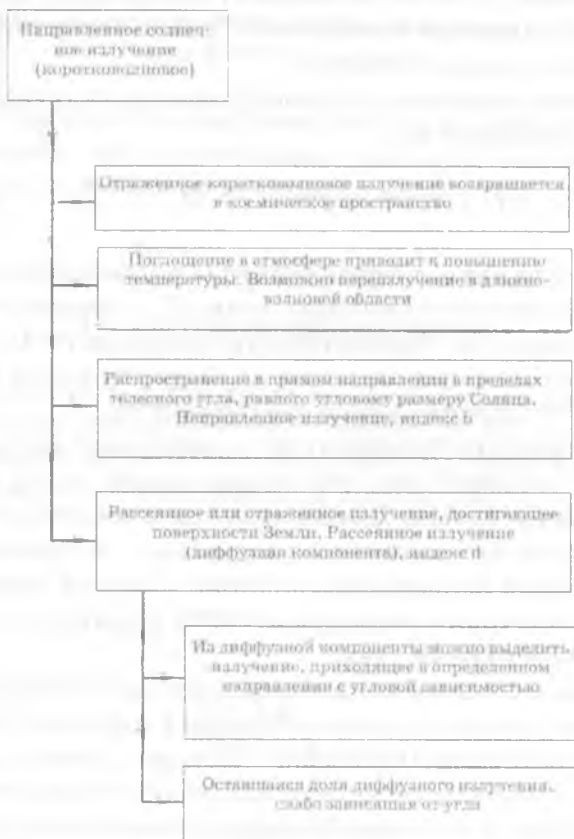
Рисунок 5.5. Прохождение солнечного излучения сквозь атмосферу
