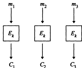
Рис. 5.8. Шифрование в режиме ECB
