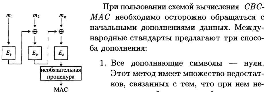
Рис. 5.15. Схема работы СВС-MAC
