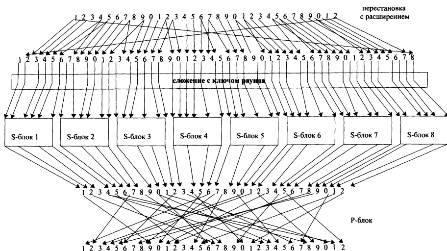
Рис. 5.7. Структура функции F алгоритма DES
