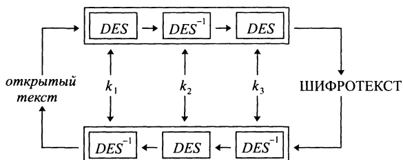
Рис. 5.5. Тройной DES
