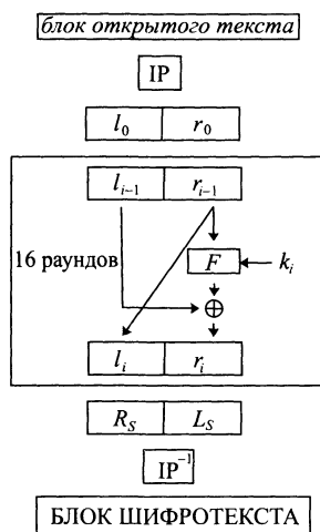
Рис. 5.6. Алгоритмы DES и Фейстеля
