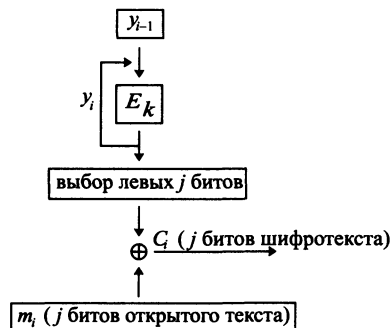
Рис. 5.12. Шифрование в режиме OFB
