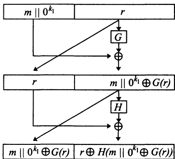
Рис. 17.1. OAEP как сеть Фейстеля
