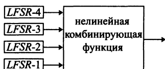
Рис. 5.19. Комбинирование РСЛОС
