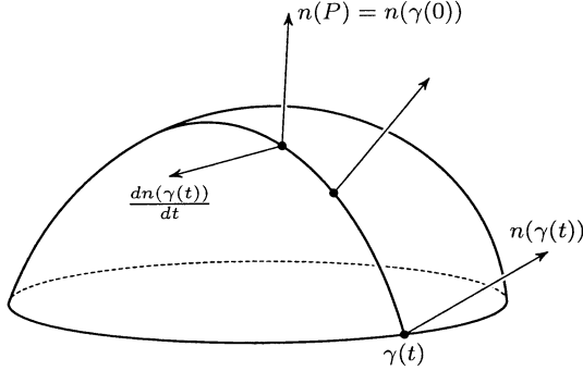
Рис. 7. Оператор Вейнгартена
