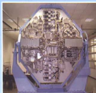
Бортовой ретранслятор для геостационарной орбиты
