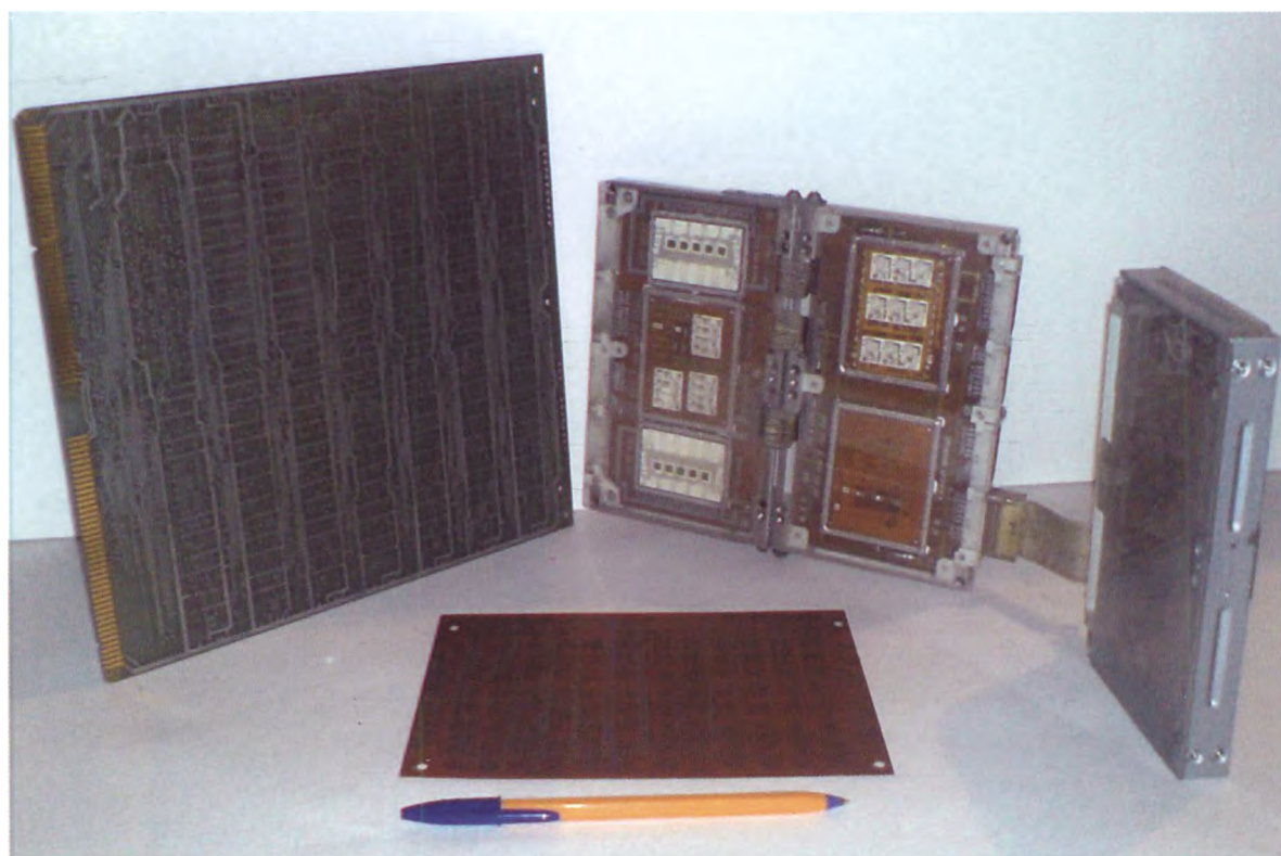
Печатные платы бортовых приборов ТМ-систем. Годы изготовления 1965-1980
