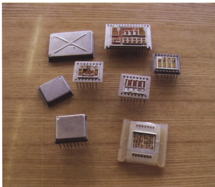
Образцы тонкопленочных микросхем, установленных в корпусах с планарными и штыревыми расположениями выводов. Годы изготовления 1970–1975
