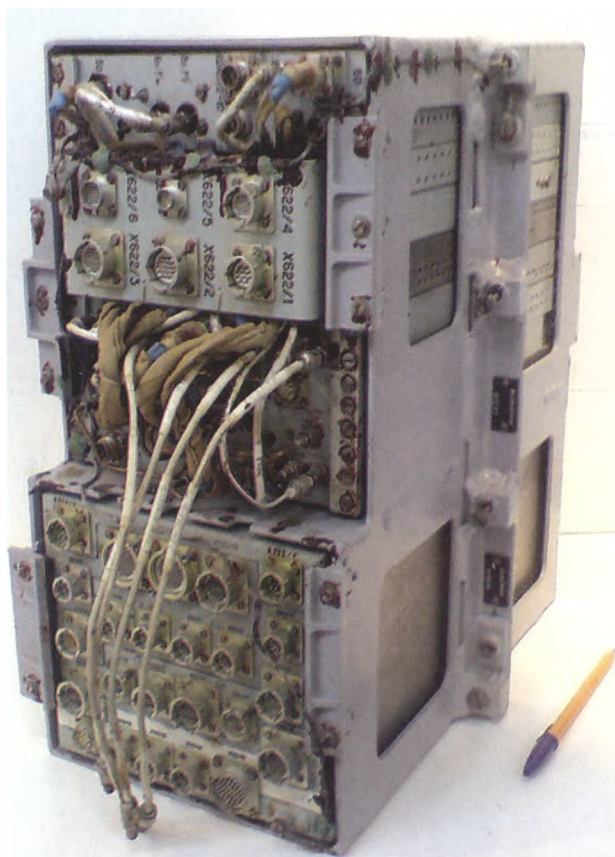
«РЕГУЛ-ОС» Бортовой комплекс управления и связи. Устанавливался на МТКС «Буран», на кораблях «Союз», «Прогресс» и на разгонных блоках. Работает в структуре единого цифрового потока (ЕЦП) как с наземным радиокомплексом КИС «Квант», так и со спутниковым контуром управления через СР «Альтаир». Год разработки – 1985
