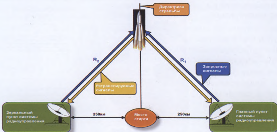
Схема импульсной разностно-дальномерной системы радиоуправления ракетой Р-7 первого этапа. Разработка 1953-1957 гг.
