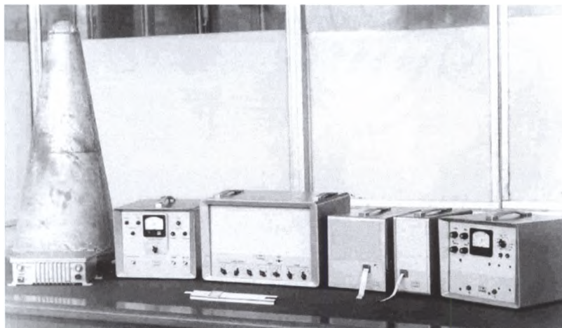
Абонентская навигационная аппаратура первого поколения для гражданских морских судов (1968)
