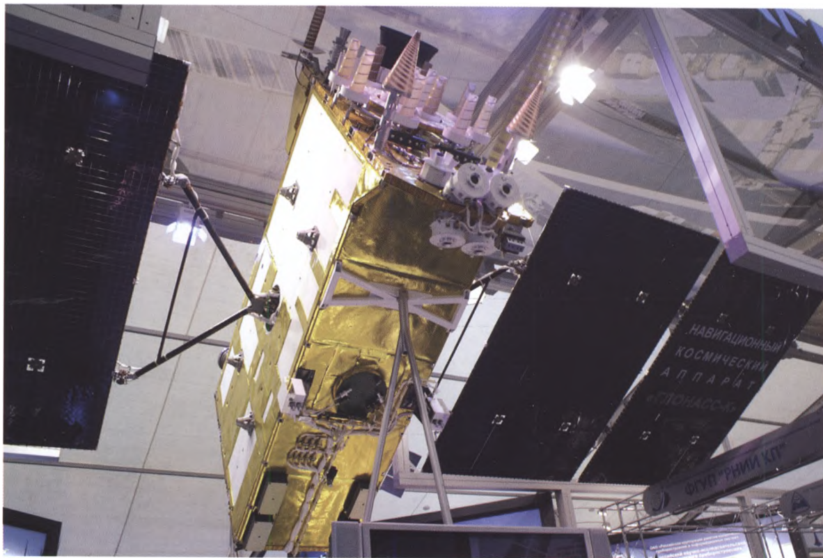
Космический аппарат «Глонасс-К» Третье поколение КА системы ГЛОНАСС. Срок активного существования – 10 лет. Запущен 26 февраля 2011 г.
