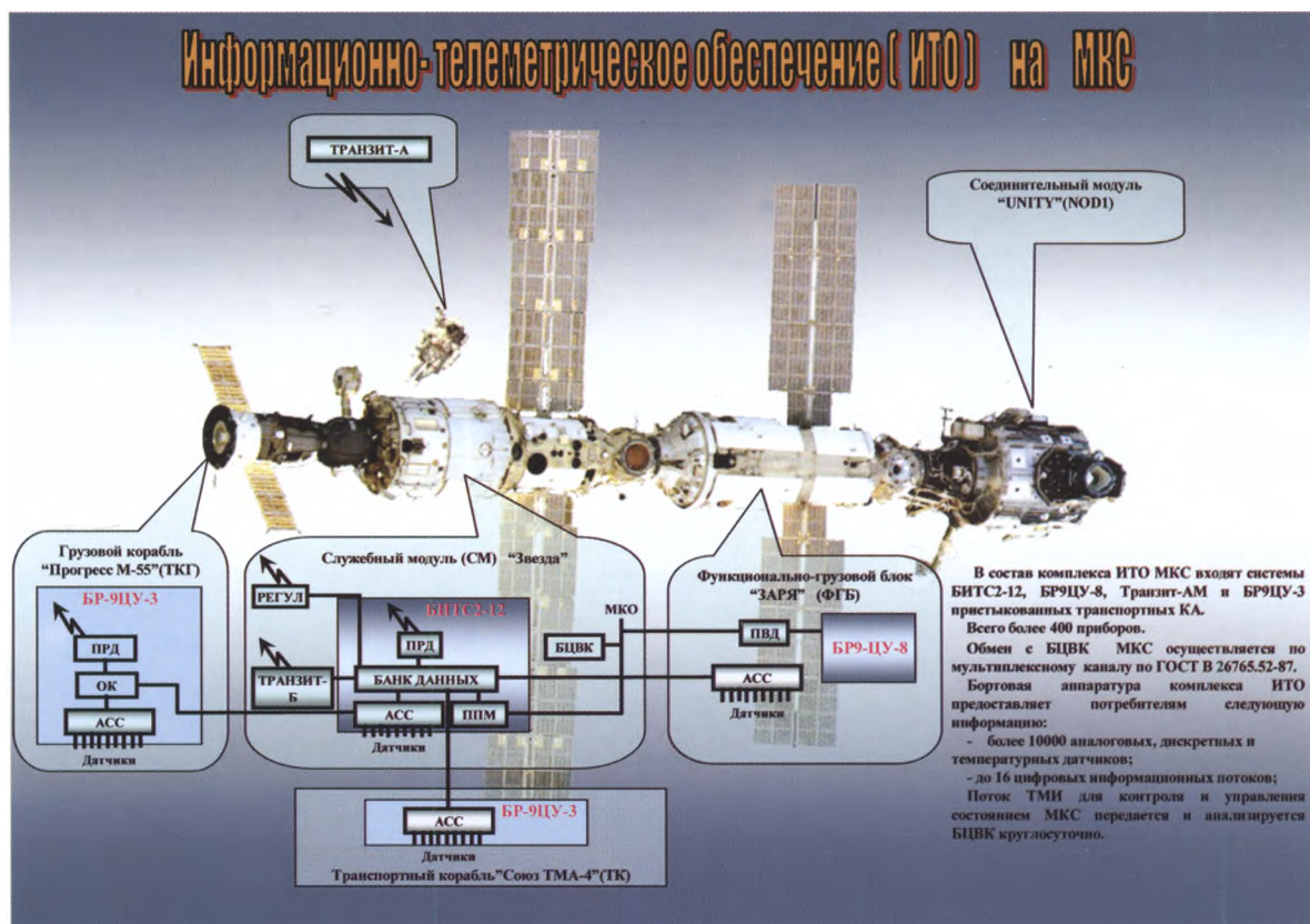
Структура бортовой ТМ-системы международной космической станции (МКС)
