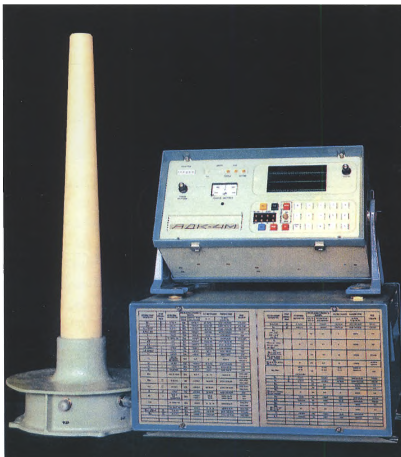
Абонентская навигационная аппаратура второго поколения для гражданских морских судов (1975)
