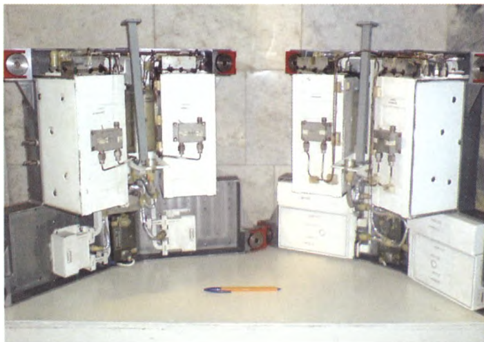
ША317 Дублированный комплект приемного устройства широкополосной радиолinii передачи информации системы «Лира» СМ-диапазона. Применяется в служебном модуле МКС. Год разработки – 1980
