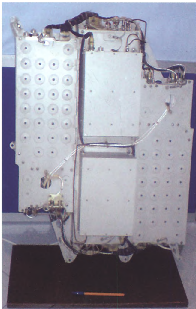
ЦА023 Бортовая навигационная аппаратура первого поколения. Год разработки – 1979
