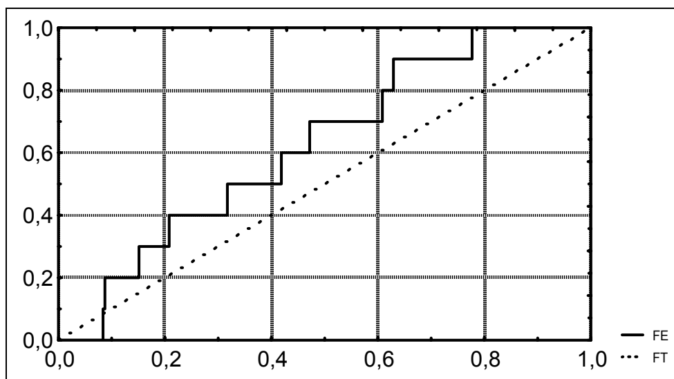
Рис. 7.7. Функции эмпирического FE и теоретического FT распределений равномерно распределенной случайной величины X при числе наблюдений n=10
