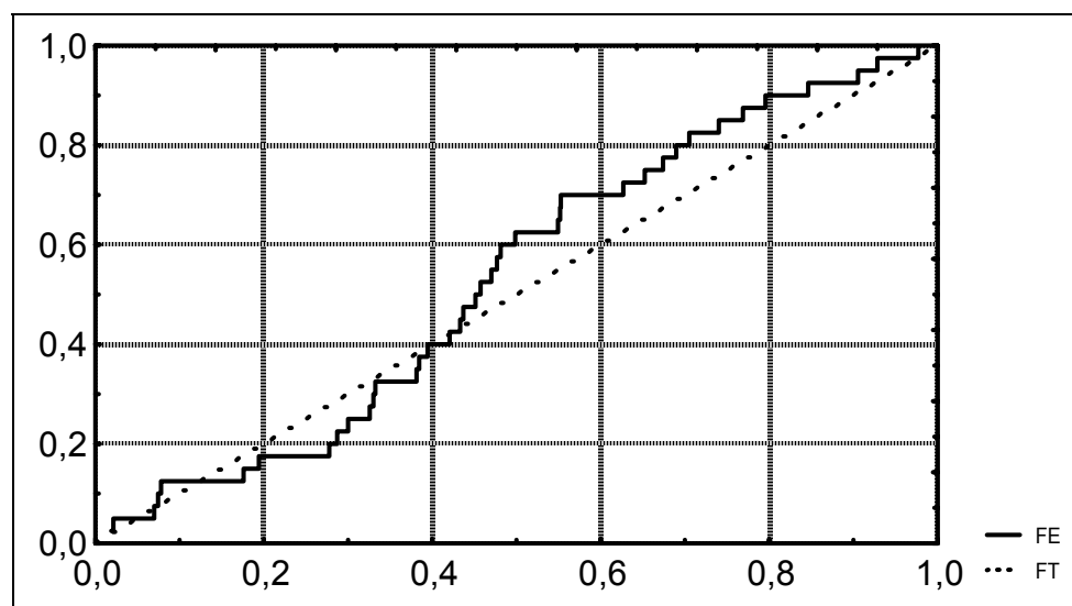
Рис. 7.8. Функции эмпирического FE и теоретического FT распределений равномерно распределенной случайной величины X при числе наблюдений n = 40
