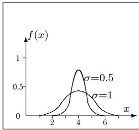
Рис. 6. Распределение Гаусса
