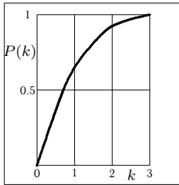
Рис. 5. P(k)
