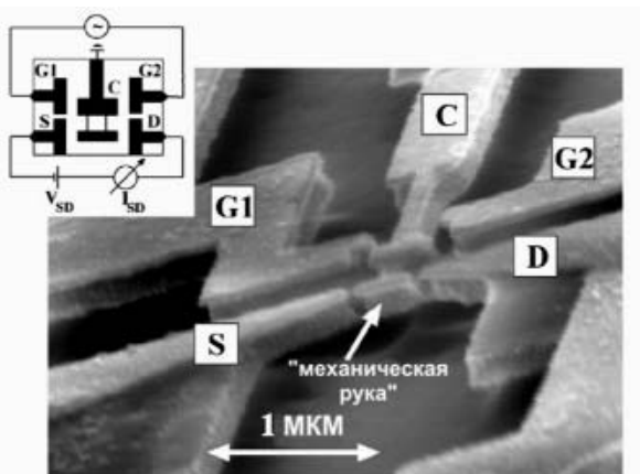
Рис 116. Наномеханический осциллятор Блайка*
