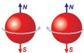
Рис 44. Магнитные полюсы электрона
