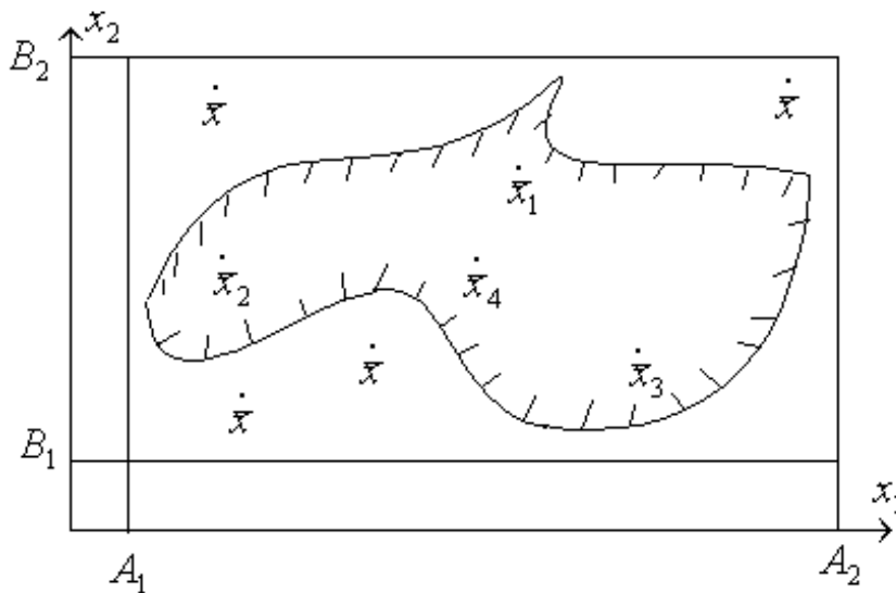
Рис. 24. Построение включающего гиперпараллелепипеда ( A, B – границы параллелепипеда)
