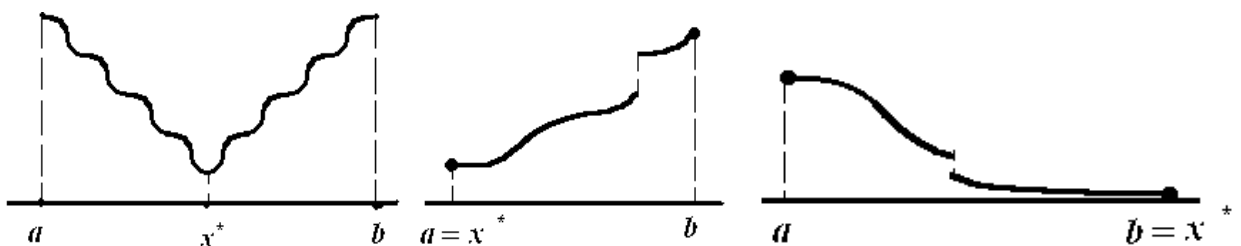
Рис. 5. Унимодальные функции
