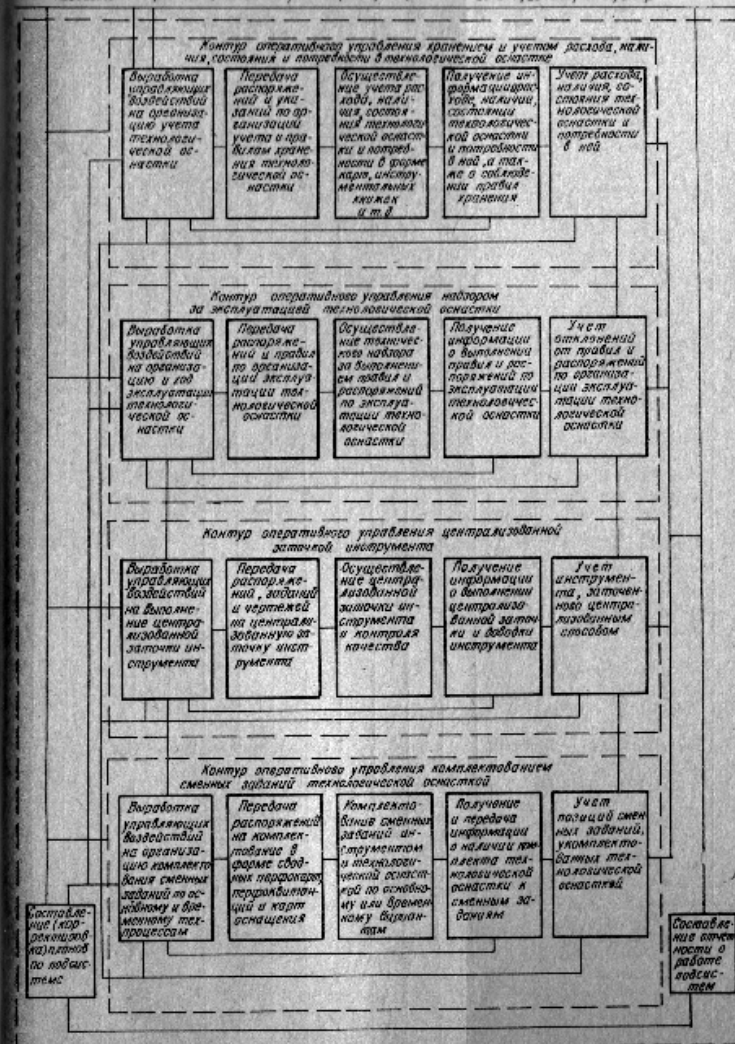
Рис. 10. Структурная схема системы управления организацией, осуществляющей учет, хранение и подготовку технологической оснастки к эксплуатации по оперативным производственным заданиям.
