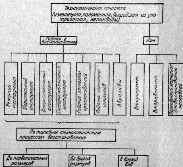
Рис. 9. Схема классификации отработавшей технологической оснастки при ее сортировании на ПСП.
