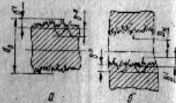
Рис. 7. Схема расположения изношенного и «рыхлого» слоев на поверхности отработавшей детали: а — вал; б — отверстие.
