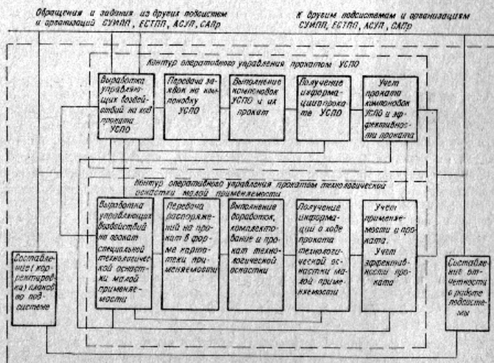
Рис. 3. Структурная схема системы управления организацией, осуществляющей прокат технологической оснастки
