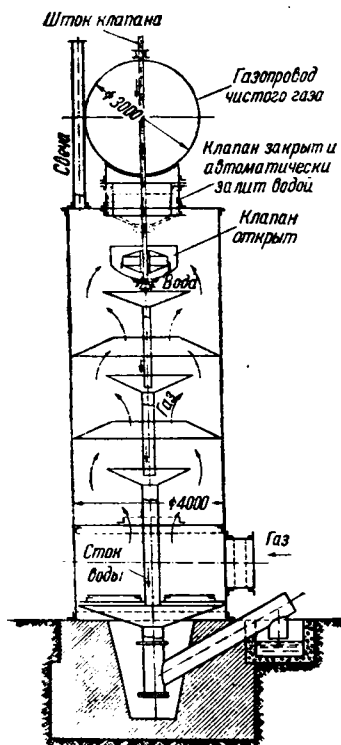
Рис. 37. Водоотделитель Тейзена.
