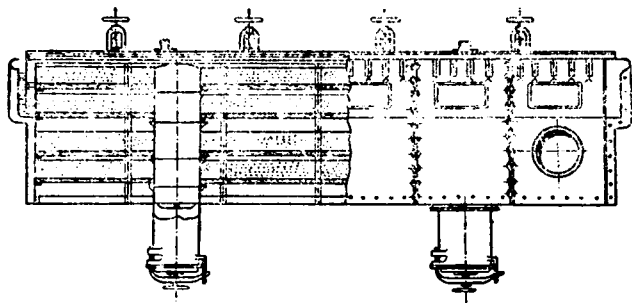
Рис. 93. Разпружные трубы с разборными звеньями в газоочистном ящике.
