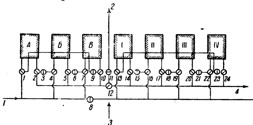
Рис. 87. Схема расположения гидравлики в очистном отделении завода «Мосгаз»:
