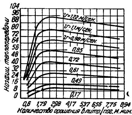
Рис. 15. Влияние количества орошения на коэффициент теплопередачи для разных скоростей газа (при температуре входящего насыщенного газа 69° и выходящего 15°).
