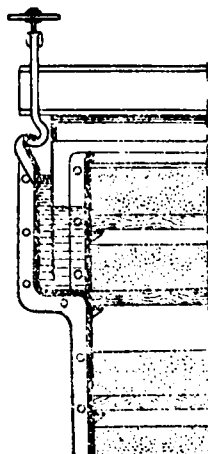
Рис. 83. Мокрый затвор и сопряжение крышки.
