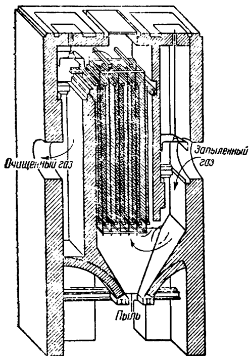
Рис. 69. Схема устройства вертикальной камеры.
