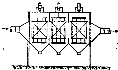
Рис. 71. Горизонтальный электро-фильтр.
