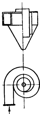
Рис. 28. Схема циклона-улитки.
