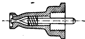
Рис. 12. Форсунка Кершняга.
