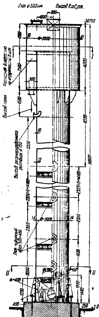
Рис. 109. Регенератор конструкции треста «Газоочистка».
