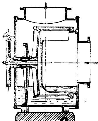
Рис. 48. Смолоотделитель Малле.
