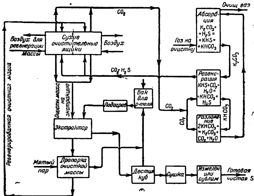
Рис. 118. Последовательность операций при поташно-углекислотном способе Пити.
