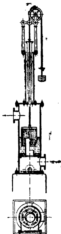
Рис. 46. Раз- рез пелузы.
