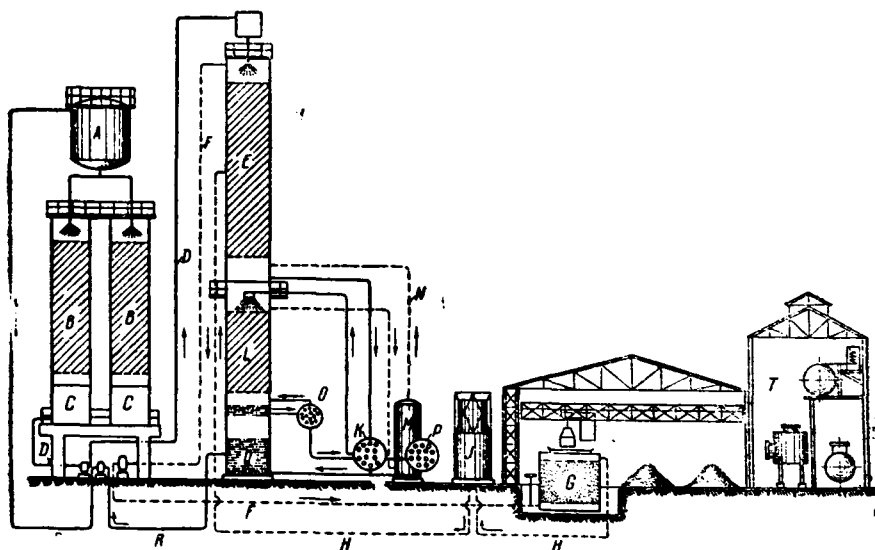
Рис. 119. Схема установки по способу Пити:
