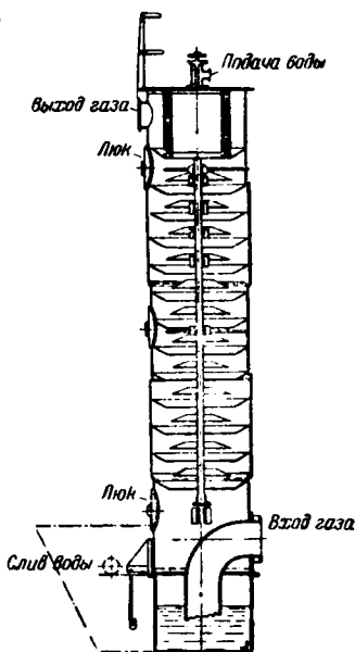
Рис. 13. Холодильник «Лимн».
