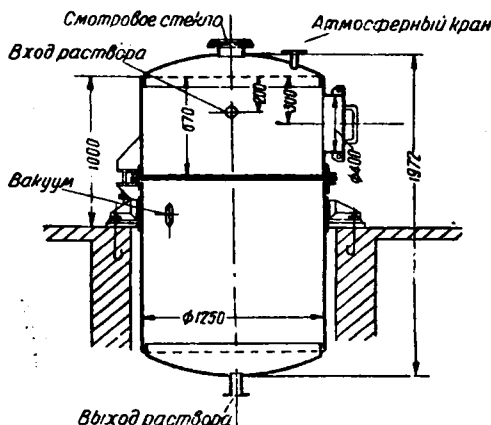
Рис. 117. Контрольный фильтр.
