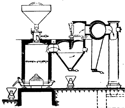
Рис. 25. Пыльная камера с перегородкой при газогенераторе.
