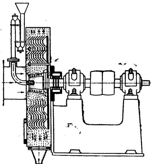
Рис. 38. Тарельчатый дезинтегратор Тейзенз
