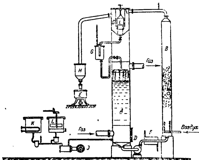
A —абсорбер, B —регенератор, C —флотационное устройство, D —насос, E —центрифуга, F —подогреватель, G —переливной бачок, H —седловатник, J —насос, K —бак для \text{Na}_2\text{CO}_3 , L —бак для \text{Fe}(\text{OH})_3 .
