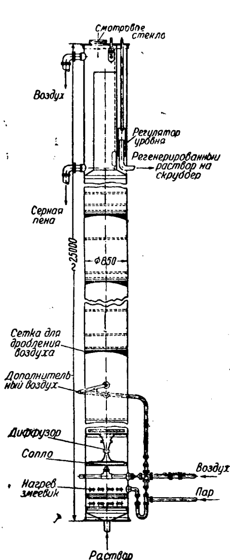
Рис. 108. Регенератор УХИНа.
