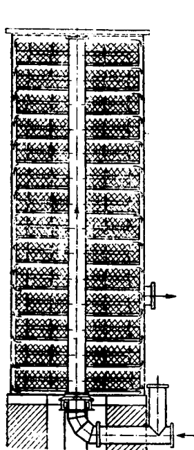
Рис. 95. Схема газоочисточной башни.
