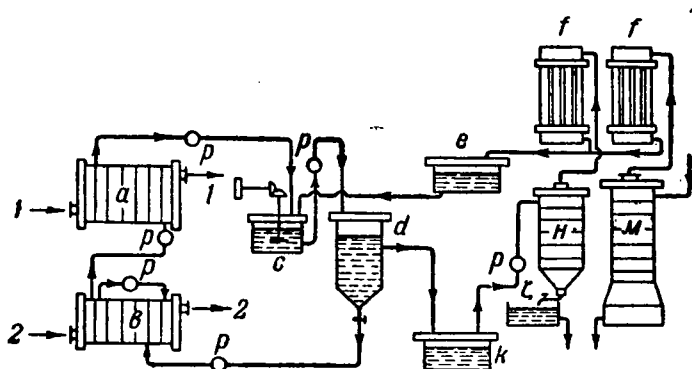
Рис. 122. Сульфитбисульфитный способ Буркгейзера: а—очиститель, б—оживитель, с—пасторизатор серы, d—отстойник для сернистого аммония, e—сборник сернистого аммония, f—холодильник, p—насосы, H—выпариватель, K—сборник полисульфида аммония, M—дистилляционная колонна; 1—ход газа, 2—ход воздуха.
