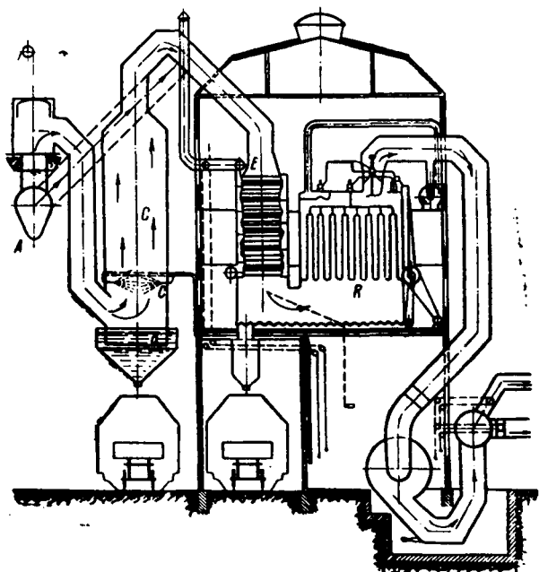
Рис. 41. Сухая газоочистка по системе Гальберг-Бет.
