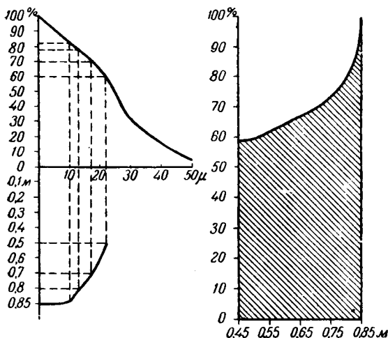
Рис. 33. Графическое определение к. п. д. циклона.
