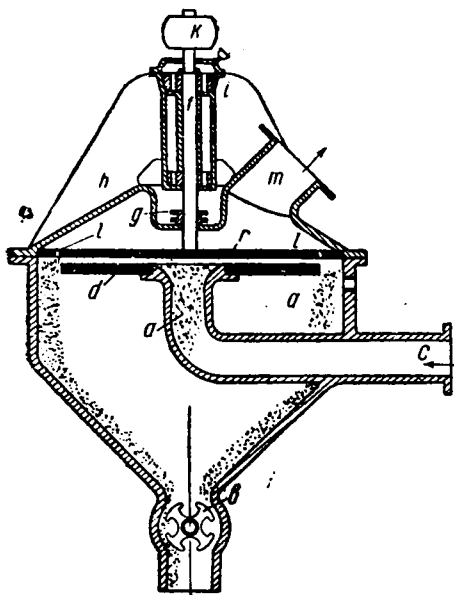
Рис. 55. Центробежный отделитель Барглинга.
