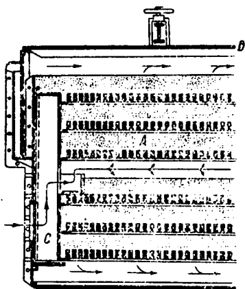
Рис. 86. Газоочистной ящик с двойным потоком газа.
