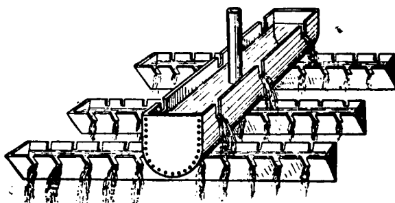
Рис. 10. Коротный распределитель жидкости.
