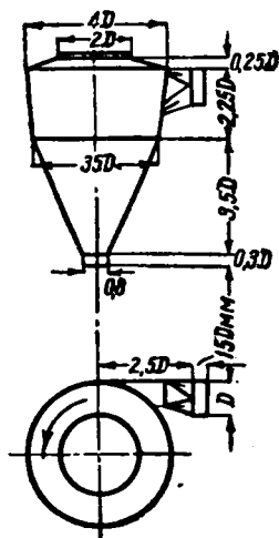
Рис. 32. Относительные размеры циклона фирмы Буфалю (США).
