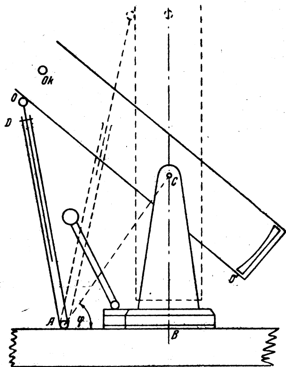
Рис. 9. Схема простого штатива, описанного в тексте.
