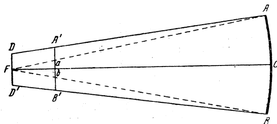
Рис. 4. Определение размеров плоского малого зеркальца для рефлектора системы Ньютона.
