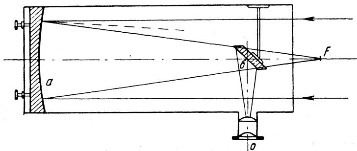
Рис. 1. Схема рефлектора системы Ньютона
