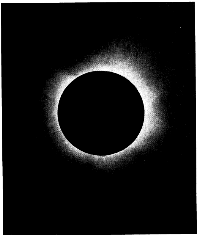
Рис. 8. Фотография солнечной короны (полное солнечное затмение 19 июня 1936 г.), полученная автором с помощью зеркала диаметром в 160 мм, без всякого штатива. В течение полной фазы было сделано 3 фотографии. Поперечник лунного диска на негативах — около 12 мм.
