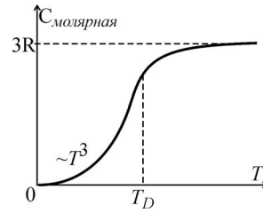
Рис. 8.10. Температурная зависимость молярной теплоемкости трехмерной кристаллической решетки.
