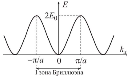
Рис. 9.12. Закон дисперсии электрона.
