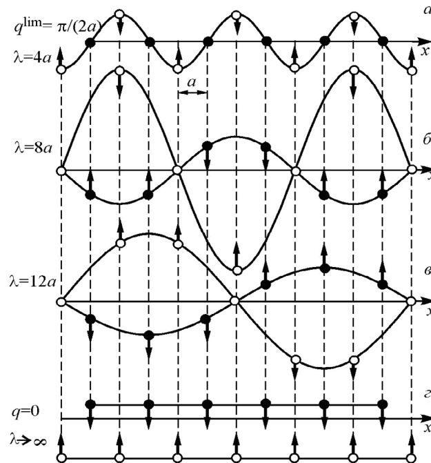
Рис. 8.9. Смещение атомов в линейной цепочке при возбуждениях, соответствующих оптическим фононам с длинами волн: а–в — \lambda = 4a , 8a и 12a соответственно; г — \lambda \rightarrow \infty , колебания атомов одного сорта происходят синфазно, но в противофазе с атомами второго сорта.
