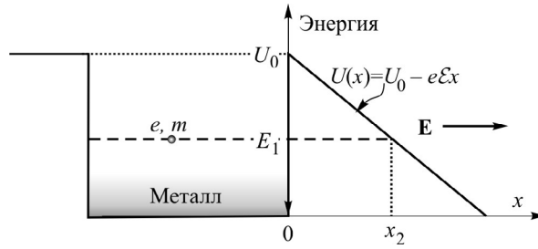
Рис. 5.16. Потенциальный барьер для электрона в металле при наложении внешнего электрического поля с напряженностью \mathbf{E} . m – масса, e – заряд электрона.
