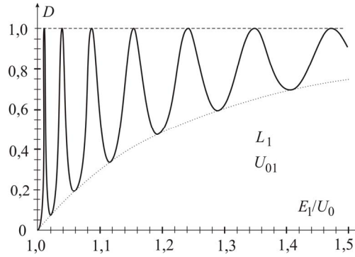
Рис. 5.4. Зависимость коэффициента прохождения D от безразмерного энергетического параметра \chi = E_1 / U_0 , где E_1 — энергия падающей на барьер частицы.
