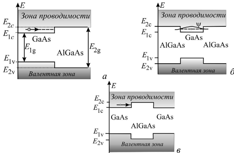
Рис. 11.8. Энергетические схемы гетероструктур — контактов полупроводников арсенида галлия GaAs (ширина запрещенной зоны E_{1g} = 1,5 \text{ эВ} ) и твердого раствора \text{Al}_x\text{Ga}_{1-x}\text{As} , в котором часть x атомов галлия замещена атомами алюминия (ширина запрещенной зоны 1,5 \text{ эВ} \leq E_{2g} \leq 2,2 \text{ эВ} ).
