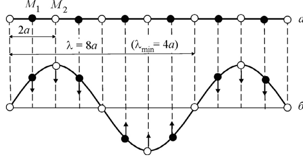
Рис. 8.6. a — одномерная цепочка из атомов двух сортов: масса атомов, отмеченных черными кружками больше массы атомов, отмечены светлыми кружками M_1 > M_2 ; б — акустическая волна в цепочке с длиной волны \lambda = 8a
