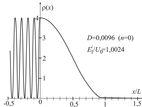
Рис. 5.8. Зависимость плотности вероятности \rho(x) = |\psi(x)|^2 от координаты x частицы в случае минимального прохождения ( D = 0,0096 при E_1' = 1,0024 U_0 ((5.25) при n = 0 ).
