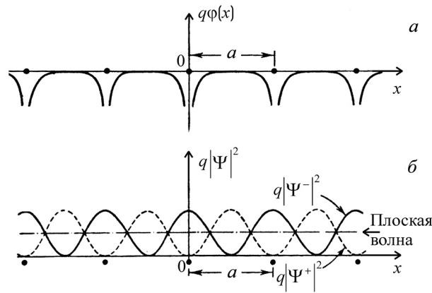
Рис. 9.8. a — потенциальная энергия электрона в одномерной цепочке атомов; б — распределение электронной плотности q|\Psi(x)|^2 для электрона, описываемого плоской волной (9.15) (штрихпунктирная прямая) и стоячими волнами (9.21) и (9.22) (штриховая и сплошная кривые).
