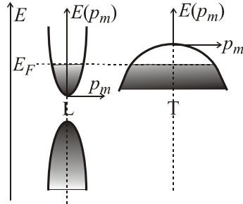
Рис. 10.2. Энергетический спектр полуметалла \text{Bi} , в котором потолок валентной зоны в точках T (их две) зоны Бриллюэна расположен выше дна зоны проводимости в точках L (их всего шесть). Число свободных состояний в экстремуме T равно числу занятых электронами состояний в точках L.
