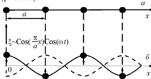
Рис. 8.5. Смещение атомов ( b ) в линейной цепочке ( a ) при возбуждении фононов с волновыми векторами q = \pm \pi/a ( \lambda = 2a ).
