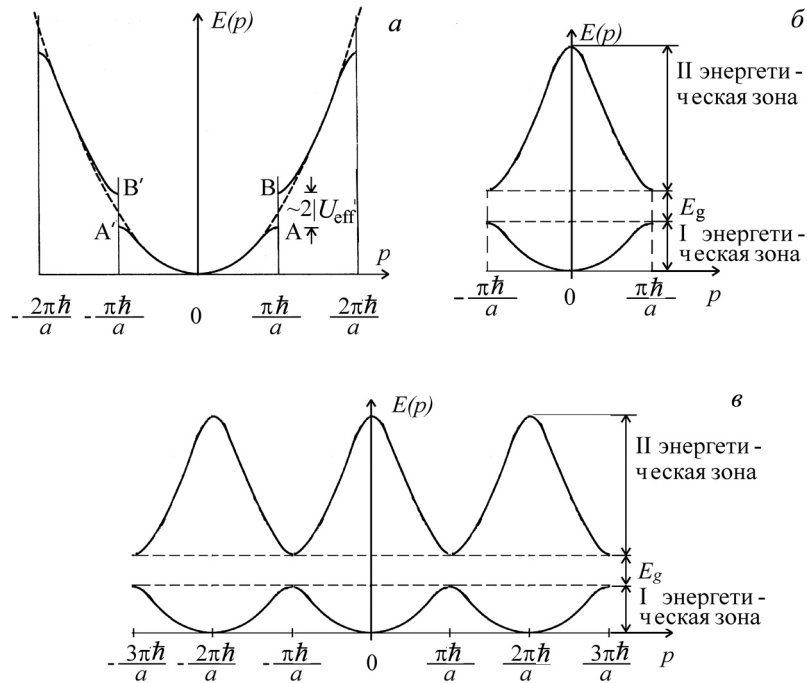
Рис. 9.9. Изменения закона дисперсии электрона при учете величины эффективного потенциала (а). Закон дисперсии в приведенной зоне Бриллюэна (б) и в схеме расширенных зон (в) при учете как величины, так периодичности эффективного потенциала.
