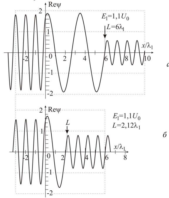
Рис. 4.7. Действительная часть волновой функции частицы, падающей на прямоугольный барьер в случае L = 6\lambda_1 (a) и L = 2,12\lambda_1 (б).
