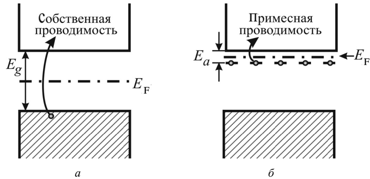
Рис. 10.7. a — зонная структура чистого полупроводника. Уровень Ферми E_F расположен в середине запрещенной зоны E_g . При T \neq 0 К осуществляется собственная проводимость за счет перехода (указан стрелкой) электронов из валентной зоны (заштрихована) в зону проводимости. b — зонная структура полупроводника слабо легированного донорными примесями. Донорные уровни расположены ниже дна зоны проводимости на энергию E_a . Примесная проводимость осуществляется за счет переходов (указаны стрелкой) электронов с донорных уровней в зону проводимости.
