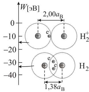
Рис. 3.7. Изменение межатомного расстояния и энергетического состояния электрона в молекуле \text{H}_2 по сравнению с ионом \text{H}_2^+ . Пунктиром обозначены сферы, радиус которых равен боровскому радиусу.
