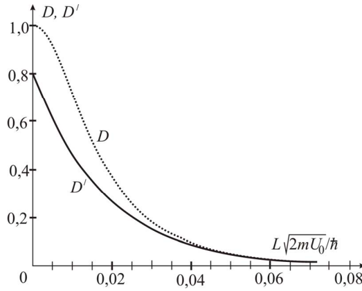
Рис. 5.14. Сравнение зависимостей точного коэффициента прохождения D(L) и асимптотического приближения D'(L) (5.37) от ширины барьера L при значении E_1 / U_0 = 0,05 .
