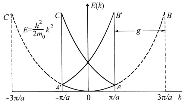
Рис. 9.7. Изменение квадратичного закона дисперсии электрона (штриховая кривая) под влиянием периодического потенциала решетки: эквивалентный сдвиг на векторы обратной решетки всех участков закона дисперсии в область приведенных значений волнового вектора. Результирующий закон дисперсии электрона изображен сплошными линиями.
