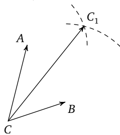
Рис. 12. Построение суммы двух векторов
