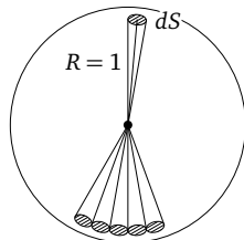
Рис. 23. Объём пирамиды
