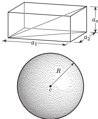
Рис. 19. Параллелепипед и шар
