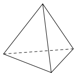
Тетраэдр
