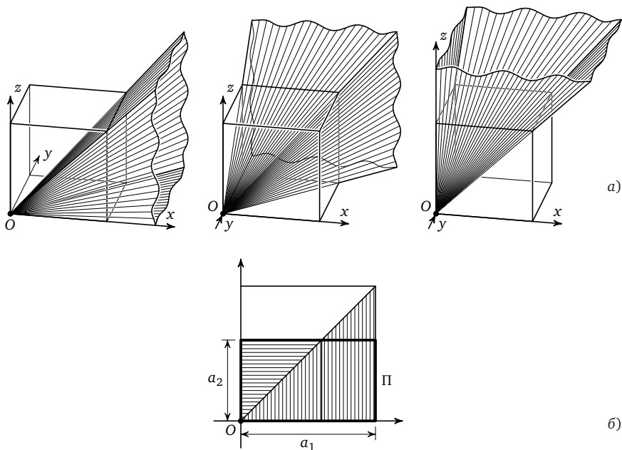
Рис. 29. а) x -, y -, z -пирамиды трёхмерного куба; б) x_1 -, x_2 -, ..., x_n -пирамиды полностью покрывают параллелепипед \Pi
