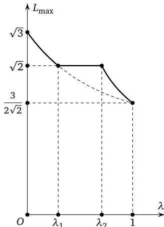
Рис. 26. График функции L_{\max}(\lambda)
