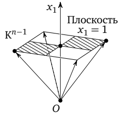
Рис. 30. Вершины, входящие в множество F
