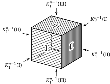
Рис. 14. Различные способы нумерации вершин n -куба
