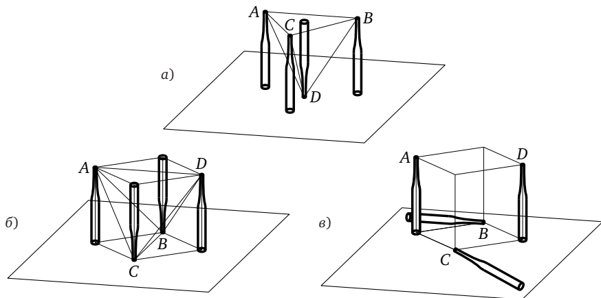
Рис. 47. Расположение бутылок: а) «тетраэдральное»; б), в) «кубическое»
