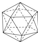
Икосаэдр
