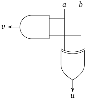
Рис. 8. Реализация полусумматора с помощью элемента XOR
