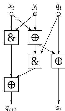
Рис. 13. Модуль вычисления очередного разряда и переноса
