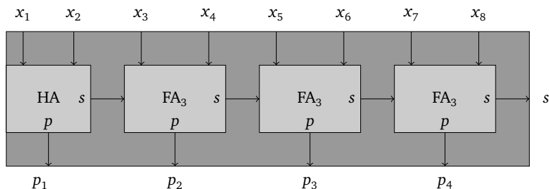
Рис. 10. Модуль FA_8^1 . Входы и выходы схемы связаны соотношением x_1 + \dots + x_8 = 2(p_1 + \dots + p_4) + s
