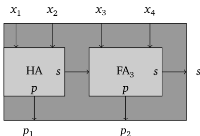
Рис. 9. Модуль FA_4^1 . Входы и выходы схемы связаны соотношением x_1 + x_2 + x_3 + x_4 = 2(p_1 + p_2) + s
