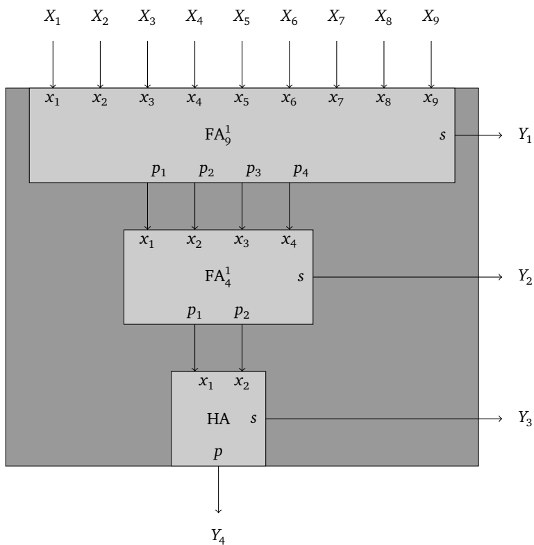
Рис. 12. Модуль FA_9^1 . Входы и выходы схемы связаны соотношением X_1 + \dots + X_9 = 2^3 Y_4 + 2^2 Y_3 + 2 Y_2 + Y_1 , то есть схема является счетчиком числа единиц в наборе (X_1, \dots, X_9)
