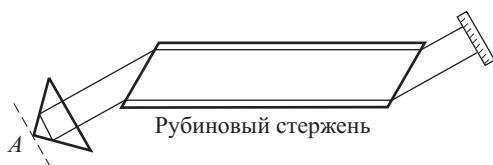
Рис. 40.9. Схема лазера с модулированной добротностью
