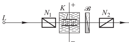
Рис. 27.2. Схема расположения приборов для наблюдения двойного лучепреломления в электрическом поле
