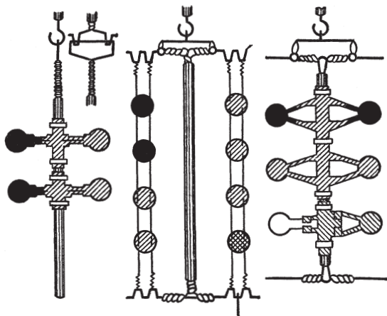
Рис. 34.2. Различные системы крепления крылышек в приборе П.Н. Лебедева
