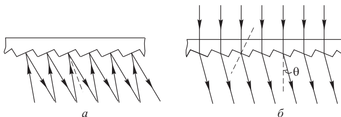
Рис. 9.22. Фазовые решетки со специальным профилем для концентрации энергии в отдельных спектрах различных порядков: a — отражательная решетка; б — пропускающая решетка
