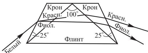
Рис. 13.14. Сложная спектральная призма
