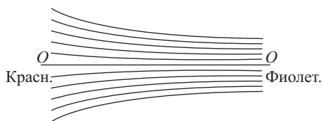
Рис. 28.6. Расположение полос интерференции при скрещении интерферометра Жамена и спектрографа
