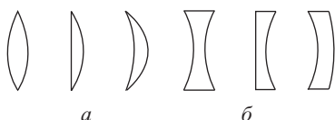
Рис. 12.17. Различные типы тонких линз: а — собирающие, б — рассеивающие
