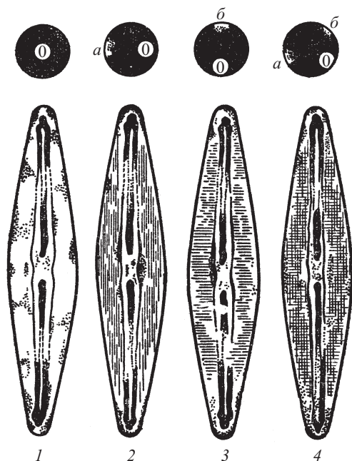
Рис. 15.5. Влияние характера освещения на изображение в микроскопе
