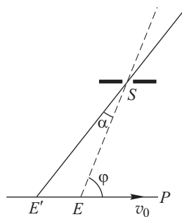
Рис. 20.3. К вычислению абберационного смещения
