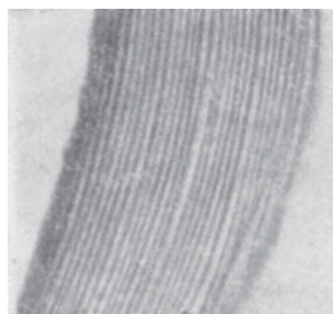
Рис. 5.5. Разрез эмульсии, обработанной по методу Липпмана
