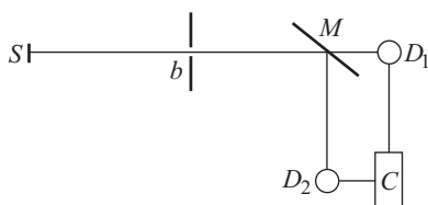
Рис. 4.24. Схема опыта для измерения корреляции интенсивностей
