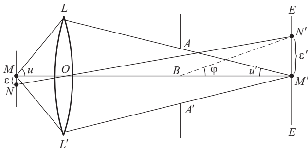
Рис. 15.2. К вычислению разрешающей силы микроскопа: LL' — объектив; AA' — его апертурная диафрагма; на рисунке масштаб искажен: расстояние OM' примерно в 100 раз больше LL' (или AA' )
