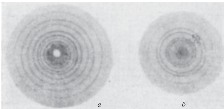
Рис. 15.7. Дифракционные кольца, получаемые при прохождении через металлическую фольгу рентгеновских лучей (а) и электронного пучка (б)
