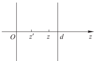
Рис. 41.9. К расчету интерференции вторичных волн при генерации второй гармоники
