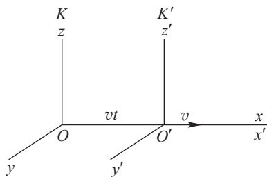
Рис. 22.1. Две инерциальные системы координат
