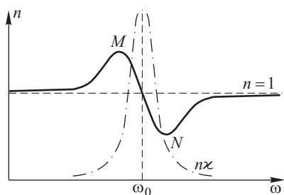
Рис. 28.10. Кривые дисперсии и поглощения вблизи одиночной полосы поглощения
