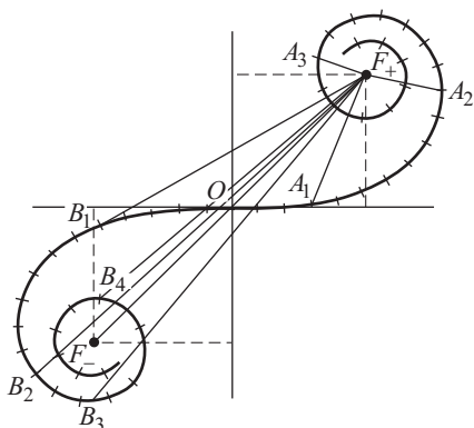
Рис. 8.19. Спираль Корню
