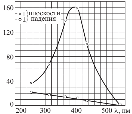
Рис. 32.11. Зависимость фотоэффекта от длины волны для двух различных направлений колебания
