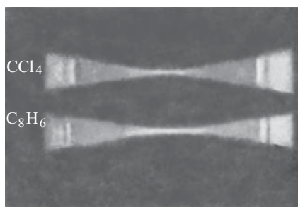
Рис. 29.5. Сравнительная интенсивность молекулярного рассеяния в четыреххлористом углероде ( \text{CCl}_4 ) и бензоле ( \text{C}_6\text{H}_6 )
