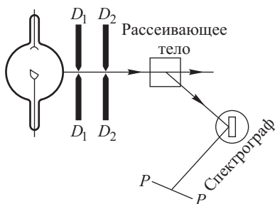
Рис. 33.1. Схема опыта Комптона
