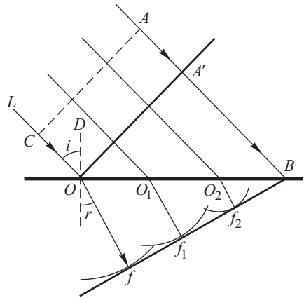
Рис. 1.5. Построение преломленной волны по Гюйгенсу
