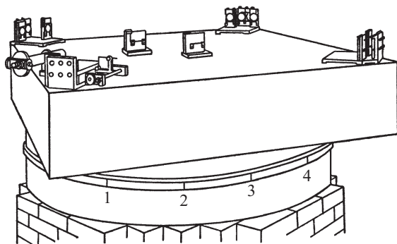
Рис. 22.7. Общий вид установки Майкельсона–Морлей
