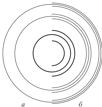
Рис. 40.13. Интерференционные кольца, полученные с эталоном Фабри-Перо при его освещении излучением гелий-неонового лазера ( \lambda = 632,8 нм): а — монохроматический режим, б — трихроматический режим. Эквиливантность линий в шкале частот искажена непостоянством дисперсии эталона
