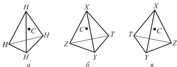
Рис. 30.8. Симметричные и дисимметричные молекулы типа C ( XYZT ): a — симметричная молекула метана; б и в — зеркальные модификации молекулы C ( XYZT )
