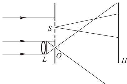
Рис. 11.10. Схема получения голограмм Фурье
