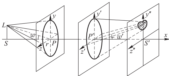
Рис. 13.4. Кома
