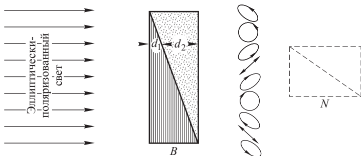
Рис. 18.5. Анализ эллиптически-поляризованного света с помощью компенсатора и поляризатора: В — компенсатор Бабиня; свет, проходящий через разные участки компенсатора, имеет различное состояние поляризации
