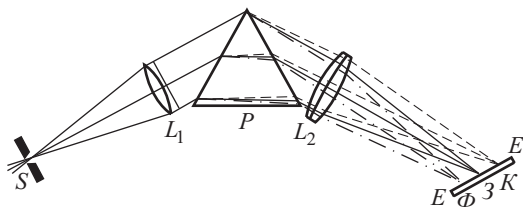
Рис. 14.21. Схематическое изображение хода лучей в спектрографе: S — щель; L_1 — объектив коллиматора; P — призма; L_2 — объектив камеры; EE — фотопластинка
