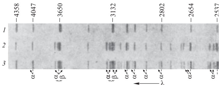
Рис. 29.14. Спектр комбинационного рассеяния кварца: 1 — спектр ртутной лампы; 2 — спектр рассеяния кварца при температуре 20 °C; 3 — спектр рассеяния кварца при температуре 210 °C; \alpha — «красные» спутники, \beta — «фиолетовые» спутники
