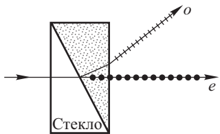
Рис. 17.7. Двокопреломляющая призма из исландского шпата и стекла
