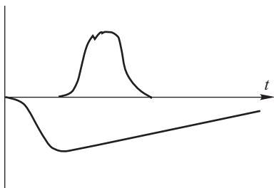
Рис. 40.8. Осциллограммы свечения возбуждающей лампы-вспышки и излучения рубинового лазера
