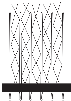
Рис. 36.5. Щетка из полированных иголок вследствие многократных отражений обладает большой поглощательной и испускающей способностью
