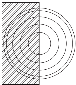
Рис. 8.15. Пересечение зон Френеля экраном с прямолинейным краем
