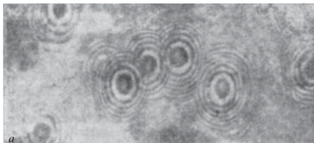
Рис. 11.6. Фотография объектов исследования
