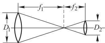
Рис. 14.15. Ход лучей в телескопической системе: увеличение перевернутым (астрономические трубы), \mathcal{N} = \varphi'/\varphi = f_1/f_2 = D_1/D_2
