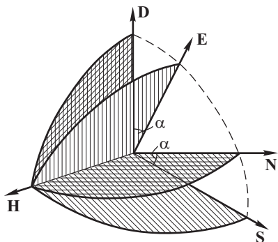
Рис. 26.4. Взаимное расположение векторов \mathbf{E} , \mathbf{D} , \mathbf{H} , \mathbf{S} и \mathbf{N} . Вектор \mathbf{H} нормален к плоскости, в которой лежат остальные векторы
