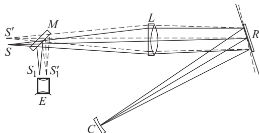
Рис. 20.6. Определение скорости света методом вращающегося зеркала
