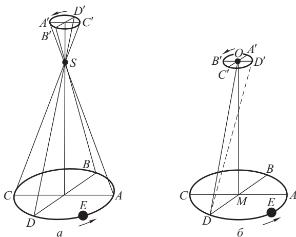
Рис. 20.2. Кажущееся смещение звезд, обусловленное годичным движением Земли: a — вследствие годичного параллакса; б — вследствие абберации света. Кажущиеся положения звезды A' , B' , C' , D' сопоставлены соответствующим точкам траектории Земли E
