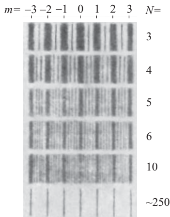
Рис. 9.17. Изменение характера дифракционного спектра в зависимости от числа щелей N (напротив)
