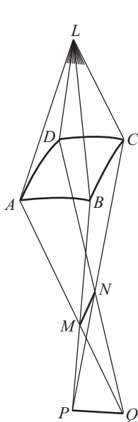
Рис. 12.6. Астигматическое изображение точки L . При прохождении через оптическую систему гомотцентричность пучка нарушается
