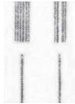
Рис. 31.5. Сложный эффект Зеемана для дублета натрия. Внизу — дублет в отсутствие поля, вверху — расщепление в магнитном поле Рис. 31.6. Сложный эффект Зеемана для септета хрома. Внизу — четырнадцать \sigma -компонент, вверху — семь \pi -компонент
