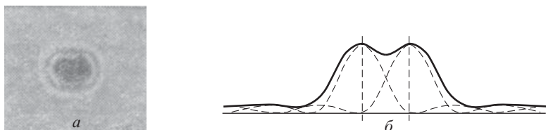
Рис. 15.1. Общий вид дифракционной картины при наблюдении двух удаленных звезд, находящихся на небольшом угловом расстоянии (а); предел разрешения при изображении двух точек (критерий Рэлея) (б)
