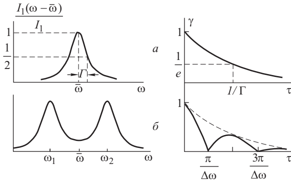
Рис. 4.19. Спектральные плотности и степени когерентности для случаев, описываемых соотношениями (22.13), (22.14) (а) и (22.15), (22.16) (б)
