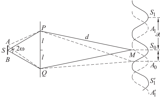
Рис. 4.11. К выводу условия 2b \sin \omega = \lambda/4
