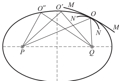
Рис. 12.4. К принципу Ферма: действительный путь света соответствует стационарному времени распространения
