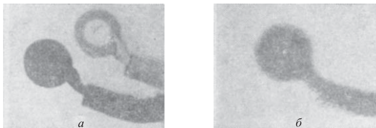
Рис. 8.18. Моделирование картины дифракции на экране: а — тень от руки, держащей тарелку, отбрасывается на близко расположенный экран; тень и объект геометрически подобны; б — тень от руки, держащей тарелку, отбрасывается на экран, расположенный на большом расстоянии (11 км); тень искажена дифракцией. (Фотография Аркадьева, выполненная на модели, рассчитанной по принципу подобия.)
