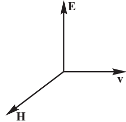
Рис. 2.1. Взаимное расположение векторов \mathbf{E} , \mathbf{H} и вектора скорости \mathbf{v} в электромагнитной среде
