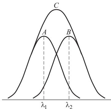
Рис. 9.27. Распределение освещенности при наложении двух близких спектральных линий одинаковой интенсивности
