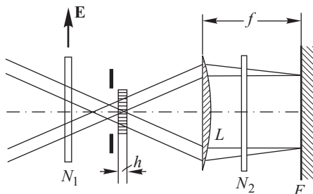
Рис. 26.20. Схема расположения для наблюдения цветов кристаллической пластинки в сходящихся лучах
