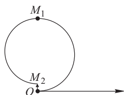
Рис. 8.9. Векторная диаграмма действия первой и второй зон: OM_2 — результирующий вектор
