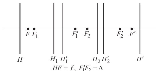
Рис. 12.28. К определению параметров сложной оптической системы
