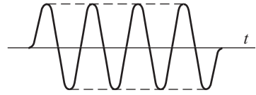
Рис. 2.2. Пример немонхроматической волны: «обрывок» синусоиды, или волновой пуг
