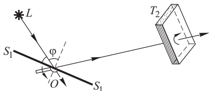
Рис. 16.2. Исследование поляризации при отражении: S_1S_1 — стеклянное зеркало, поляризующее лучи света, T_2 — пластинка турмалина, служащая анализатором
