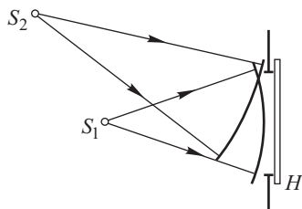
Рис. 11.1. К вопросу о регистрации фазы волны
