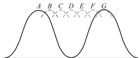
Рис. 4.16. Распределение максимумов интерференции немонохроматических лучей: сплошная кривая — распределение освещенности для длины волны \lambda , причем A — максимум m -го порядка, G — максимум (m + 1) -го порядка, B, C, D \dots — максимумы m -го порядка для длин волн в интервале \lambda < \lambda_i \leq \lambda + \Delta\lambda
