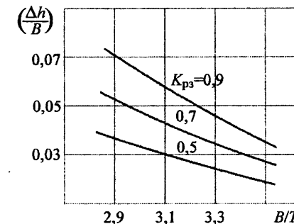
Рис. 37. Графическая интерпретация зависимости (59)
