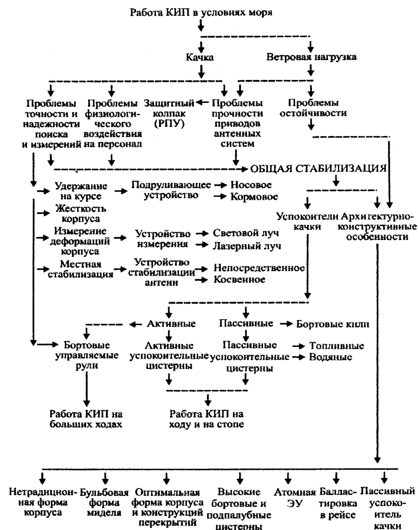
Рис. 36. Упрощенная схема проблем и конструктивных решений обеспечения работы КИП в условиях моря
