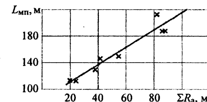
Рис. 47. Зависимость L_{\text{мп}} от \Sigma R_a
