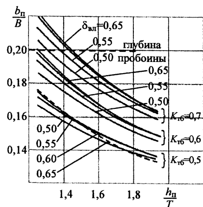
Рис. 18. Графическая интерпретация зависимости b_n/B
