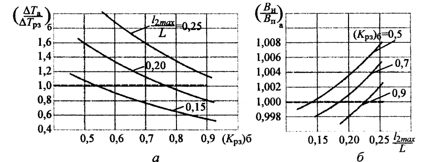
Рис. 20. Зависимости: а – (\Delta T_a/\Delta T_{рз})_6 от (K_{рз})_6 и l_{2 max}/L ; б – (B_n/B_n)_a от l_{2 max}/L и (K_{рз})_6
