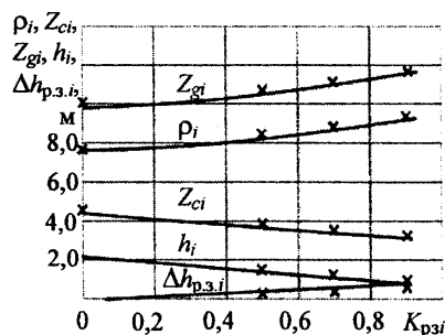
Рис. 33. Результаты расчета элементов остойчивости при различных K_{рзi}
