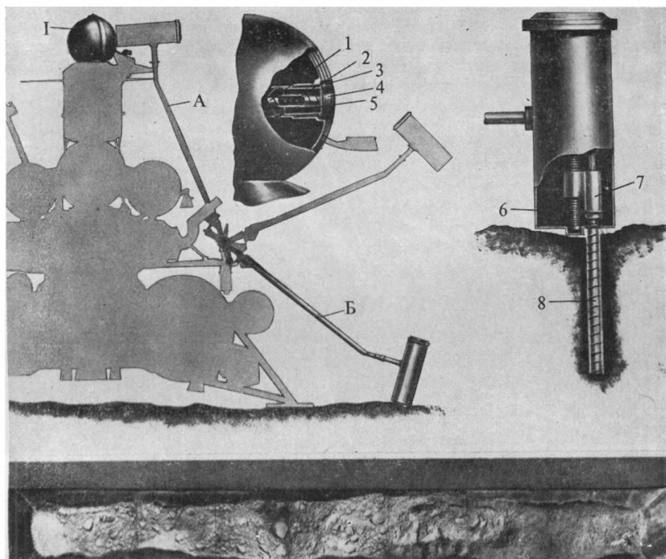
Рис. 23. Работа грунтозаборного устройства станции «Луна-16» на поверхности Луны
