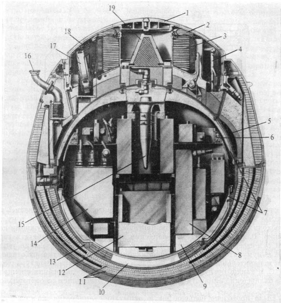
Рис. 31. Спускаемый аппарат автоматической станции «Венера-8» (разрез)
