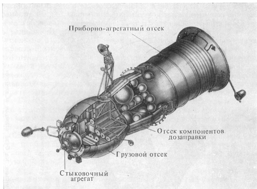
Рис. 57. Грузовой корабль «Прогресс»
