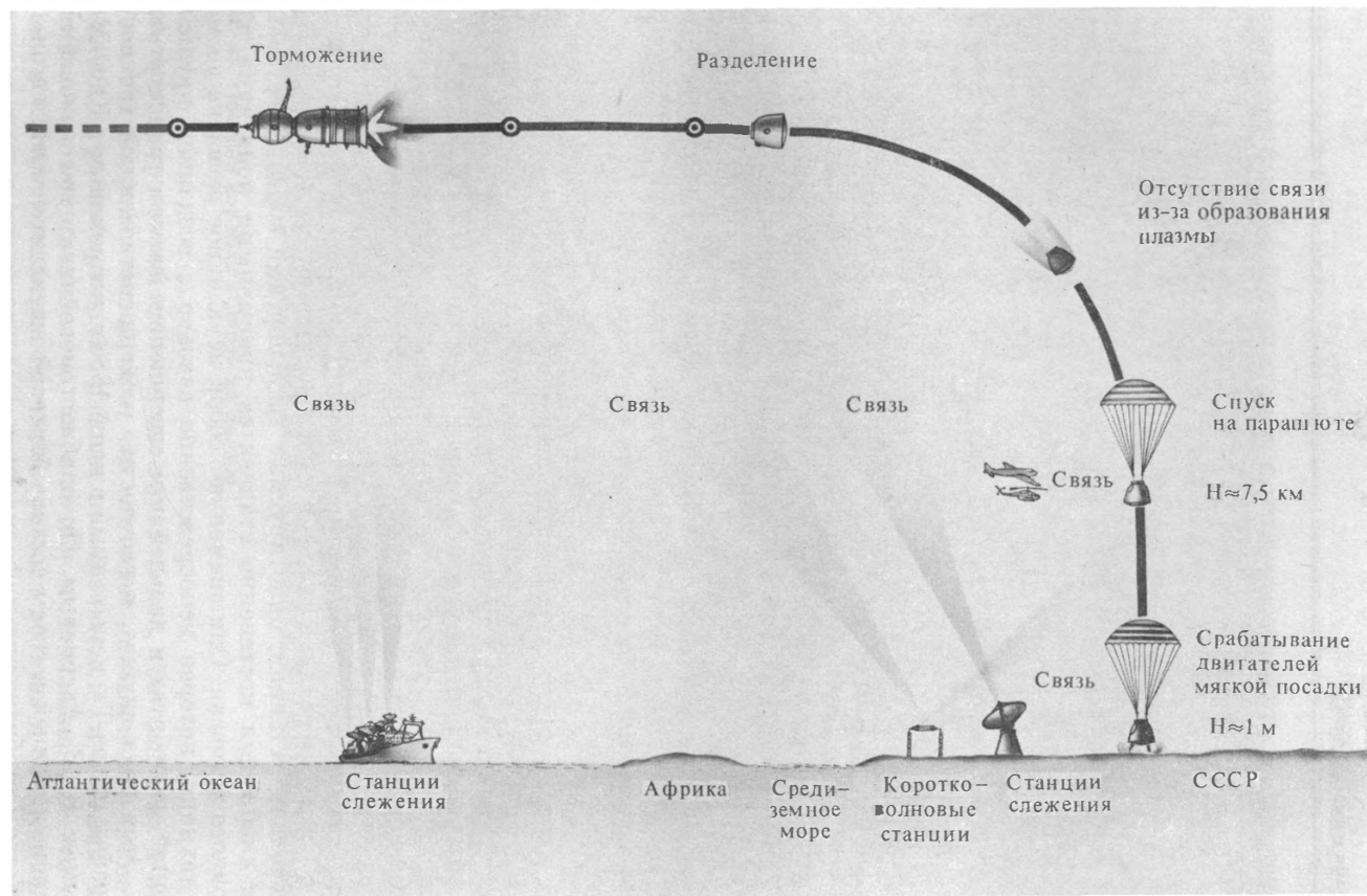
Рис. 59. Схема спусков космонавтов на Землю в транспортном корабле «Союз» и функционирование наземных средств обеспечения посадки и поиска
