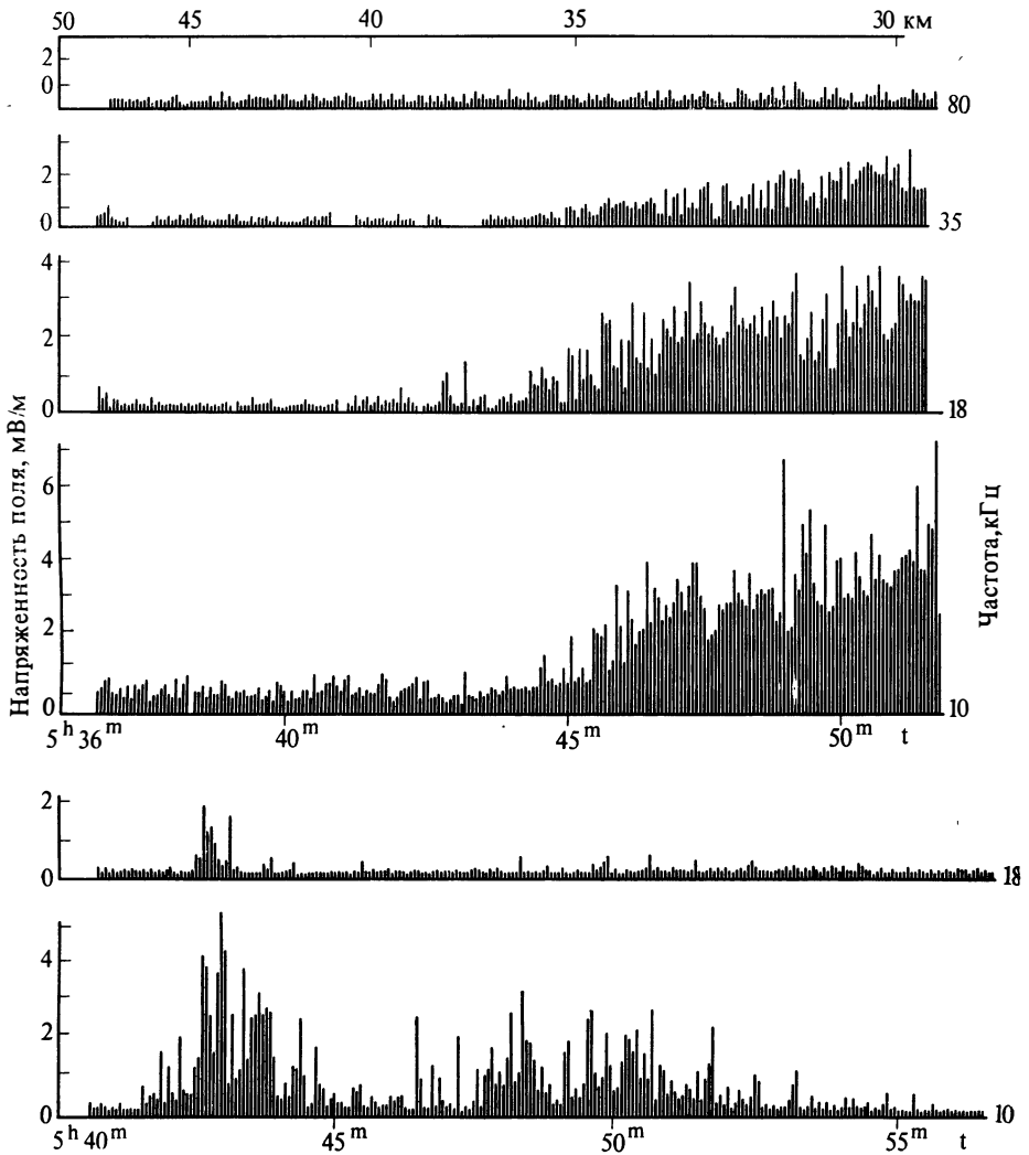
Рис. 40. Напряженности электромагнитных полей, регистрировавшиеся в процессе спуска аппаратов станций «Венера-11 и 12», свидетельствующие о грозовой активности в атмосфере Венеры
