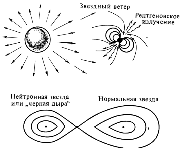
Рис. 47. Механизм генерации рентгеновского излучения в тесной двойной системе (модель)
