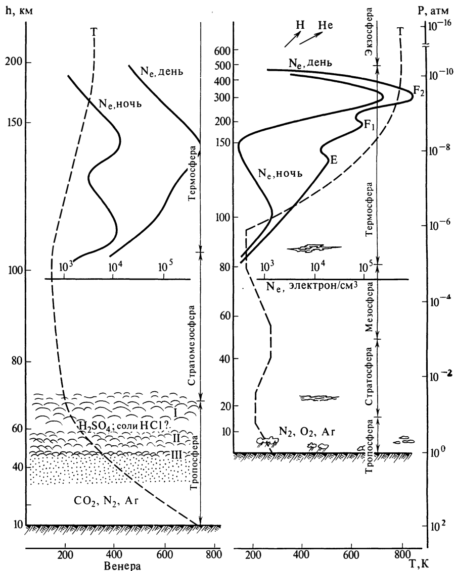
Рис. 29. Модель атмосферы Венеры (слева) и Земли (справа)
