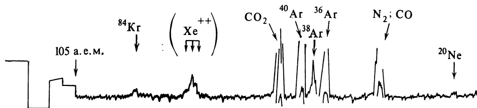
Рис. 39. Масс-спектр газового состава атмосферы Венеры по данным измерений на станции «Венера-11»
