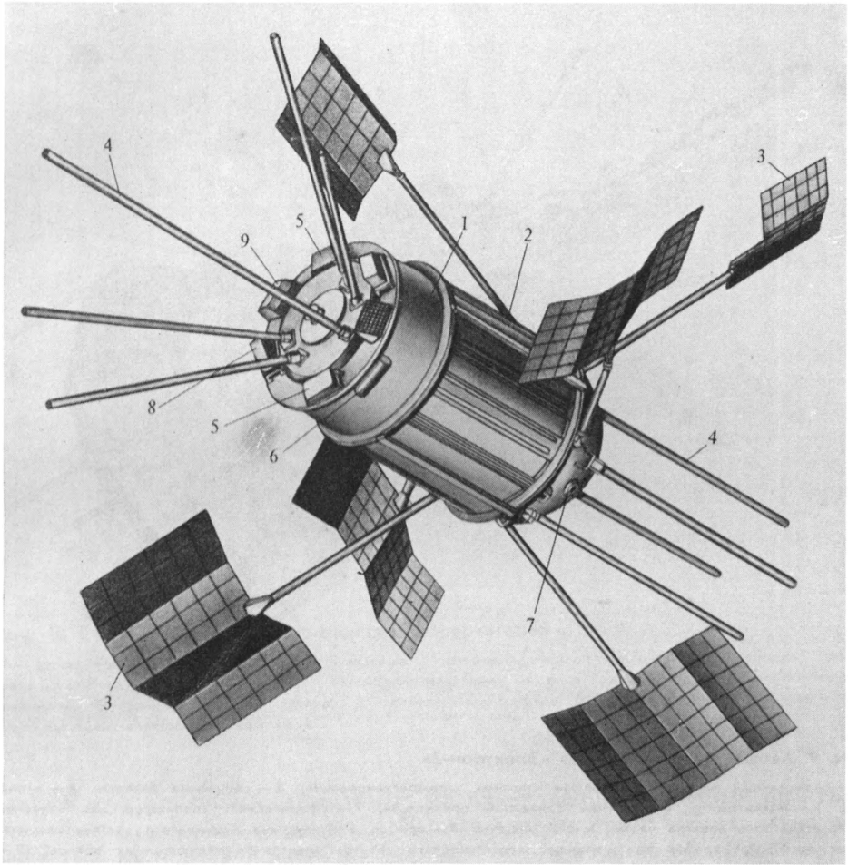
Рис. 8. Автоматическая станция «Электрон-1»
