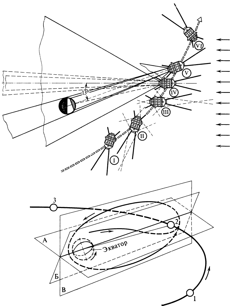
Рис. 18. Схема облета Луны автоматической станцией «Луна-3» и фотографирования обратной стороны Луны
