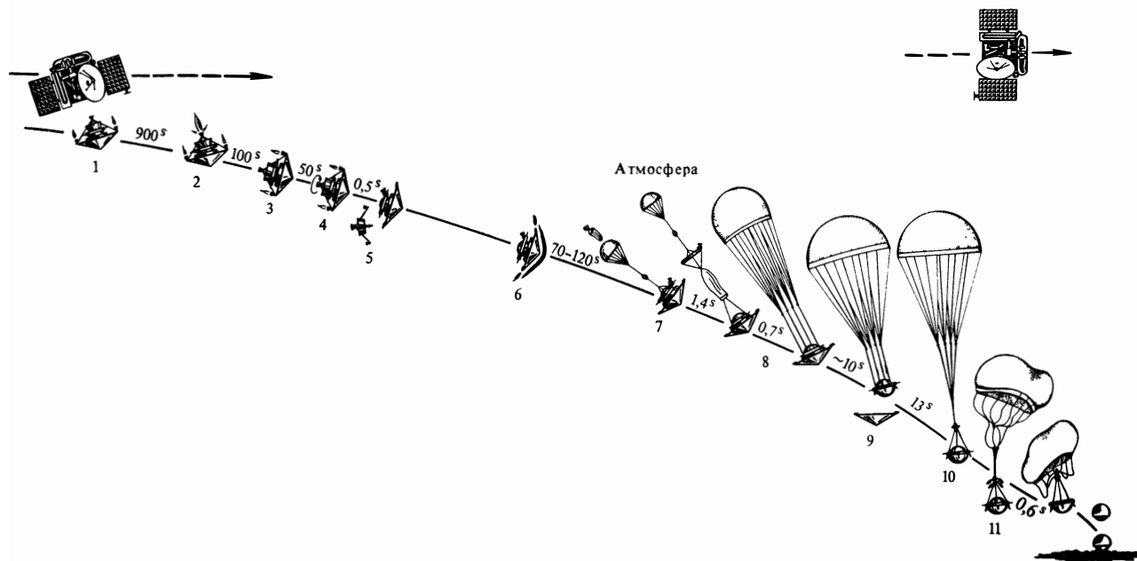
Рис. 43. Схема посадки спускаемого аппарата станции «Марс-6» на планету
