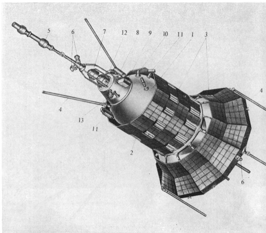
Рис. 9. Автоматическая станция «Электрон-2»
