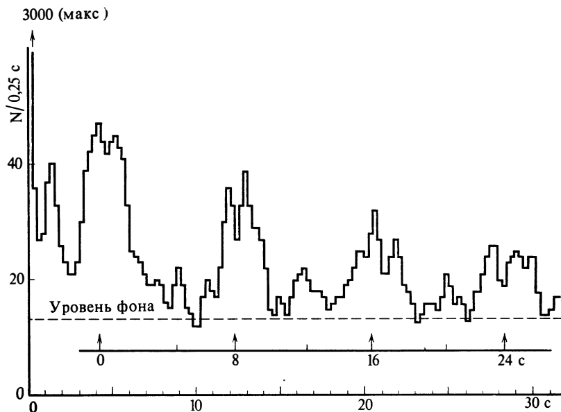
Рис. 48. Мощный всплеск и последующее пульсирующее затухание рентгеновского излучения, зарегистрированного станцией «Венера-12» 5.III 1979 г.
