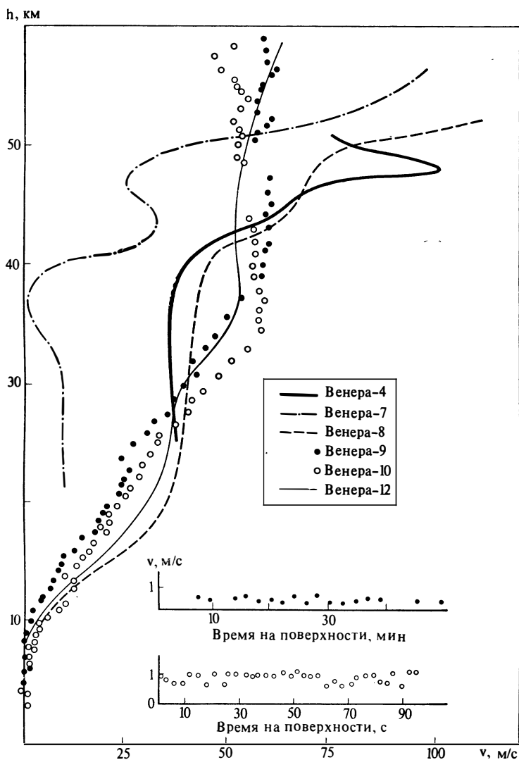
Рис. 38. Изменение скорости ветра с высотой в атмосфере Венеры по данным радиоизмерений на спускаемых аппаратах автоматических станций «Венера»
