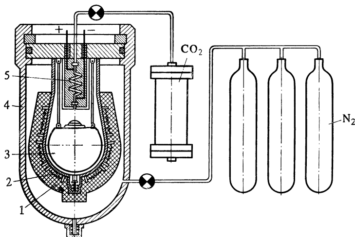
Рис. 32. Установка для тепловых испытаний и имитации спуска в атмосфере Венеры 1 — теплоизолятор, 2 — электронагреватель, 3 — спускаемый аппарат, 4 — корпус камеры, 5 — подача газа с подогревом
