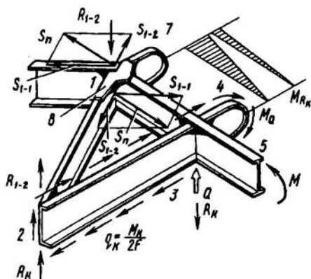
Рис. 3.5. Конструктивная схема корневой треугольной рамы и нагружение ее элементов
