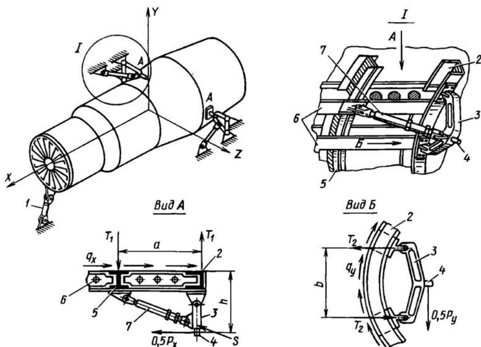
Рис. 9.4. Конструкция узлов крепления двигателя в фюзеляже, схемы их нагружения и уравнивания на силовых элементах фюзеляжа
