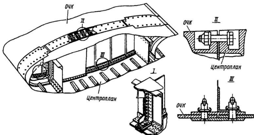
Рис. 2.63. Конструкция стыкового соединения центроплана с ОЧК
