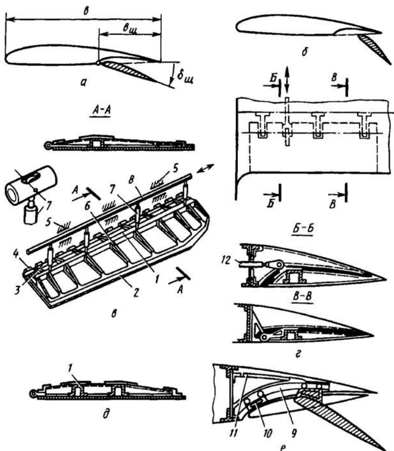
Рис. 4.3. Конструкция щитков
