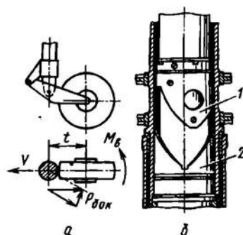
Рис. 7.35. Вынос колес передней стойки. Кулачковый механизм для установки колес передней опоры по полету после отрыва от ВПП
