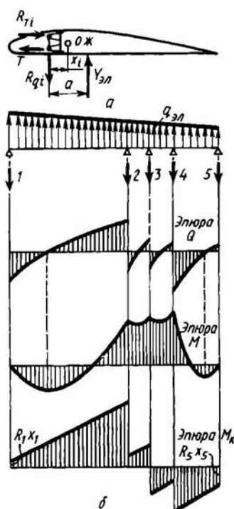
Рис. 4.15. Нагрузки на элерон и эпюры Q , M и M_k
