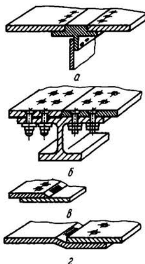
Рис. 2.30. Типовые соединения обшивки
