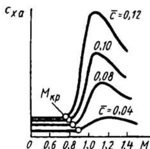
Рис. 2.7. Зависимость c_{xa} = f(M, \bar{c})
