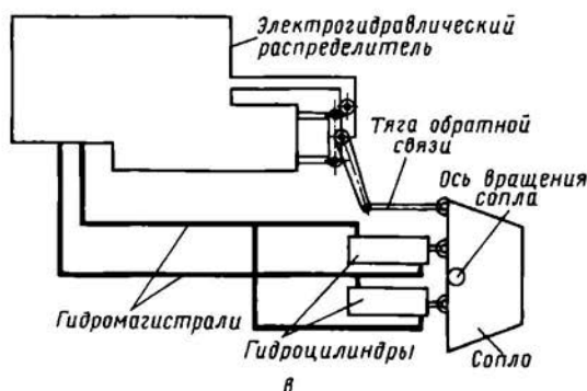
Рис. 8.27. Электродистанционная система управления
