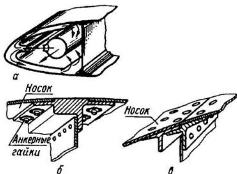
Рис. 2.68. Носок крыла и конструкция стыковых соединений носка с лонжероном крыла
