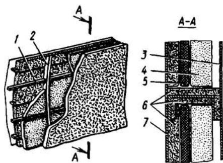
Рис. 6.34. Конструктивная схема тепло- и звукоизоляции кабины
