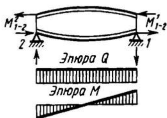
Рис. 3.8. Схема нагружения бортовой нервюры 1—2 двухлонжеронного крыла
