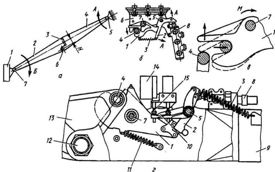
Рис. 7.15. Замки фиксации стоек в выпущенном и убранном положениях (подкос со стрелой прогиба, замок типа крюк-защелка)
