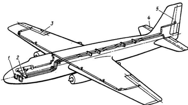
Рис. 8.1. Элементы системы неавтоматического управления самолетом
