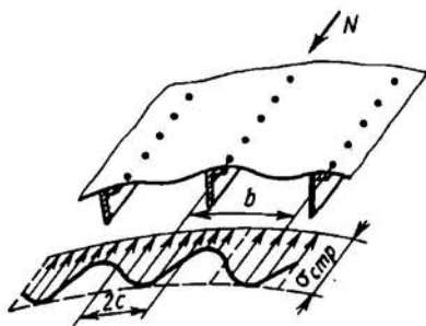
Рис. 2.32. Работа панели на осевые сжимающие силы. Распределение напряжений в элементах панели
