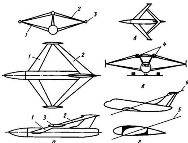
Рис. 3.35. Схемы сочлененных крыльев
