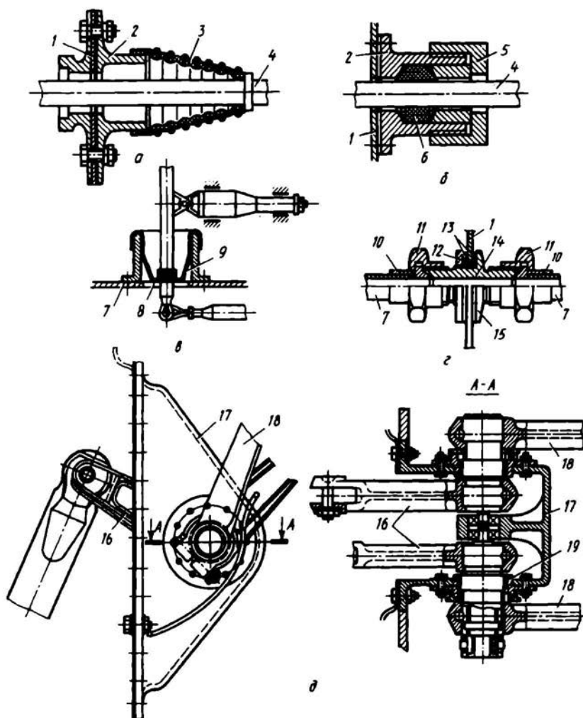
Рис. 6.25. Варианты гермовыводов элементов проводки управления
