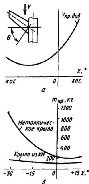
Рис. 3.17. Сравнительная оценка по затратам массы и по критической скорости дивергенции крыльев прямой и обратной стреловидности
