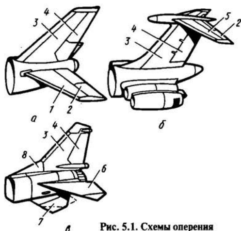
Рис. 5.1. Схемы оперения
