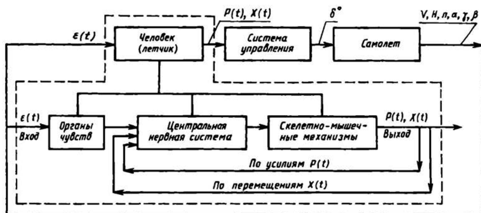
Рис. 8.2. Контур управления «человек—система управления—самолет»
