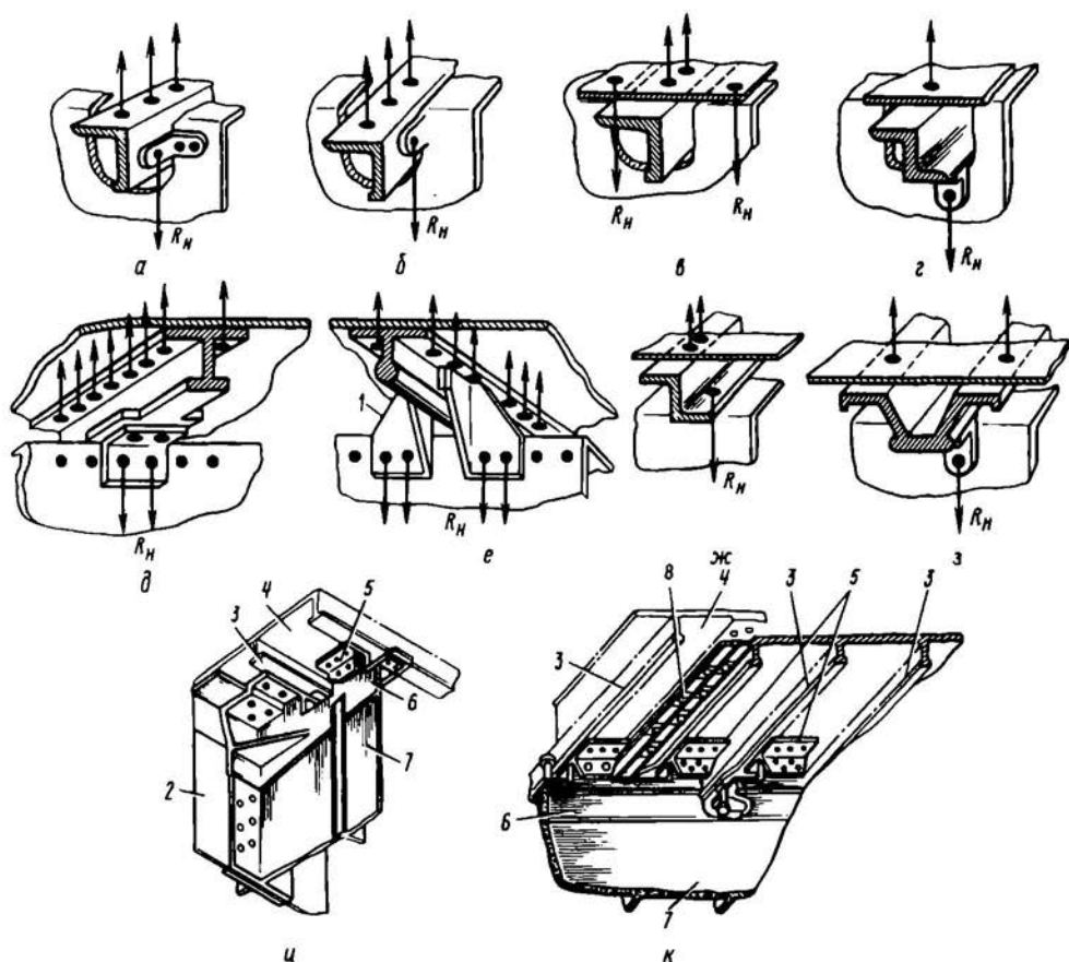
Рис. 2.26. Варианты соединений обшивки, нервюр и стрингеров между собой
