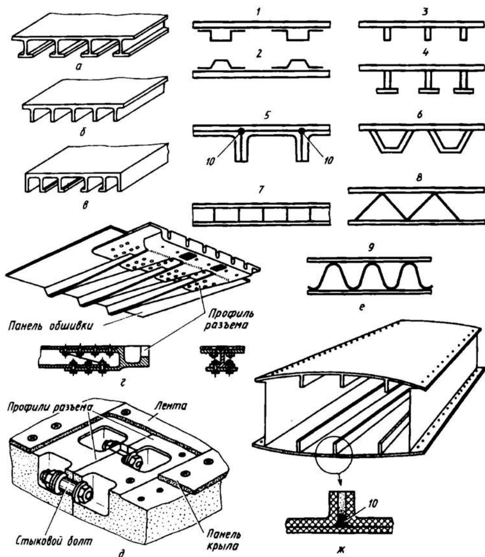
Рис. 2.37. Типовые сечения монолитных панелей ( а, б, в ). Монолитная панель с профилем разреза ( г, д ). Панели из КМ ( е, ж )
