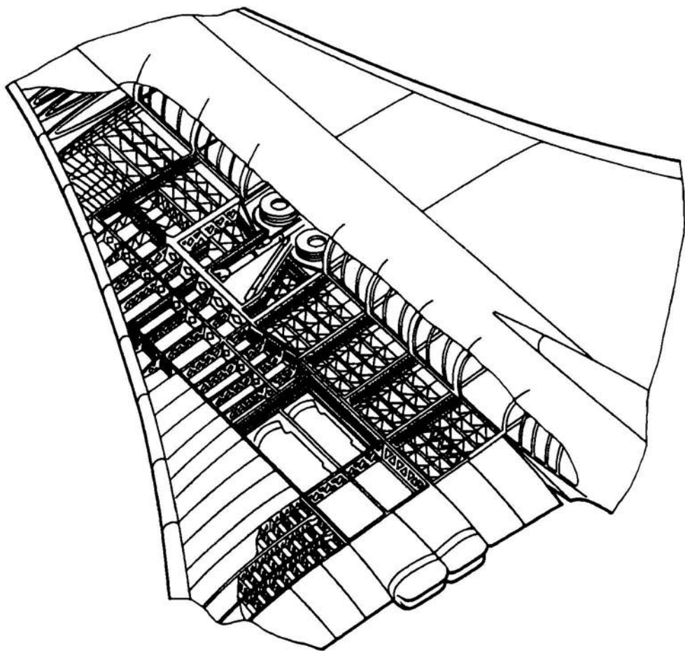
Рис. 3.32. Конструкция треугольного крыла с параллельными лонжеронами
