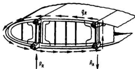
Рис. 2.51. Конструкция и нагружение корневой нервюры
