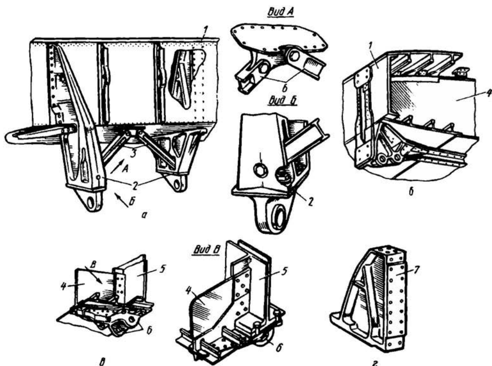
Рис. 7.14. Конструкция узлов крепления стойки шасси и двигателя
