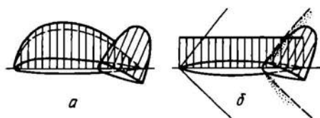
Рис. 5.2. Картина обтекания ГО: а — M < 1 ; б — M > 1
