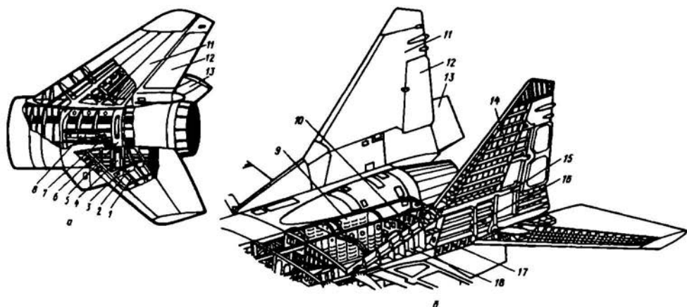
Рис. 5.19. Конструкции одно- и двухкилевого оперения с ЦПГО
