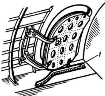
Рис. 6.28. Варианты дверей, открывающихся внутрь фюзеляжа
