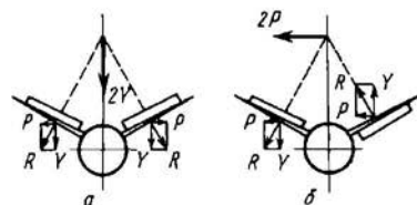
Рис. 5.21. V-образное оперение. Схема сил на оперении при симметричном и антисимметричном отклонении рулей
