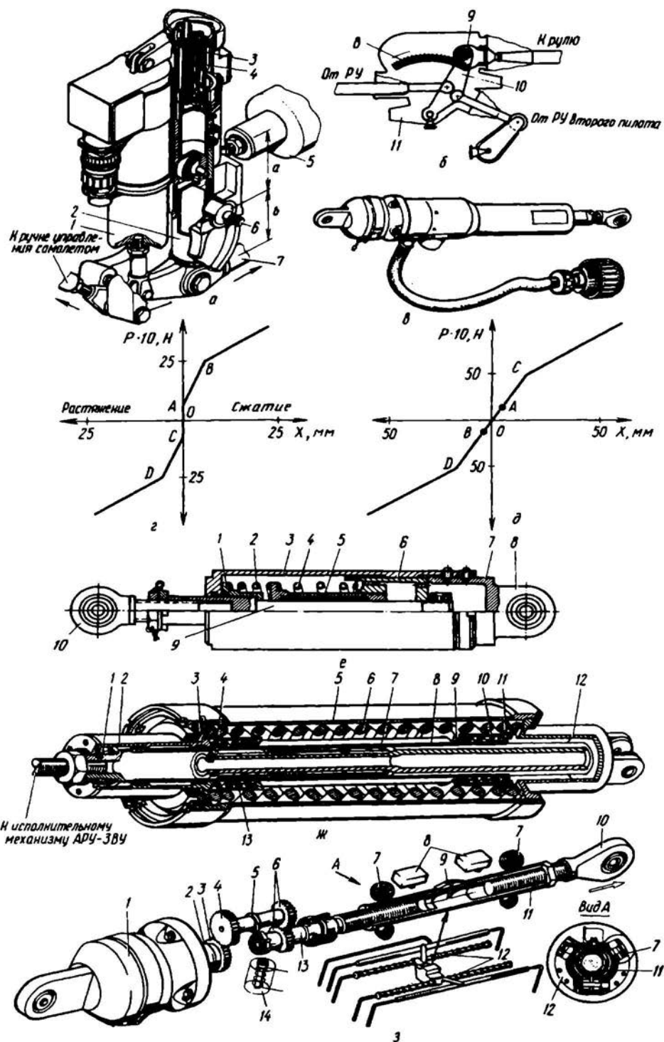
Рис. 8.21. Конструкция элементов автоматики систем управления современных самолетов
