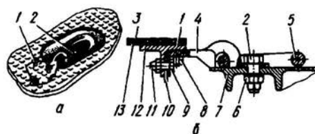
Рис. 6.37. Конструкция швартовочных приспособлений
