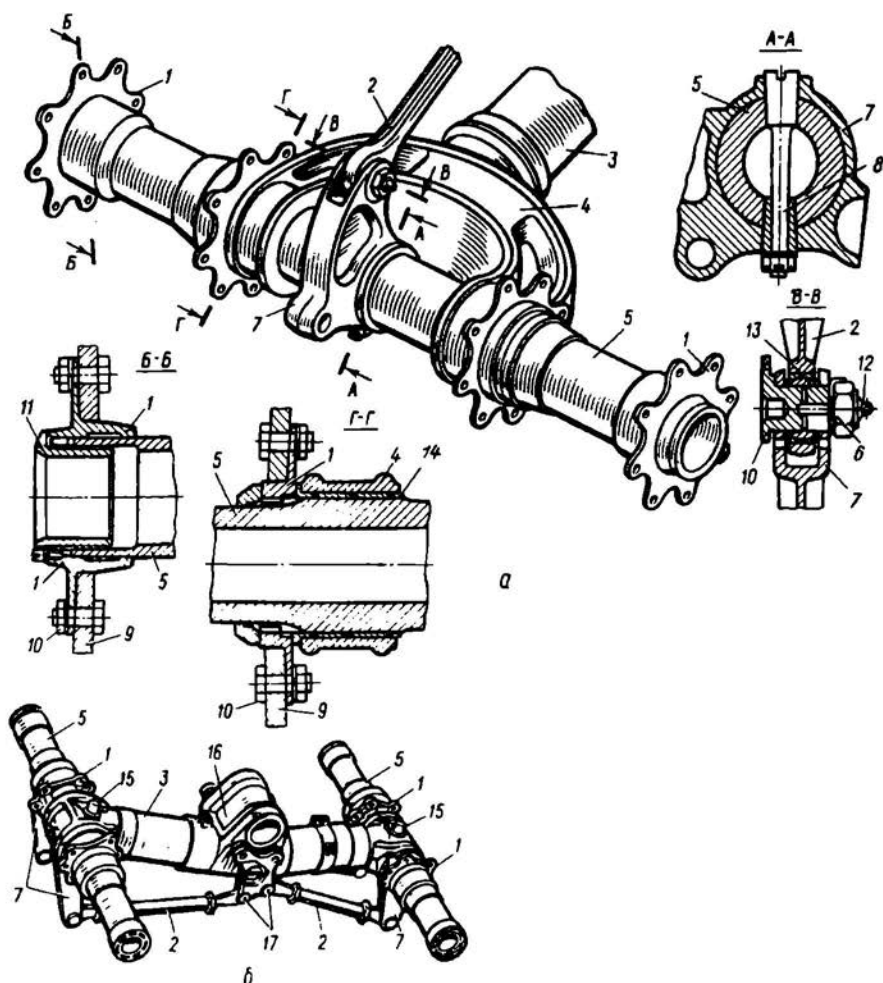
Рис. 7.23. Элементы конструкции тележек
