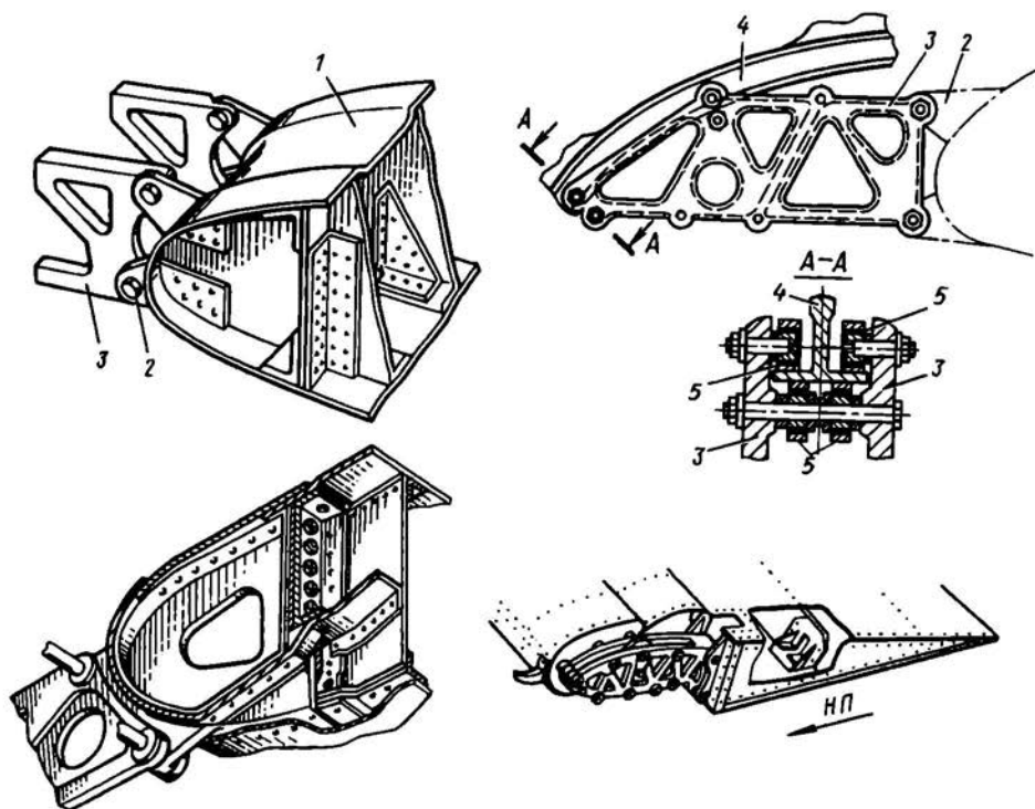
Рис. 4.6. Конструкция каретки и узлов ее крепления
