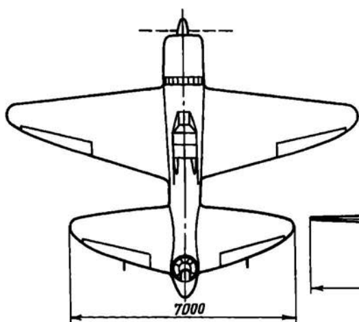
Рис. 3.37. Самолет «Ш-Тандем»
