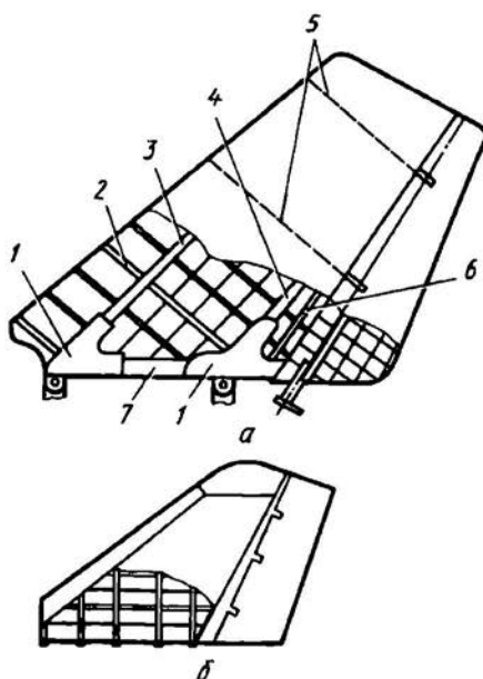
Рис. 5.14. КСС стреловидного ВО
