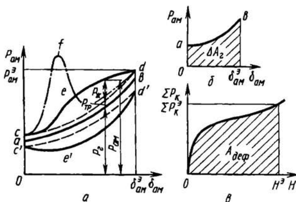
Рис. 7.41. Диаграмма работы однокамерного амортизатора
