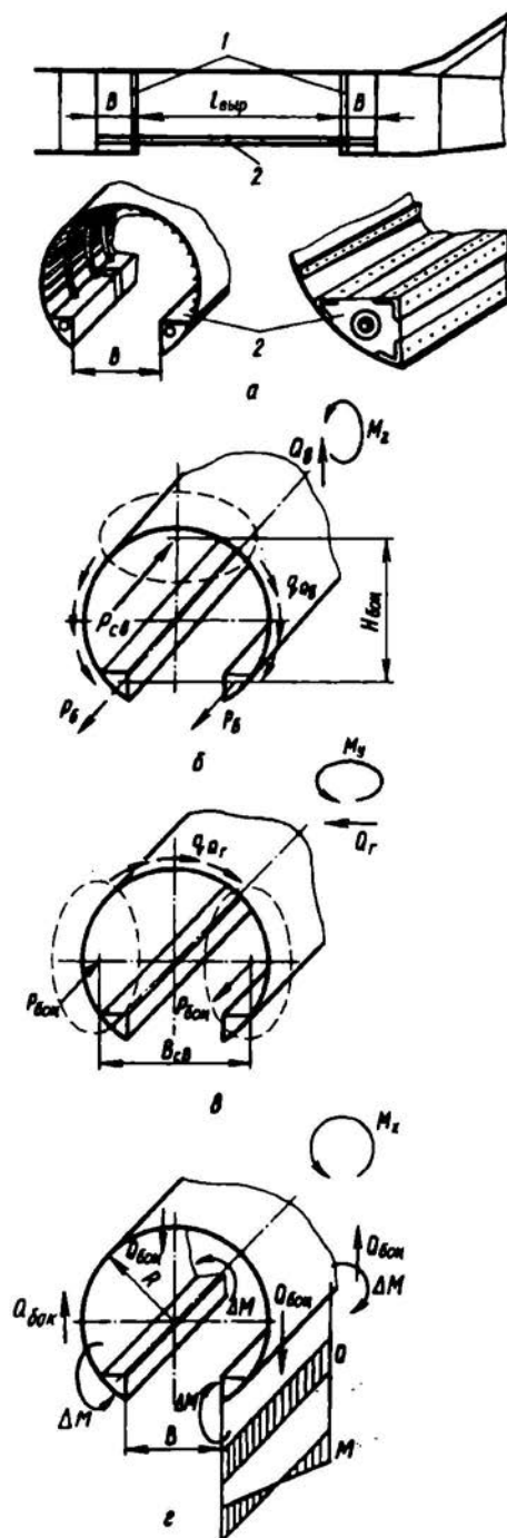
Рис. 6.17. Конструктивное оформление большого выреза в фюзеляже. Схема работы фюзеляжа в районе большого выреза при передаче сил Q_B , Q_T и моментов M_z , M_y и M_K
