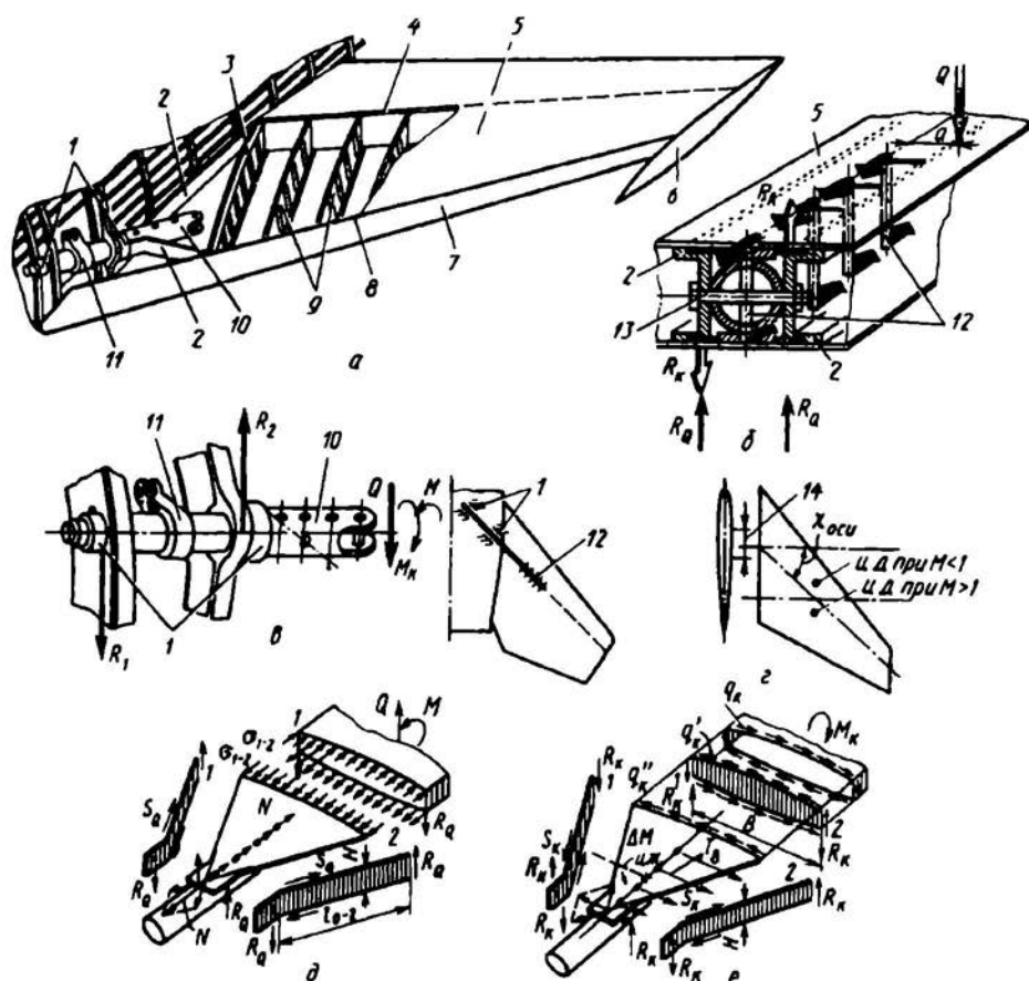
Рис. 5.16. Общий вид, конструкция, нагружение и работа под нагрузкой ЦПГО, выполненного по схеме вала
