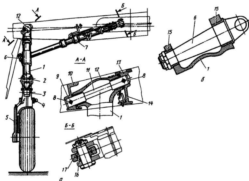
Рис. 7.9. Конструкция основной опоры с цилиндром-подъемником, выполняющим функции подкоса, и узлами крепления стойки
