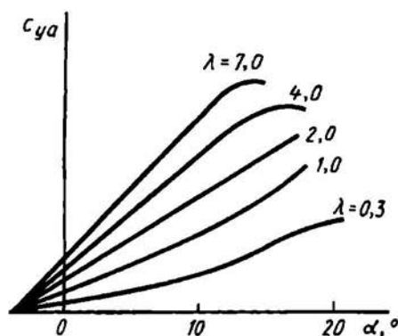
Рис. 2.3. Зависимость c_{ya} = f(\alpha, \lambda)
