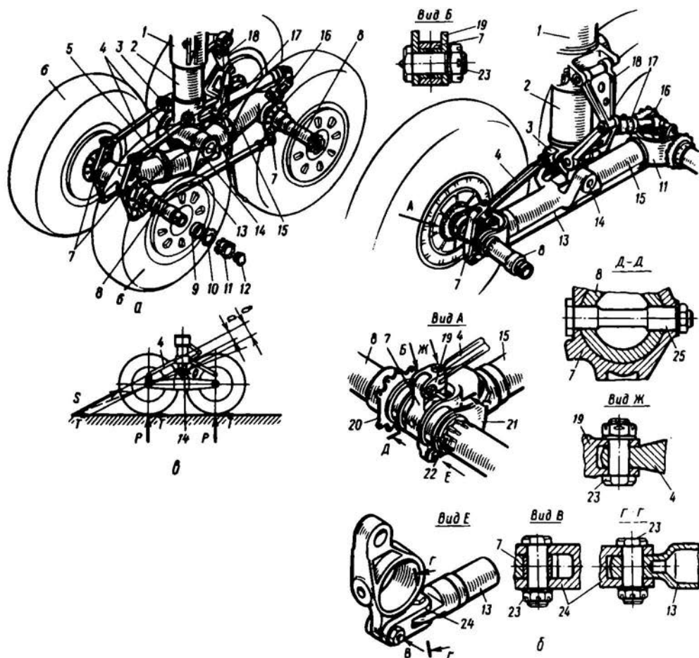
Рис. 7.22. Варианты конструкции многоколесных тележек и их отдельных узлов
