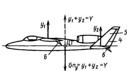
Рис. 3.39. Схема НУПС
