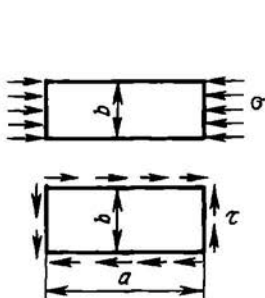
Рис. 2.31. Схема нагружения элементов обшивки сжатием и сдвигом
