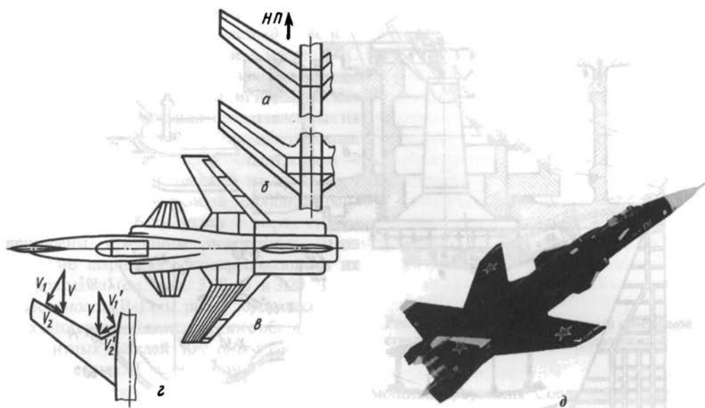
Рис. 3.18. Крылья обратной стреловидности
