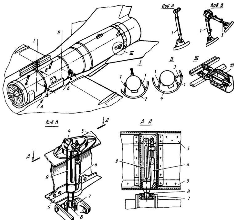
Рис. 9.3. Конструкция узлов крепления ТРД в фюзеляже
