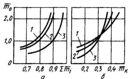
Рис. 1.6. Зависимости относительной взлетной массы самолета \bar{m}_0 от суммы относительных масс его частей без массы целевой нагрузки \Sigma \bar{m}_i (а) и от относительной массы конструкции \bar{m}_к (б)
