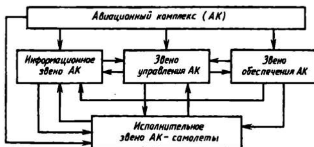
Рис. 1.2. Структура авиационного комплекса
