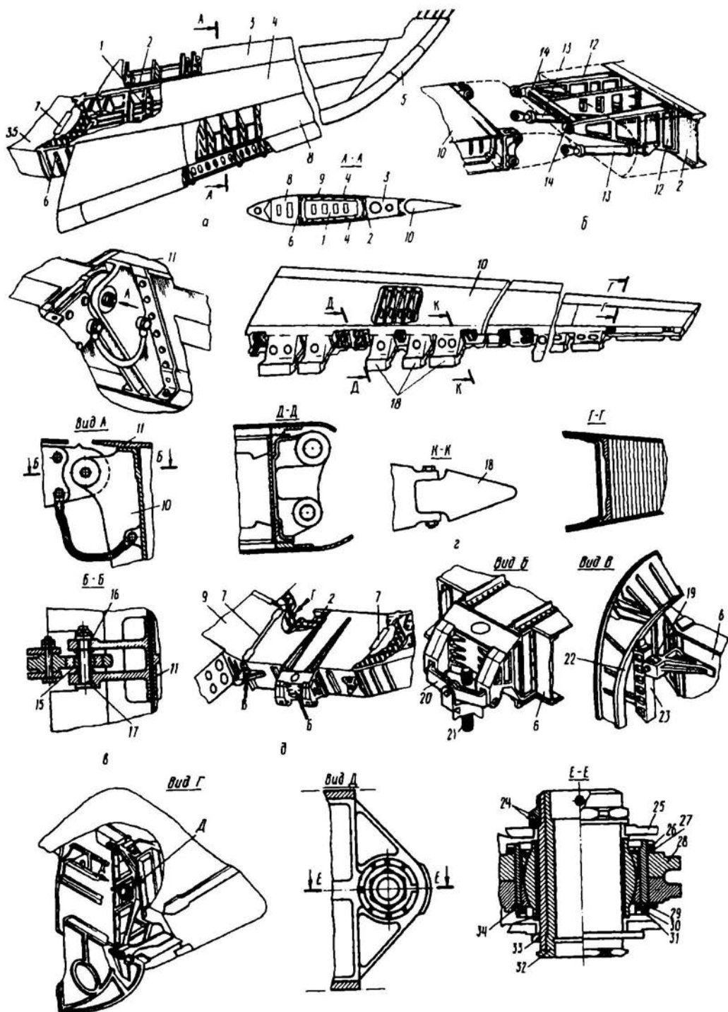
Рис. 5.8. Конструкция стабилизатора, РВ и узлов их крепления
