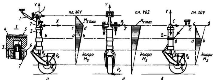
Рис. 7.26. Конструкция и нагружение передней опоры балочной КСС. Эпюры изгибающих моментов. Влияние подкоса на величину изгибающего момента
