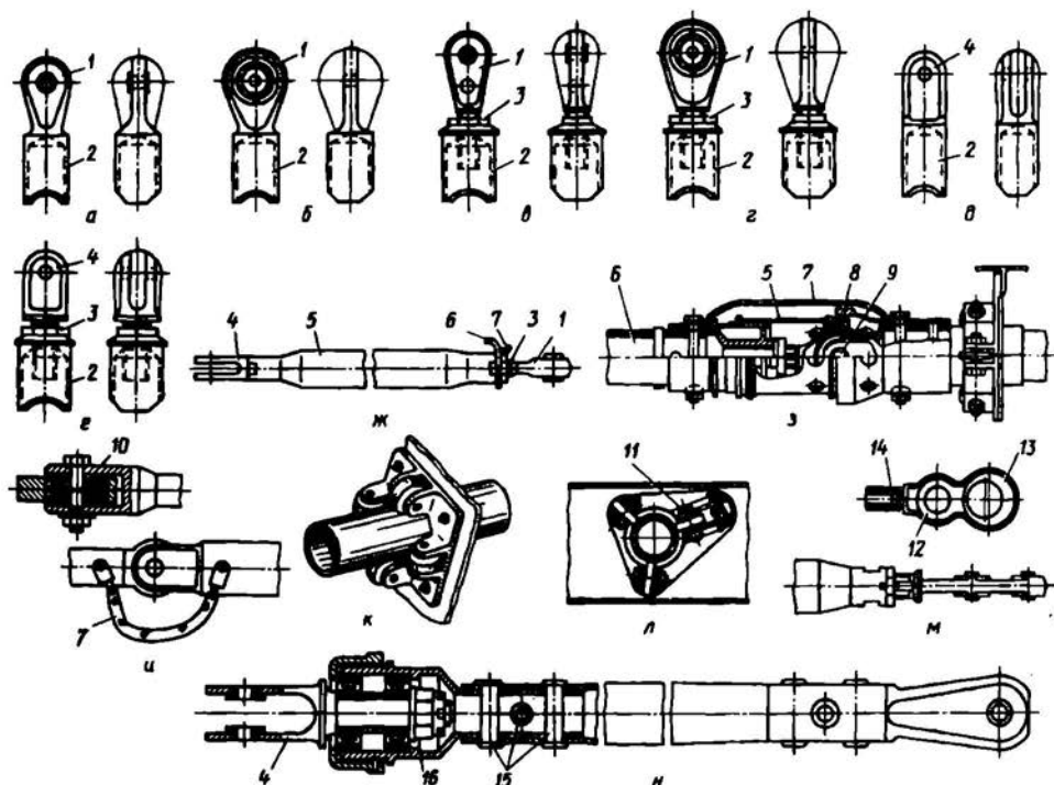
Рис. 8.11. Элементы жесткой проводки управления с помощью тяг
