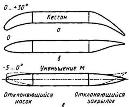
Рис. 2.14. Изменение формы профилей адаптивного крыла
