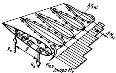
Рис. 2.29. Схема нагружения крыла кручением
