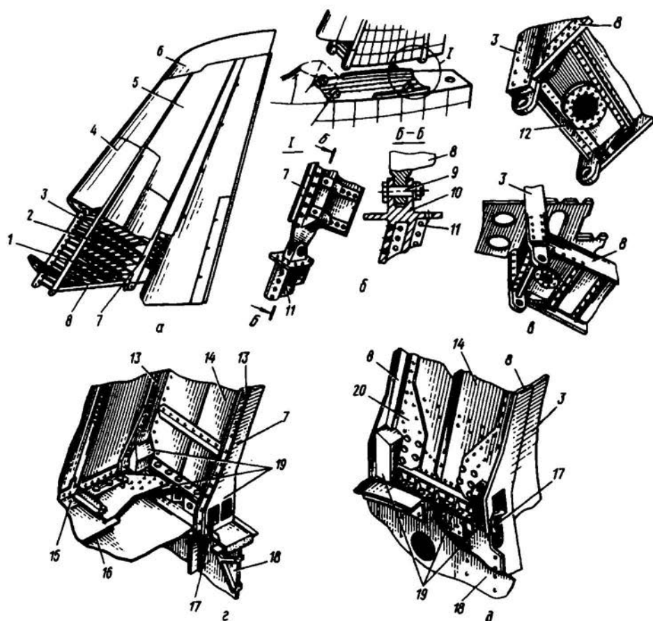
Рис. 5.13. Конструкция киля и узлов его крепления к фюзеляжу
