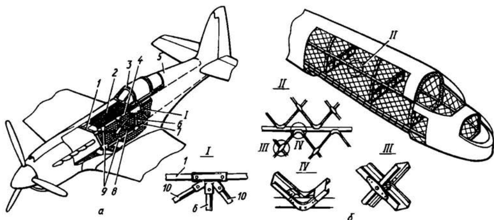
Рис. 6.5. Конструкция фюзеляжа: а — лонжеронного; б — геодезического
