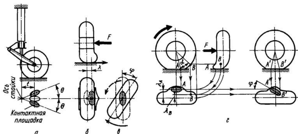
Рис. 7.48. К объяснению явления колебаний типа «шимми»
