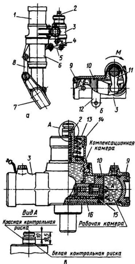
Рис. 7.19. Конструкция гасителя колебаний (демпфера «шимми»)
