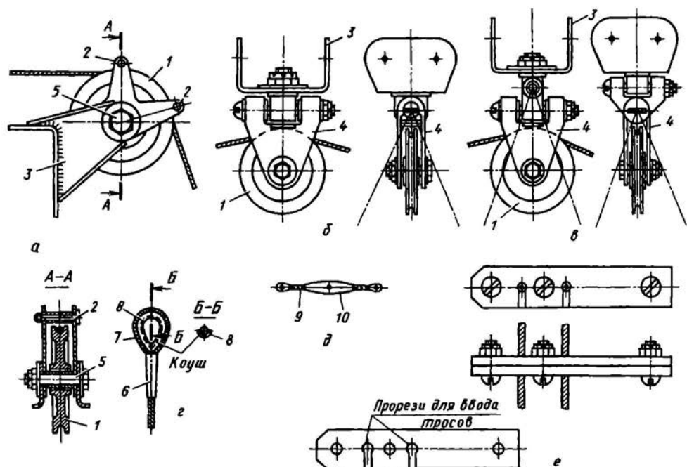
Рис. 8.9. Элементы тросовой проводки управления
