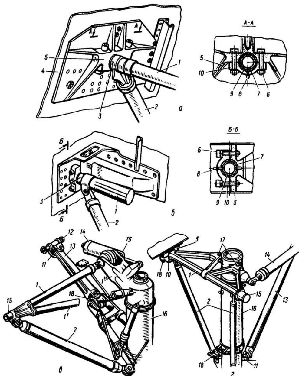
рис. 7.13. Варианты конструкций траверс стоек шасси и узлов их крепления
