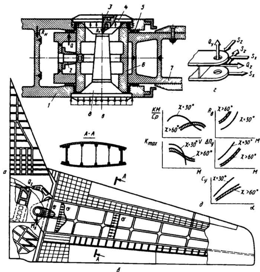
Рис. 3.19. Конструкция крыла изменяемой стреловидности и его главного шарнира. Сравнение характеристик крыльев с разными углами стреловидности
