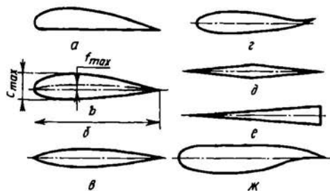
Рис. 2.13. Формы профилей крыла
