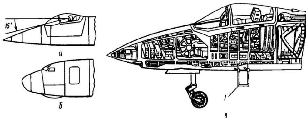
рис. 6.18. Конструкция носовой части фюзеляжа
