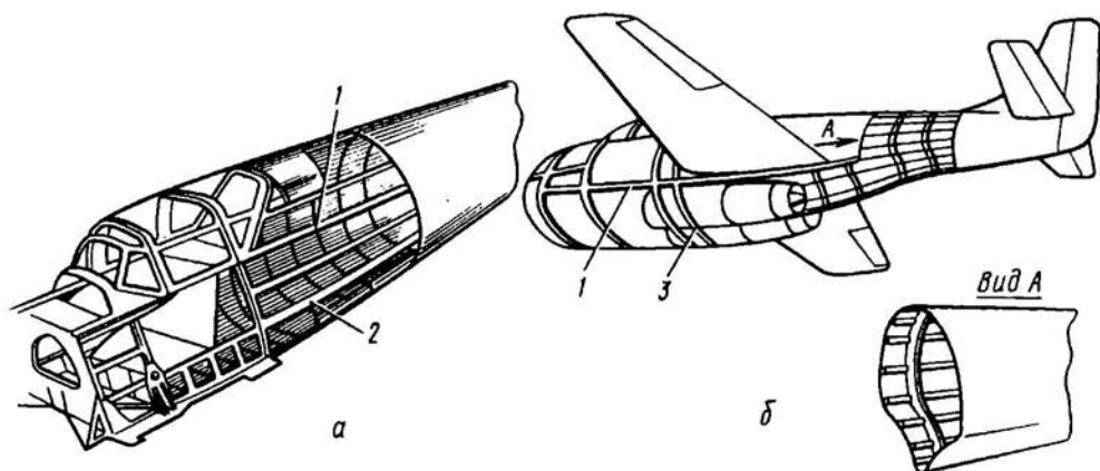
Рис. 6.6 Конструкция фюзеляжей балочно-лонжеронной КСС
