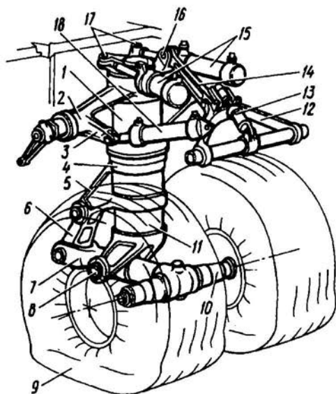
Рис. 7.33. Конструкция передней опоры балочной КСС с подкосом выше траверсы и рычажной подвеской колес
