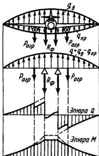
Рис. 2.20. Эпюры Q и M для крыла
