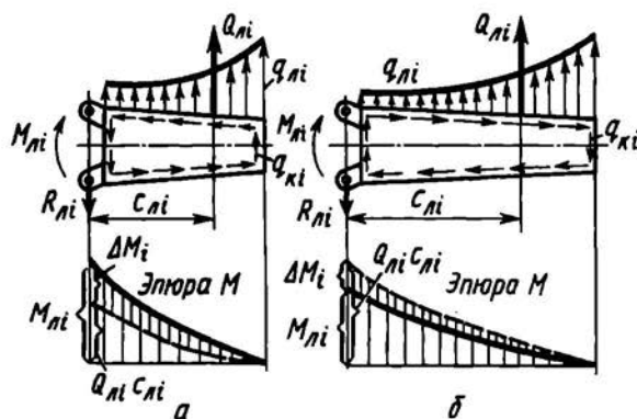
Рис. 3.31. Схема нагружения лонжеронов треугольного крыла с параллельными лонжеронами
