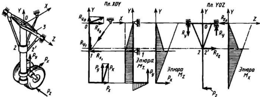
Рис. 7.27. Конструкция и нагружение передней опоры ферменно-балочной КСС
