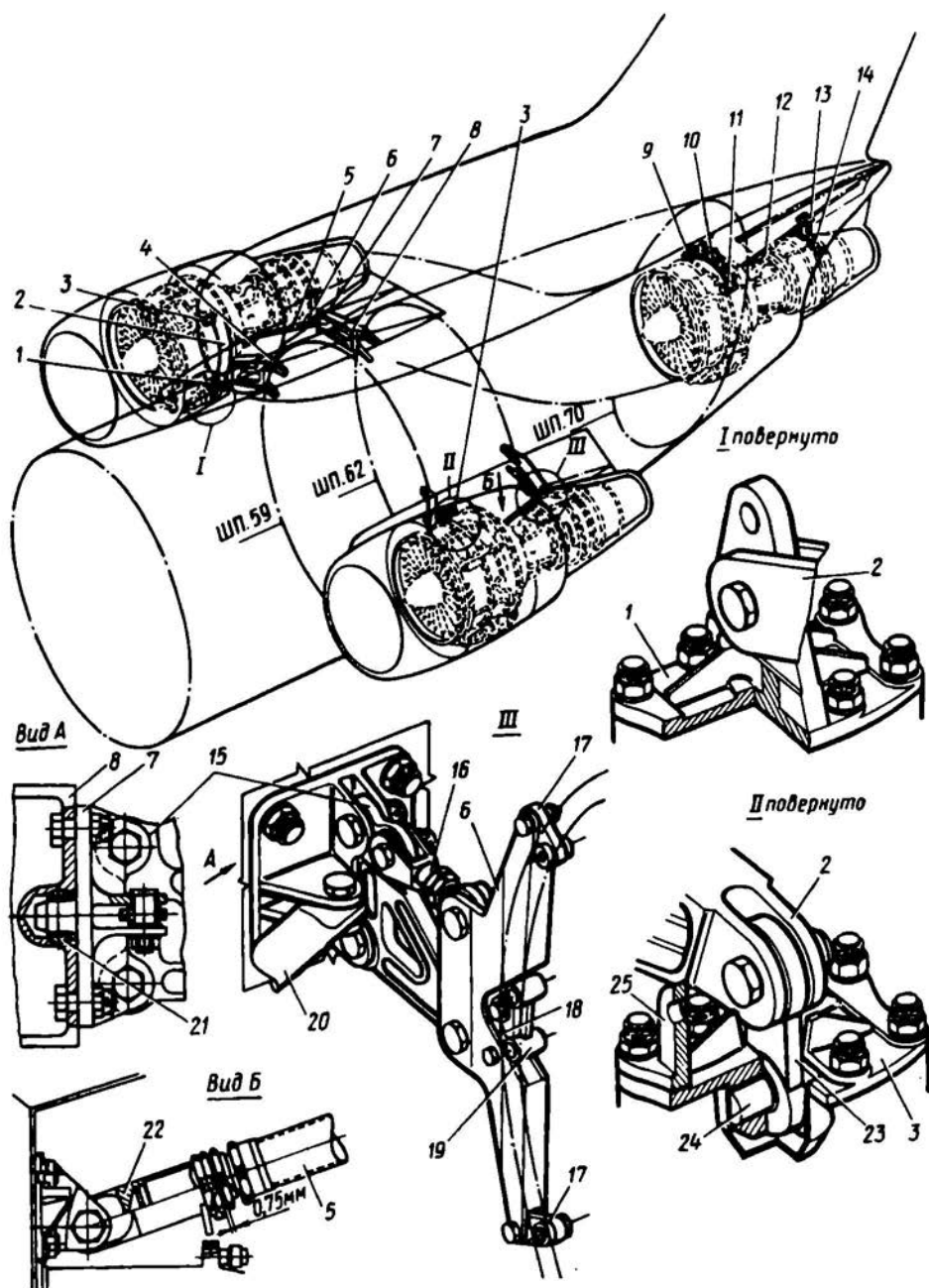
Рис. 9.6. Конструкция узлов крепления двигателей
