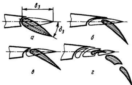
Рис. 4.4. Поворотный (а), выдвижной (б), щелевой (в) и многощелевой (г) закрылки
