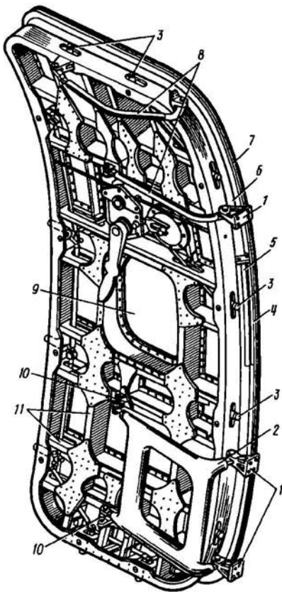
Рис. 6.30. Конструкция двери с кривошипным механизмом, обеспечивающим смещение двери при ее открытии вдоль борта фюзеляжа с внешней его стороны
