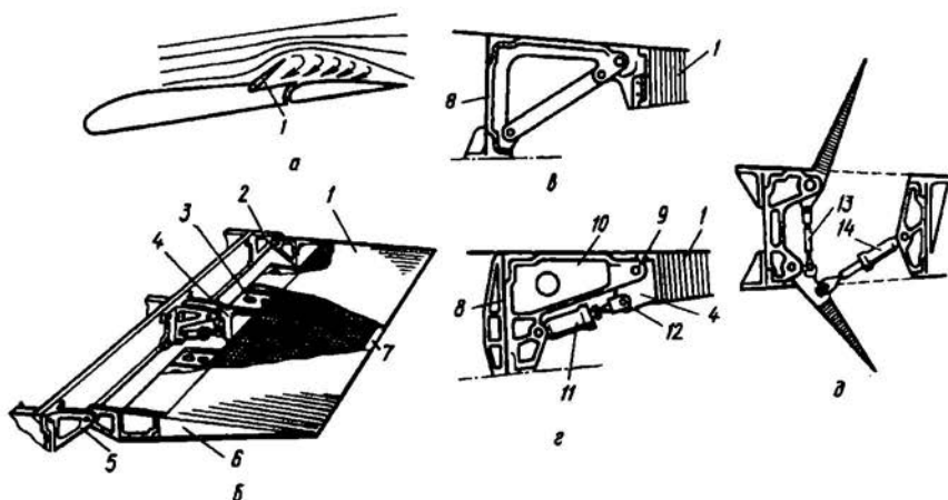
Рис. 4.9. Конструкция интерцептора и узлов его навески и управления
