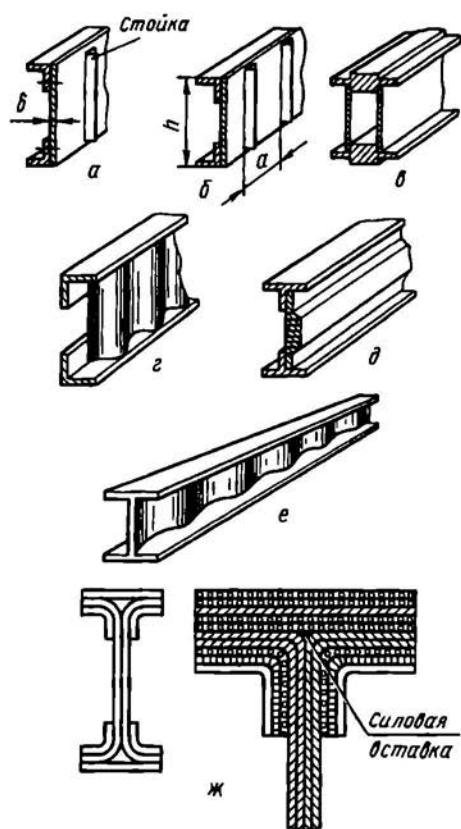
Рис. 2.43. Варианты конструкции стенок лонжеронов
