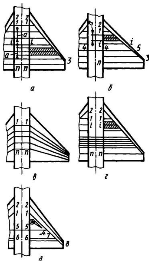
Рис. 3.29. КСС треугольных крыльев
