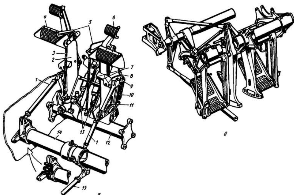
Рис. 8.8. Конструкция постов ногого управления с качающимися педалями с верхней и нижней осями вращения
