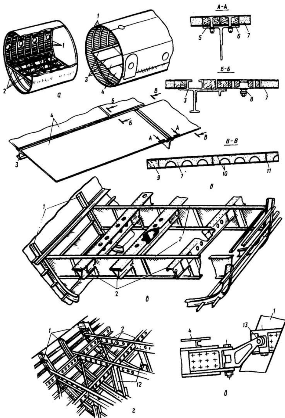
Рис. 6.36. Варианты конструкции пола
