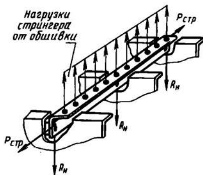
Рис. 2.25. Нагружение стрингера от обшивки и передача этой нагрузки на нервюры
