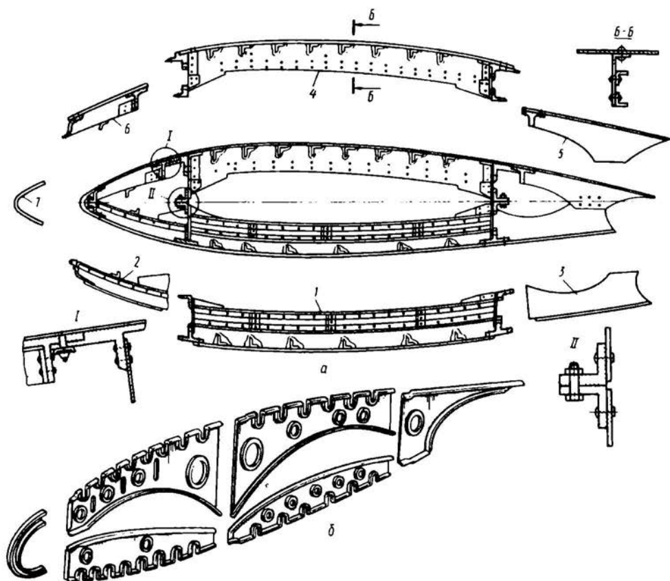
Рис. 2.48. Конструкция нервюры с разъемом вдоль плоскости хорд
