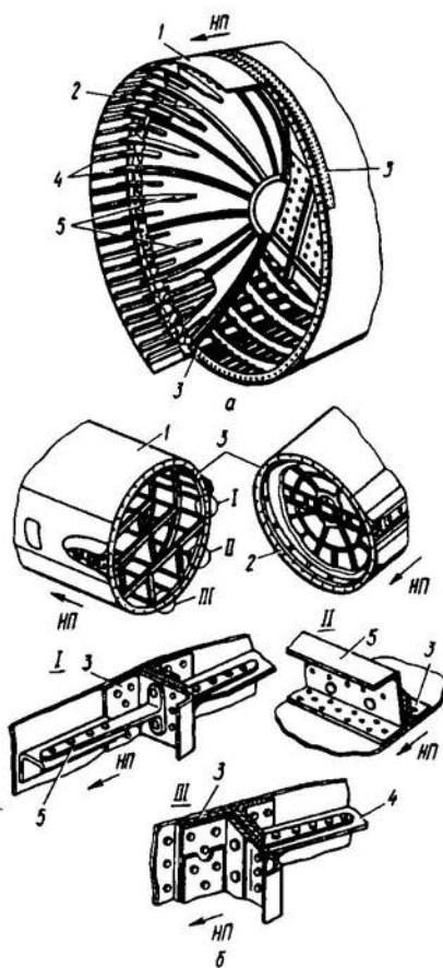
Рис. 6.23. Конструкция сферического гермоднища герметической кабины
