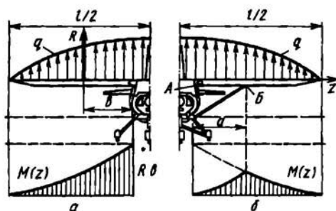
Рис. 1.24. Эпюры огйбающих моментов M_z для лонжерона однолонжеронных крыльев с подкосной балкой и без нее
