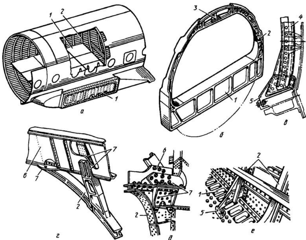
Рис. 6.14. Варианты конструкции стыковых соединений центроплана с фюзеляжем
