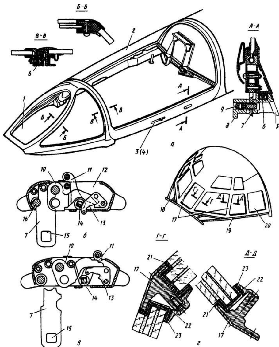
Рис. 6.26. Конструкция фонарей, замков их крепления и узлов закрепления стекол
