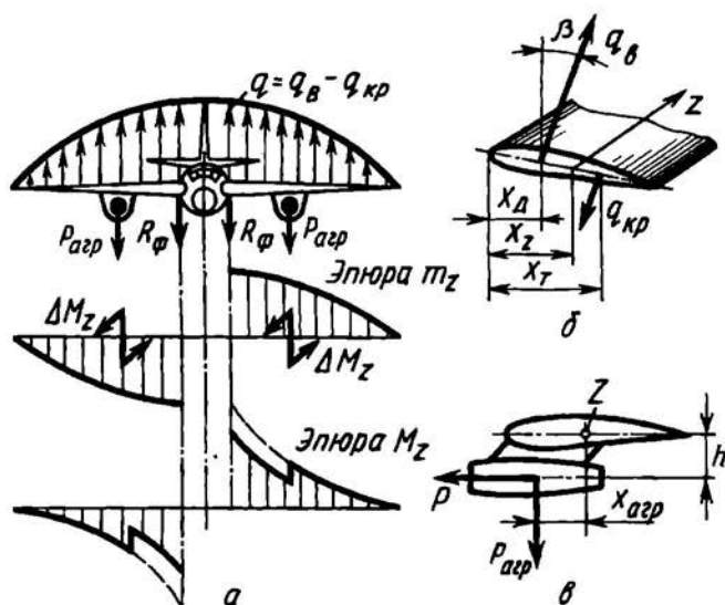
Рис. 2.22. К построению эпюры M для крыла
