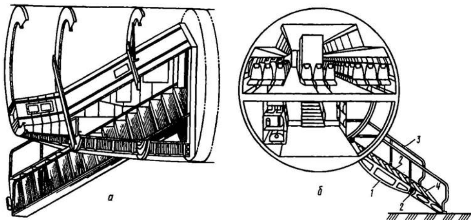
Рис. 6.27. Конструкция двери со встроенным трапом, расположенной: а — в хвостовой части фюзеляжа; б — в нижней части борта фюзеляжа
