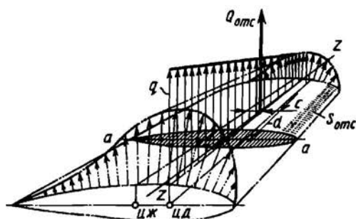
Рис. 2.18. Распределение воздушной нагрузки по размаху и по хорде крыла
