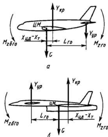
Рис. 5.4. Схема сил, действующих на самолет при разном расположении ГО
