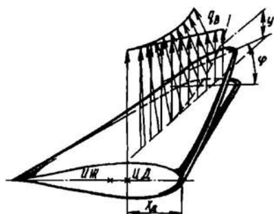
Рис. 2.19. Деформация крыла под действием воздушной нагрузки
