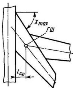
Рис. 3.23. Положение главного шарнира (ГШ)
