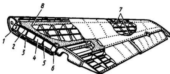
Рис. 3.9. Конструкция двухлонжеронного стреловидного крыла
