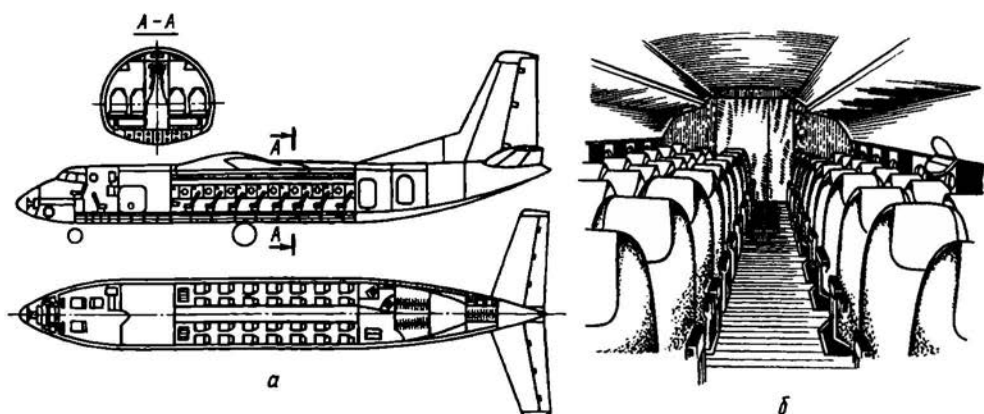
Рис. 6.20. Компоновка фюзеляжа пассажирского самолета и интерьер пассажирского салона
