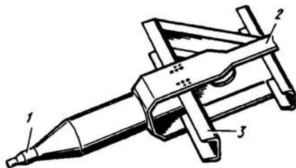
Рис. 5.18. Конструкция вала, связанного с лонжероном ЦПГО
