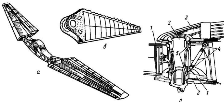
Рис. 3.20. Конструктивная схема крыла изменяемой стреловидности самолета В-1 и его главного шарнира
