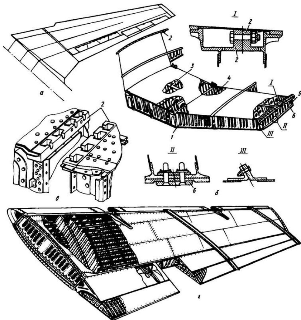
Рис. 3.12. Конструкция кессонных стреловидных крыльев с внешней балкой, лежащей в плоскости крыла
