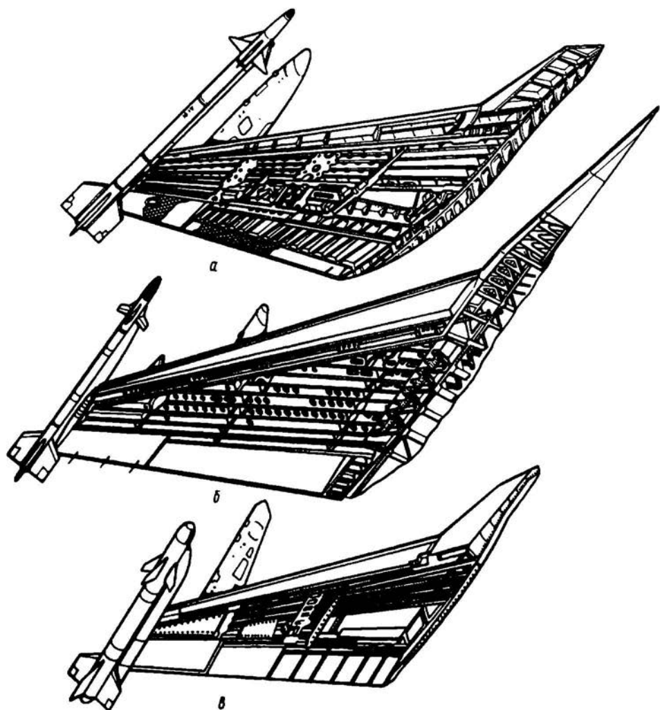
Рис. 2.54. Конструкция многолонжеронных крыльев
