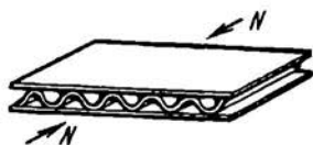
Рис. 2.36. Трехслойная обшивка с гофрированным заполнителем
