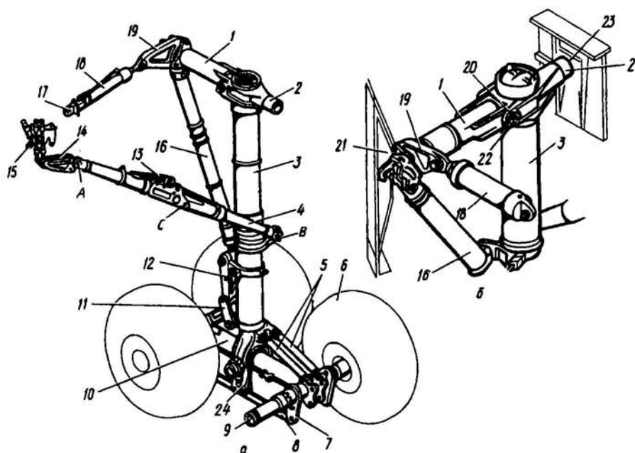
Рис. 7.8. Конструкция основной опоры с тележкой, траверсы и узлов ее крепления
