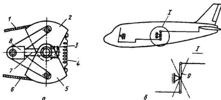
Рис. 8.10. Регулятор натяжения тросов. Компенсационная качалка
