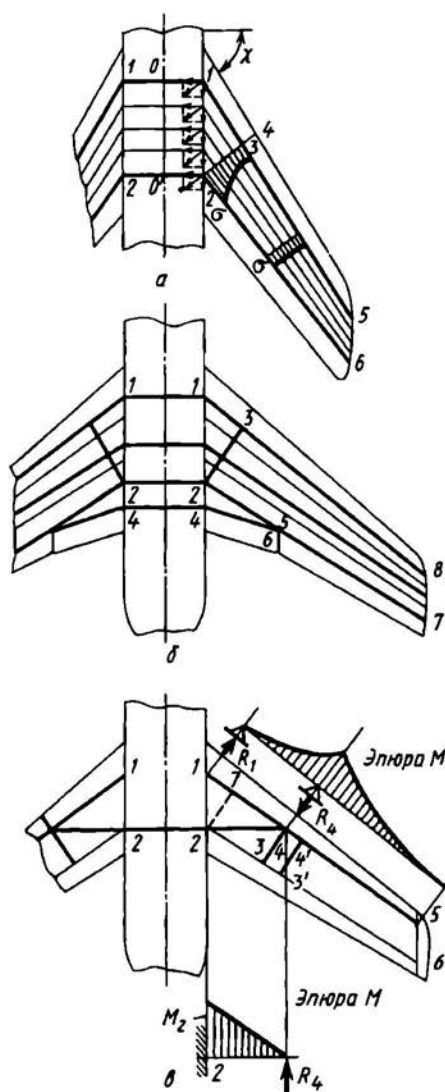
Рис. 3.2. Стреловидные кессонные крылья с переломом осей продольных силовых элементов у борта фюзеляжа (а, б). Крыло с внутренней подкосной балкой (в).
