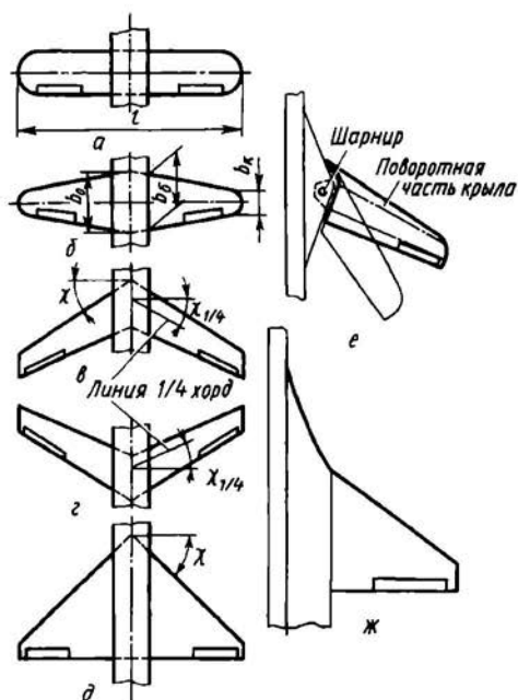
Рис. 2.2. Формы крыльев в плане. Геометрические параметры крыла
