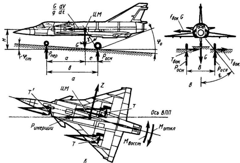
Рис. 7.3. Трекопорная схема шасси с передней опорой, параметры шасси, путевая устойчивость
