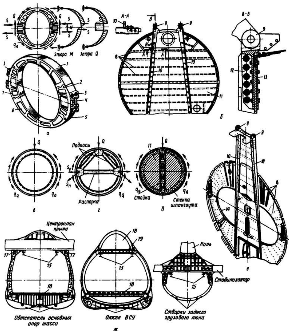
Рис. 6.11. Варианты конструкции усиленных шпангоутов (рамного и стеночного), их нагружение и уравнивание
