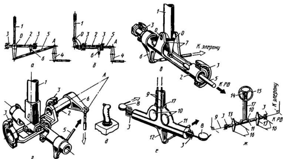
Рис. 8.5. Схемы командных постов ручного управления
