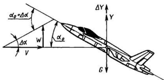
Рис. 1.17. Изменение угла атаки при полете в неспокойном воздухе при вертикальном порыве воздуха со скоростью W
