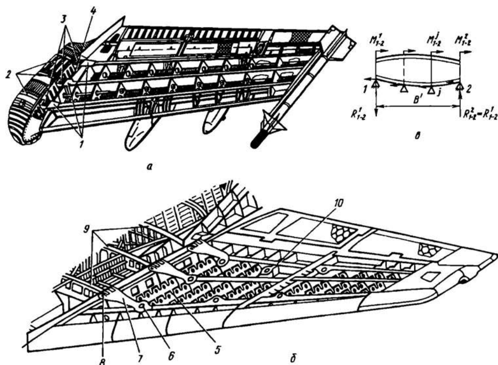
Рис. 3.10. Конструкция многолонжеронных стреловидных крыльев (а, б). Схема нагружения бортовой нервюры (в)
