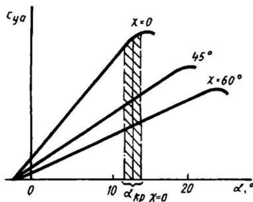
Рис. 2.4. Зависимость c_{ya} = f(\alpha, \chi)
