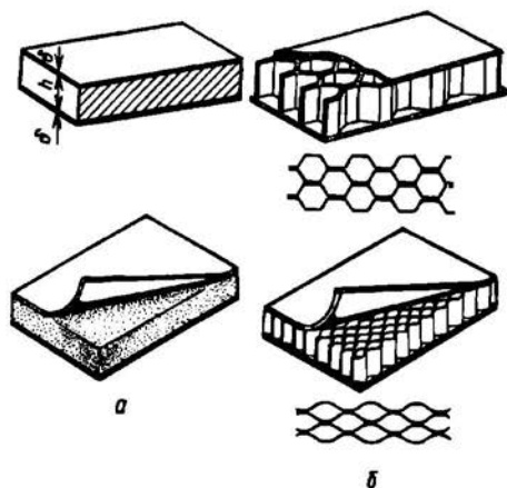
Рис. 2.34. Трехслойная обшивка
