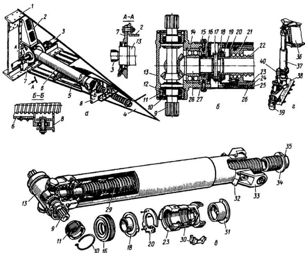
Рис. 8.14. Конструкция винтовых подъемников, используемых в системах управления закрылками, предкрылками и подвижным стабилизатором
