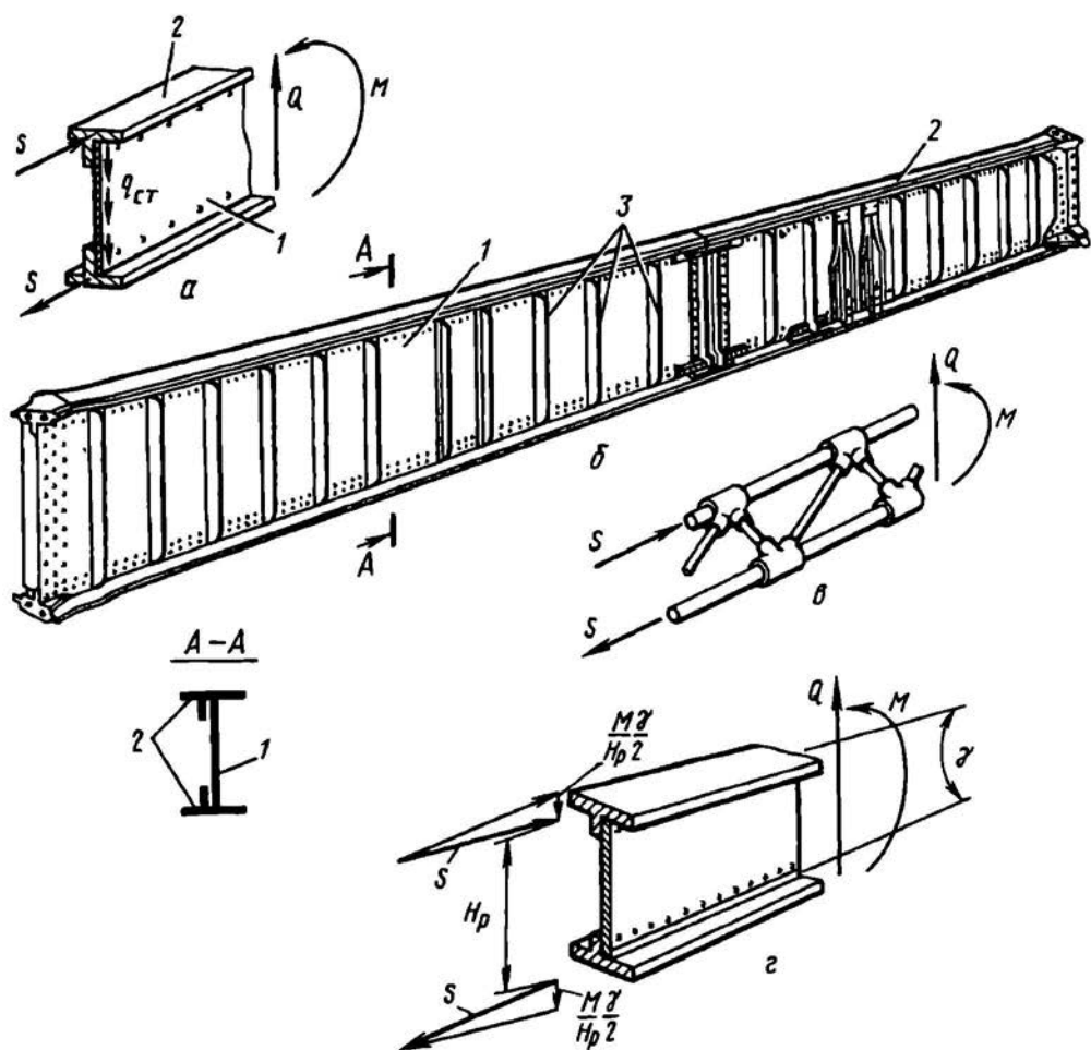
Рис. 2.39. Лонжероны балочной и ферменной конструкций. Уравновешивание поперечной силы Q и изгибающего момента M в сечениях лонжерона
