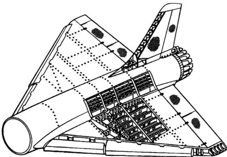
Рис. 3.34. Конструкция треугольного крыла с внутренней подкосной балкой
