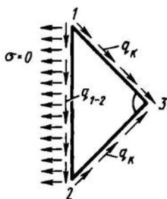
Рис. 3.3. Схема нагружения панели корневой треуголь- ника лонжеронного крыла
