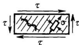
Рис. 2.33. Работа элемента панели на сдвиг
