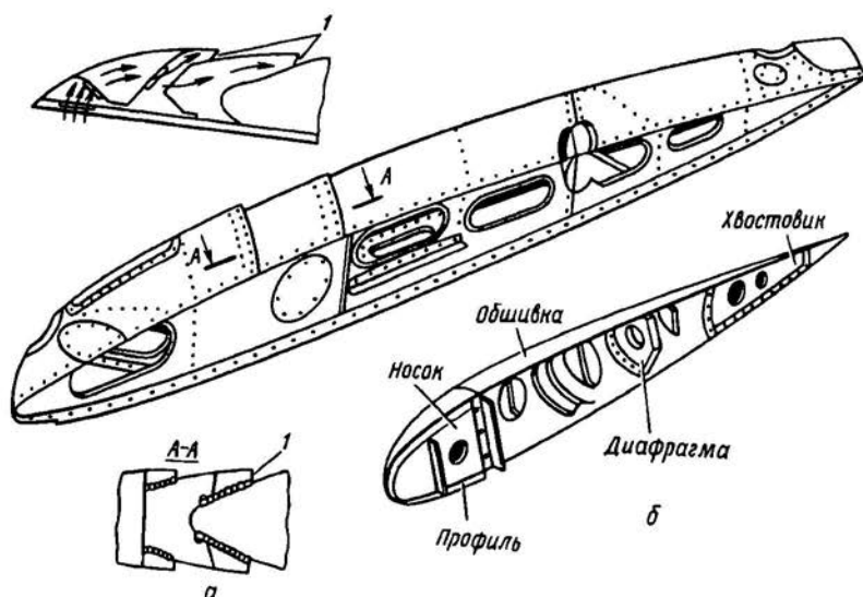
Рис. 2.73. Конструкция законцовок крыльев
