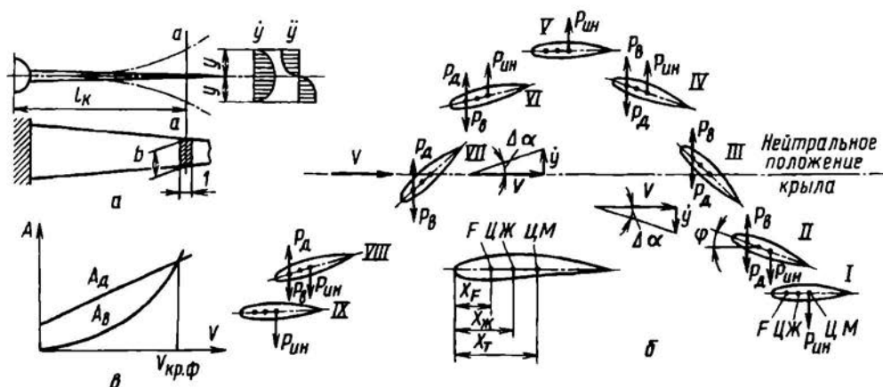
Рис. 10.3. К пояснению явления возникновения изгибно-крутильного флаттера крыла
