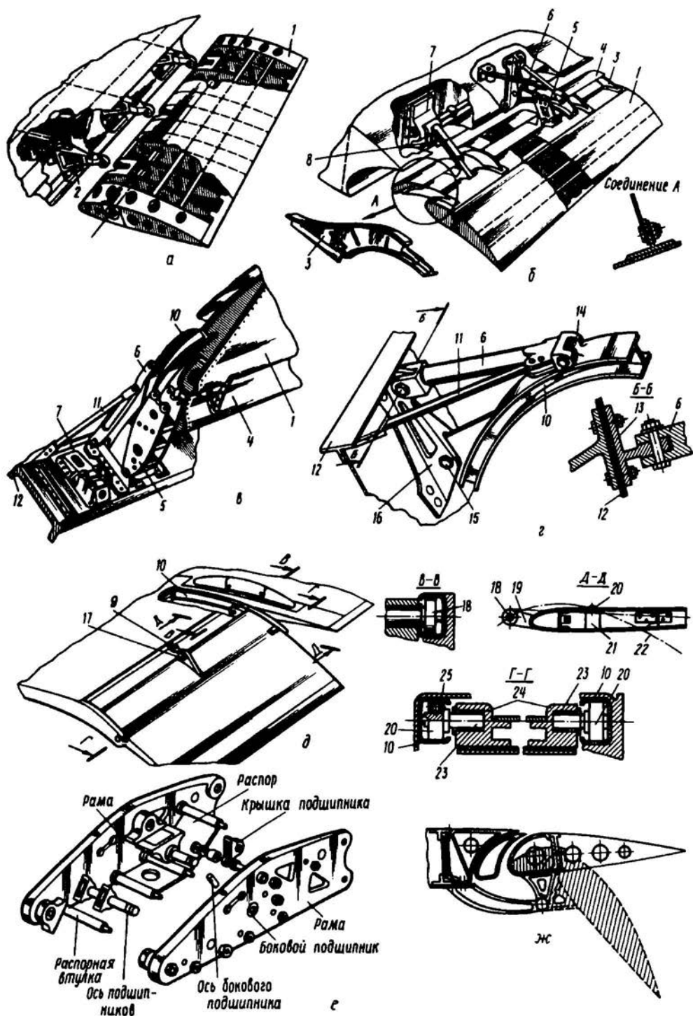
Рис. 4.5. Конструкция поворотного и выдвижного закрылков. Конструкция монорельса и каретки
