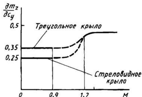
Рис. 2.17. Изменение положения фокуса крыла в зависимости от числа M полета
