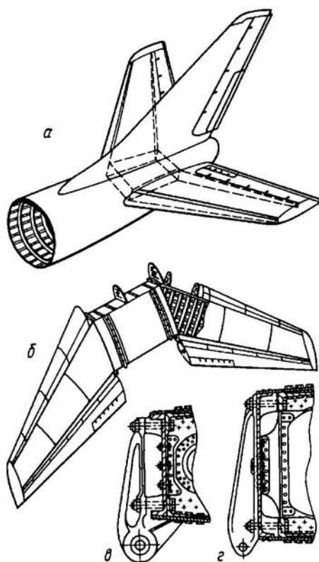
Рис. 5.9. Конструкция ГО и узлов его крепления
