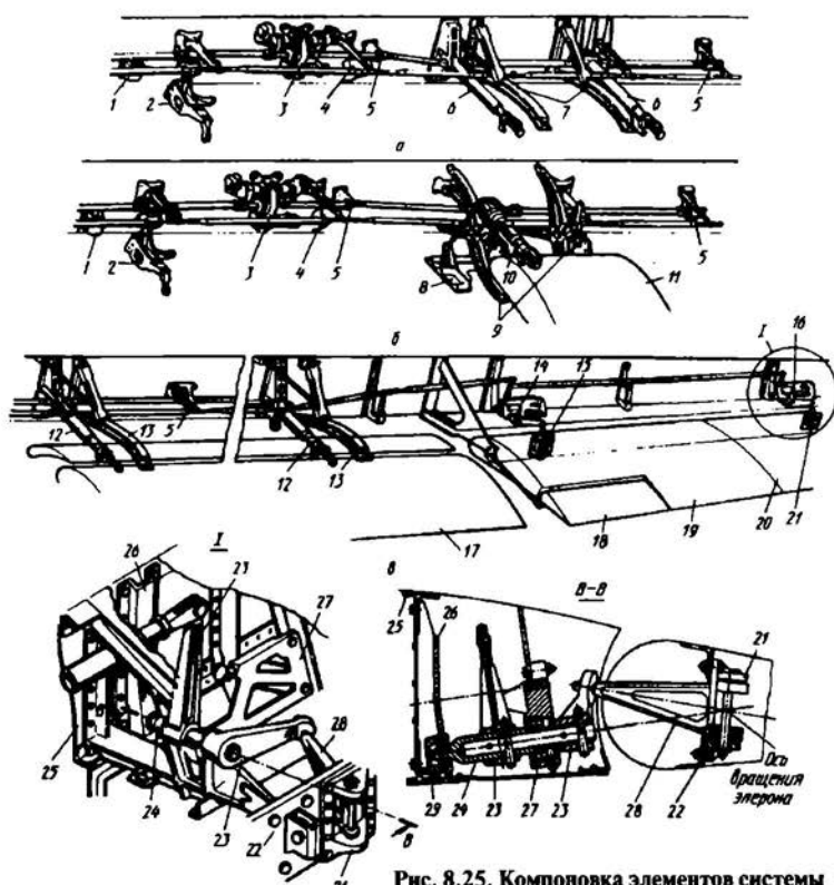
Рис. 8.25. Компонировка элементов системы управления в крыле самолета
