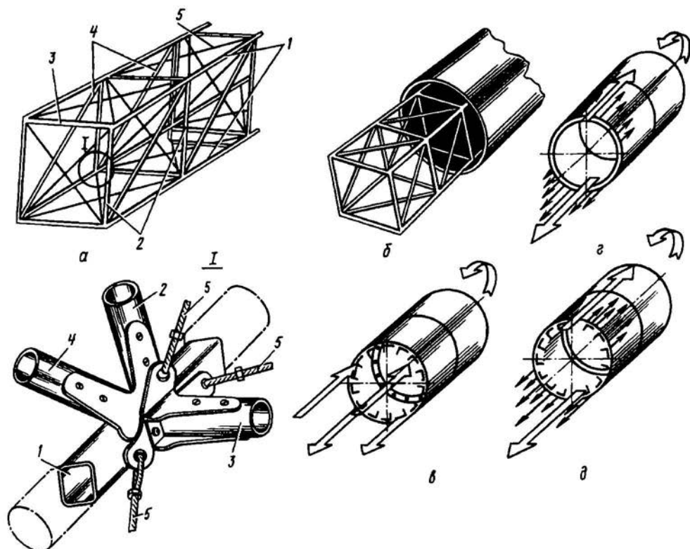
Рис. 6.4. КСС фюзеляжей
