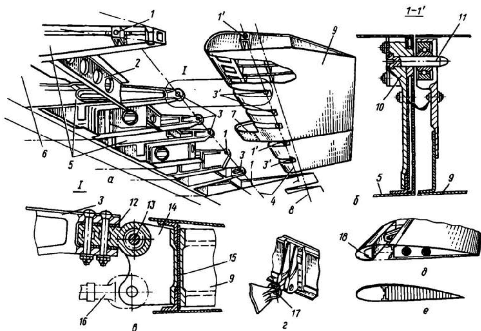
Рис. 4.12. Конструкция элеронов и узлов их навески
