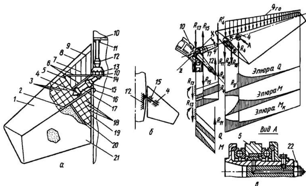
Рис. 5.17. Общий вид, конструкция, нагружение и работа под нагрузкой ЦПГО, выполненного по схеме оси
