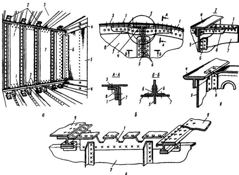
Рис. 2.49. Варианты конструкции стыковых соединений поясов и стенки нервюры с поясами и стенками лонжерона и панелями крыла
