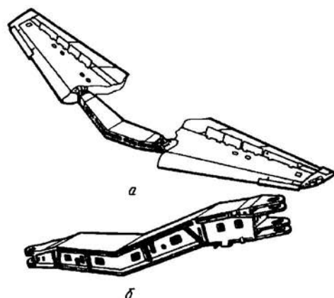
Рис. 3.21. Схема конструкции крыла изменяемой стреловидности и его корневой (неподвижной) части
