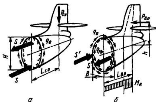
Рис. 1.23. Схема работы тонкостенной оболочки фюзеляжа от нагрузок на оперение:
