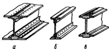
Рис. 2.40. Конструкция составного (а, б) и монолитного (в) лонжеронов
