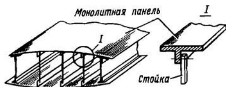
Рис. 2.57. Стойки, соединяющие верхние и нижние монолитные панели крыла
