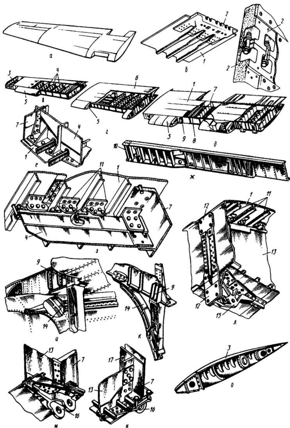
Рис. 2.55. Конструкция кессонного крыла со стыковыми узлами крепления ОЧК между собой и к центроплану (а...д), панелей крыла — к его продольным силовым элементам (е, з, л), центроплана — к фюзеляжу (и, к). Узлы крепления двигателя (л) и шасси (м...н), законцовка крыла (о)
