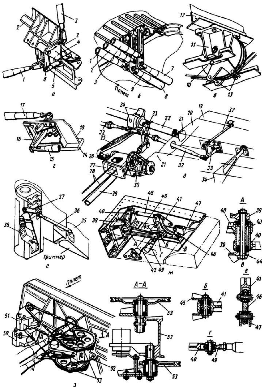
Рис. 8.23. Фрагменты компоновок элементов систем управления на самолете
