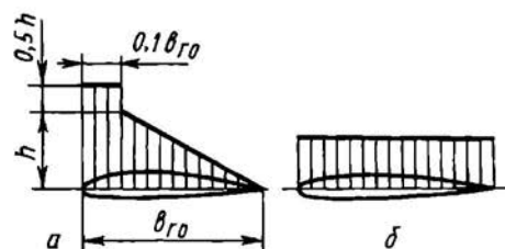
Рис. 5.5. Распределение воздушной нагрузки вдоль хорды:
