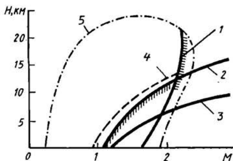
Рис. 1.21. Ограничения диапазона скоростей и высот полета
