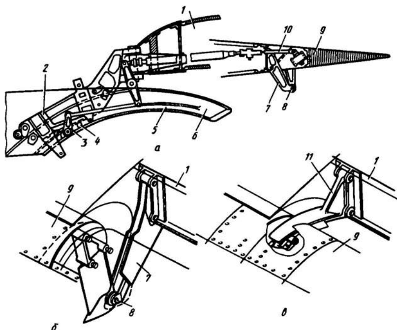
Рис. 4.8. Конструкция хвостового звена трехщелевого закрылка
