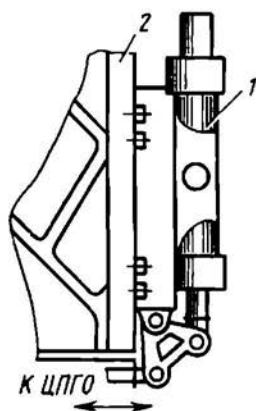
Рис. 5.20. Установка на вертикальной балке киля гидроусилителя в системе управления ЦПГО
