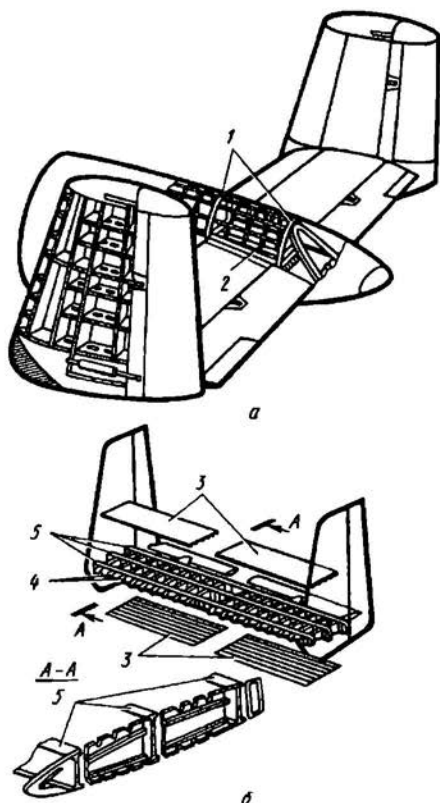
Рис. 5.7. Конструкция оперения самолета А-10
