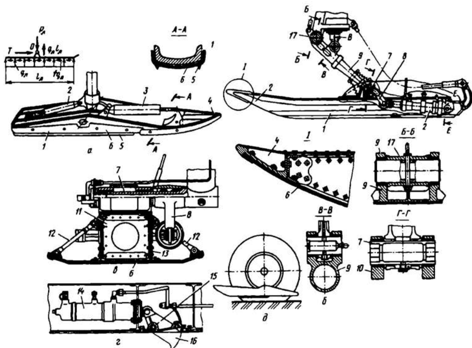
Рис. 7.40. Конструкция лыжи и отдельных ее частей
