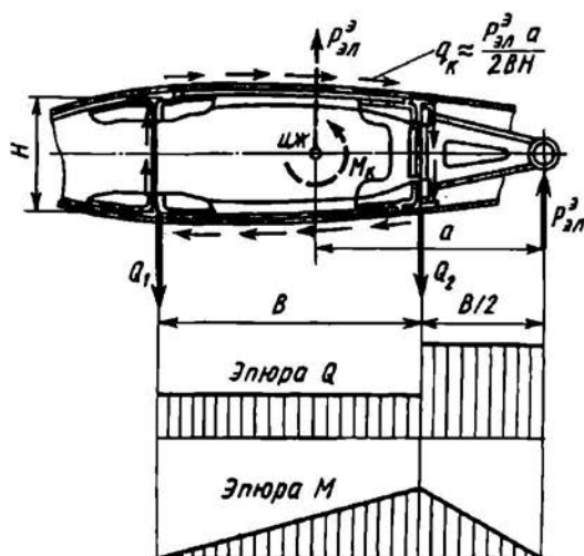
Рис. 2.50. Конструкция, нагружение и уравнивание усиленной нервюры
