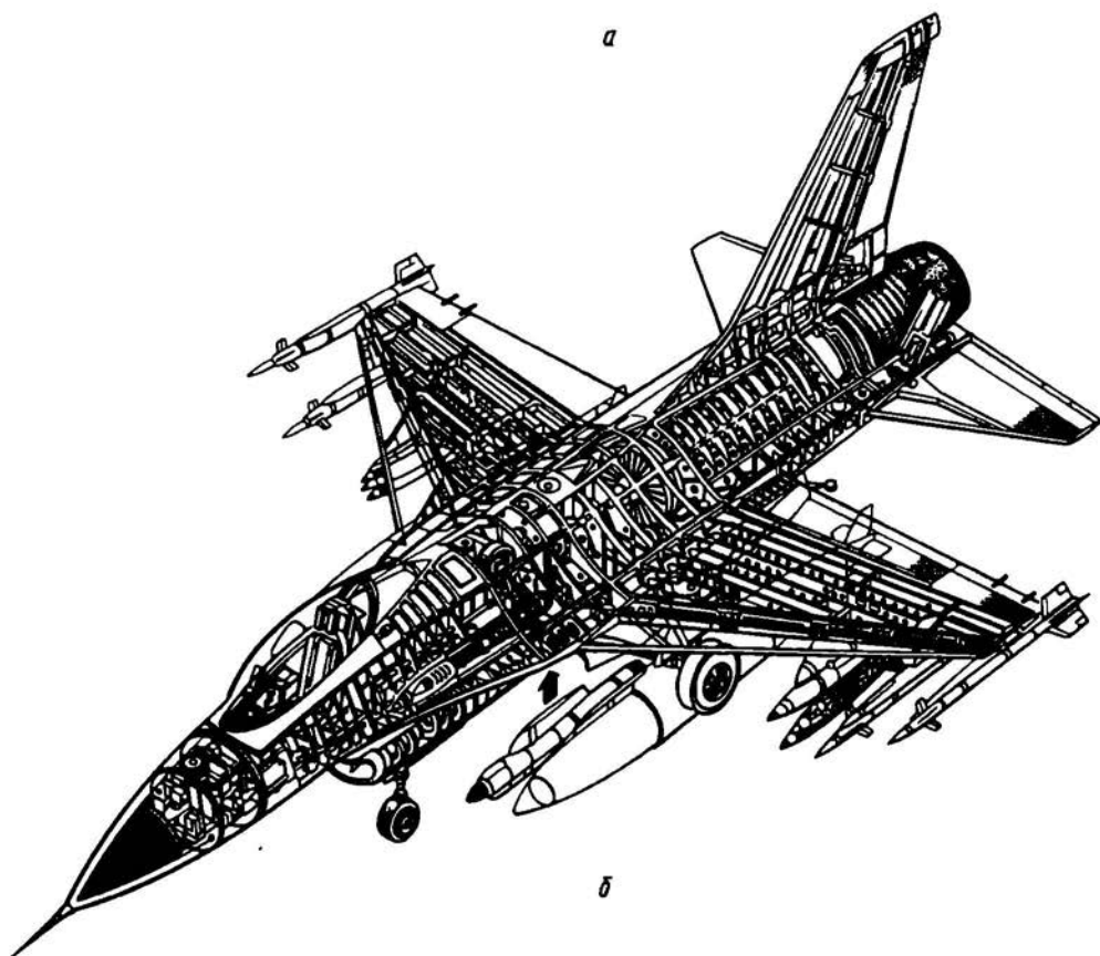
Рис. 6.1. Общий вид, конструкция и компоновка фюзеляжа
