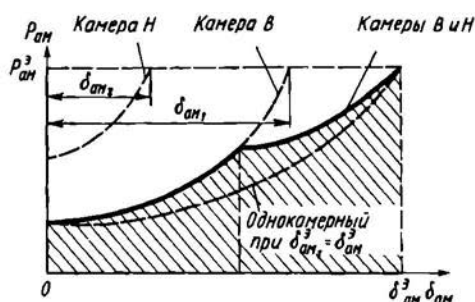
Рис. 7.44. Диаграмма работы двухкамерного амортизатора
