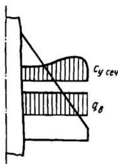
Рис. 2.16. Распределение воздушной нагрузки для треугольного крыла
