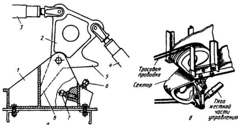
Рис. 8.13. Фрагменты конструкции проводок управления
