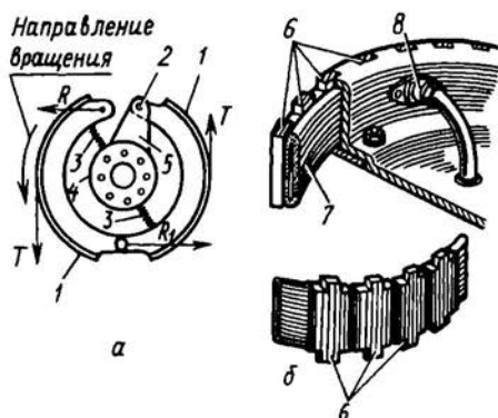
Рис. 7.39. Элементы конструкции тормозов колодочного и камерного типов
