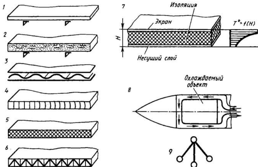
Рис. 1.18. Примеры конструктивных мер борьбы с нагревом
