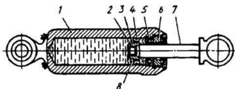
Рис. 7.45. Жидкостный амортизатор
