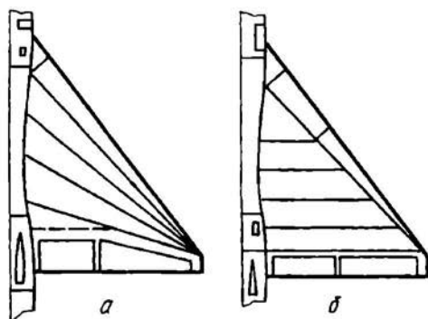
Рис. 1.25. Треугольные крылья со сходящимися (а) и параллельными (б) лонжеронами
