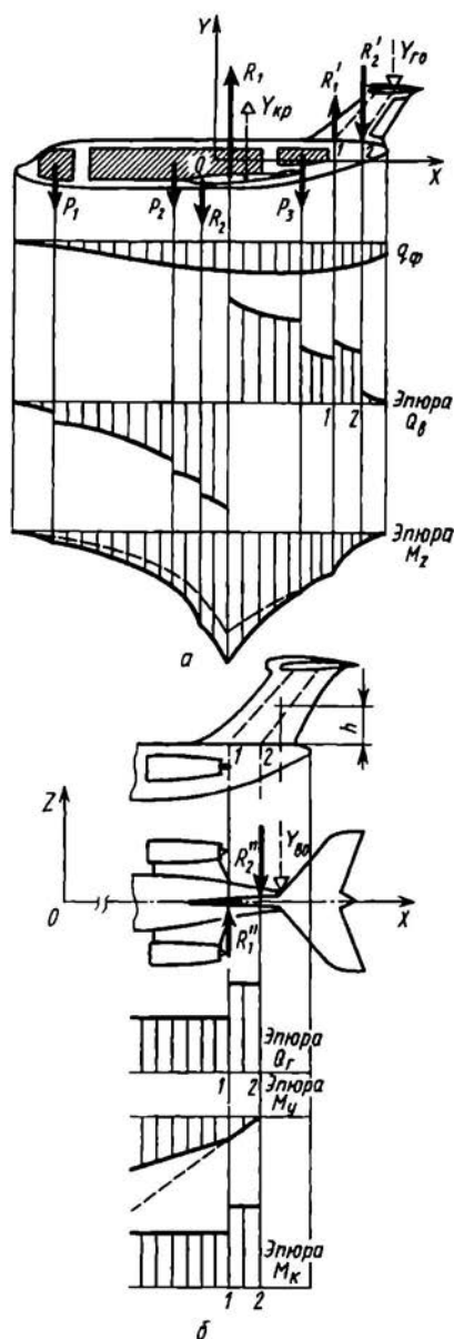
Рис. 6.3. Нагрузки на фюзеляж. Эпюры Q_\phi , Q_g , M_z , M_y , M_k
