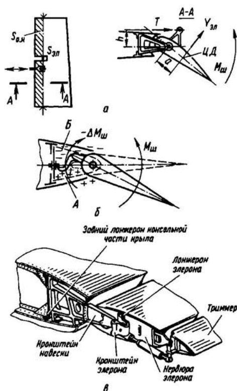
Рис. 4.13. Аэродинамическая компенсация
