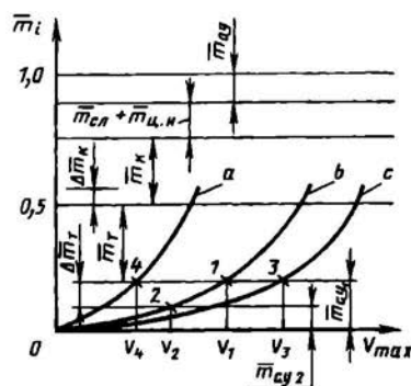
Рис. 1.5. Графическая интерпретация одной из форм уравнения существования самолета (уравнения (1.3))
