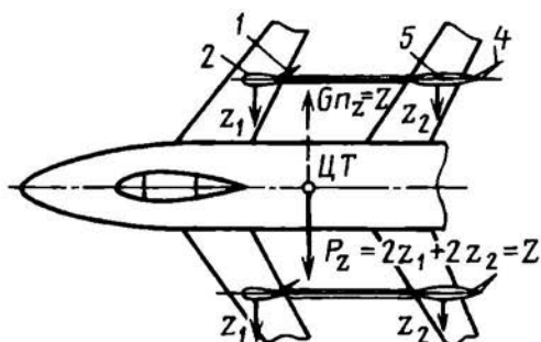
Рис. 3.40. Схема НУБС
