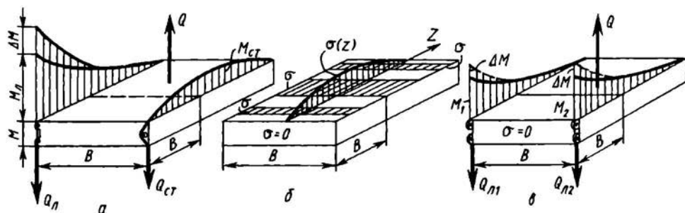
Рис. 2.66. Влияние типа узлов крепления крыла на характер нагружения (работы) его силовых элементов
