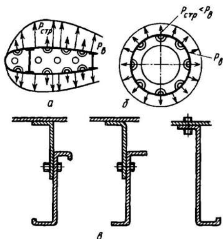
Рис. 6.10. Формы сечений и нагружение нервюры и шпангоутов
