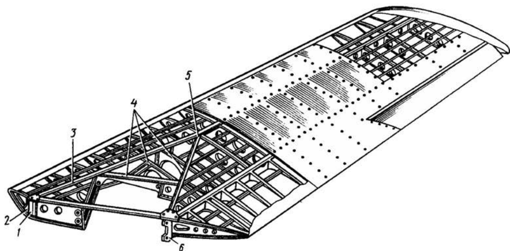
Рис. 3.16. Конструкция стреловидного крыла с внутренней подкосной балкой
