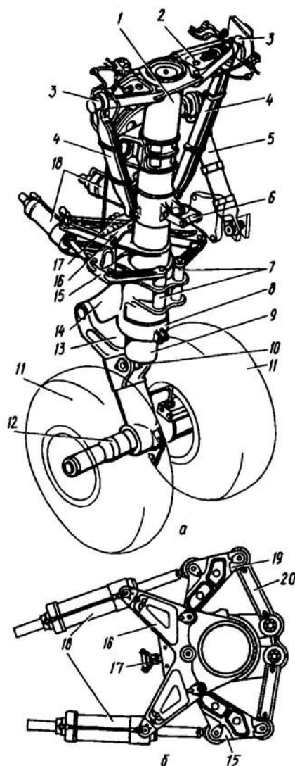
Рис. 7.10. Конструкция передней опоры
