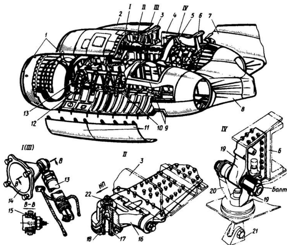
Рис. 9.7. Конструкция спаренных гондол и узлов крепления двигателей самолета Ил-62
