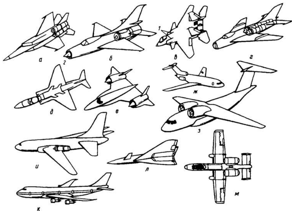
Рис. 9.1. Варианты компоновок двигателей на самолете
