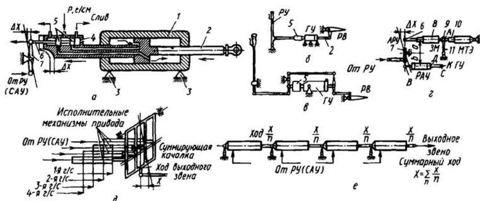
Рис. 8.16. Принципиальная схема конструкции ГУ. Автоматика в системе управления с ГУ, включенным по необратимой схеме
