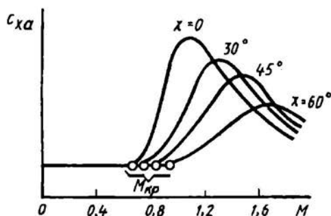
Рис. 2.5. Зависимость c_{xa} = f(M, \chi)
