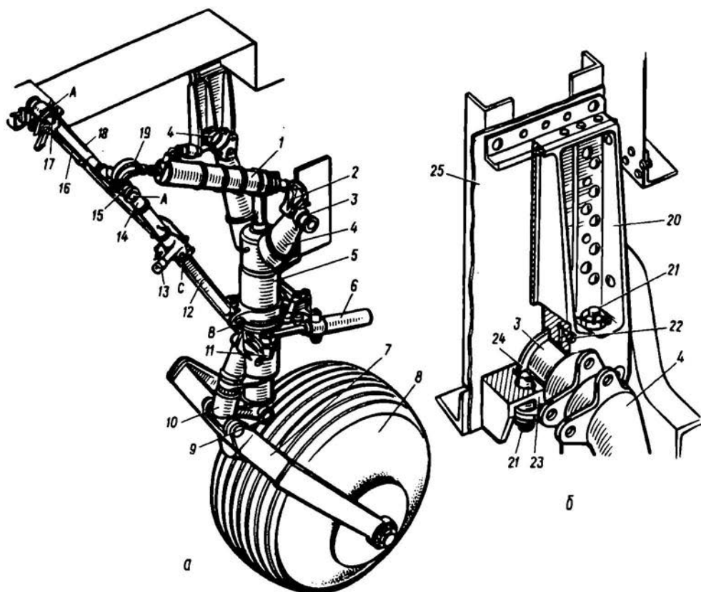
Рис. 7.11. Конструкция передней опоры с узлами ее крепления в фюзеляже
