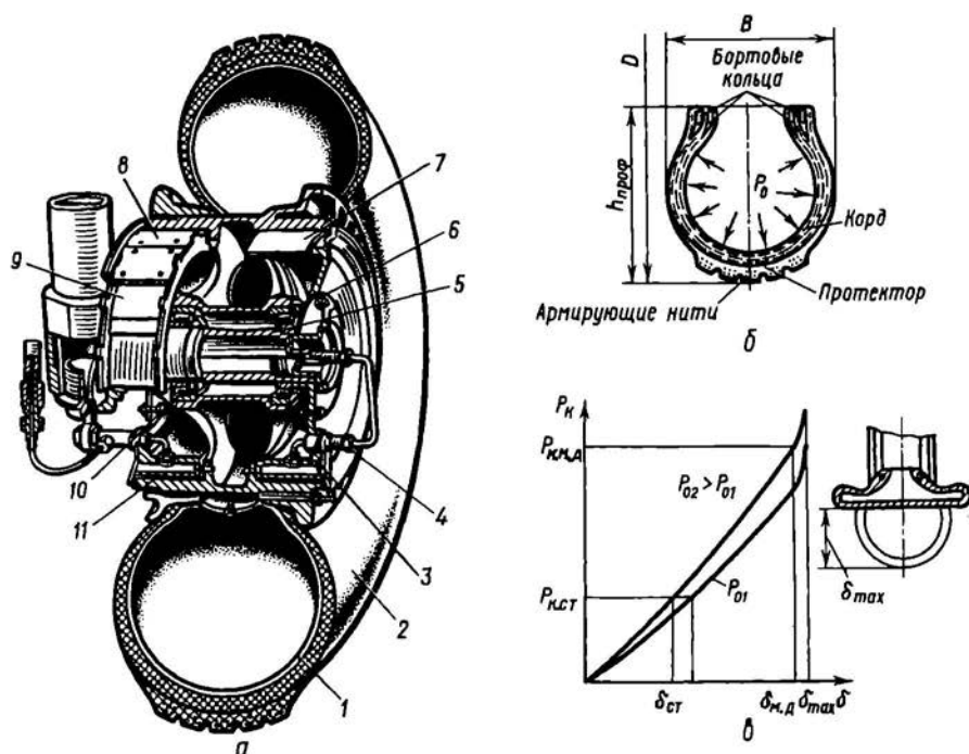
Рис. 7.37. Конструкция колеса и диаграмма его работы
