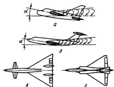
Рис. 5.3. Аэродинамические схемы самолета с различным расположением ГО
