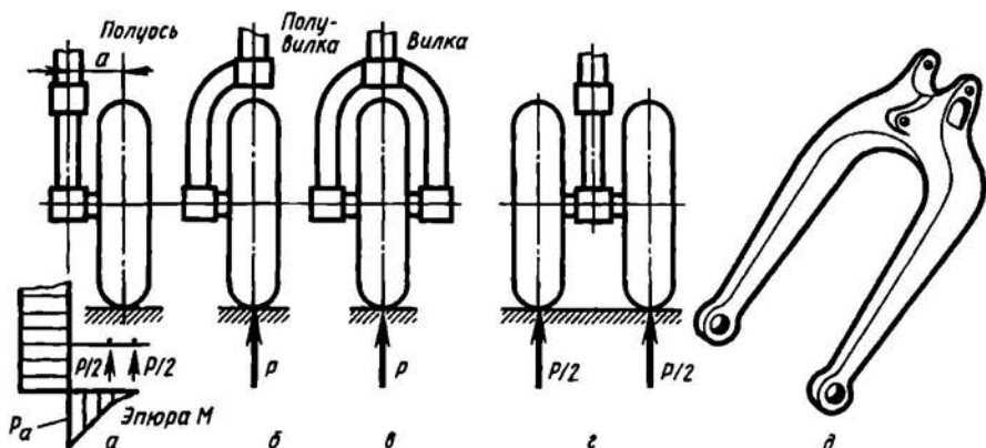
Рис. 7.21. Варианты крепления колес к штоку стойки
