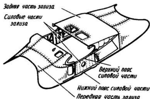
Рис. 2.70. Конструкция зализов крыла
