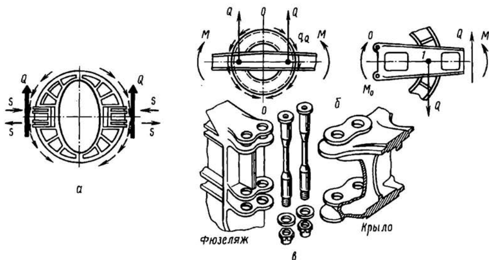
Рис. 2.62. Варианты нагружения и уравнивания усиленных шпангоутов от нагрузок крыла (а, б). Вариант конструкции узлов крепления крыла (в)
