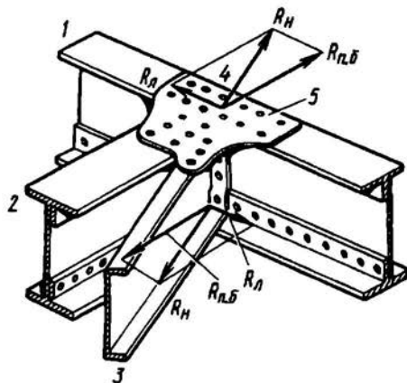
Рис. 3.15. Конструкция стыкового узла лонжерона, подкосной балки и корневой нервюры
