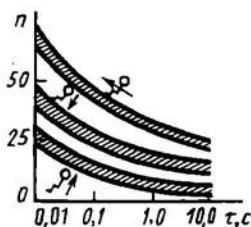
Рис. 1.15. Уровни перегрузок, переносимых летчиком, в зависимости от направления их действия и продолжительности
