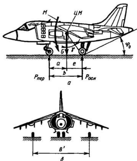
Рис. 7.4. Двухопорное велосипедное шасси и его параметры
