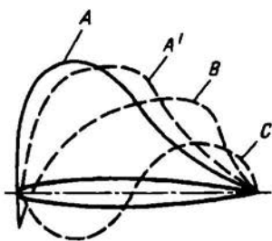
Рис. 1.19. Распределение воздушной нагрузки вдоль хорды крыла для различных случаев нагружения
