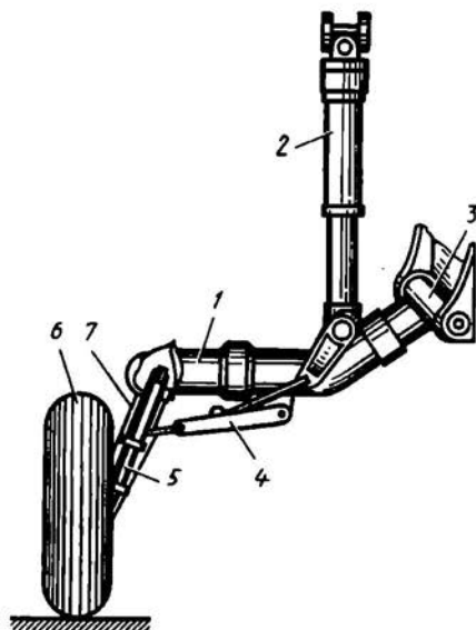
Рис. 7.30. Конструкция основной опоры балочной КСС с подкосом и рычажной подвеской колеса
