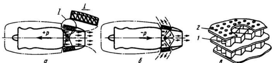
Рис. 9.10. Схемы реверсоров тяги на двигателе
