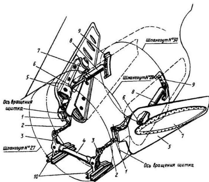
Рис. 8.24. Тормозные щитки и их установка
