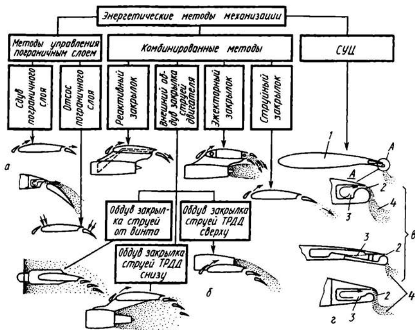
Рис. 4.11. Энергетические методы механизации крыла
