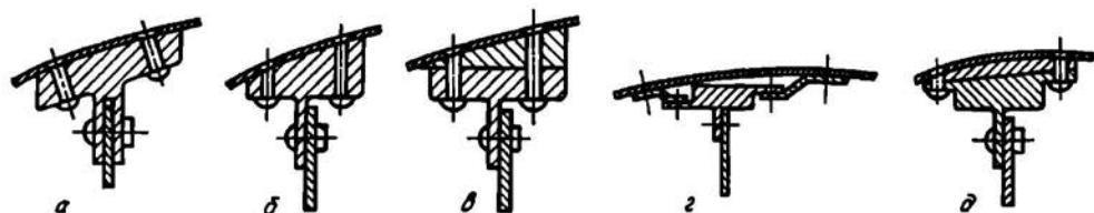
Рис. 2.42. Типовые соединения обшивки с поясом лонжерона
