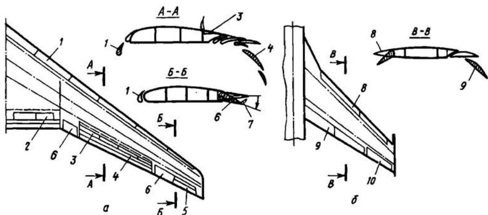
Рис. 4.1. Подвижные части крыла
