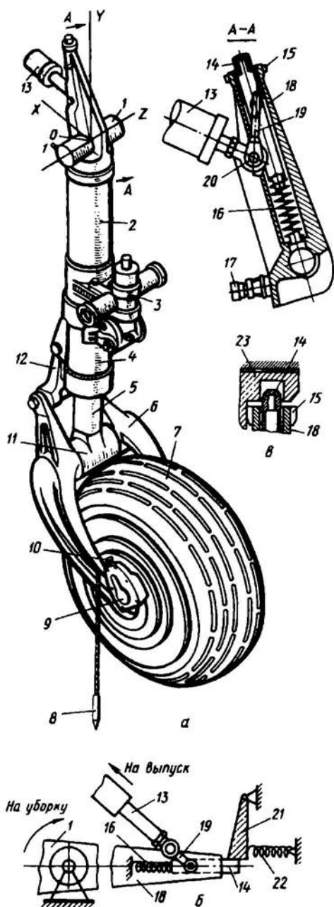
Рис. 7.12. Конструкция передней опоры и замков выпущенного и убранный положений
