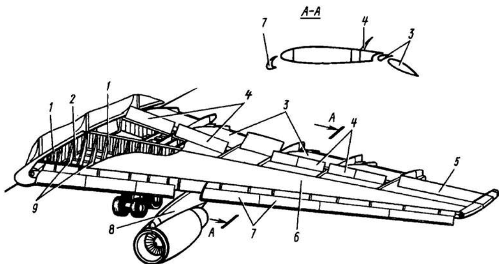
Рис. 2.1. Крыло современного пассажирского самолета
