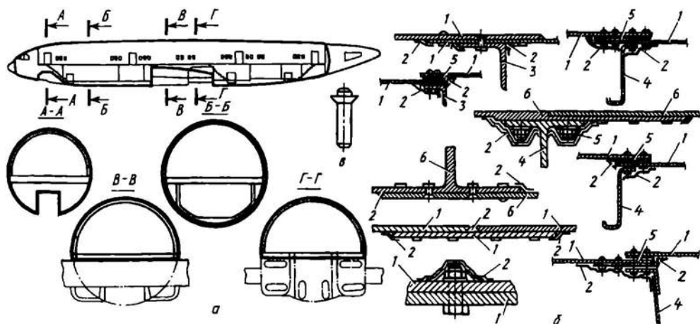
Рис. 6.24. Гермокабина с сечениями. Варианты герметизации стыковых соединений
