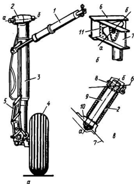
Рис. 7.29. Конструкция основной опоры балочной КСС с подкосом
