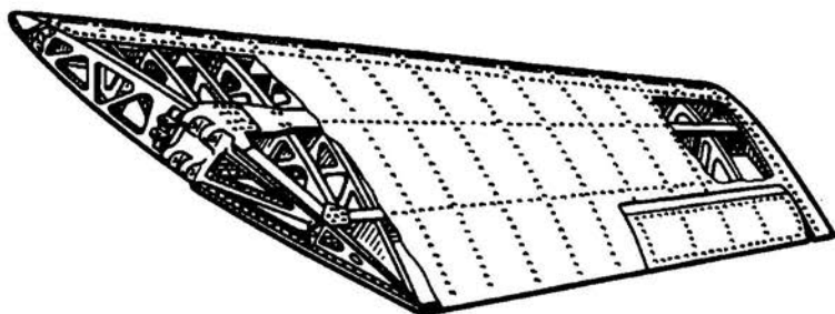
Рис. 3.7. Конструкция однолонжеронного стреловидного крыла
