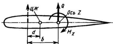
Рис. 2.23. К определению крутящего момента M_K
