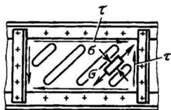
Рис. 2.44. Работа стенки лонжерона на сдвиг
