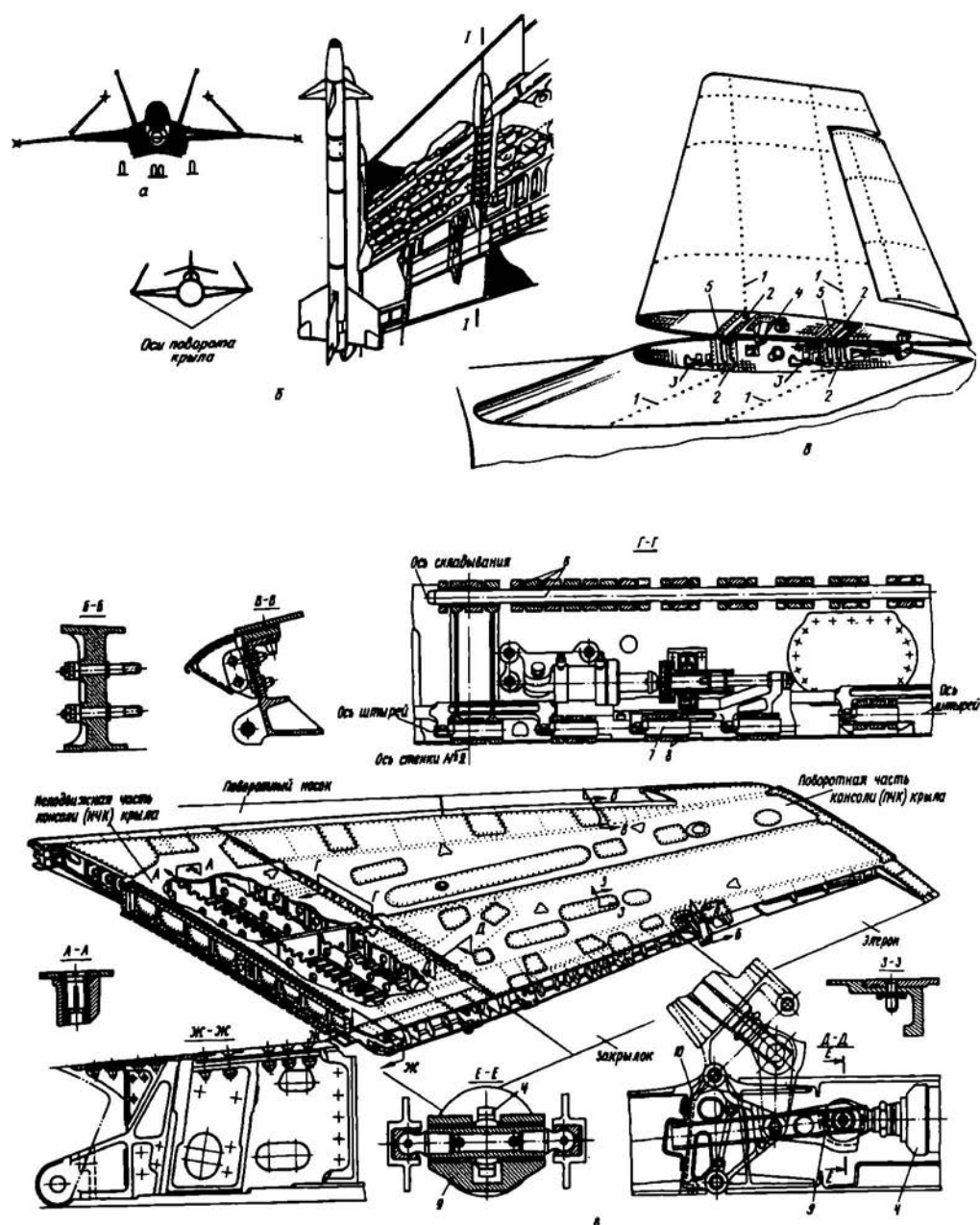
Рис. 3.28. Складывающиеся крылья
