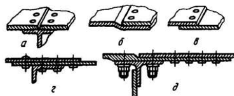
Рис. 6.9. Варианты соединений листовой обшивки
