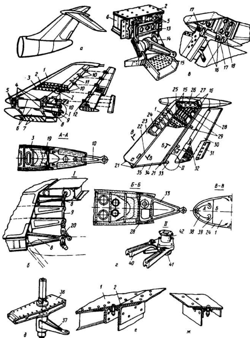
Рис. 5.10. Конструкция частей Т-образного оперения и узлов крепления киля к фюзеляжу, стабилизатора — к килю, рулей — к кронштейнам их навески
