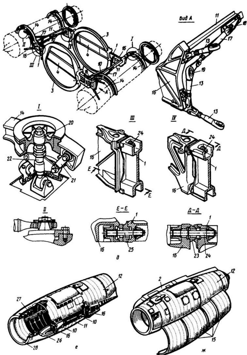
Рис. 9.5. Конструкция узлов крепления двигателей на пилонах в хвостовой части фюзеляжа. Конструкция гондол
