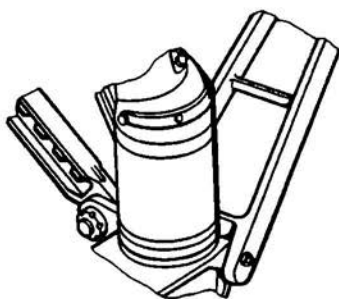
Рис. 7.28. Подкос с моментным узлом крепления к стойке
