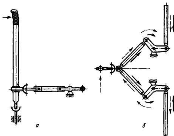
Рис. 8.19. Схема управления элевонами
