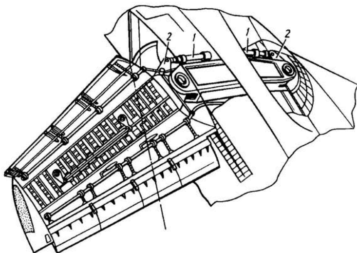
Рис. 3.22. Крыло изменяемой стреловидности самолета F-14
