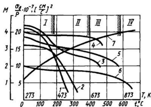
Рис. 1.11. Зависимости удельной прочности различных материалов \sigma_v/\rho от температуры T (в кельвинах) (кривые 1...6) и температуры T от числа M (кривая 7)
