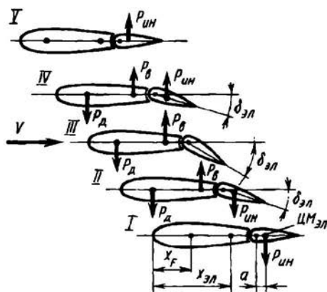
Рис. 10.4. К пояснению явления возникновения изгибно-элеронного флаттера
