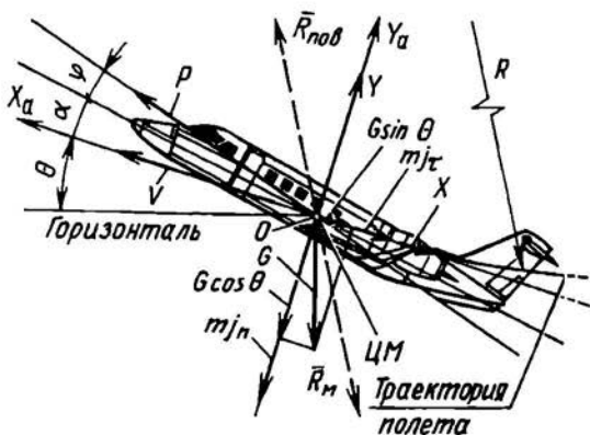
Рис. 1.13. Силы, действующие на самолет в криволинейном полете в вертикальной плоскости
