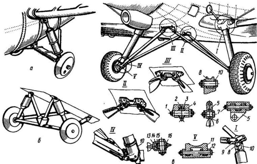
Рис. 7.25. Варианты конструкции ферменного шасси
