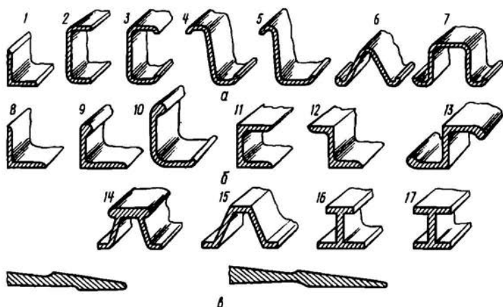
Рис. 2.38. Типовые профили стрингеров
