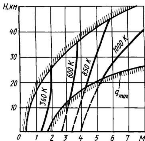
Рис. 1.21. Ограничения диапазона скоростей и высот полета
