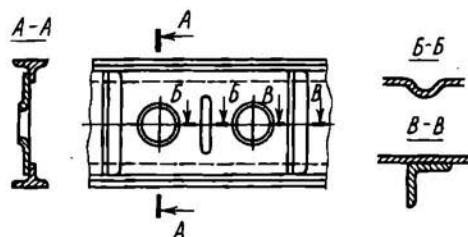
Рис. 2.45. Конструкция стенки лонжерона
