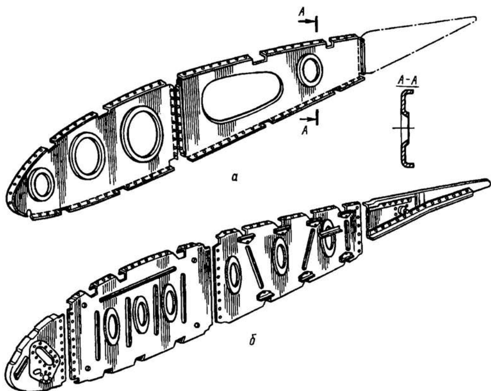
Рис. 2.47. Варианты конструкции нервюры
