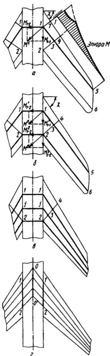
Рис. 3.1. Стреловидные крылья с переломом осей продольных силовых элементов у борта фюзеляжа и в плоскости симметрии самолета
