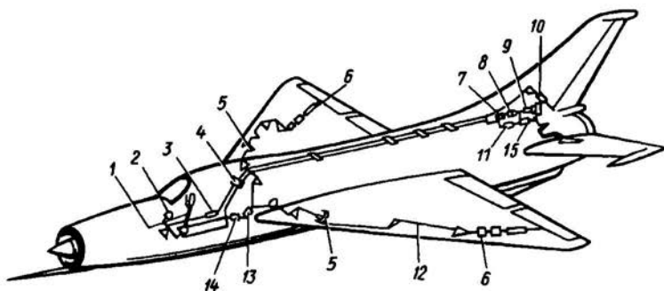
Рис. 8.20. Схема управления сверхзвуковым самолетом
