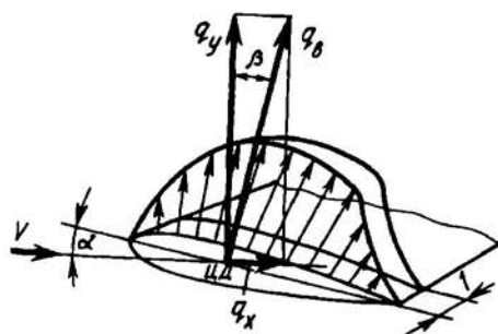
Рис. 2.15. Распределение по хорде воздушной нагрузки
