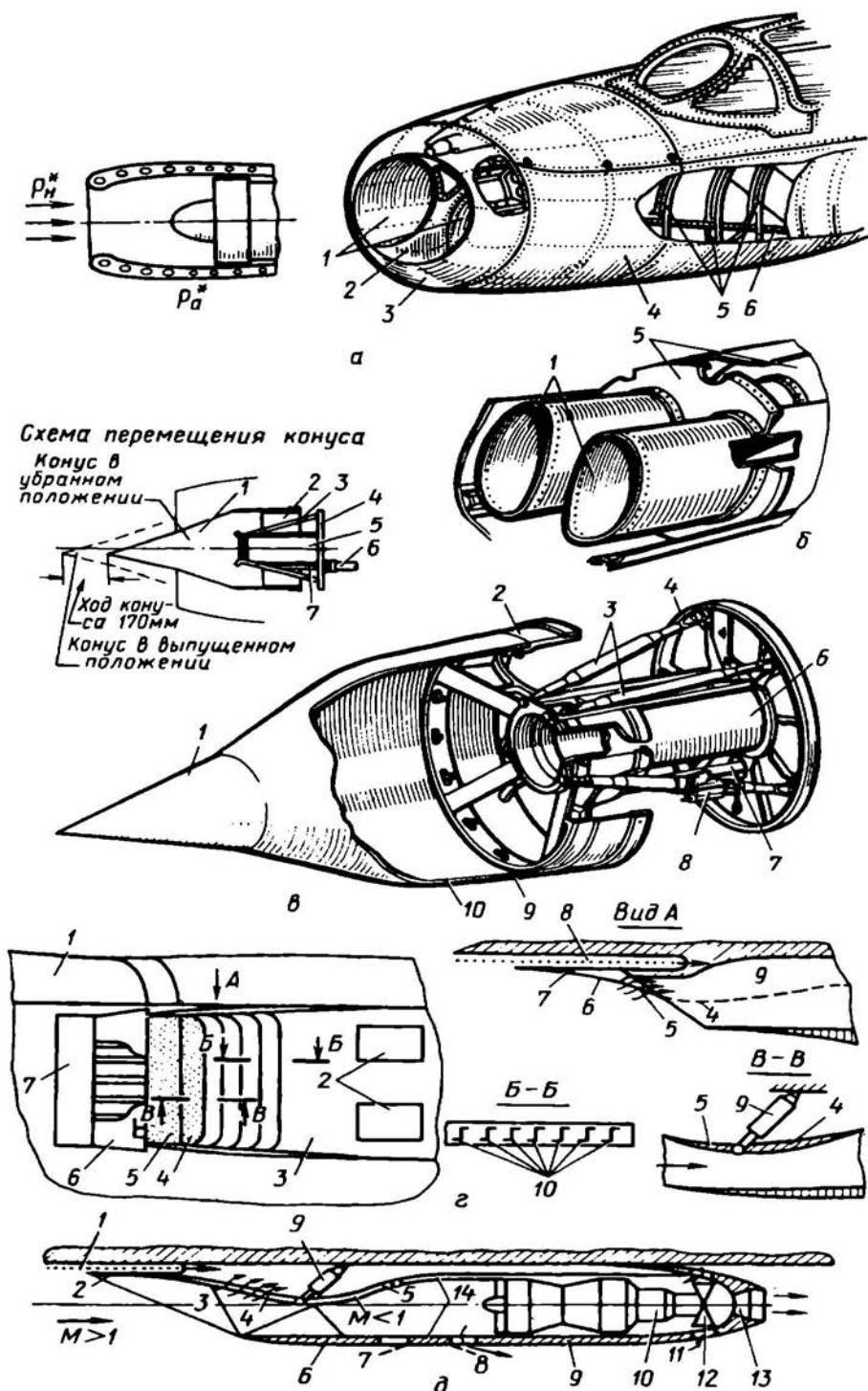
Рис. 9.9. Схемы и конструкция воздухозаборников различных типов
