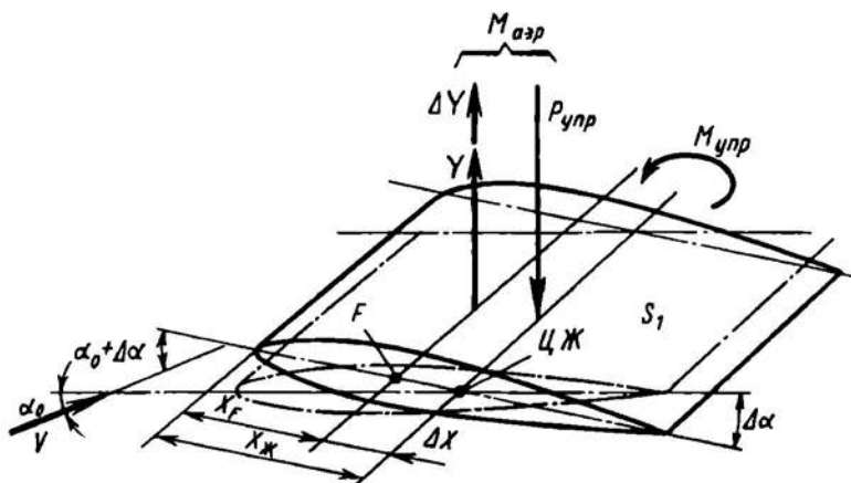
Рис. 10.2. К пояснению явления потери статической устойчивости крыла (дивергенции)
