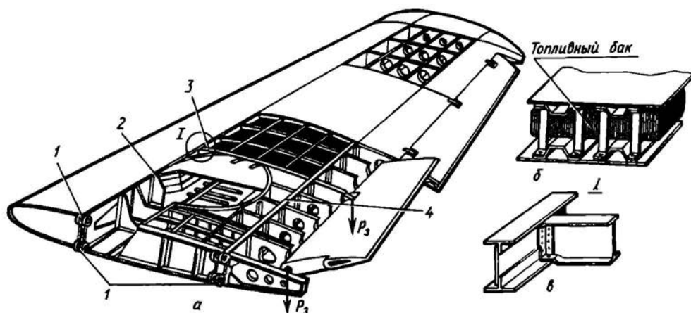
Рис. 2.53. Конструкция двухлонжеронного прямого крыла
