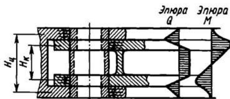
Рис. 3.27. Схема нагружения ГШ крыла изменяемой стреловидности
