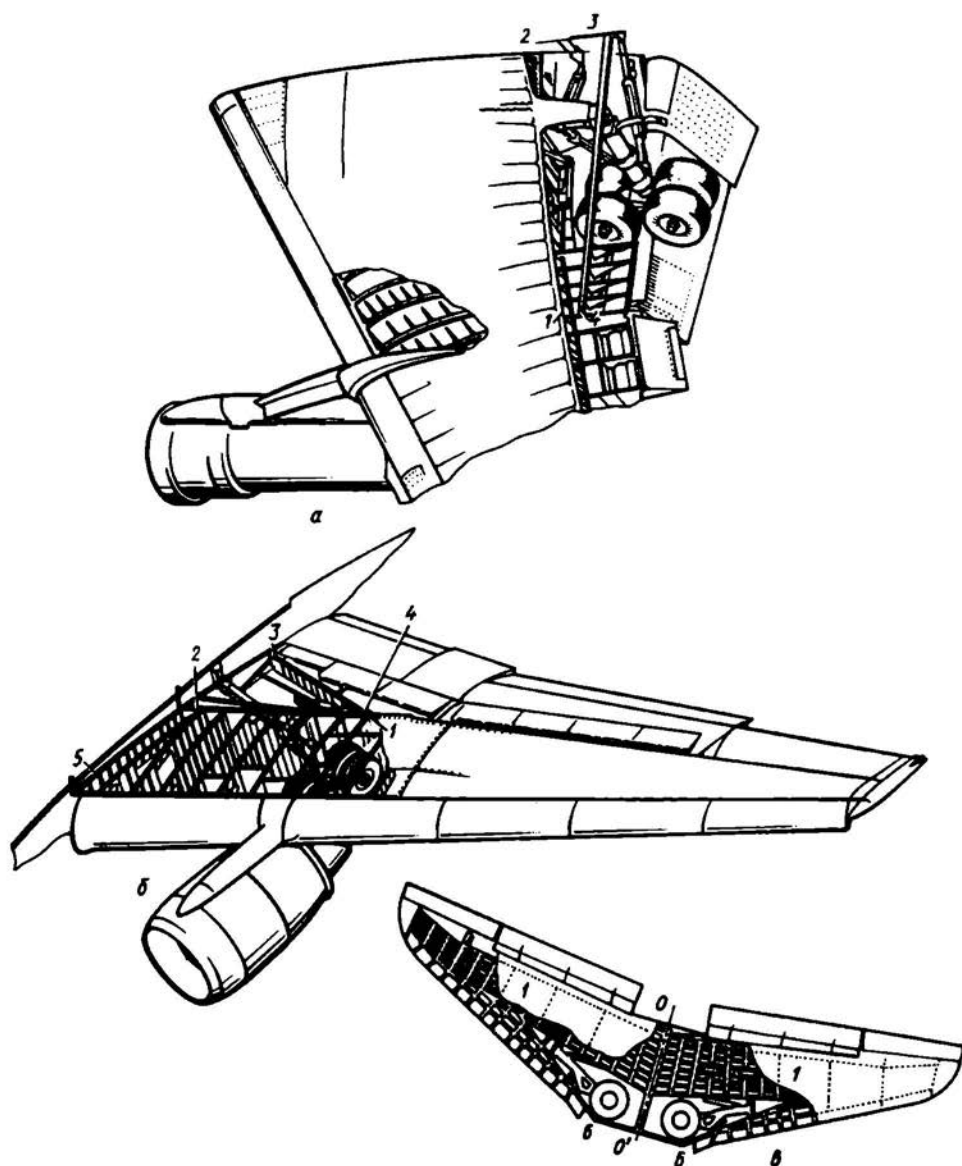
Рис. 3.13. Конструкция кессонных стреловидных крыльев с внешней балкой, лежащей в плоскости крыла
