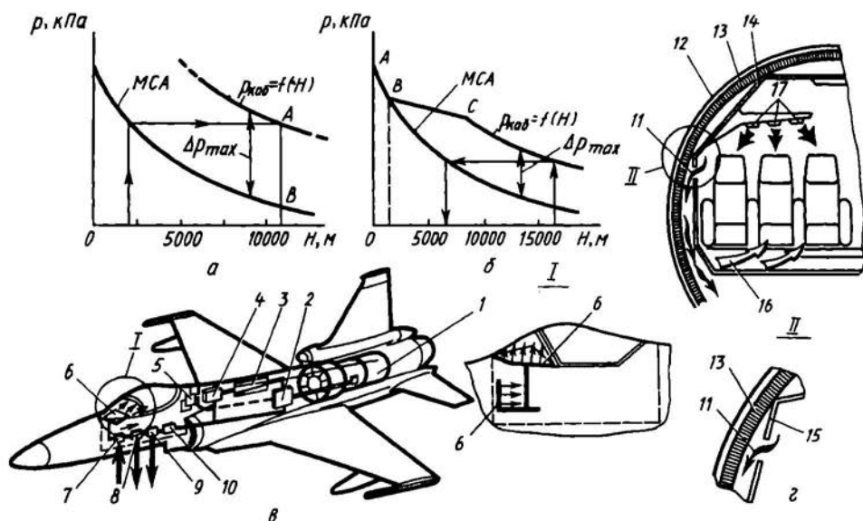
Рис. 6.33. Схема системы жизнеобеспечения и графики изменений давления в кабине по высоте полета
