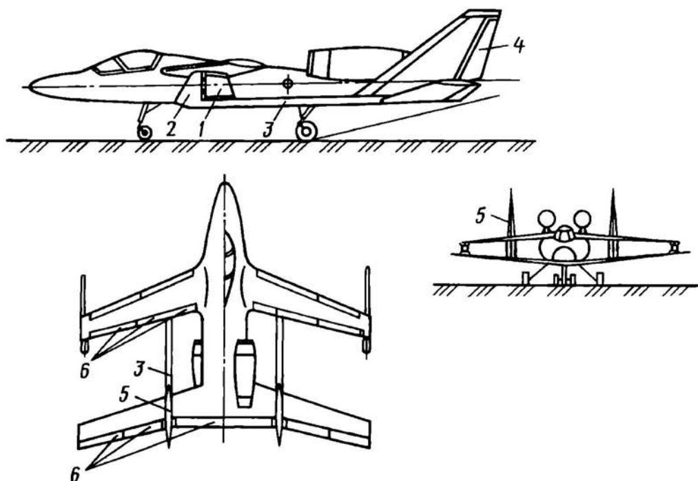
Рис. 3.38. Общий вид самолета
