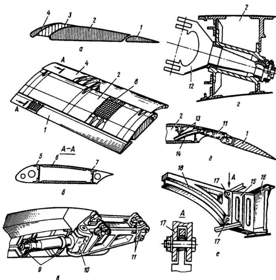
Рис. 4.7. Конструкция трехщелевого закрылки и его элементов
