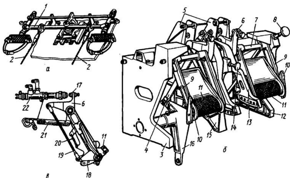
Рис. 8.7. Конструкция постов ножного управления с педалями на параллелограммном механизме и с качающимися педалями
