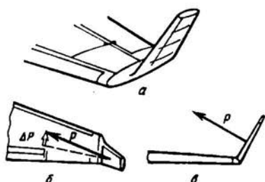
Рис. 2.69. К вопросу применения на крыле концевых крылышек
