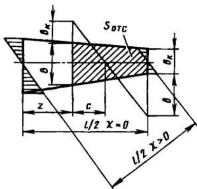
Рис. 2.21. К определению приближенных значений Q и M в сечениях спрямленного стреловидного крыла
