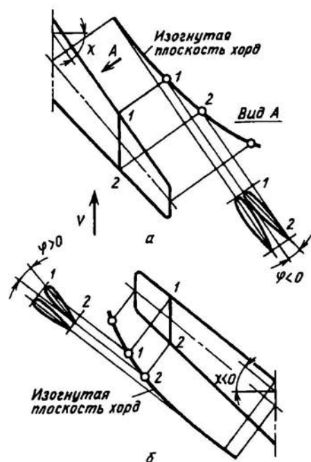
Рис. 2.10. Изменение угла атаки сечений крыла прямой (а) и обратной (б) стреловидности при изгибе крыла
