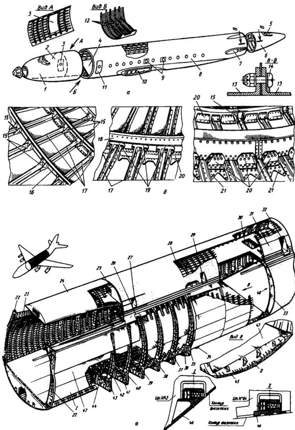
Рис. 6.7. Конструкции фюзеляжа пассажирского самолета, соединений обшивки, шпангоутов и стрингеров между собой
