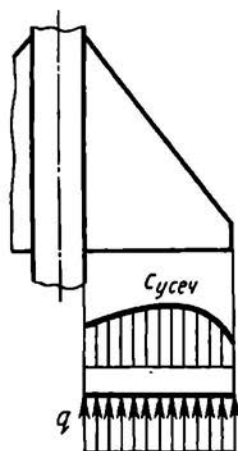
Рис. 3.30. Схема распределения воздушной нагрузки по треугольному крылу
