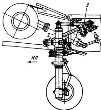
Рис. 7.36. Конструкция передней опоры с винтовым подъемником
