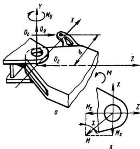
Рис. 3.25. Силы и моменты, действующие на главный шарнир
