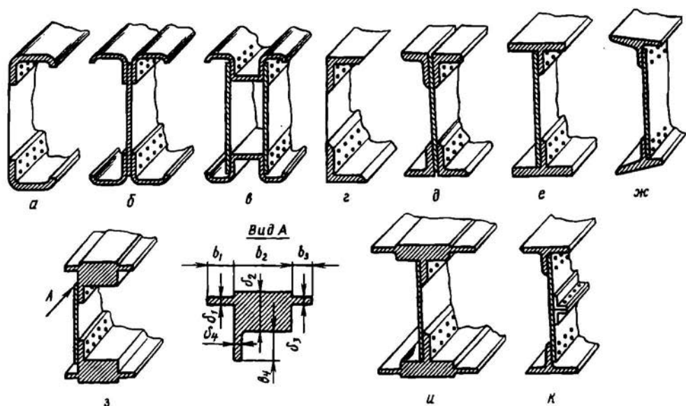
Рис. 2.41. Сечения лонжеронов
