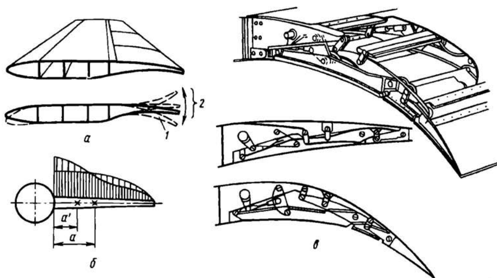
Рис. 4.16. Адаптивное крыло и элементы его конструкции
