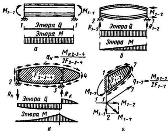
Рис. 3.6. Схемы нагружений:
