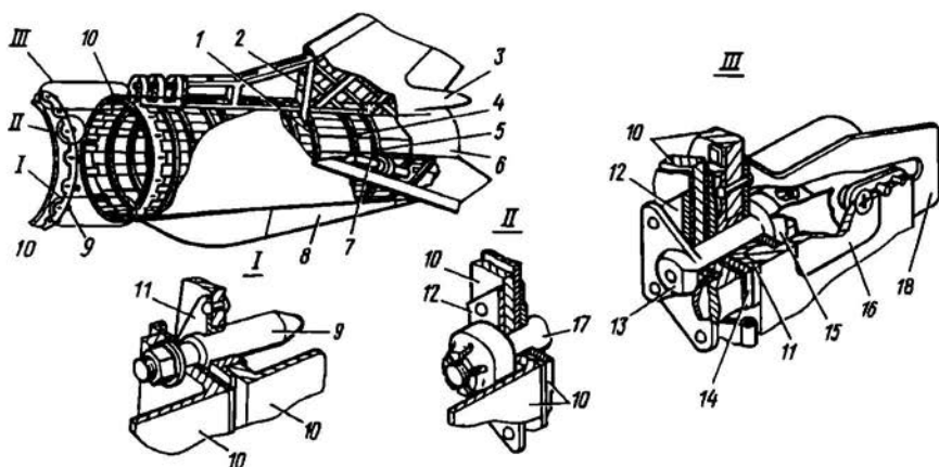
Рис. 6.8. Конструкция стыкового соединения хвостовой и носовой частей фюзеляжа
