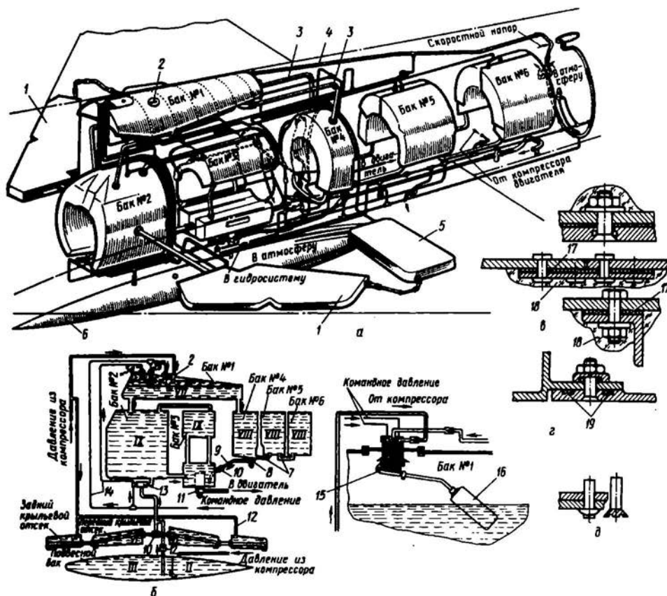
Рис. 9.11. Топливная система самолета. Схема выработки топлива. Способы герметизации топливных отсеков в крыле и фюзеляже
