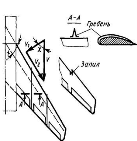
Рис. 2.8. Стреловидное крыло
