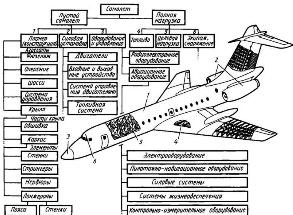
Рис. 1.1. Структурная схема самолета
