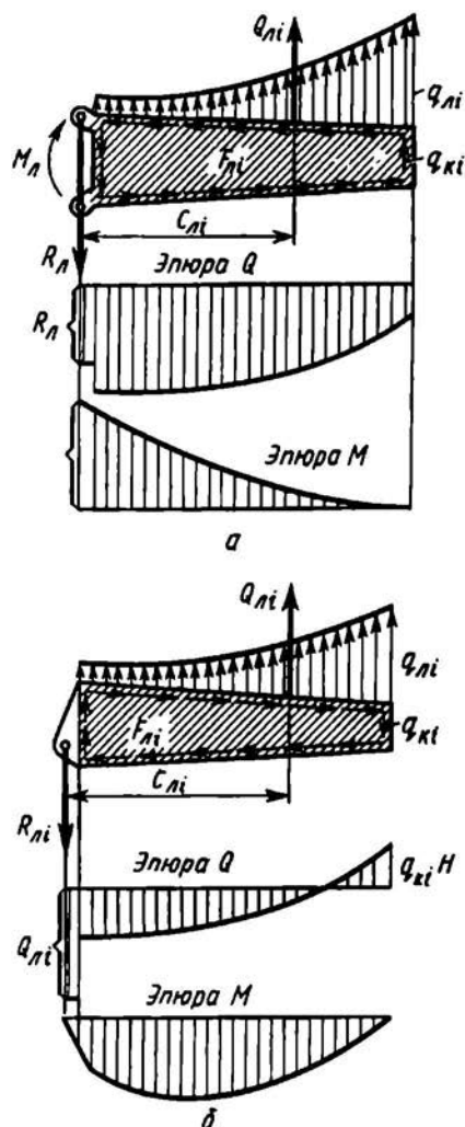
Рис. 3.33. Схема нагружения основных и вспомогательных лонжеронов треугольного крыла
