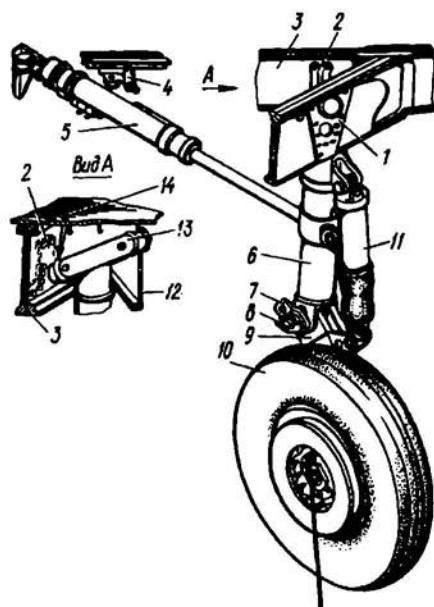
Рис. 7.32. Конструкция основной опоры балочной КСС с подкосом и рычажной подвеской колеса
