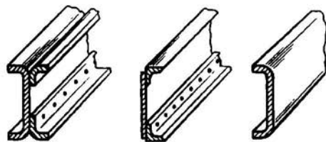
Рис. 2.46. Варианты конструкции стенок
