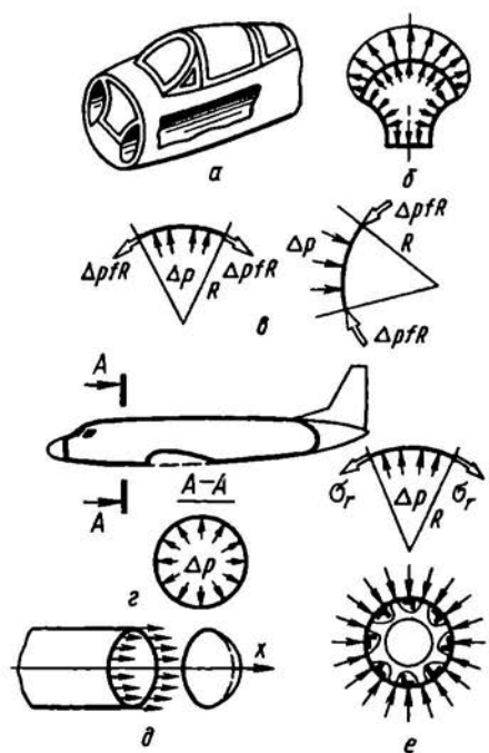
Рис. 6.22. Герметические кабины самолетов. Схема нагружения элементов герметической кабины избыточным давлением
