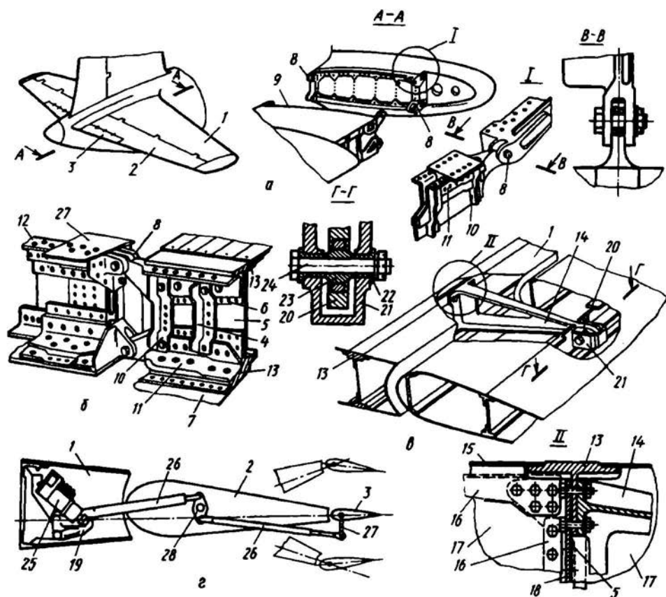
Рис. 5.6. Конструкция ГО и узлов его крепления к фюзеляжу. Узел навески руля высоты
