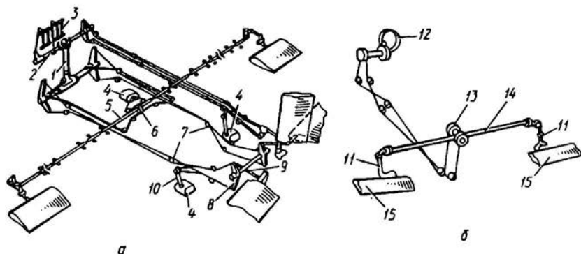
Рис. 8.15. Схема системы управления дозвуковым самолетом
