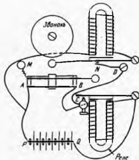
Рис. 48. Грозоотметчик Попова
