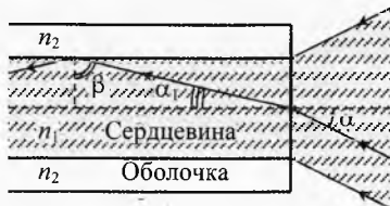
Рис. 61. Оптическое волокно
