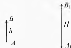
Рис. 19. Восстановить положение зеркала
