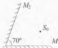
Рис. 32. Сколько будет изображений?
