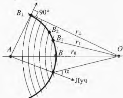
Рис. 33. Зоны Френеля
