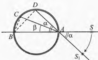
Рис. 9. Показатель преломления жидкости
