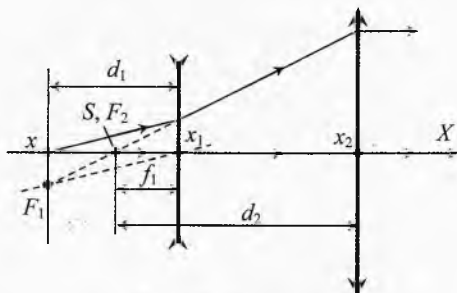
Рис. 60. Система линз
