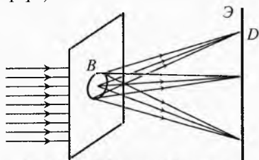
Рис. 37. Дифракция Френеля
