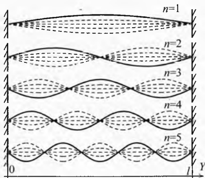
Рис. 13. Стоячая волна
