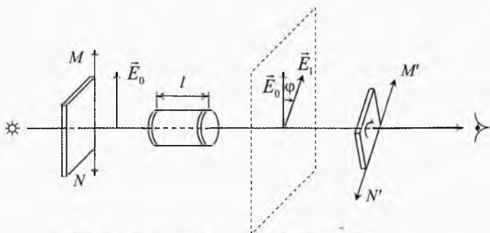
Рис. 24. Вращение плоскости поляризации
