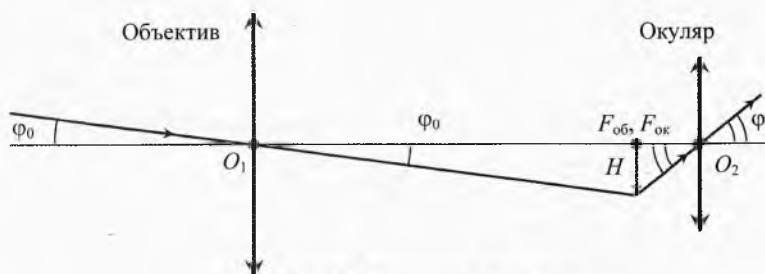
Рис. 59. Телескоп рефрактор
