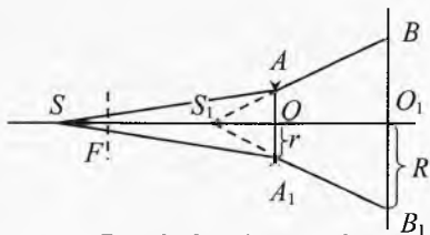
Рис. 8. Определение фокуса рассеивающей линзы
