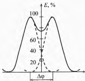
Рис. 40. Критерий Рэлея
