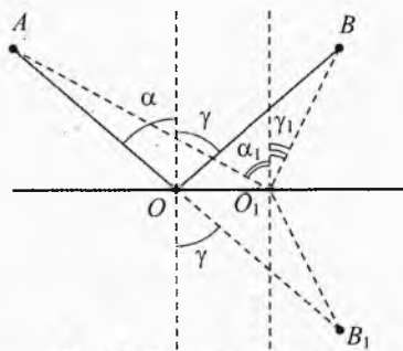
Рис. 3. Отражение света
