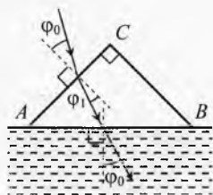
Рис. 21. Призма на воде
