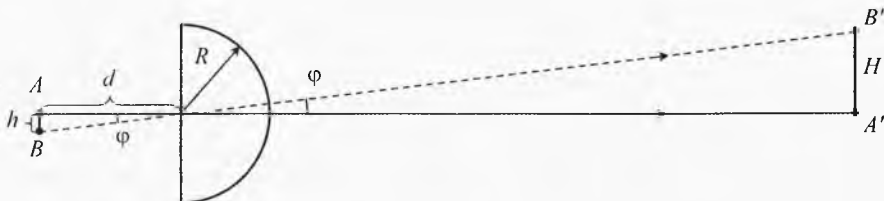
Рис. 42. Разрешающая способность микроскопа
