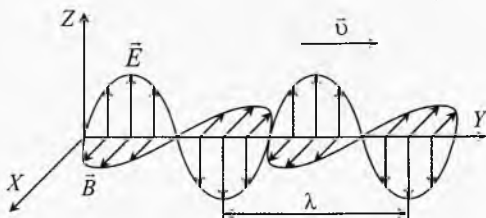
Рис. 46. Электромагнитная волна
