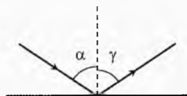
Рис. 1. Закон отражения
