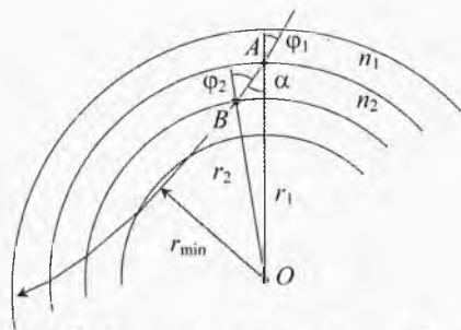
Рис. 42. Преломление луча на слоях сферы
