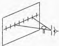
Рис. 14. Отношение диаметров шляпки и иглы
