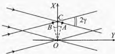
Рис. 37. Интерференция пучков
