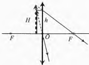
Рис. 41. При приближении к линзе увеличение устремится к единице
