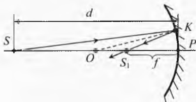
Рис. 12. Вывод формулы сферического зеркала
