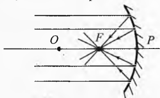
Рис. 10. Вогнутое зеркало
