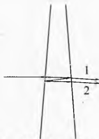
Рис. 55. Интерференция на мыльном клине
