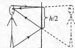
Рис. 7. Размер зеркала
