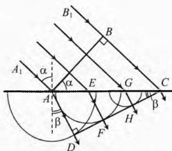
Рис. 16. Преломление волны
