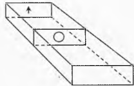
Рис. 38. Линза в аквариуме
