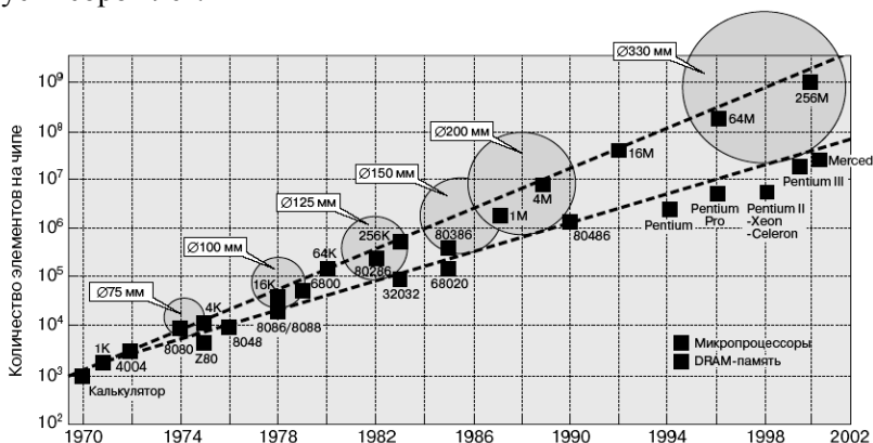
Рис. В.1. Закон Мура для микропроцессоров и запоминающих устройств (кругами обозначены диаметры кремниевых пластин)
