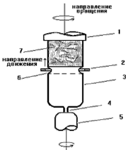
Рис. 7.8. Метод вертикальной зонной плавки [15]: 1 – держатель; 2 – обмотка нагревателя; 3 – монокристаллический кремний; 4 – затравочный монокристалл; 5 – держатель; 6 – расплавленная зона; 7 – стержень из поликристаллического кремния
