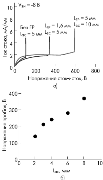
Рис. 3.13. Результаты применения метода FP для увеличения пробивного напряжения затвор/сток: BAX AlGaIn/GaN ГПТШ и ГПТШ с полевым электродом (а); зависимость пробивного напряжения транзистора от расстояния затвор/сток (б)
