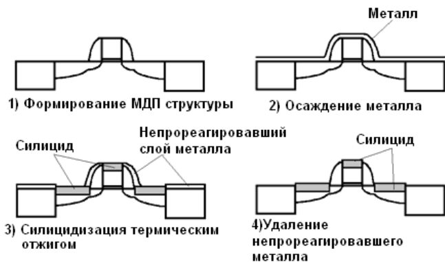
Рис. 7.16. Последовательность операций “Salicide”
