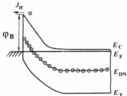
Рис. 2.8. Зонная структура выпрямляющего контакта металл–полупроводник: J_n – ток основных носителей заряда; \Phi_B – высота потенциального барьера металл–полупроводник; E_C – энергия дна зоны проводимости; E_F – энергия уровня Ферми; E_{DN} – энергия глубоких уровней; E_V – энергия потолка валентной зоны
