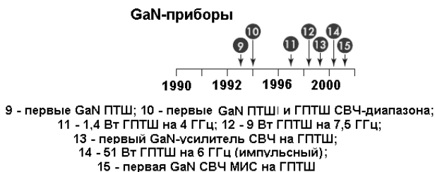
Рис. 3.20. Хронология разработок GaAs- и GaN-транзисторов и микросхем
