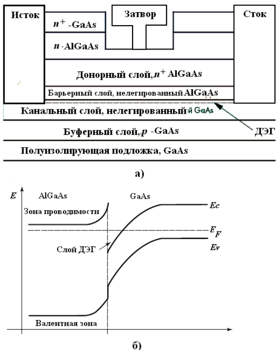
Рис 3.1. Типичная структура GaAs ГПТШ (а) и его зонная диаграмма вблизи области ДЭГ(б)
