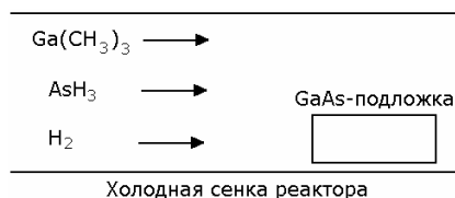
Рис. 2.3. Схематическое представление процесса ГФЭ с использованием МО
