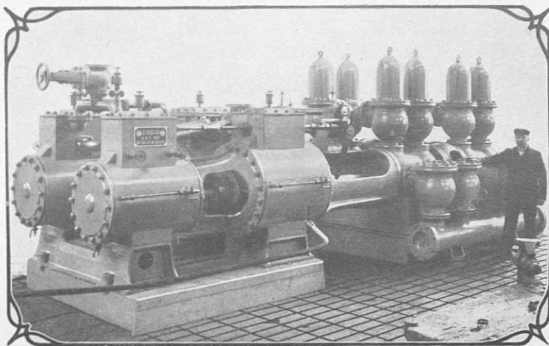
Большой насосъ, установленный въ Баку для подачи 18.000 ведеръ въ часъ.
