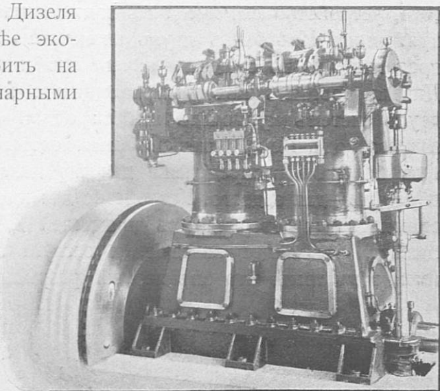
Быстроходный двигатель Дизеля въ 70 д. л. с.
