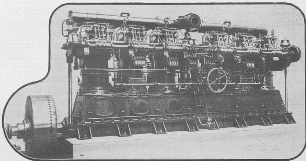
Двигатель канонерокъ „Карсъ“ и „Ардаганъ“. 6-цилиндровый, 500 д. л. с.
