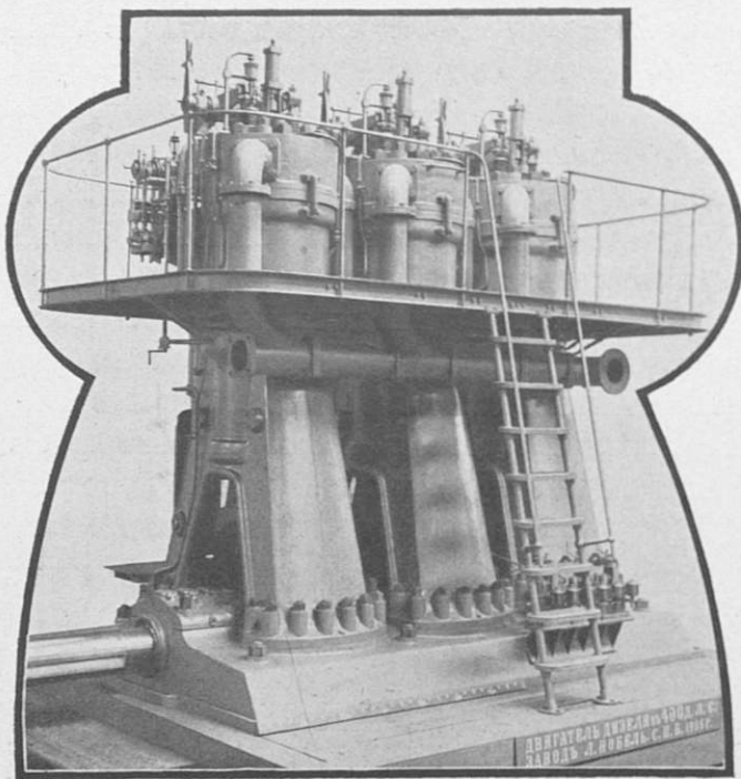
Двигатель Дизеля въ 400 д. л. с., модель 1906 г.
