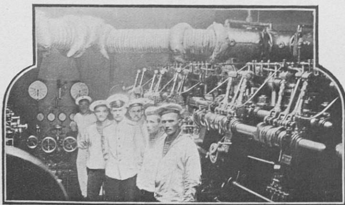
Машинное помѣщеніе „Ардагана“. (2 двигателя по 500 д. л. с. и 2—по 80 д. л. с.).
