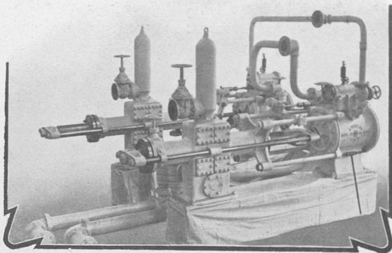
Насосъ по американской системѣ Вортингтона.
