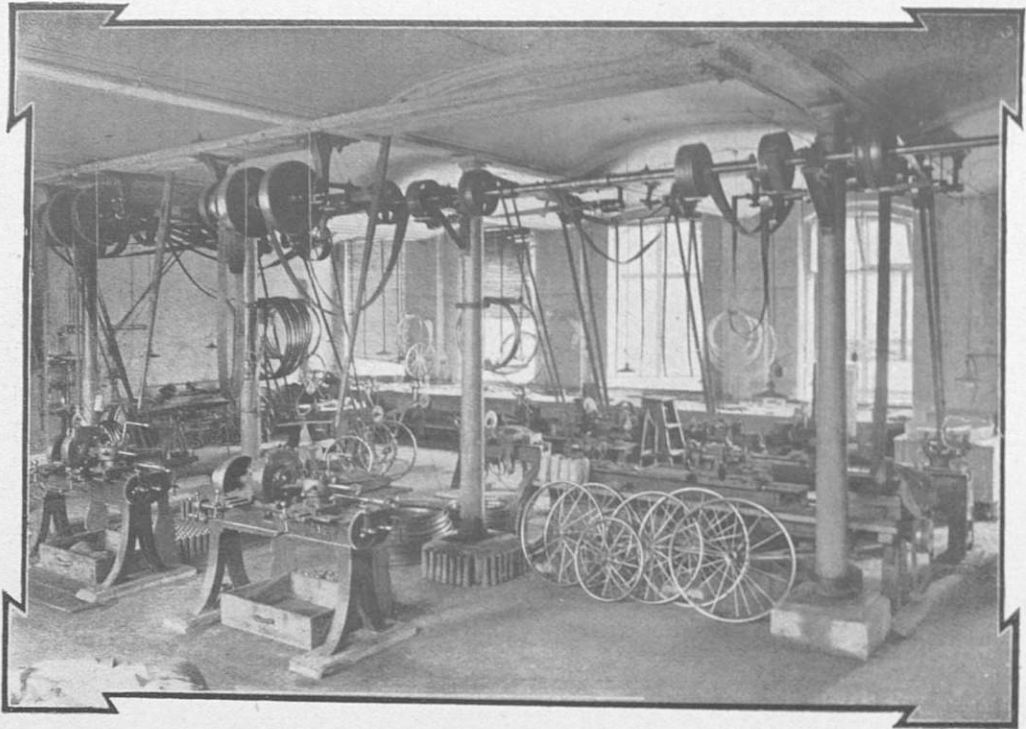
Изготовленіе металлическихъ колесъ.
