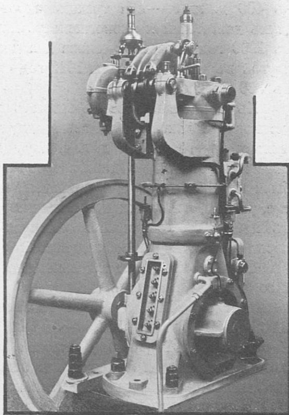
Опытный двухтактный двигатель въ 20 д. л. с. 1903 г.
