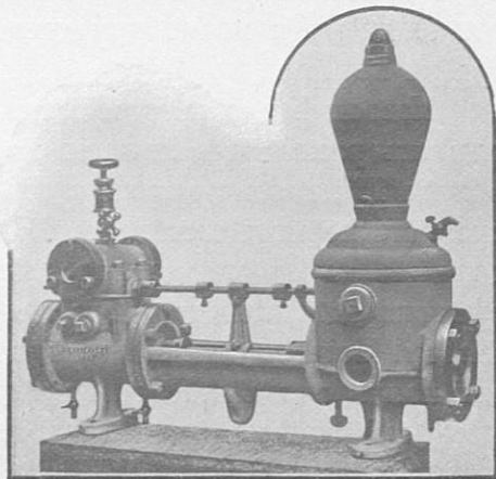
Образецъ насоса Блэка.
