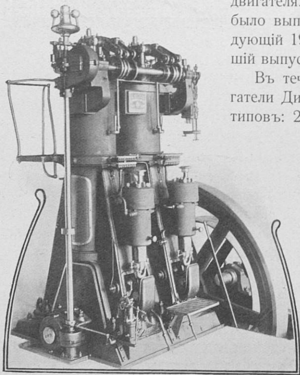
Двухцилиндровый двигатель въ 60 д. л. с. высокаго типа А съ крейцкопфомъ.
