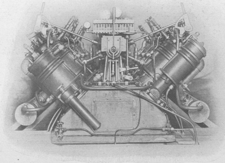
Опытный 8-цилиндровый двигатель Дизеля V-образной формы. (Видъ спереди).
