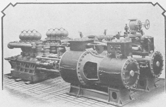
Насосъ-дуплексъ образца Ворthingтона.
