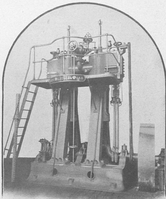
— Вертикальная паровая машина типа Компаундъ 1882 г.
