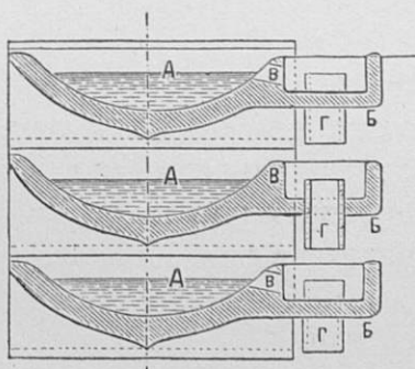
Колосники для обжиганія нефти - Л. Э. Нобеля.
