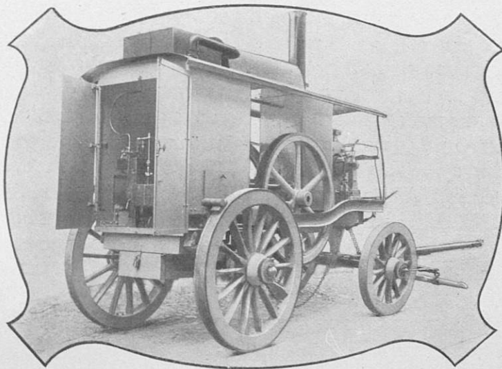
Генераторная повозка образца 1895 г.
