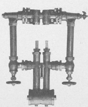
Форсунка Нобеля.
