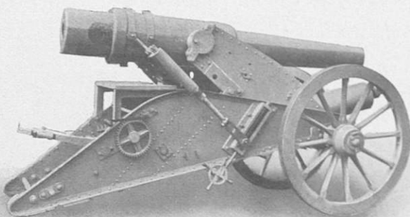
Лафетъ подь 6" пушку и пушка.
