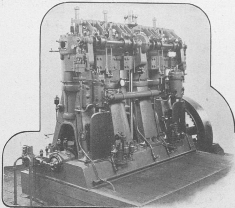
Двигатель судна „Сармат“: 4 цилиндра, 180 д. л. с.
