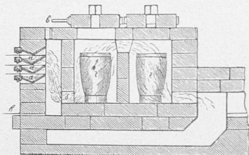
Желѣзоплавильная печь Л. Э. Нобеля.
