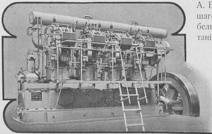
Быстроходный двигатель Дизеля въ 300 д. л. с.
