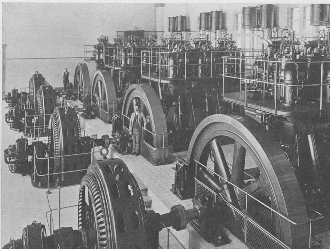
Городская электрическая станція г. Астрахани въ 1911 году. (4 двигателя по 300 л. с.).
