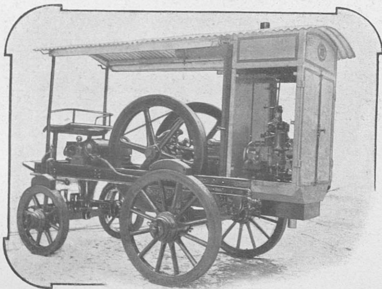
Генераторная повозка образца 1894 г.
