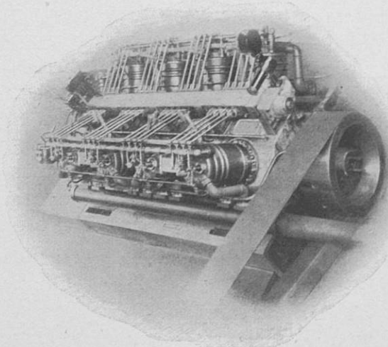
Опытный 8-цилиндровый двигатель Дизеля V-образной формы. (Видъ сверху).
