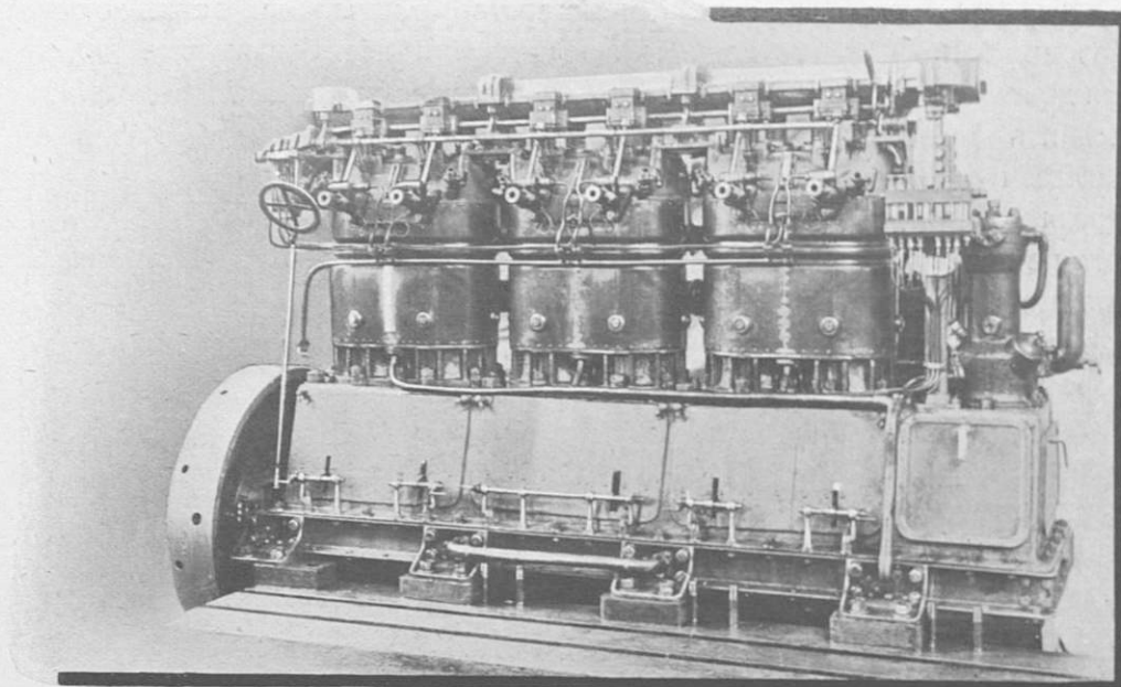
Двигатель въ 160 д. л. с. для подводных лодокъ типа „Стерлядь“.
