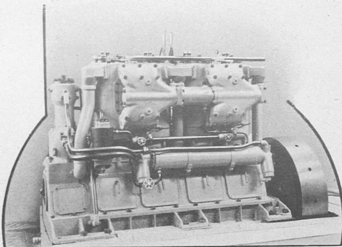
Двигатель для подводной лодки типа „Касатка“. (Видъ сзади).
