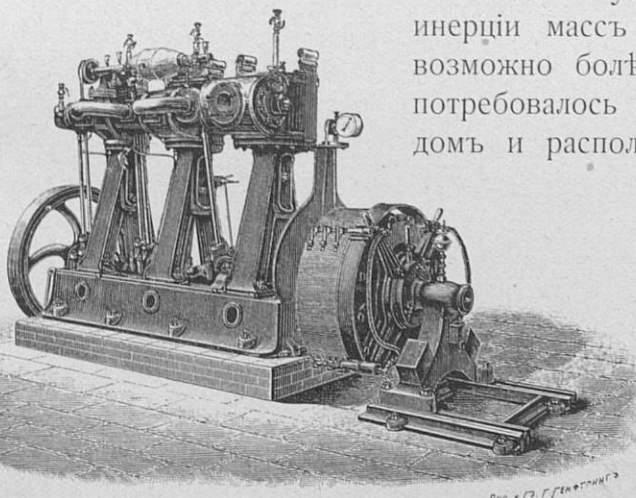
Паровая машина тройного расширенія.
