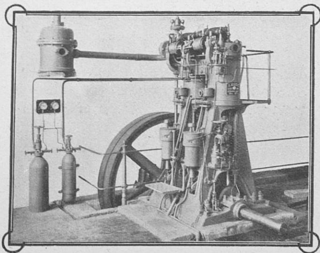
Двухцилиндровый двигатель высокаго типа мощности 40 д. л. с.
