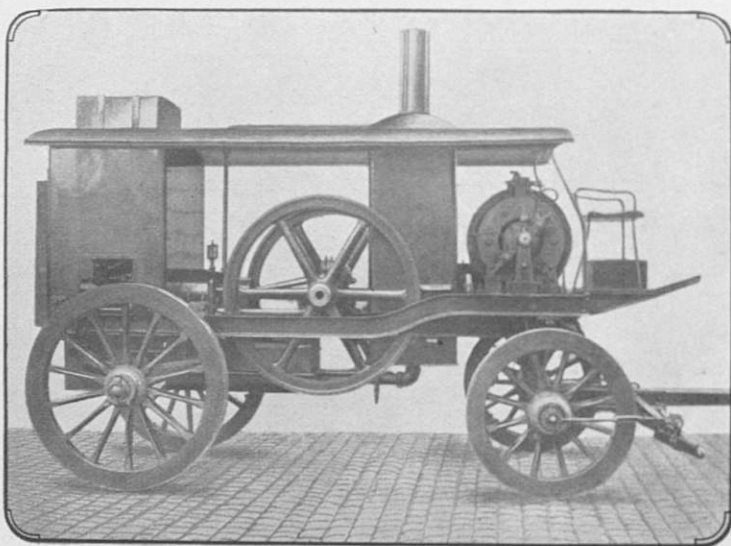
Генераторная повозка съ холодильникомъ.
