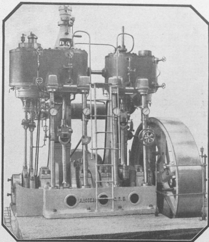
Паровая машина типа Компаундъ 1887 г.
