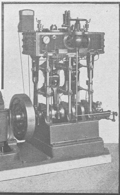
Пародинамо судового типа.
