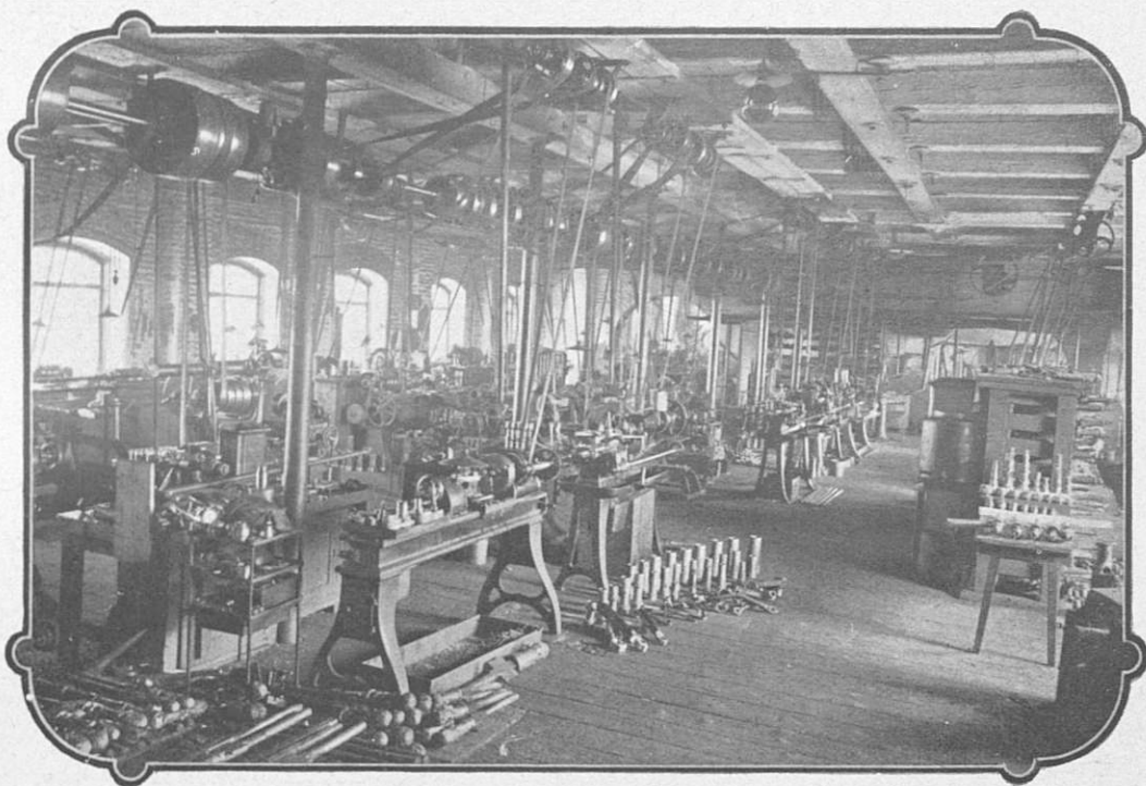
Осейная мастерская.
