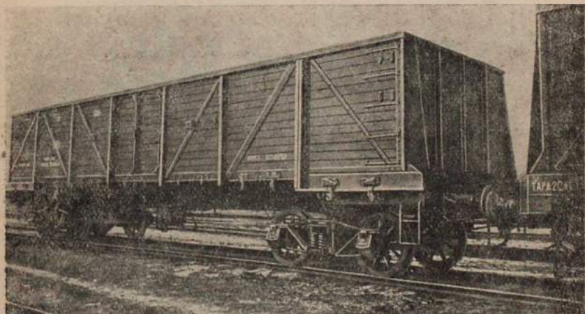
Саморазгружающийся полувагон-гондола
