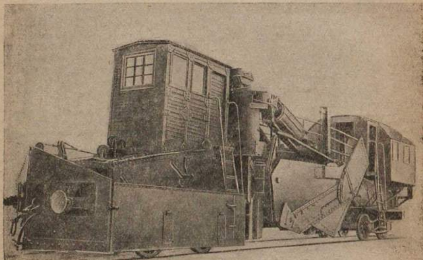
Путевой струг
