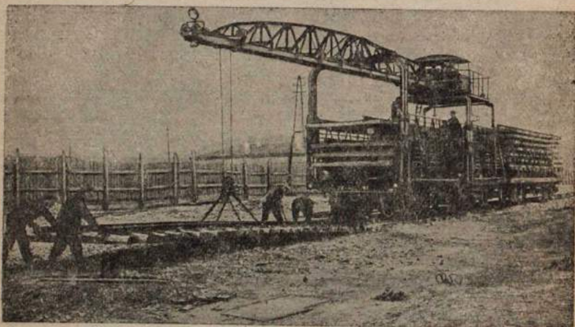
Путеукладчик Платова
