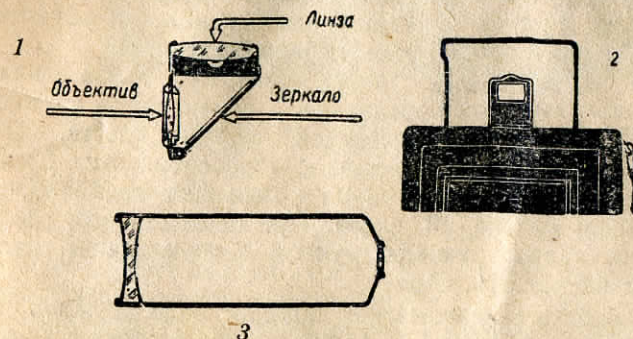
Рис. 11. Типы видоискателей: 1 — зеркальный видоискатель «Бриллиант», 2 — рамочный видоискатель-иконметр, 3 — видоискатель «Альбада»
