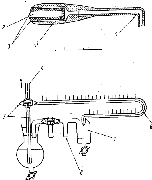
Рис. 151. Прибор Воннегата для определения водности облаков.
