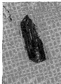
Рис. 103. Формы кристаллов в облаках Ns — As. а — 16 марта 1952 г., б — 18 марта 1952 г.
