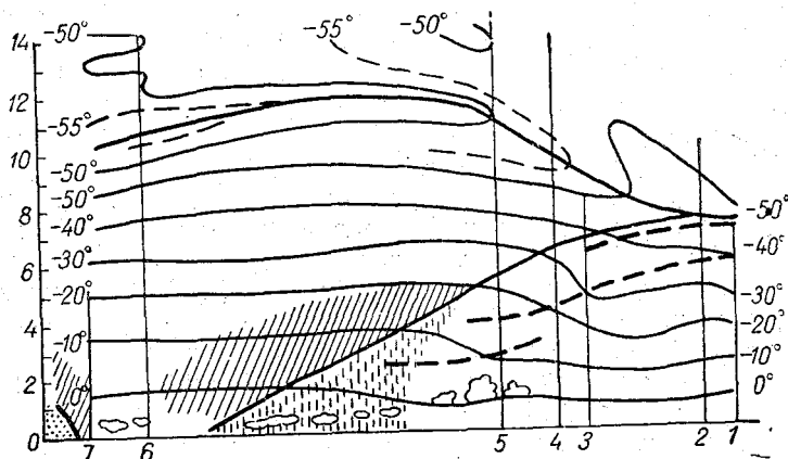
Рис. 87. Разрез через облачность теплого фронта (по Бьеркнесу).
