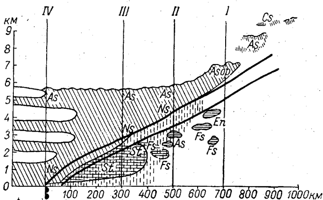
Рис. 90. Схема облачной системы теплового фронта.
