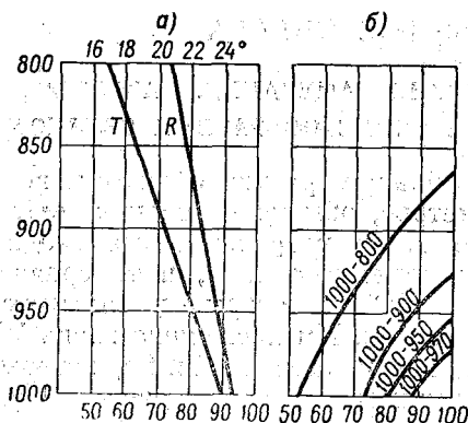
Рис. 74. Перераспределение влажности в слое воздуха при перемешивании.
