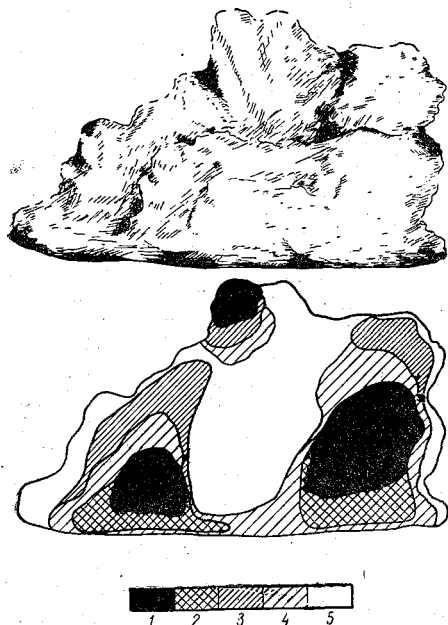
Рис. 63. Схема внутреннего строения Сисог. в квазистационарном состоянии. Концентрация капель: 1 — большая, 2 — средняя, 3 — малая, 4 — очень малая, 5 — капель нет.
