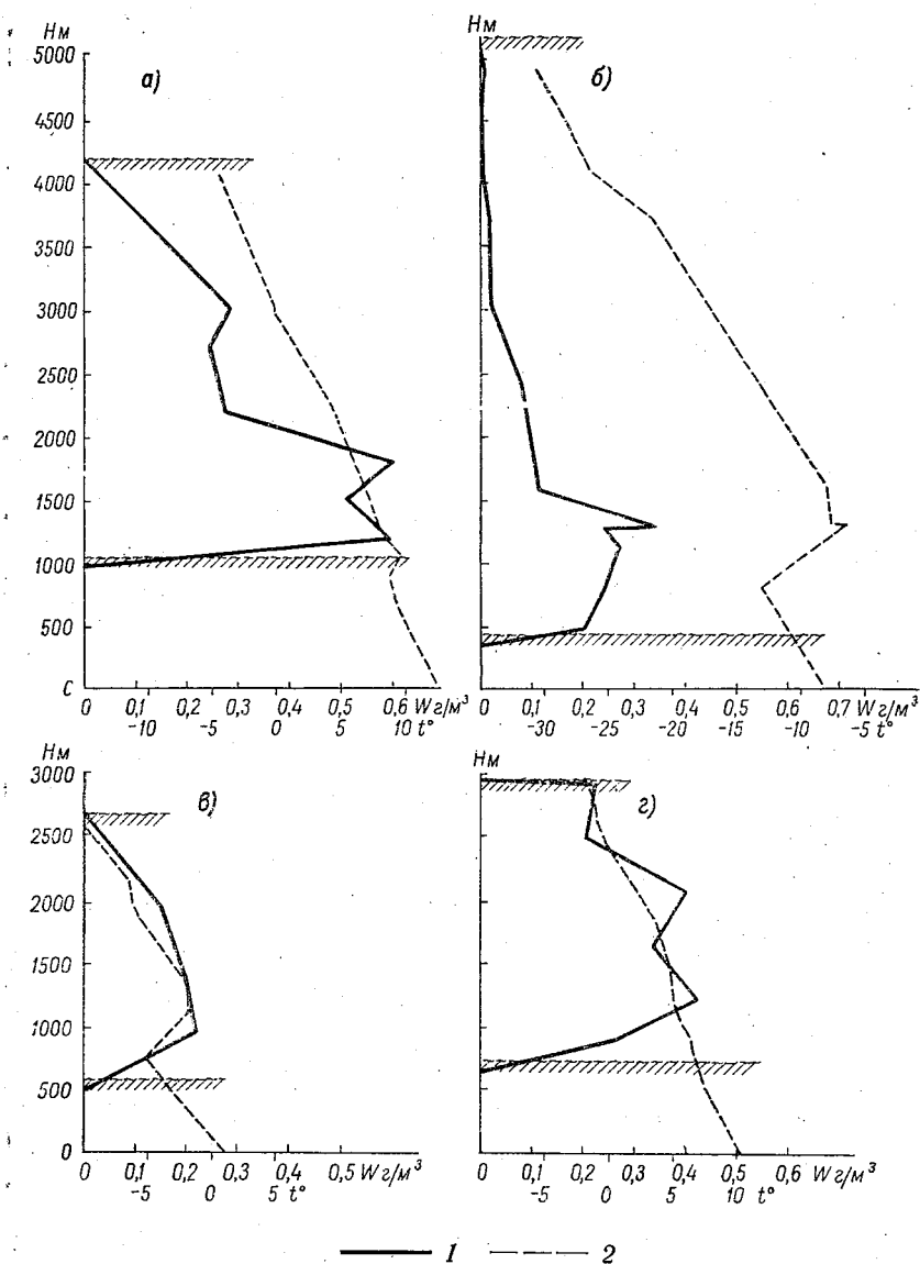
Рис. 37. Распределение водности в отдельных облаках Ns, Ns — As. 1 — водность, 2 — температура, а — Минск, 2/VI 1958 г. 16 ч. 54 м., б — Сыктывкар, 18/III 1951 г. 12 ч. 30 м., в — Архангельск, 27/III 1957 г. 17 ч. 21 м., г — Рига, 27/III 1957 г. 23 ч. 09 м.
