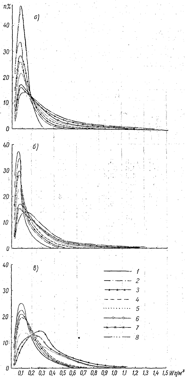
Рис. 33. Повторяемость средних значений водности в зависимости от температуры.
