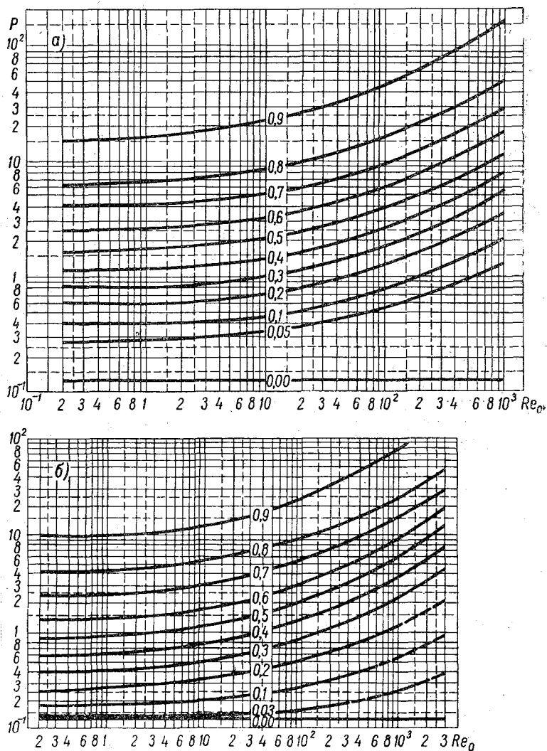
Рис. 121. Диаграмма зависимости коэффициента захвата для круглого цилиндра от параметров P и Re_0 . а — полный коэффициент захвата E , б — коэффициент захвата в критической точке E_* .
