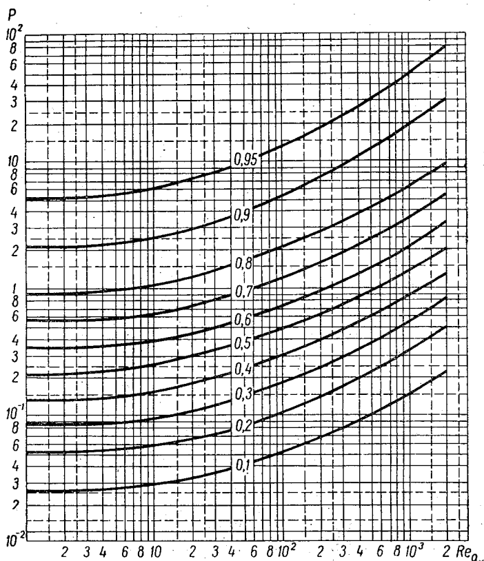
Рис. 122. Диаграмма зависимости полного коэффициента захвата \tilde{E} для крылевых профилей от параметров P и Re_0 .
