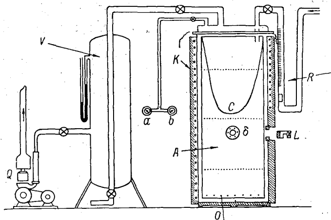
Рис. 7. Адиабатная камера Финдайзена — Шульца.
