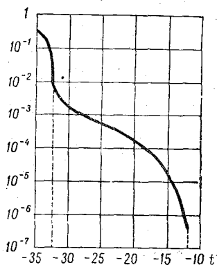
Рис. 8. Спектр концентрации ядер сублимации (по Финдайзену).
