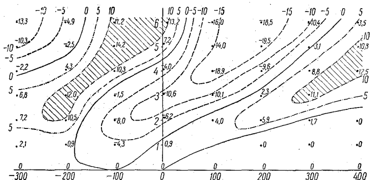
Рис. 88. Поле вертикальных скоростей в области теплого фронта (по А. Ф. Дзюбюку).
