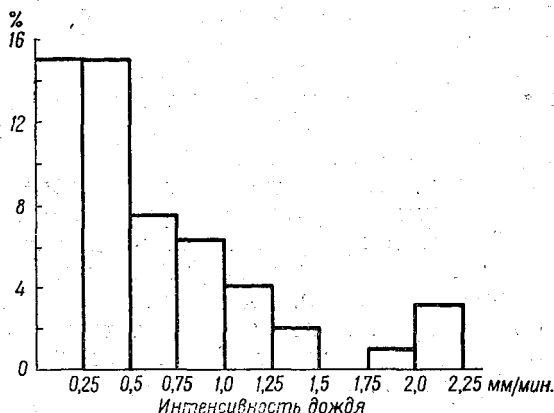
Рис. 73. Интенсивность ливневых дождей из 53 ячеек грозowych облаков (по наблюдениям Брейама).
