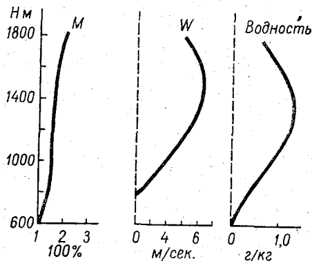
Рис. 69. Вовлечение в облако: вертикальный поток массы M , вертикальная скорость в облаках w и водность в функции высоты над основанием облака.
