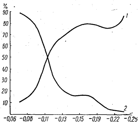
Рис. 14. Повторяемость пластинчатых (1) и столбчатых (2) форм кристаллов в функции дефицита влажности на поверхности кристаллов ( \Delta E ) по данным Е. Г. Зак и А. Д. Малкиной.
