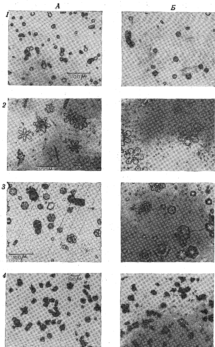
Рис. 13. Формы кристаллов (по Вейкману и по работам ЦАО).
