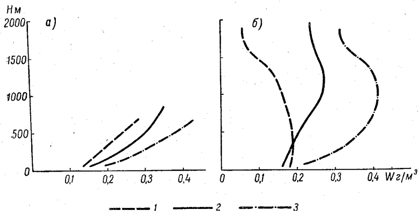
Рис. 36. Средняя водность облаков в зависимости от высоты над нижней границей: а — Sc, St, Ac; б — Ns, As, Ns — As.
