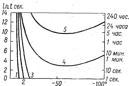
Рис. 18. Скорость полного замораживания монодисперсного аэрозоля (по Л. Г. Качурину).
