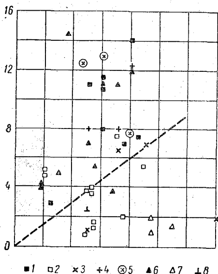
Рис. 141. Вероятность выпадения осадков из мощных кучевых облаков, засеянных сухим льдом, в зависимости от мощности облака (ось ординат) и высоты основания над землей (ось абсцисс), в тысячах футов.
