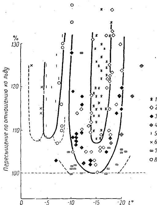
Рис. 11. Зависимость форм кристаллов от температуры (по Накай).
