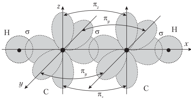
Рис. 5.20. Перекрывание орбиталей в молекуле ацетилена
