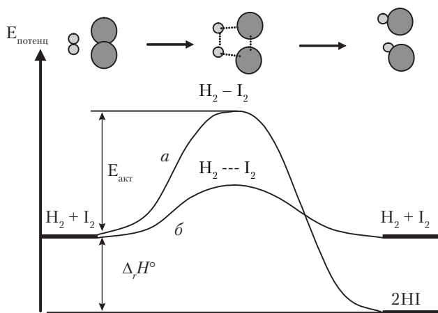
Рис. 6.5. Превращение молекул в результате столкновений:
