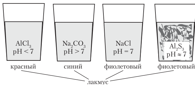
Рис. 7.2. pH растворов некоторых солей (схема к опыту 7.1)
