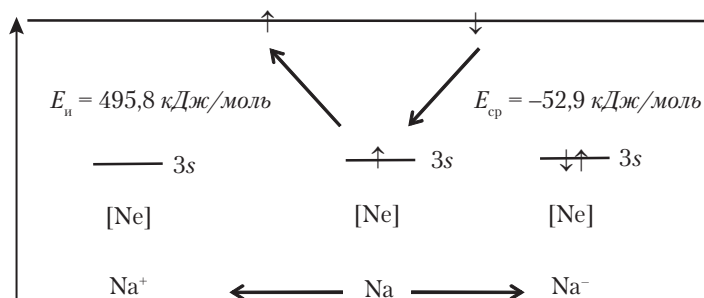
Рис. 5.11. Ионизация атома натрия
