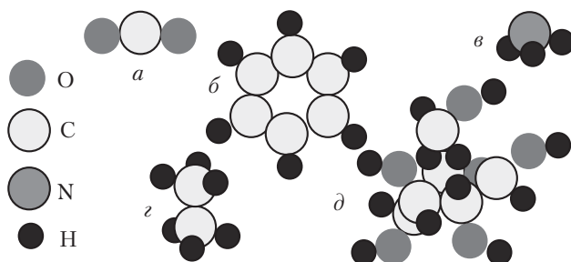
Рис. 1.9. Модели некоторых молекул:
