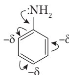
+M-эффект заместителя
