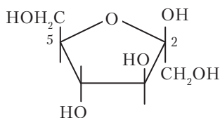
\beta -D-фруктоза
