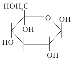
\beta -D-глюкоза
