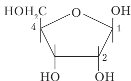
\beta -D-рибоза
