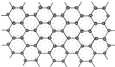
Рис. 13.1. Строение плоского слоя в структуре графита
