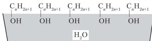
Рис. 16.1. Концентрирование поверхностно-активного вещества на поверхности
