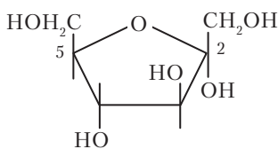
\alpha -D-фруктоза
