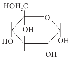
\alpha -D-глюкоза
