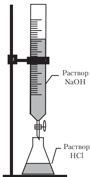
Рис. 3.1. Титрование кислоты щелочью
