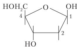
\beta -D-дезоксирибоза
