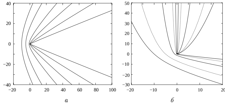
Рис. 6. Поляризационные кривые около особых точек “метеор” (a) и “соха” (б).
