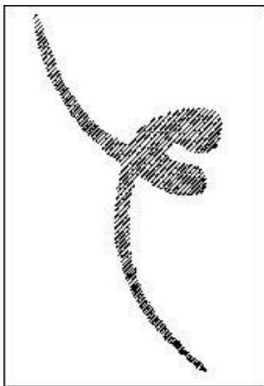
Рис.1 Галактические хвосты (NGC 4038 and 4039)
