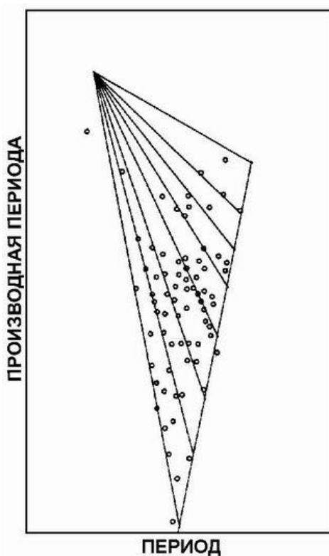
Рис. 24 ПЕРИОДЫ ПУЛЬСАРА
