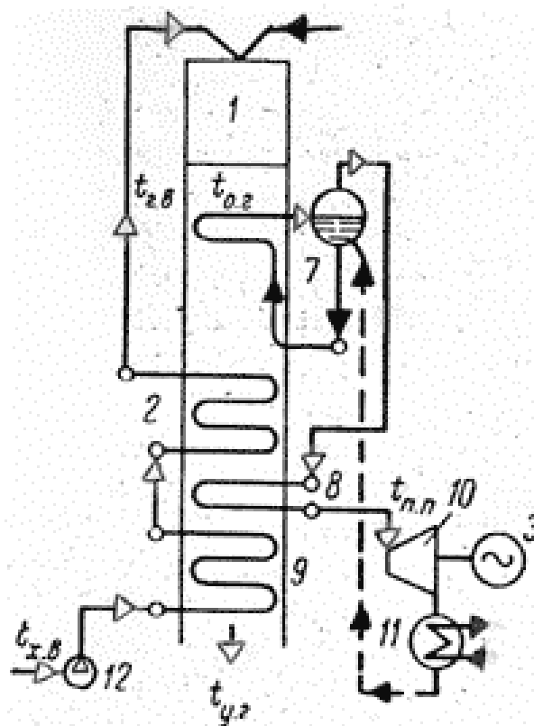
Рис. 6.2. Схема ПТУ на теплоте отходящих газов:
