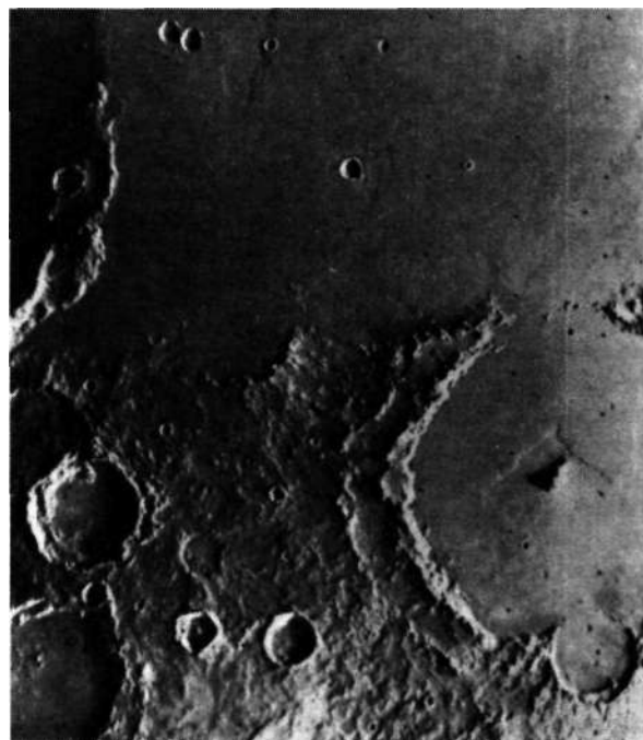
Рис. 4.15. Обильные излияния вулканических лав привели к затоплению обширных районов на расстояниях до 1500 км от вулкана. Участок поверхности выше и левее кратера Пикеринг (справа, диаметр 120 км) и само дно кратера подверглось затоплению при извержениях вулкана Арсия. Снимок NASA
