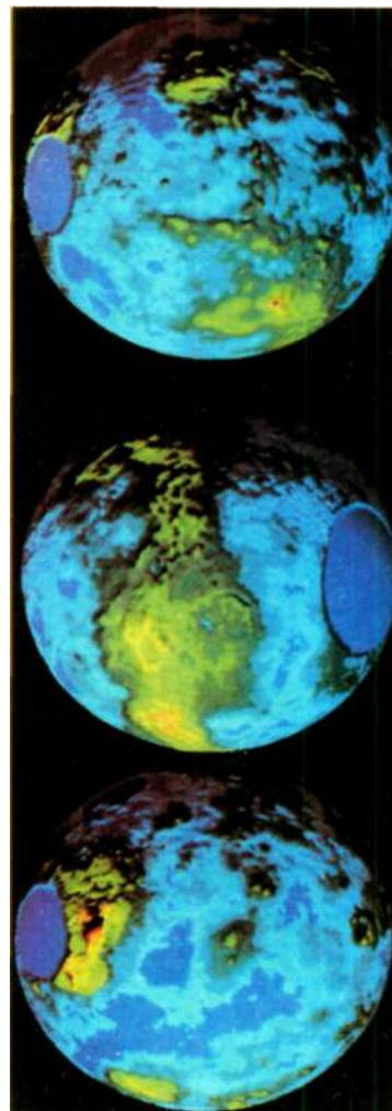
Фото 7. Вид глобуса Венеры в трех положениях: слева — с долготой центрального меридиана 0 (в центре — область Альфа), в середине — с долготой 150°, справа — 240° (левее и ниже центра земля Афродиты с каньоном Артемиды). Глобус представляет собой компьютерную программу с банком данных радиосальтиметрии «Пионер-Венера» и позволяет вызывать на экран любую проекцию. В области северного и южного полюсов (темно-синие овалы) данных тогда не было. Из работы Дж.Блинна и др.
