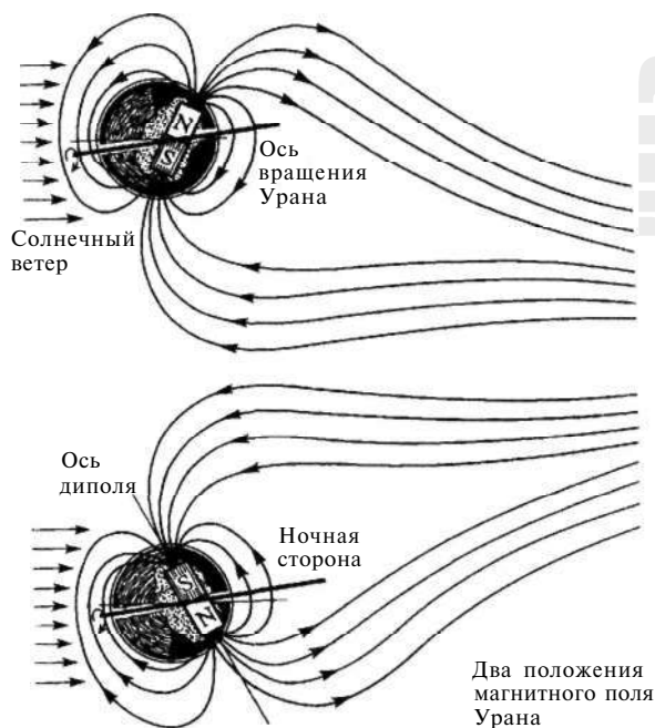
Рис. 7.1. Магнитное поле Урана имеет сложную структуру. Очень приблизительно его можно считать дипольным, если ось диполя сместить от центра на 1/3 радиуса и наклонить к оси вращения на 60^\circ
