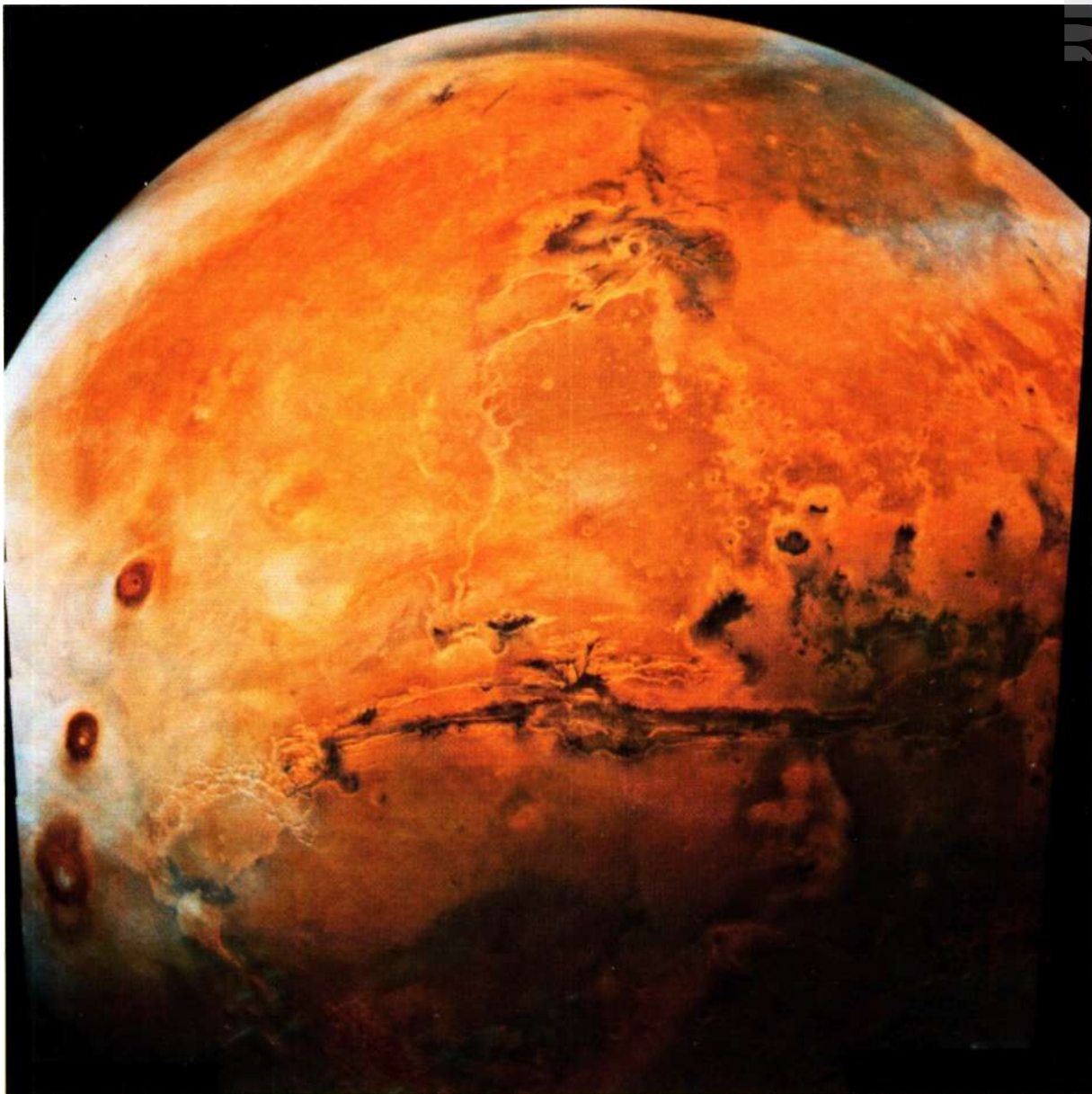
Фото 14. Более подробные изображения получены последующей обработкой. Марс в двух положениях; с долготой центрального меридиана около 75^{\circ} (слева) и 180^{\circ} (справа)
