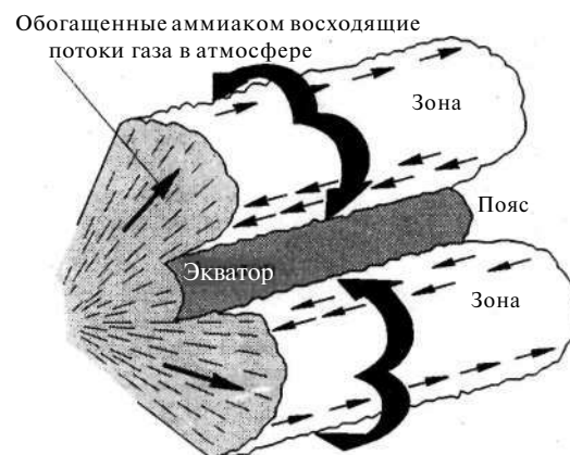
Рис. 5.2. Структура поясов и зон Юпитера и, возможно, Сатурна. Зоны представляют собой облачную «крышу» восходящих более теплых потоков, пояса — холодные районы нисходящих потоков. Благодаря действию кориолисовых сил потоки вытягиваются в долготном направлении
