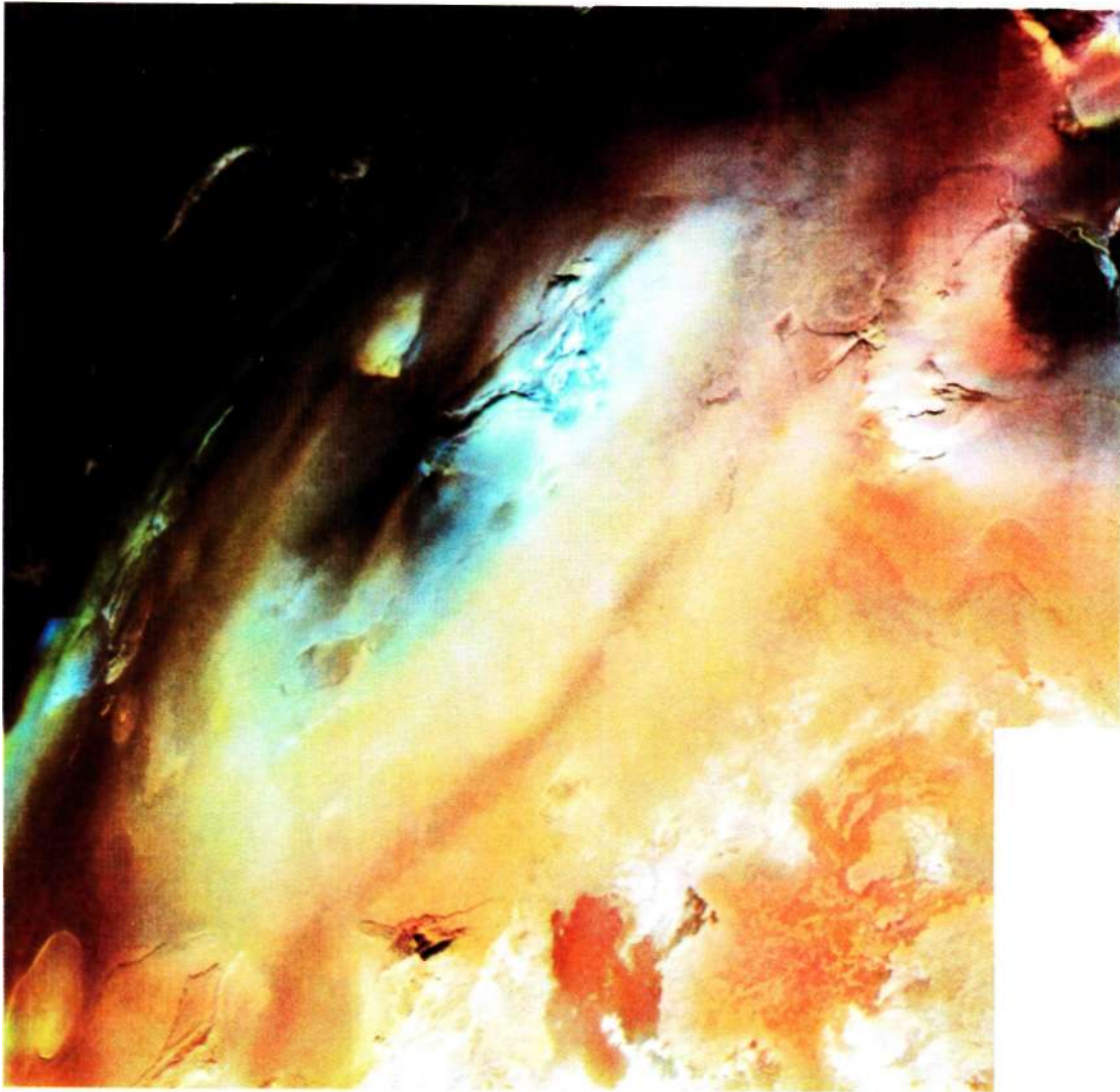
Фото 43. Извержение вулканического комплекса Пеле. Газовый султан, сквозь который видны средняя и верхняя части снимка, поднимается над поверхностью на 280—300 км. Из работы А.Мак-Ивена и Л.Солербома
