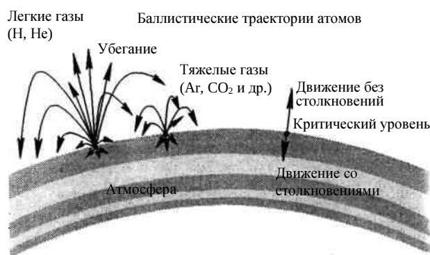
Рис. 3.10. Потери водорода («убегание» с критического уровня) для Венеры и Земли
