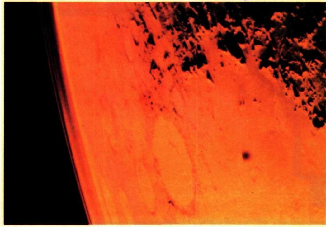
Фото 26. Снимок, полученный с орбитального аппарата «Викинг-1» в условиях необычайно высокой прозрачности атмосферы, показывает детали равнины Аргир. Заметна белая морозная мгла над южным полярным районом, где в этот период была середина зимы. Два слоя тонких облаков на высоте от 25 до 40 км, по-видимому, состоят из кристаллов сконденсированного углекислого газа. Снимок NASA
