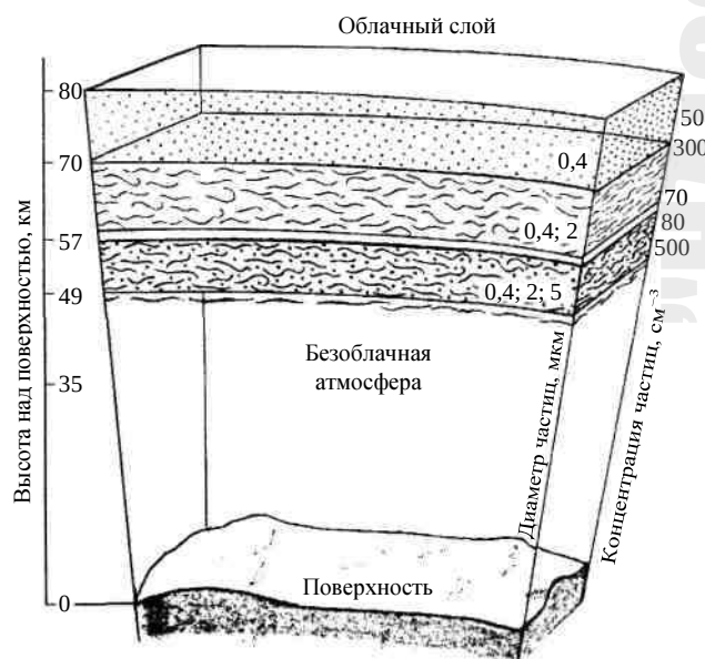
Рис. 3.13. Схема строения туманоподобных облаков Венеры. Облака состоят из трех слоев, отличающихся размерами и концентрацией частиц. Под нижней границей облачного слоя (49 км над поверхностью) аппараты «Пионер—Венера» и «Венера-13, -14» обнаружили слоистые образования, похожие на земные перистые облака
