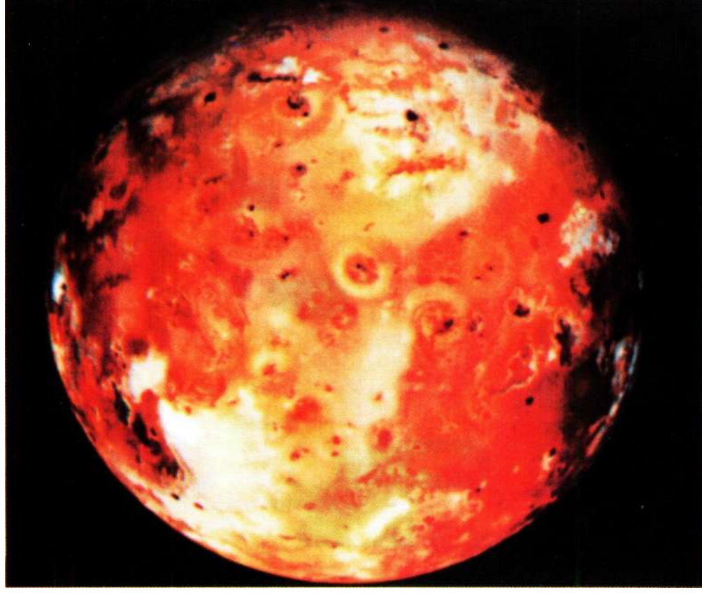
Фото 42. Ио — спутник, поверхность которого образована конденсацией продуктов постоянных вулканических извержений. В извержениях выбрасываются главным образом газообразная двуокись серы. Извержения можно видеть на этом снимке в виде неправильного туманного кольца в центре и таких же колец ниже и выше центра изображения. Снимок NASA
