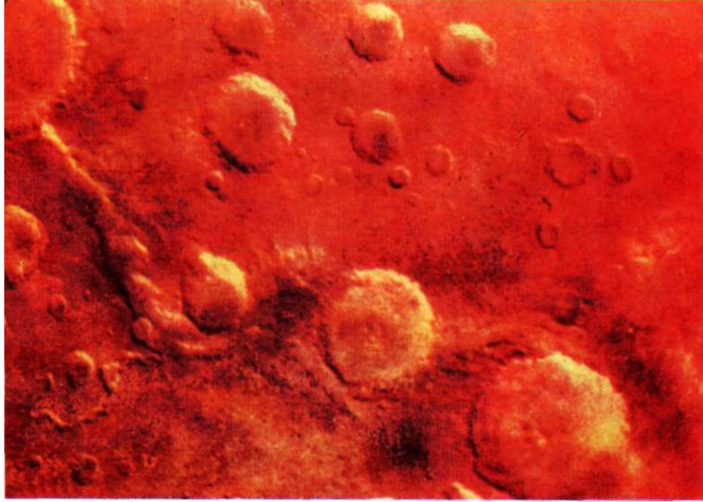
Фото 18. Снимок района Эритрейского моря. Большие кратеры, вытянутые цепью 800 км, вероятно, когда-то образовывали единое водохранилище, в которое впадала древняя река Нертал (слева вверх). Снимок «Марса-5»
