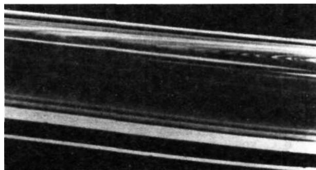
Рис 6 7 Вид колец за 88 с до пересечения аппаратом их плоскости. На первом плане — кольцо F постоянной ширины, за ним — кольцо А и деление Энке. Самое дальнее — удаленная часть кольца А. Светлые вытянутые детали — спокы. Слева — схема изображения. Снимок NASA
