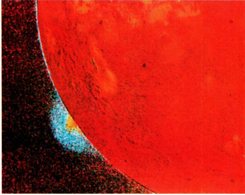
Фото 41. Извержение над лимбом Ио. Газовые потоки над извержением поднимаются на высоту до нескольких сотен километров. Снимок NASA
