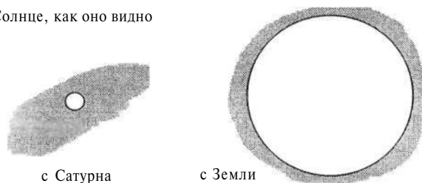
Рис. 6.3. Сравнительные угловые размеры Солнца, видимого с Сатурна (слева) и с Земли. Если рассматривать рисунок с расстояния 3,5 м, угловой диаметр изображения будет равен углу, под которым видно Солнце
