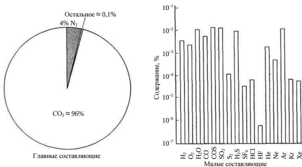
Рис. 3.9. Состав атмосферы Венеры. Справа — малые составляющие
