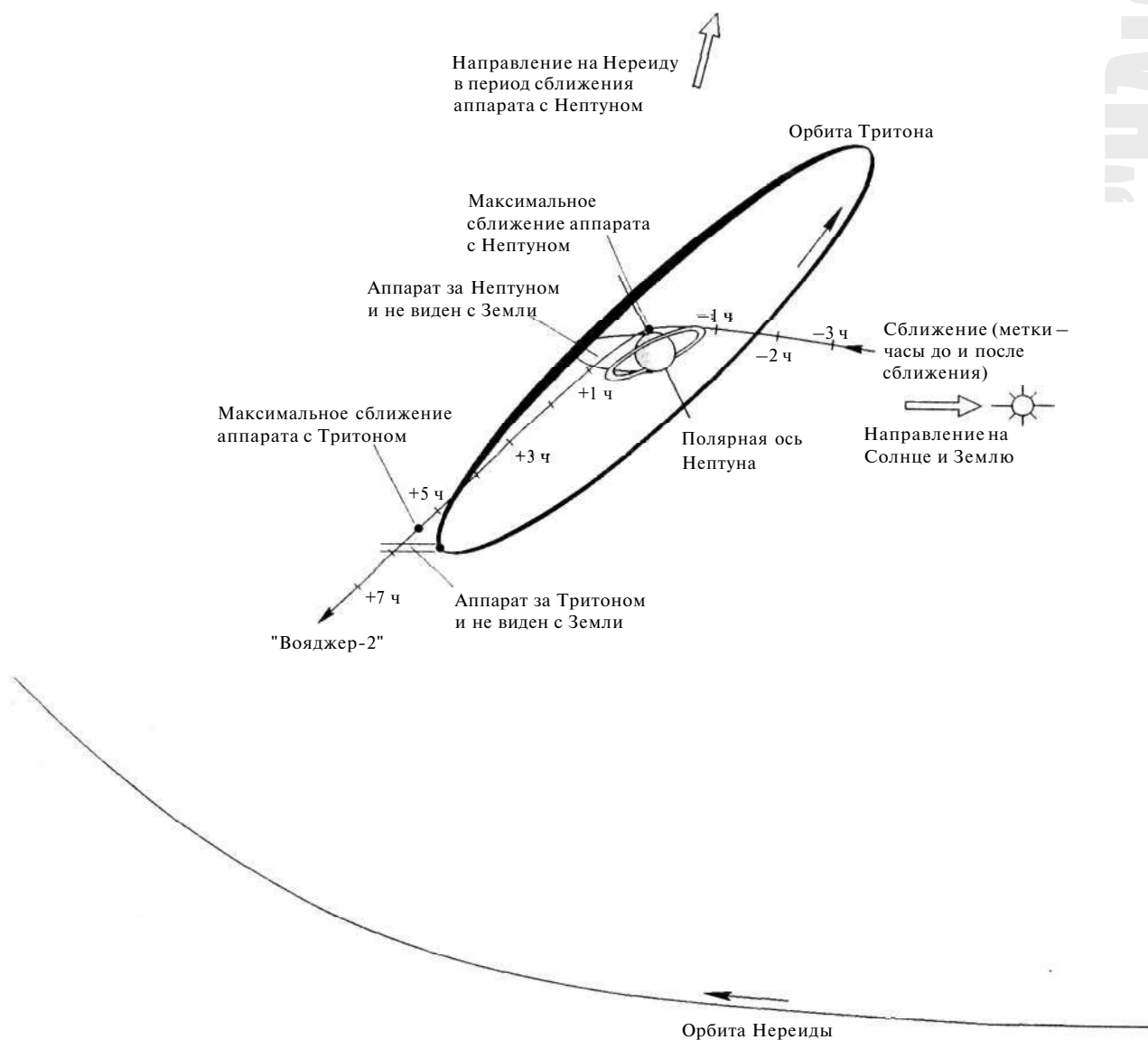
Рис. 8.1. Схема сближения «Вояджера-2» с Нептуном
