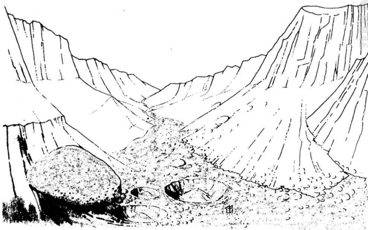
Рис. 4.20. Такой вид когда-нибудь откроется космонавтам, опустившимся на дно каньона
