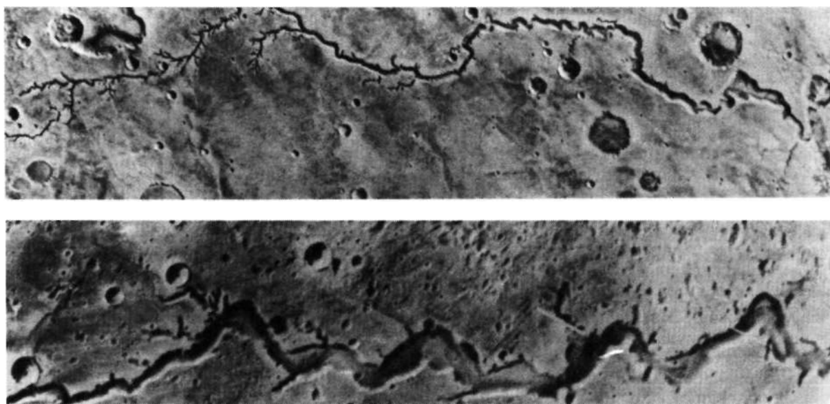
Рис. 4.21. Вверху: сухое русло древней марсианской реки Нергал с притоками (долина глубоко прорезает лавовую равнину). Полная ее длина около 400 км. Внизу: долина Маадим длиной около 700 км. В средней ее части видна тонкая, более поздняя долина. Маадим находится в южном полушарии и вытянута вдоль меридиана 187° от 29 до 14° ю.ш., где соединяется с большим кратером. Снимок NASA
