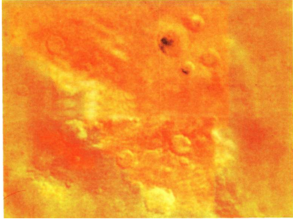
Фото 21. Район горного края высотой 9 км в области Тавмасия — Босфорское плато. На снимке видны темные и светлые кратеры и голубоватые неплотные конденсационные облака над вершинами. Склоны очень пологие, поэтому резких теней нет. Снимок «Марса-5»
