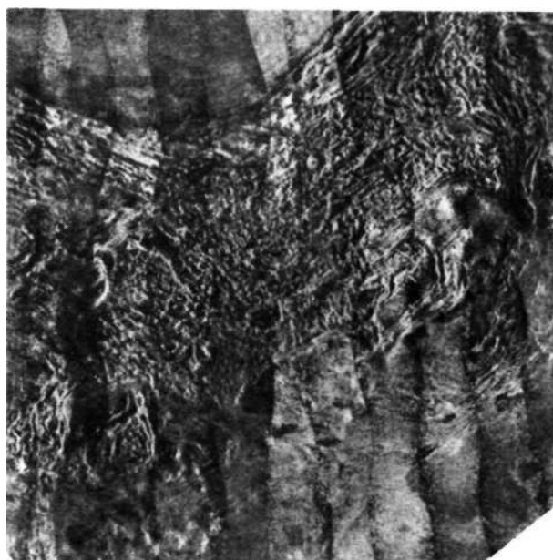
Рис. 3.41. Уступ Весты и уступ Ут (в нижней части рисунка). Из работ А.Базилевского, О.Ржиги и др.
