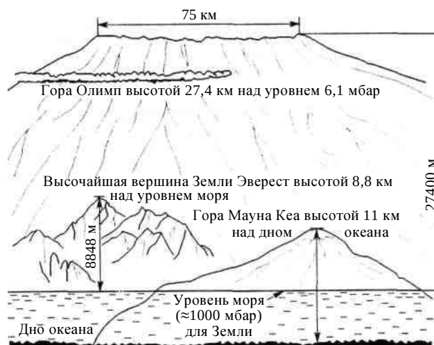
Рис. 4.14. Сравнительная схема высот горы Олимп и Эвереста
