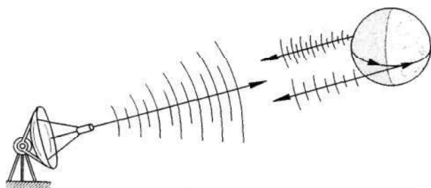
Рис. 2.2. Схема радиолокации Меркурия. При отражении радиоволн вследствие вращения планеты возникают различия в доплеровских сдвигах сигналов. Частота сигнала, отраженного движущимся на наблюдателя краем планеты, несколько возрастает, а отраженного удаляющимся краем — убывает
