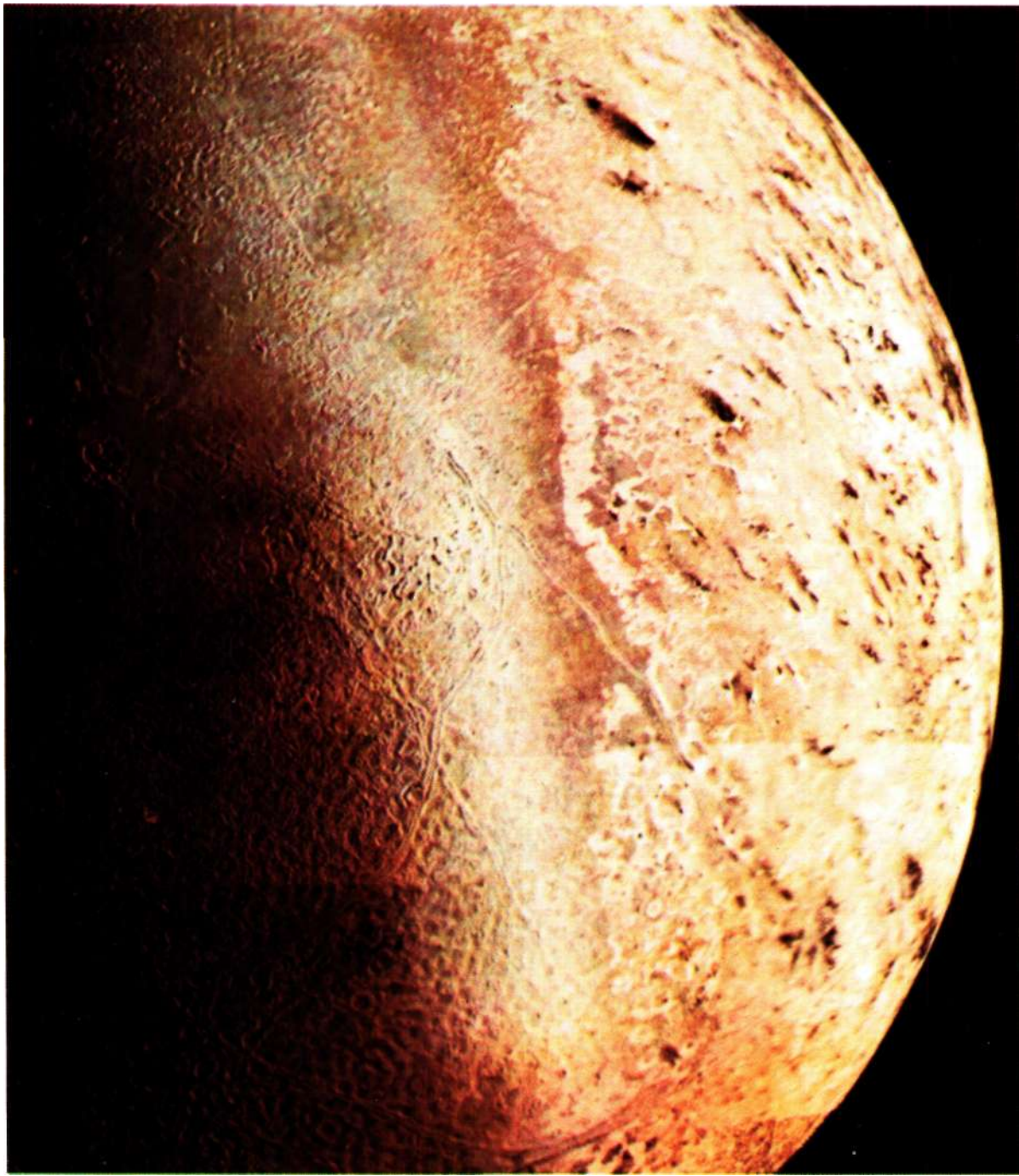
Фото 75. Мозаика поверхности Тритона (внизу — южный полюс). Снимок NASA
