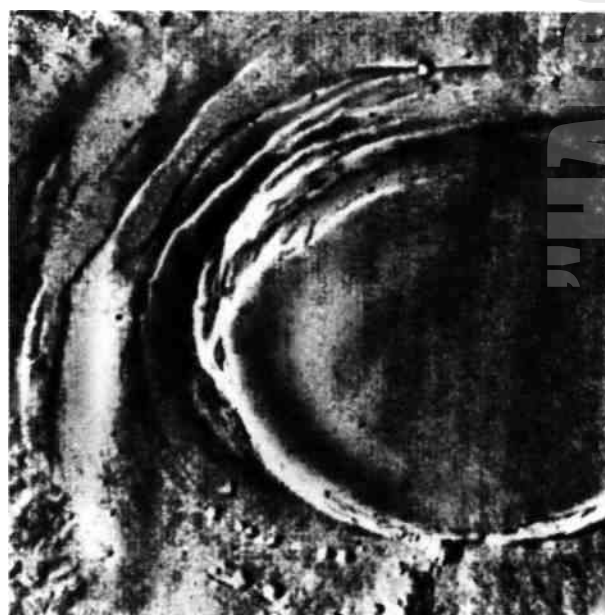
Рис. 4.13. Огромная вулканическая кальдера диаметром 130 км венчает вершину горы Арсия — древнего и давно не действующего вулкана. Снимок NASA
