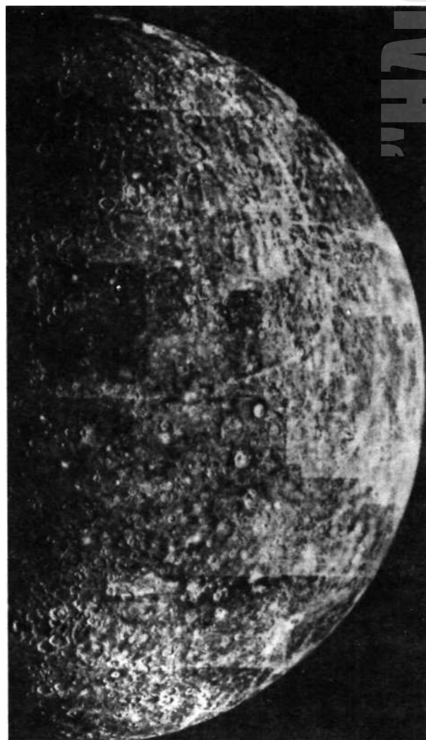
Рис. 2.8. Другая часть того же полушария Меркурия. Угол фазы около 78°. Кроме кратеров с лучами на этом снимке в центре, на терминаторе видно единственное известное пока на Меркурии море — Равнина Жары. Снимок NASA
