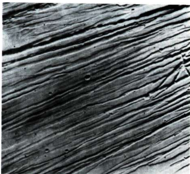
Рис. 4.12. Узкие Керавнские борозды в северной части Фарсиды. Вертикальный размер снимка около 100 км. Снимок NASA
