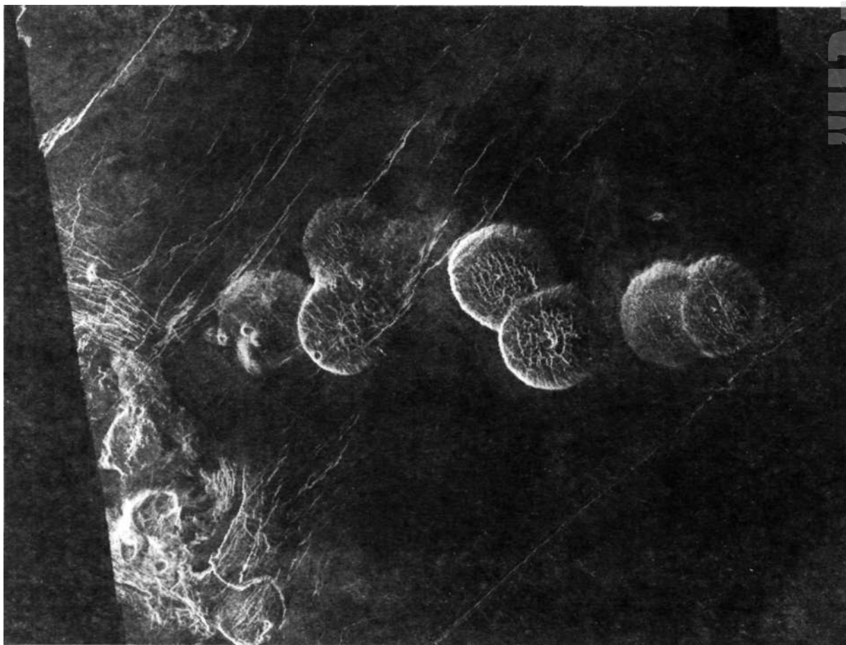
Рис. 3.34. Семь круглых холмов диаметром около 25 км и высотой немного меньше километра, расположенные в точке 30° ю.ш., 11,8° в.д. на равнине вблизи области Альфа, были определены как очень толстые и медленно растекающиеся лавовые потоки. Подобные образования известны и на Земле. Снимок NASA
