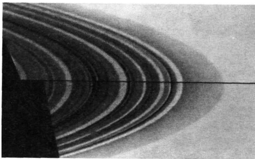
Рис. 6.9. Асимметричное узкое колечко в кольце С. Чтобы продемонстрировать его эксцентricность, здесь сложены две противоположные половинки снимка. Снимок NASA
