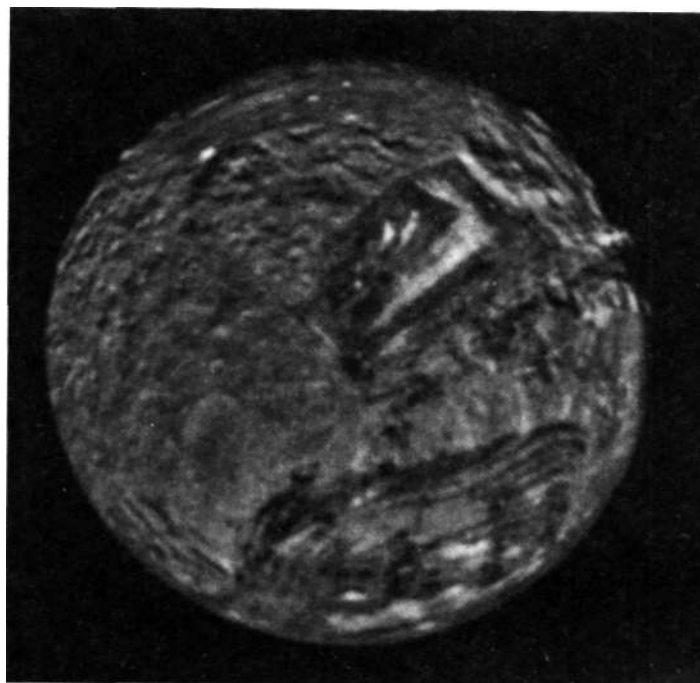
Рис. 7.5. Обработанная мозаика снимков Миранды. Два «стадиона» выше и ниже «шеvrona» размером 250—300 км в длину. Снимок NASA
