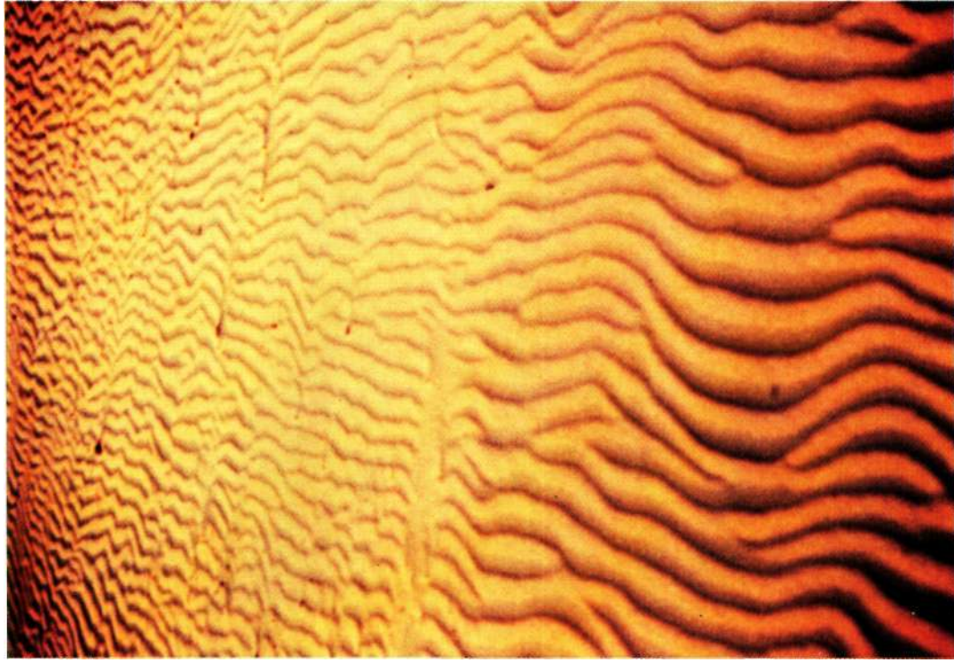
Фото 20. Мелкие дюны, которые образуются под действием ветра на песчаном берегу Юрмалы (слева) и гигантские дюны земных пустынь (справа)
