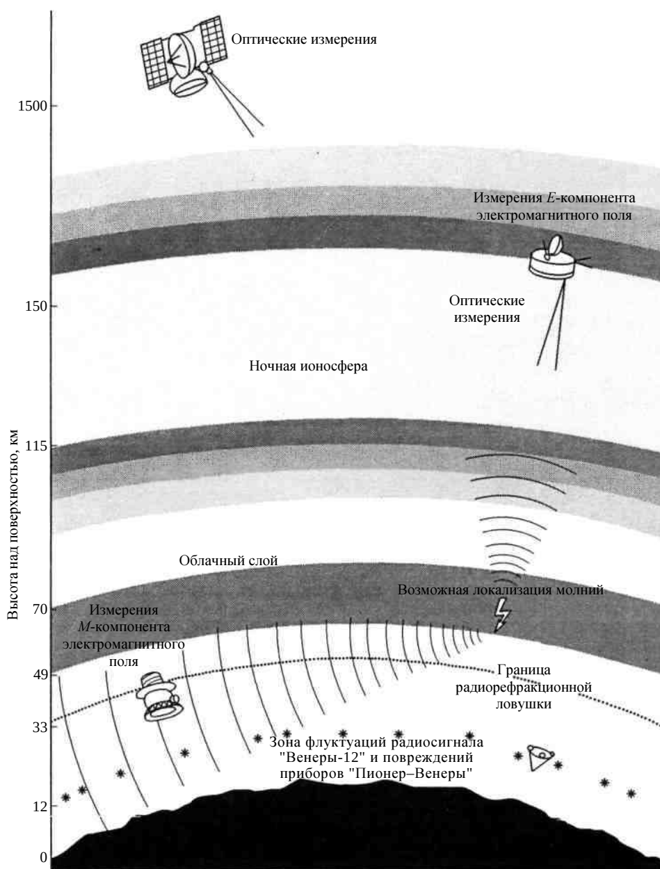
Рис. 3.51. Схема, обобщающая наблюдения электрических явлений в атмосфере Венеры. Кроме электромагнитных импульсов молнии в облаках должны создавать световые вспышки. Импульсы были обнаружены, вспышки — нет. Спускаясь в атмосфере, зонды аппарата «Пионер—Венера» испытали неизвестное электрическое воздействие на высоте около 12 км
