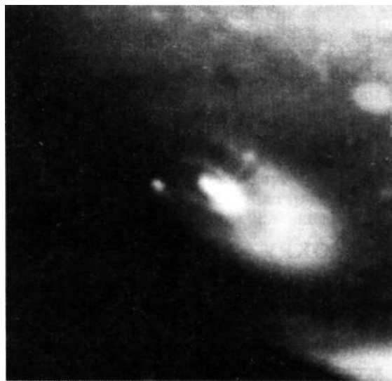
Рис. 5.24. Тот же объект, что и на рис. 5.23. Снимок сделан в полосе метана. Снимок Группы телескопа «Хаббл» и NASA
