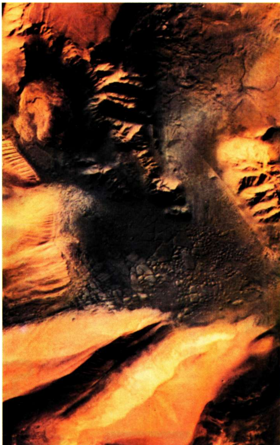
Фото 23. Каньон Кандор (часть долины Маринера). Площадь приведенного на снимке района 190 \times 225 км. Из работы А.Мак-Ивена
