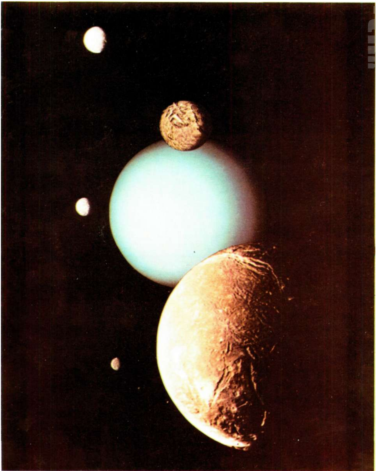
Фото 70. Семейство крупных спутников Урана: на первом плане — Ариэль, над ним — Миранда, слева (сверху вниз) — Титания, Оберон, Умбриэль. Фотомонтаж NASA
