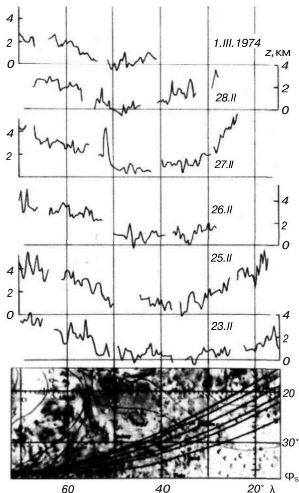
Рис. 4.22. Измерения рельефа вблизи долины Узбой, выполненные с «Марса-5», указывают на плавное понижение на несколько километров в сторону долины. Внизу показаны 6 трасс «Марса-5», пересекавшие район Нергал—Холден—Хейл
