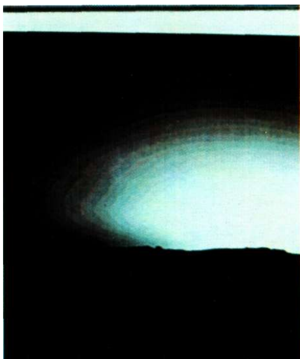
Фото 31. Ночь спускается на равнину Хриса. Снимок NASA
