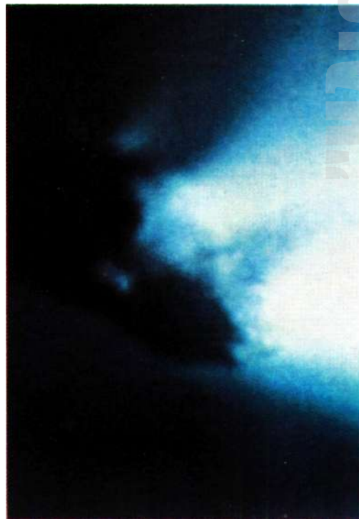
Фото 76. Слева — комбинированный снимок ядра кометы Галлея (с повышенной контрастностью), наложенного на первичное изображение выбрасываемых из ядра газовых фонтанов (снимок с аппарата «ВЕГА-2», обработка Института космических исследований РАН). Справа — другая сторона ядра кометы Галлея (аппарат «Джотто», снимок и обработка Европейского космического агентства)
