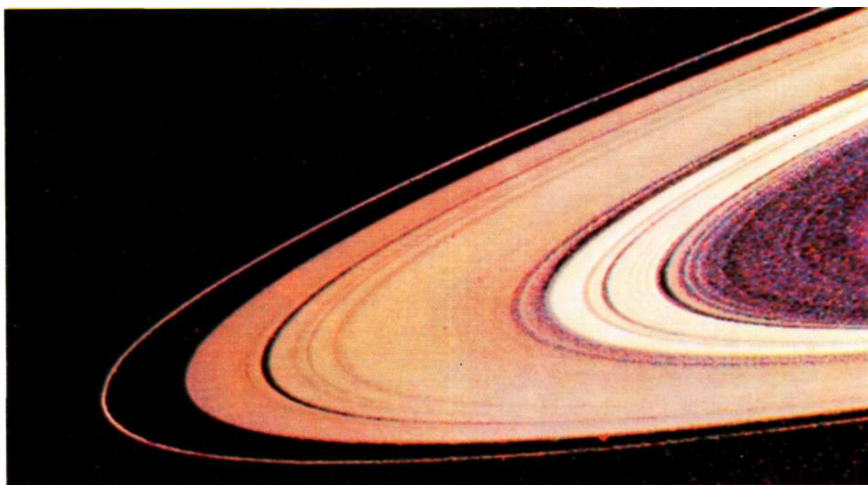
Фото 61. Кроме ярких кольца и деления Кассини, на снимке хорошо видно кольцо F — тонкая линия вдоль внешнего края кольца A. Условные цвета отражают распределение размеров частиц. Снимок NASA
