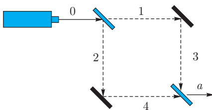
Рис. 7.2. Интерферометр Маха – Цандера выпускает фотоны только по одному направлению из двух возможных.
